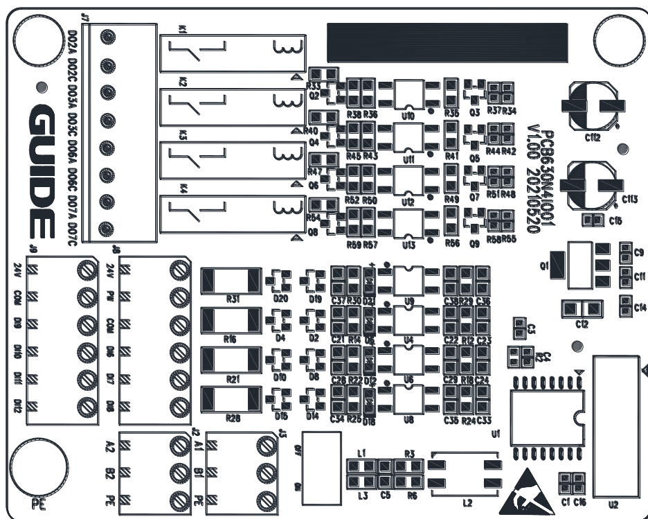
GDHF-AMBX1 通讯卡布局图
