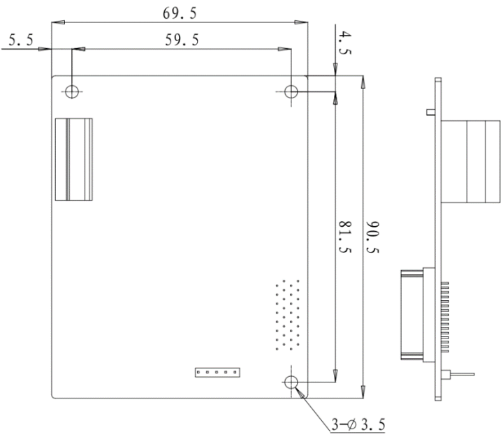
GDHF-ACNX1 通讯卡尺寸（单位 mm）
