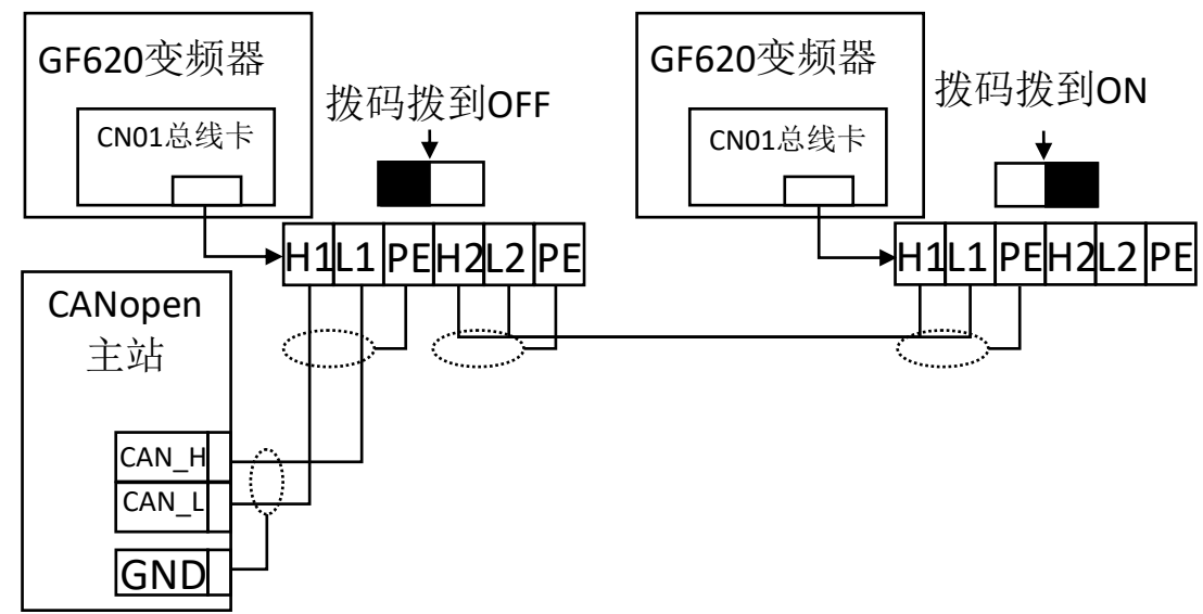
标准 CANOpen 电缆接线图
