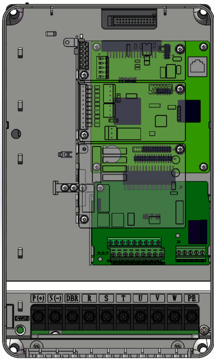
GF620 控制板安装位置示意图
