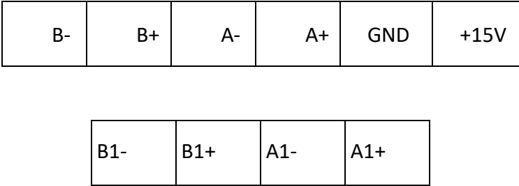
接线端子示意
