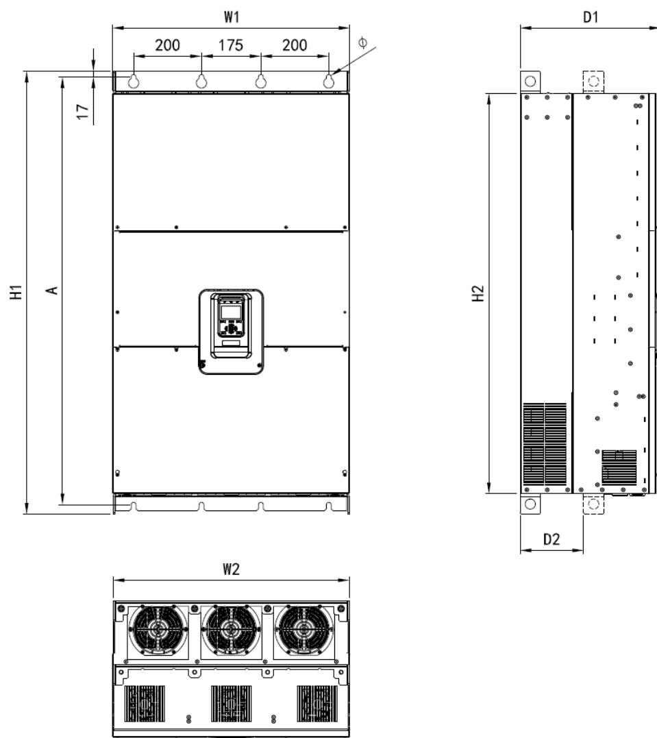
N10 机型尺寸及安装尺寸示意图
