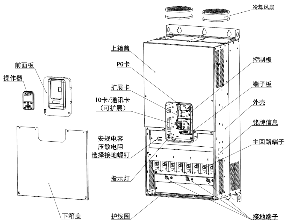
N8 产品部件示意图（三相 380V~480V，185kW~220kW）
