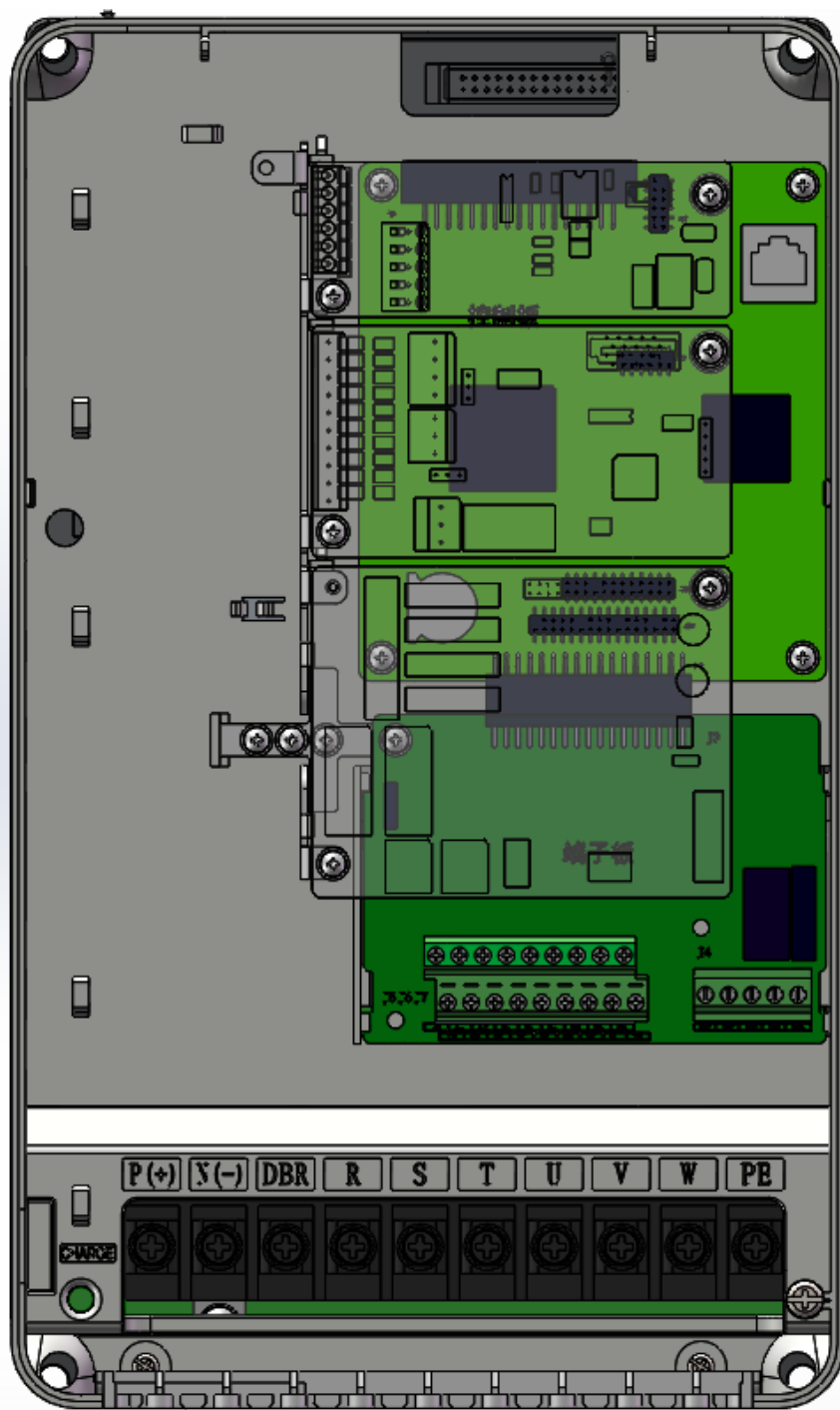
GF600 控制板安装位置示意图
