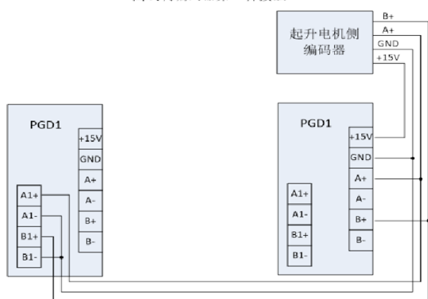
四线制编码器第一种接法
