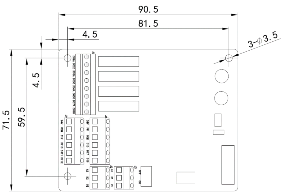
IO 扩展卡选件 GDHF-AIOX1 尺寸 (单位 mm)
