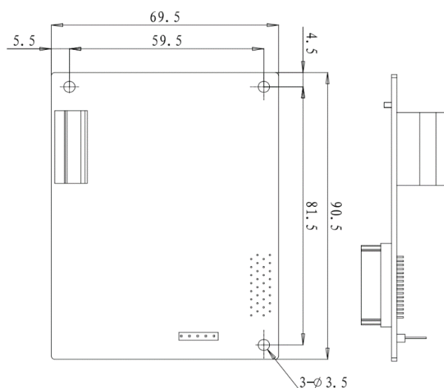
GDHF-ACNX1 通讯卡尺寸 (单位 mm)
