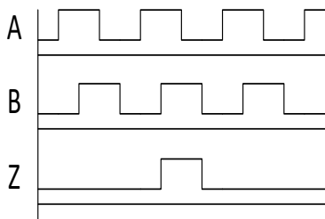
编码器单端输出信号
