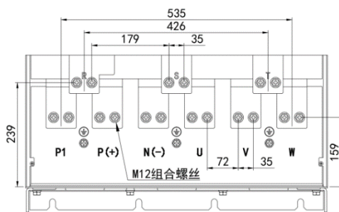
N10 主回路端子分布图
