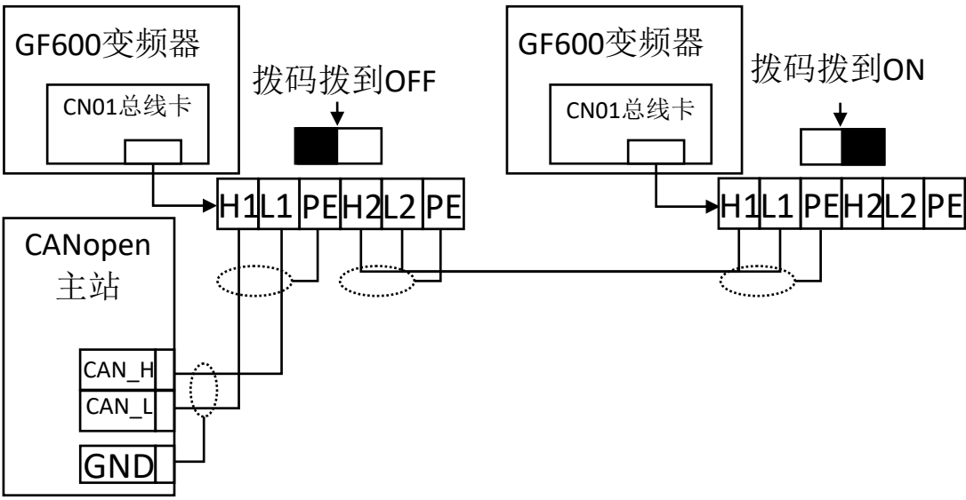
标准 CANOpen 电缆接线图
