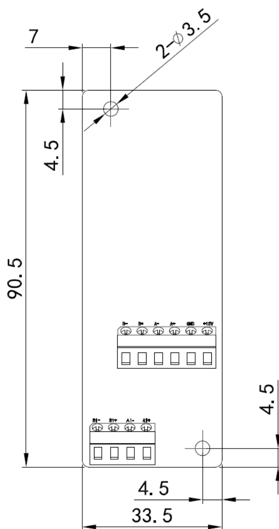
PG 卡安装示意图及 PG 卡外形尺寸
