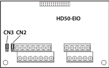
图 8-2 跳线位置
