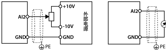
图 4-8 AI2 端子接线
