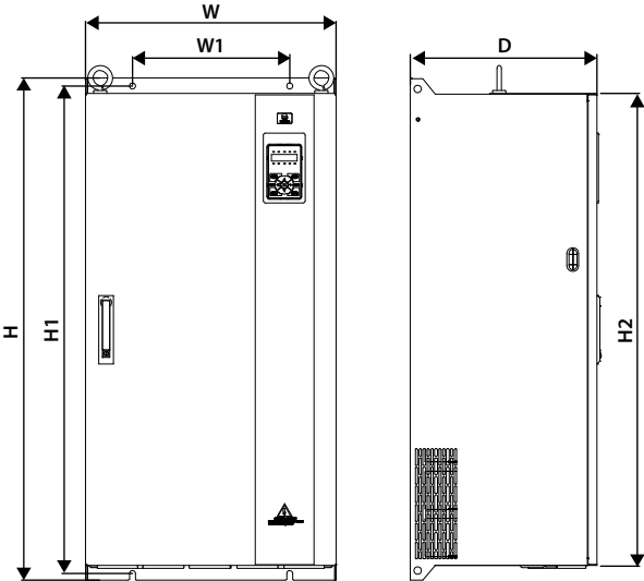
Frame15 – Frame16 外形图
