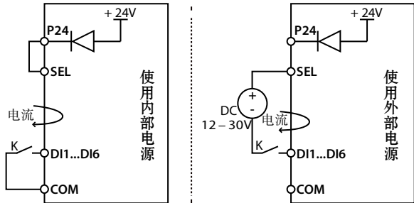
图 4-4 干接点时 DI 端子接线
