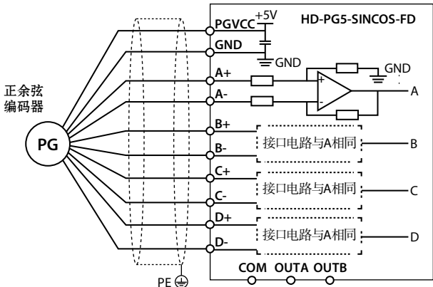
图 4-21 正弦编码器接线图
