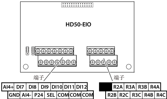
图 8-1 端子
