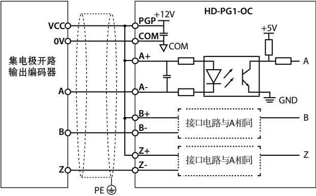
图 4-14 集电极开路输出编码器接线图
