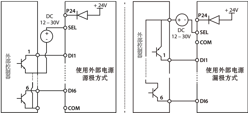
图 4-5 使用外部电源时 DI 端子接线
