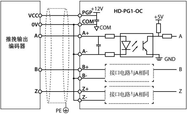
图 4-15 推挽输出编码器接线图
