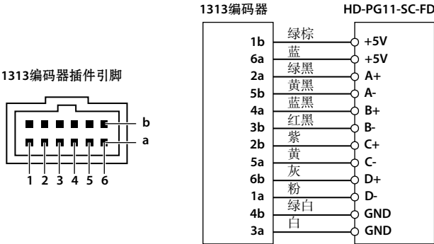
图 4-29 与海德汉 1313 编码器接线图
