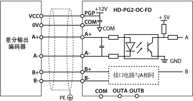
图 4-17 差分输出编码器接线图
