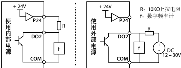
图 4-10 DO2 端子接线
