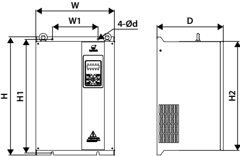
Frame12 – Frame14 外形图
