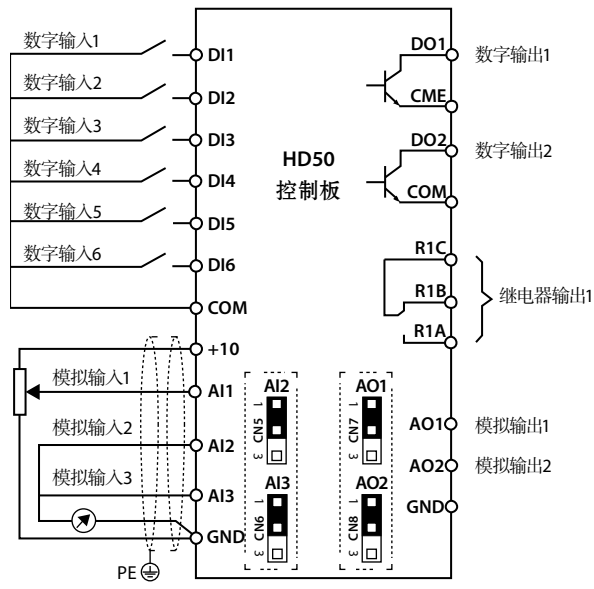
图 4-3 HD50 控制板接线图
