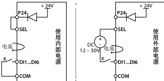
图 4-4 干接点时 DI 端子接线
