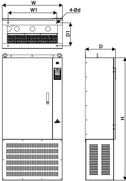
Frame8 – Frame10 (带-C) 柜机外形图
