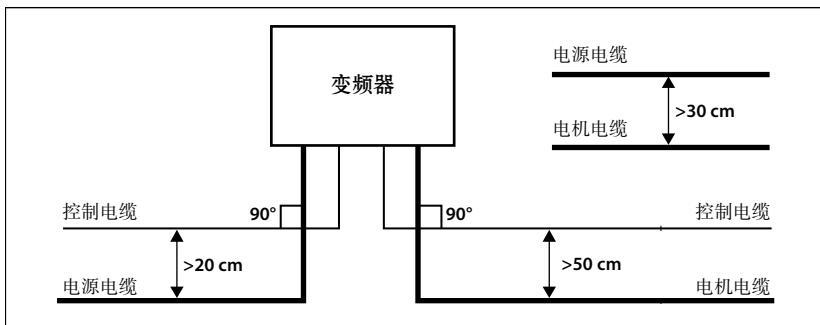
图 4-12 系统配线要求
