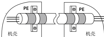
图 4-13 屏蔽电缆连接示意图
