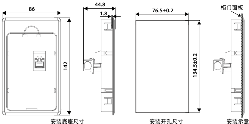
图 8-6 外引安装底座尺寸及开孔尺寸
