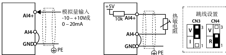
图 8-3 AI4 端子接线
