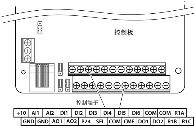
图 4-2 控制端子
