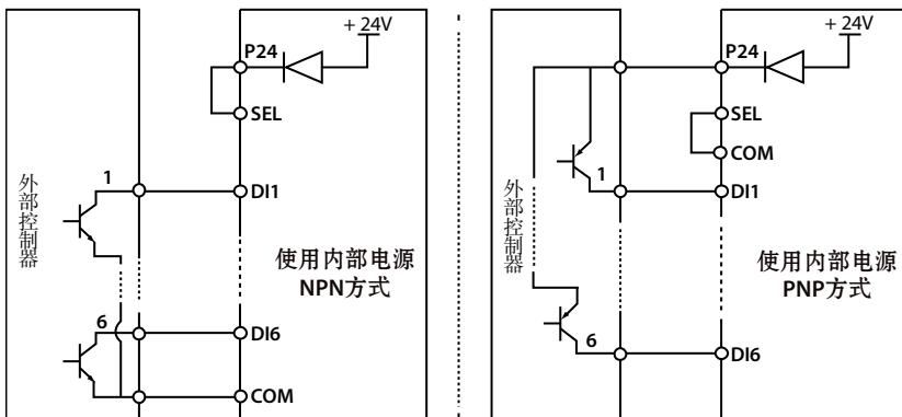
图 4-6 使用内部 24V 电源时 DI 端子输入接线
