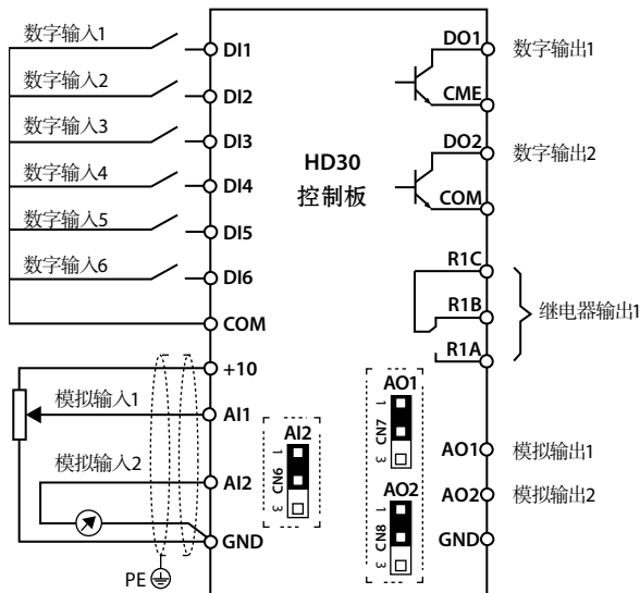
图 4-3 HD30 控制端子接线图
