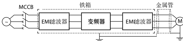
图 4-16 射频干扰措施
