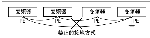
图 4-15 禁止的接地方式
