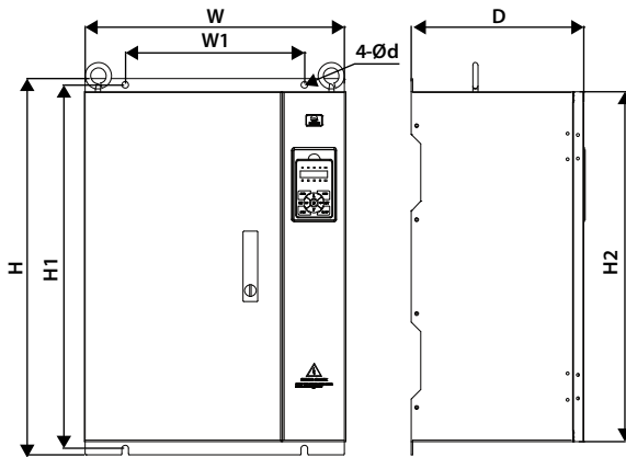
Frame7 – Frame10 外形图
