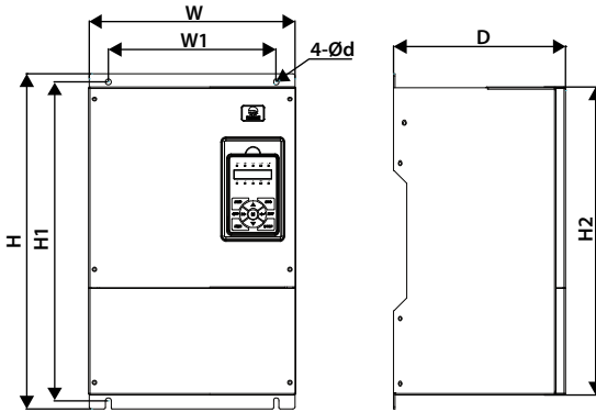
Frame5 – Frame6 外形图
