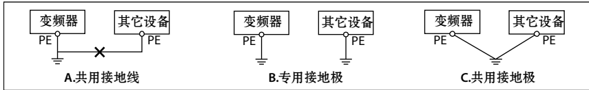
图 4-14 推荐的接地方式
