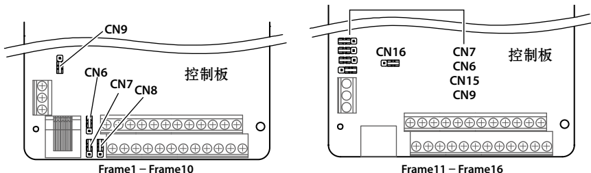
图 4-1 跳线位置
