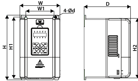
Frame1 – Frame4 外形图
