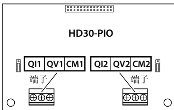
图 8-4 端子
