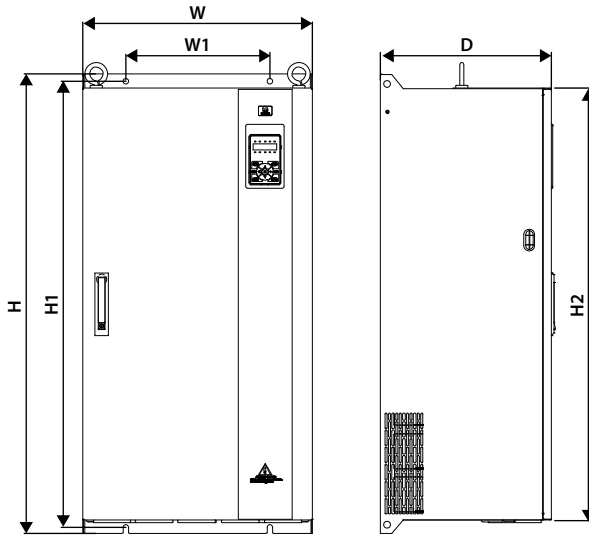
Frame15 – Frame16 外形图
