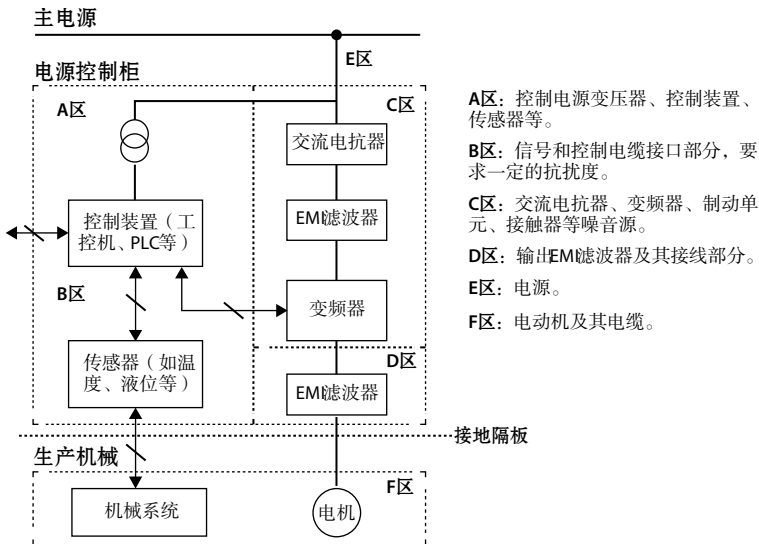
图 4-11 系统配线区域划分示意图
