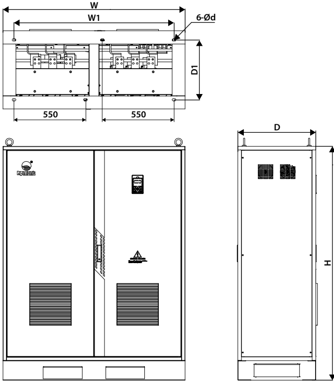
Frame11 外形图
