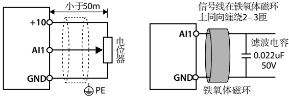
图 4-8 AI1 端子接线
