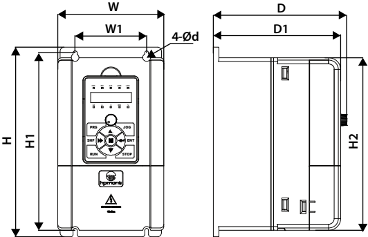
图 3-3 HD20 外型图
