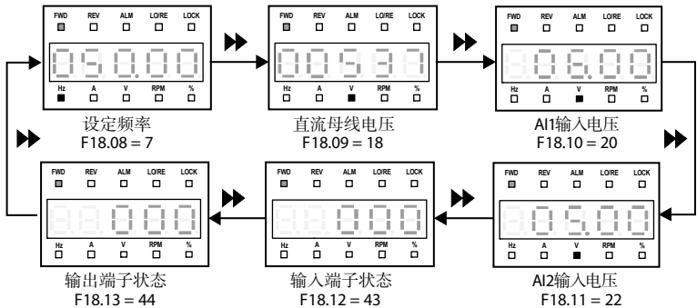
图 5-7 停机状态参数切换显示
