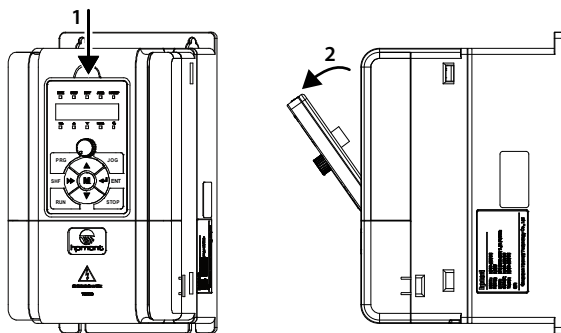
图 3-5 操作面板的拆卸
