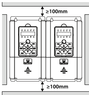
图 3-1 变频器并排安装
