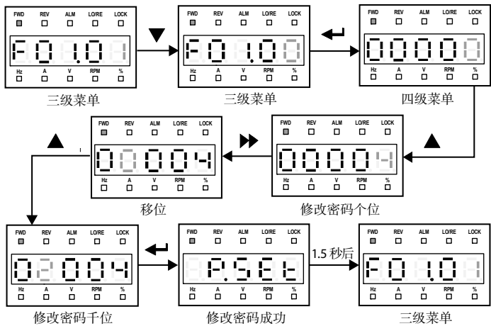
图 5-9 用户密码修改
