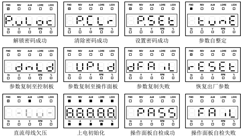
图 5-4 特殊显示状态
