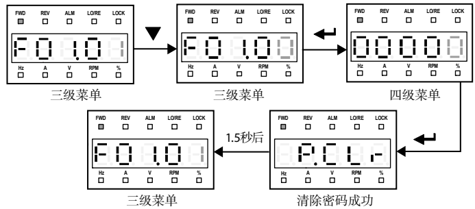
图 5-10 用户密码清除
