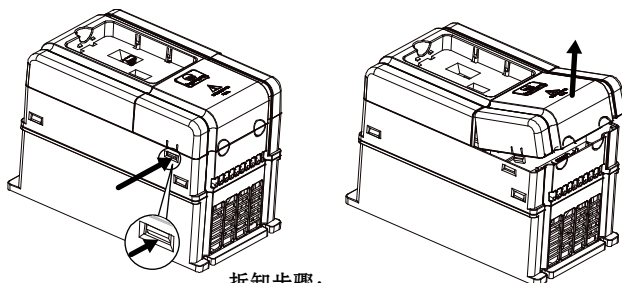
图 3-6 端子盖板拆卸示意图
