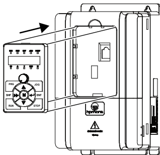
图 3-4 操作面板的安装
