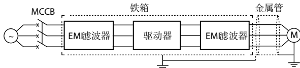
图 4-17 射频干扰措施
