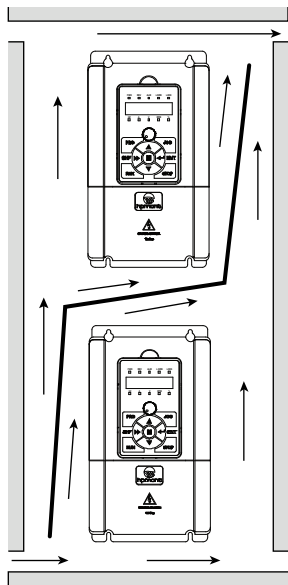
图 3-2 多台变频器上下安装
