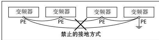
图 4-16 禁止的接地方式
