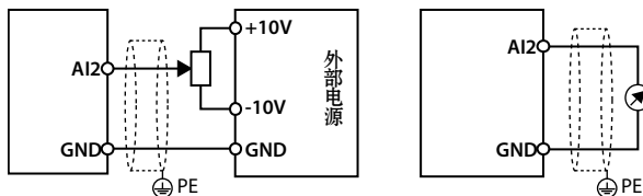
图 4-9 AI2 端子接线
