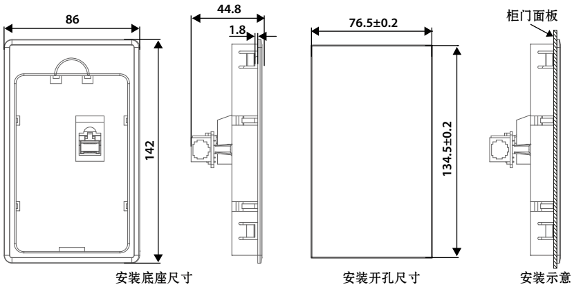
图 8-1 外引安装底座尺寸及开孔尺寸
