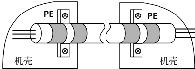
图 4-14 屏蔽电缆连接示意图
