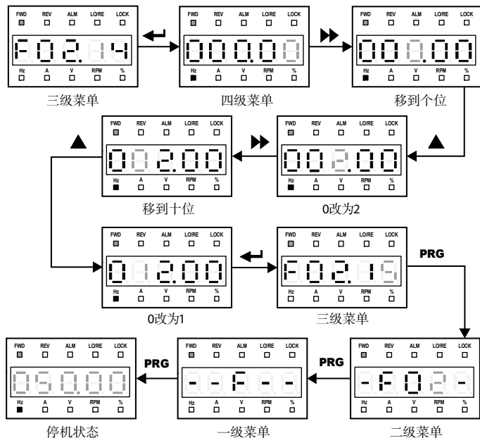
图 5-6 功能参数设置
