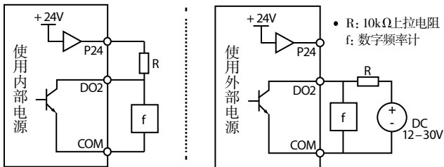
图 4-11 DO2 端子接线
