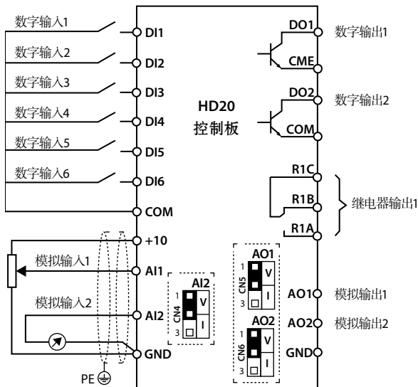
图 4-4 HD20 控制板接线图
