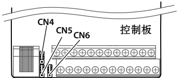
图 4-3 跳线位置
