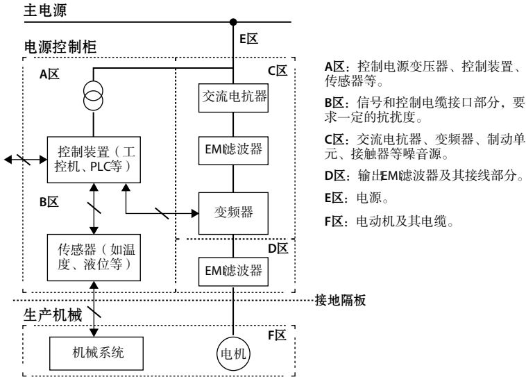
图 4-12 系统配线区域划分示意图
