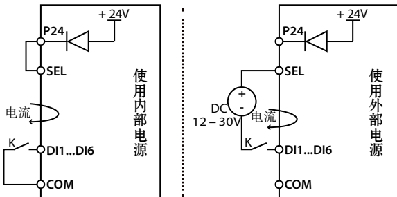
图 4-5 干接点时 DI 端子接线
