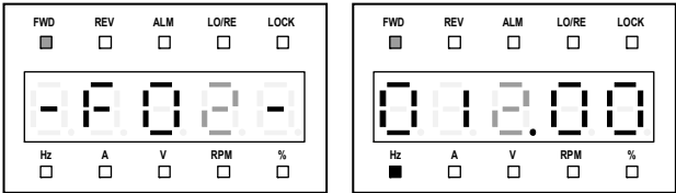
图 5-2 参数编辑状态
