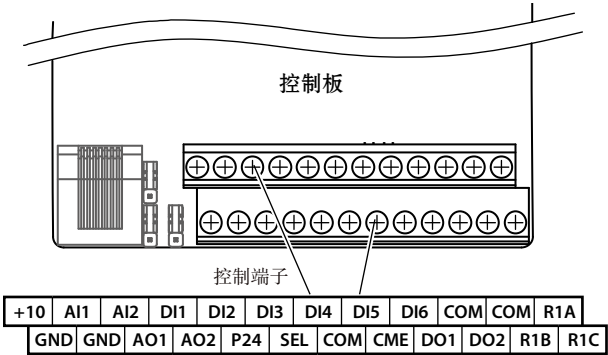
图 4-2 控制端子
