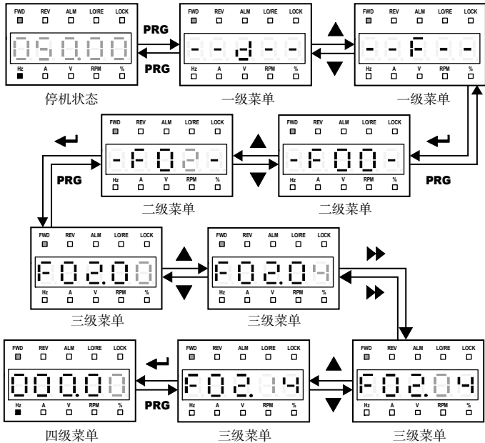
图 5-5 四级菜单操作流程图
