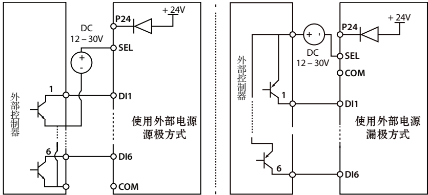
图 4-6 使用外部电源时 DI 端子接线
