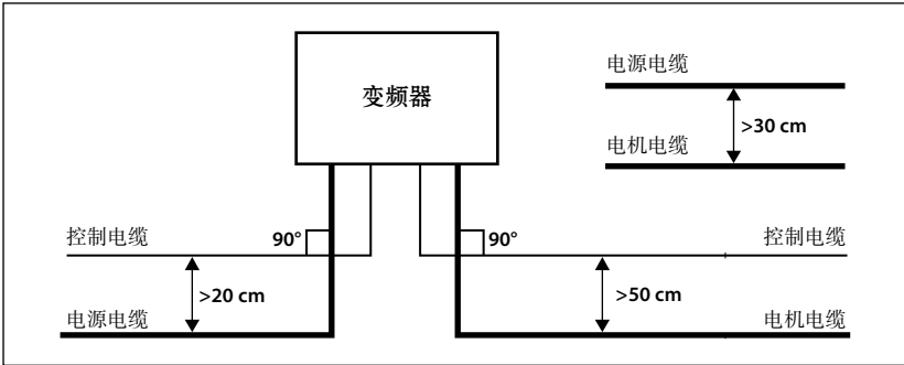
图 4-13 系统配线要求
