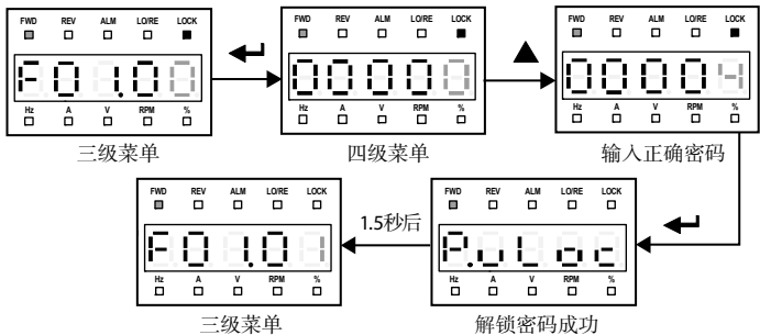
图 5-8 用户密码解锁
