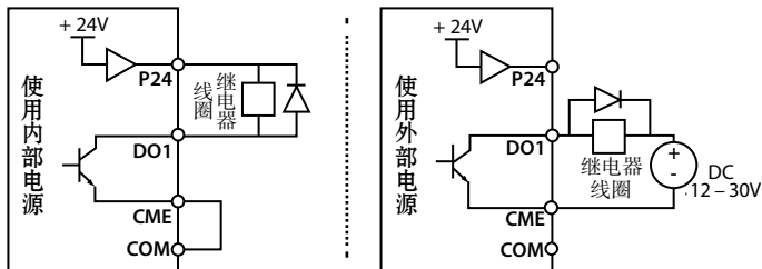
图 4-10 DO1 端子接线
