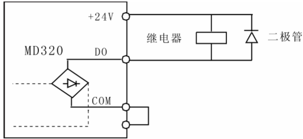
图 3-16 数字输出端子接线示意图
