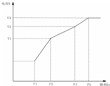
图 6-4 V/F 曲线设定示意图
