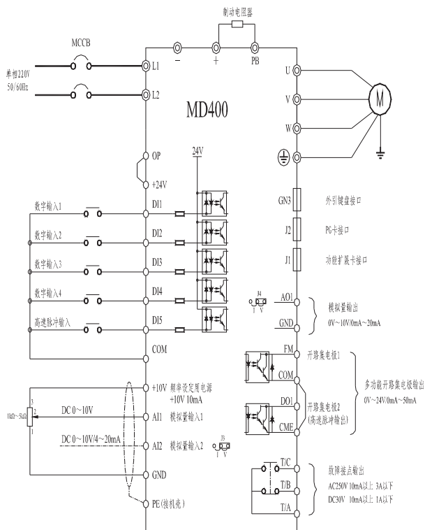
图 3-5 单相变频器接线示意图
