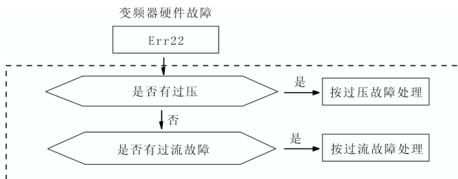
图 8-21 变频器硬件故障 (Err22)
