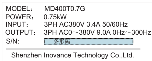
图 2-2 铭牌
