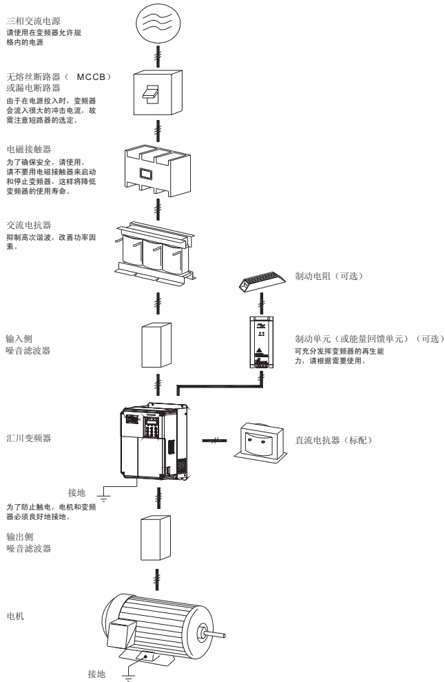
与外围机器的连接示例
