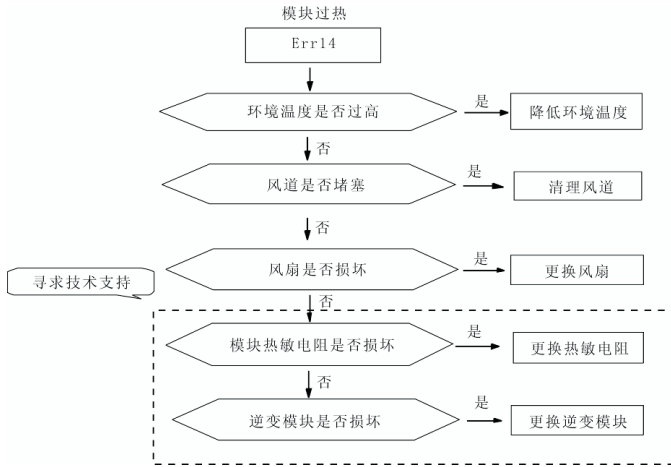
图 8-13 模块过热 (Err14)
