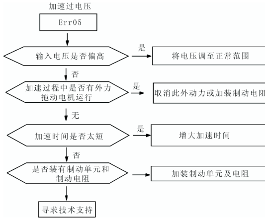
图 8-5 加速过电压（Err05）
