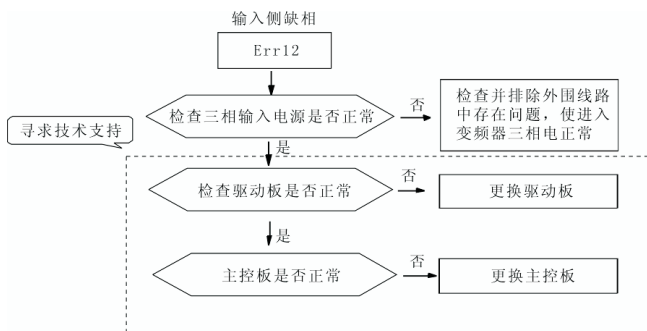
图 8-11 输入侧缺相 (Err12)
