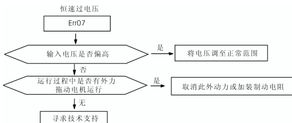
图 8-7 恒速过电压 (Err07)
