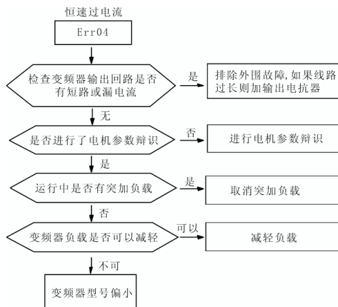
图8-4 恒速过电流 (Err04)
