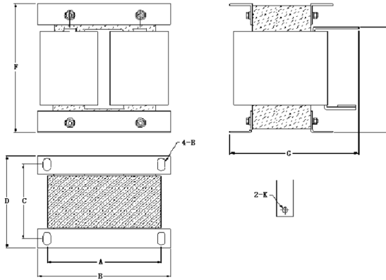
图 2-11 外置电抗器尺寸示意图
