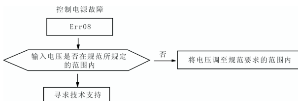
图 8-8 控制电源故障 (Err08)
