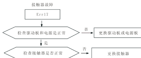
图 8-16 接触器故障 (Err17)
