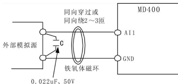
图 3-11 模拟量输入端子处理接线图
