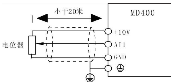
图 3-10 模拟量输入端子接线示意图
