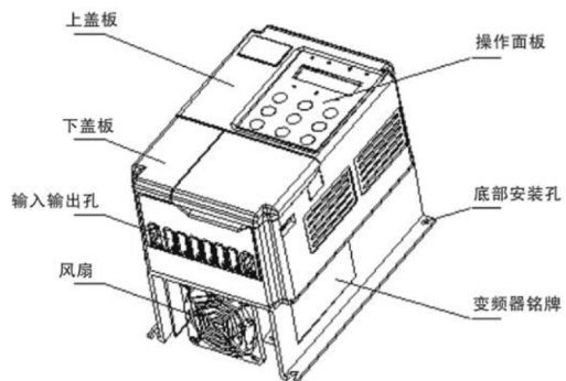
图 2-3 MD400 变频器外型图
