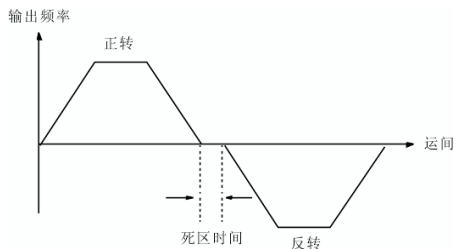
图 6-12 正反转死区时间示意图
