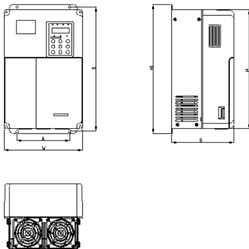
图 2-6 7.5kW~15kW 外型尺寸及安装尺寸示意图
