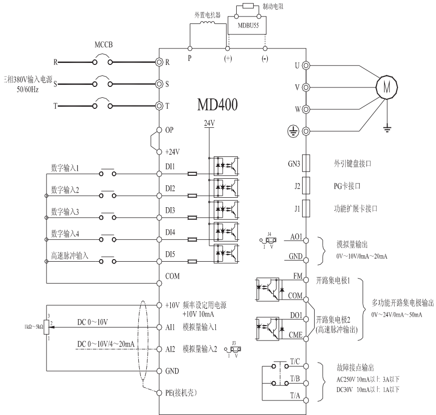
图3-8 75kW及以上外置电抗器接线示意图
