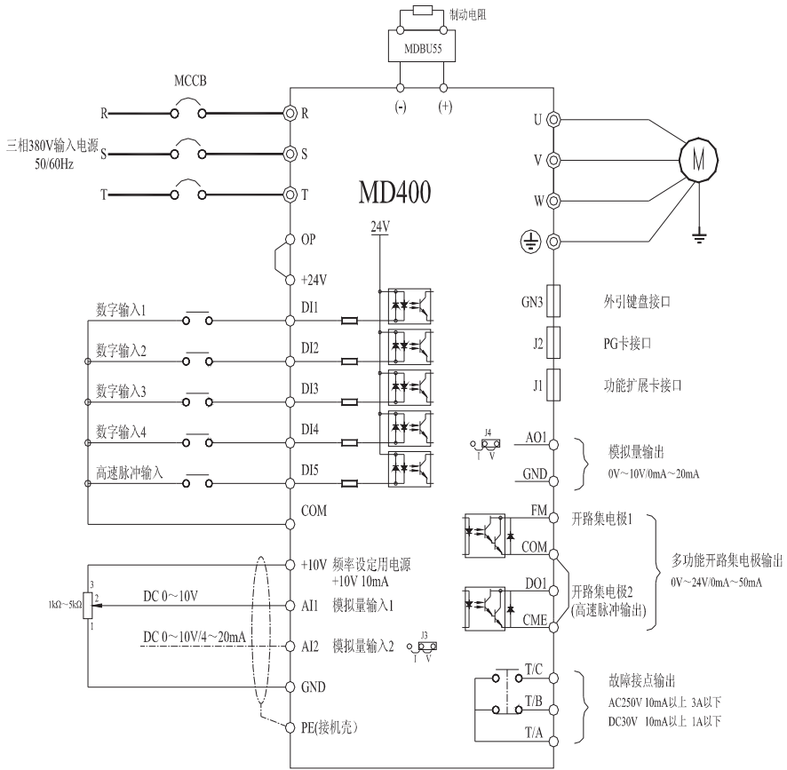
图3-7 37kW~55kW以上三相变频器接线示意图
