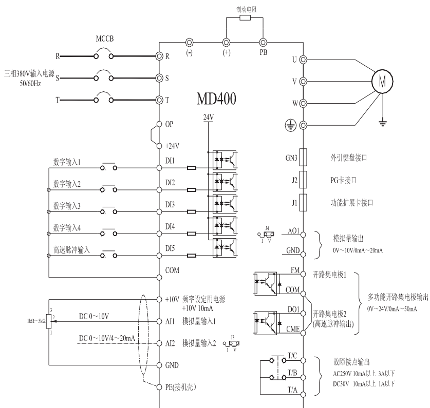
图3-6 30kW以下三相变频器
