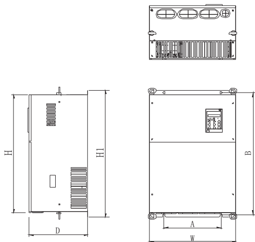
图2-7 18.5kW~450kW外型尺寸及安装尺寸示意图
