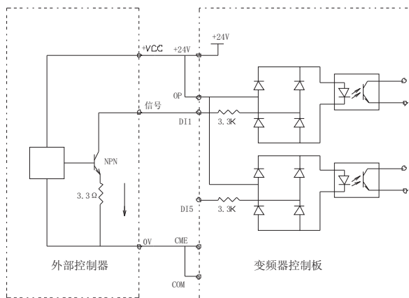
图 3-14 源极接线方式
