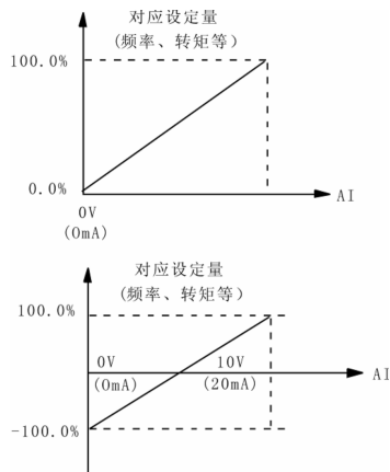
图6-9 模拟给定与设定量的对应关系
