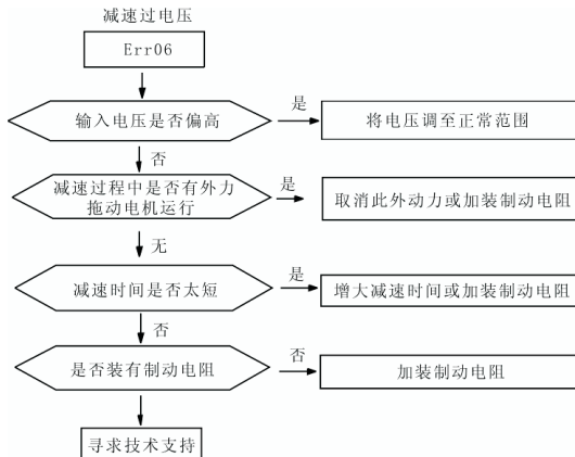
图 8-6 减速过电压（Err06）
