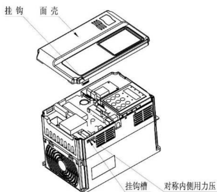
图 3-3 塑胶外壳下盖板拆卸图 (MD400N)
