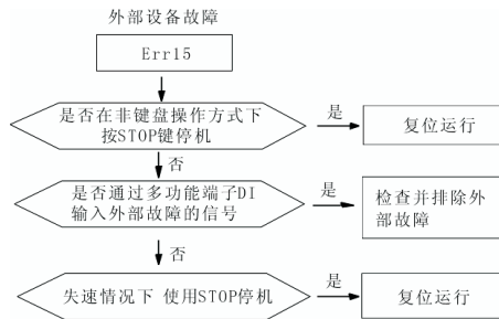
图 8-14 外部设备故障 (Err15)
