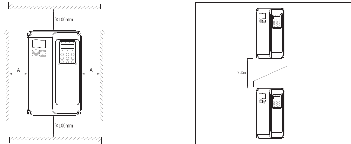
单体安装图
