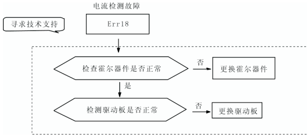
图8-17 电流检测故障（Err18）
