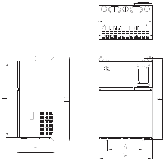
图 2-8 MD400N 系列 18.5kW~450kW 外型尺寸及安装尺寸示意图
