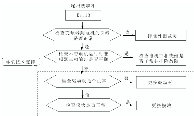
图 8-12 输出侧缺相 (Err13)
