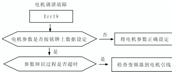
图 8-18 电机调谐故障（Err19）
