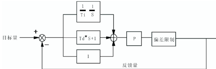
图6-15 过程PID原理框图
