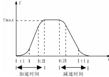
图 6-10 S 曲线加减速示意图
