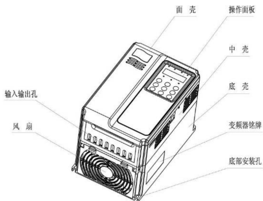
图 2-4 MD400N 变频器外型图
