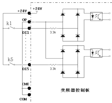
图 3-13 干接点共阳极接线示意图
