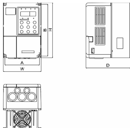
图 2-5 0.4kW~5.5kW 外型尺寸及安装尺寸示意图
