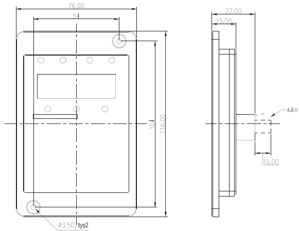
图 2-9 外引键盘的外型尺寸
