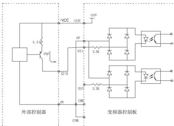
图 3-15 漏极接线方式
