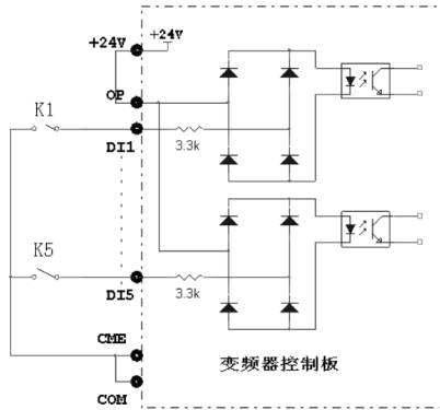
图 3-12 干接点共阴极接线示意
