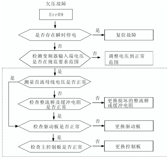
图 8-9 欠电压故障 (Err09)
