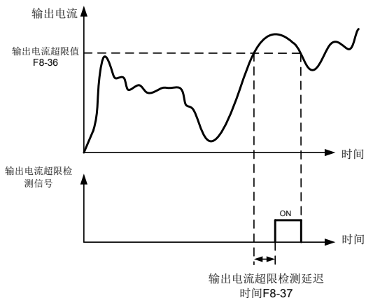
图 6-23 输出电流超限检测示意图
