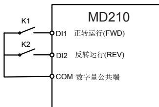
图 6-8 两线式模式 1
