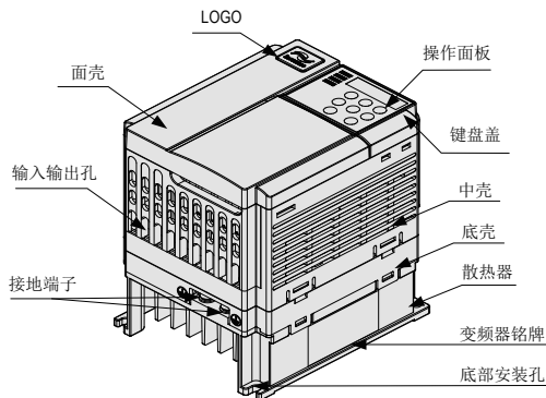
图 2-3 0.4kW-0.75kW 外形图
