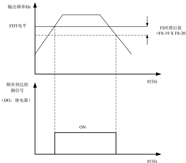
图 6-18 FDT 电平示意图
