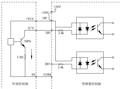
图 3-7 漏型接线方式
