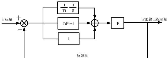
图 6-27 过程 PID 原理框图
