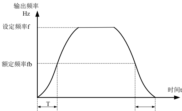
图 6-13 S 曲线加减速 A 示意图
