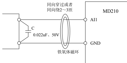
图 3-6 模拟量输入端子处理接线图
