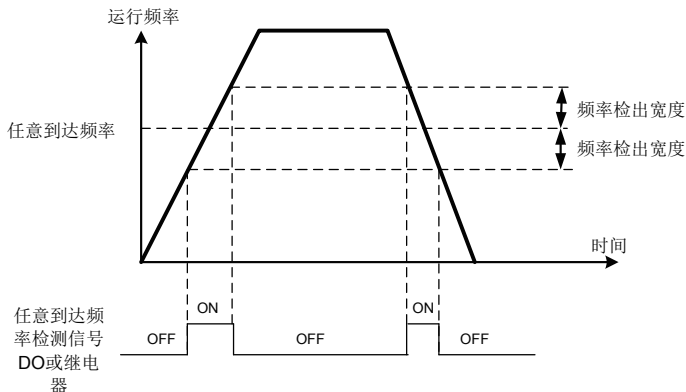
图 6-21 任意到达频率检测示意图
