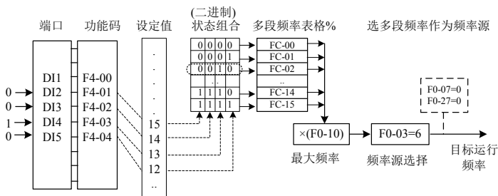
图 4-21 多段速模式的设置
