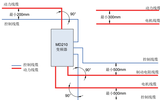
图 7-7 电缆布线图
