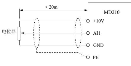
图 3-5 模拟量输入端子接线示意图
