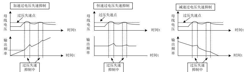
图 6-7 过压失速动作示意图
