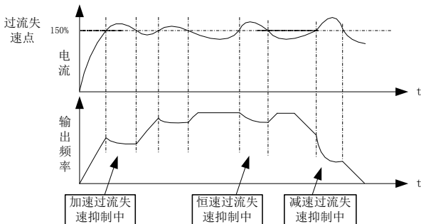
图 6-5 过流失速动作示意图
