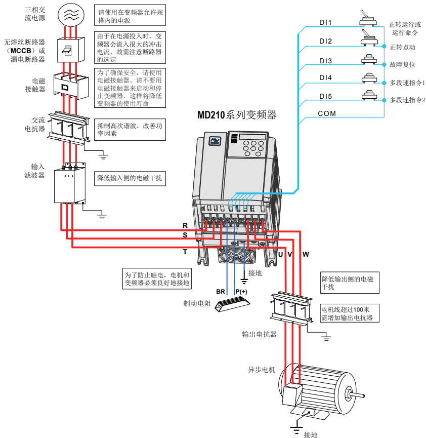
图1 与外围机器的连接示例
