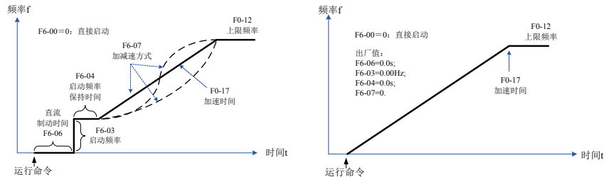
图 4-8 直接启动方式
