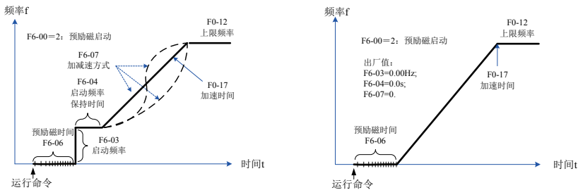
图 4-10 预励磁启动方式
