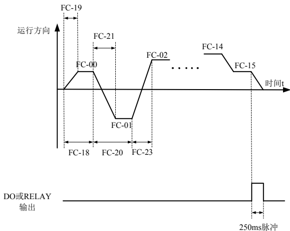
图 6-32 简易 PLC 示意图
