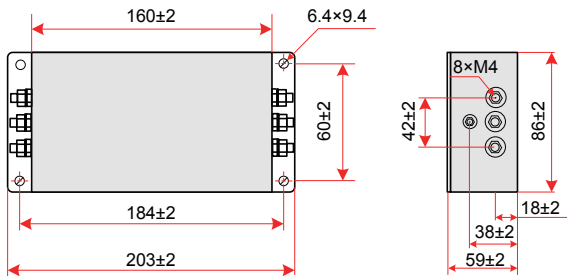
图 7-2 坚力滤波器 DL-5EBK5 尺寸图 (单位: mm)
