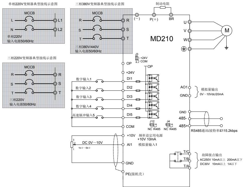
图 3-9 MD210 变频器典型接线示意图
