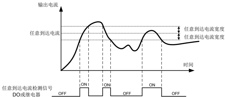
图 6-24 任意到达电流检测示意图
