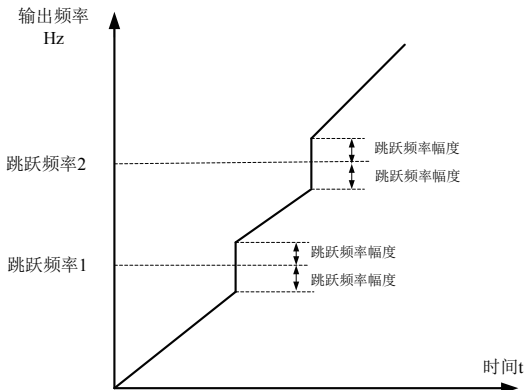
图 6-20 加减速过程中跳跃频率有效示意图
