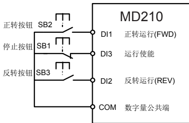
图 6-10 三线式控制模式 1
