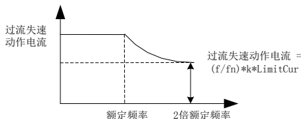
图 6-6 倍速过流失速动作示意图
