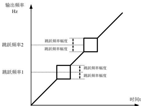
图 6-16 跳跃频率示意图
