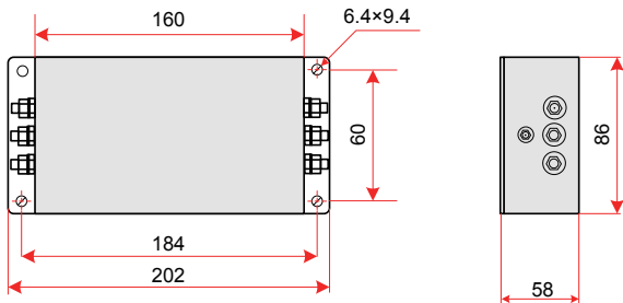
图 7-3 强力滤波器 DL-10EBK5 尺寸图 (单位: mm)
