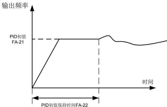
图 6-29 PID 初值功能示意图
