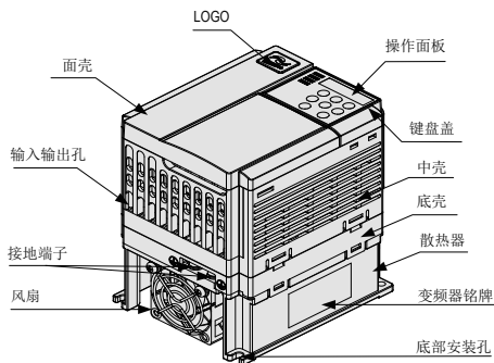
图 2-4 1.5kW-2.2kW 外形图
