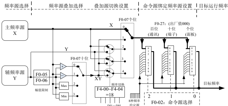
图 4-18 主辅助频率混合给定来源选择
