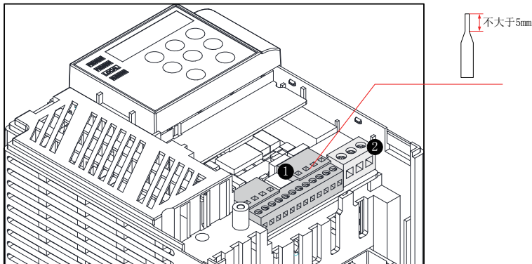
图 3-21 控制线管状端子要求
