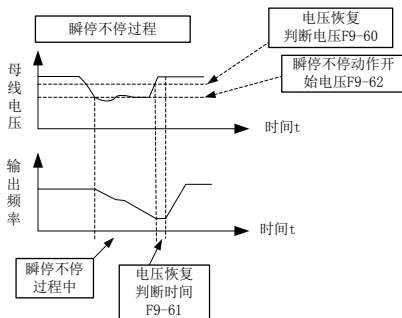
图 6-26 瞬停不停过程示意图
