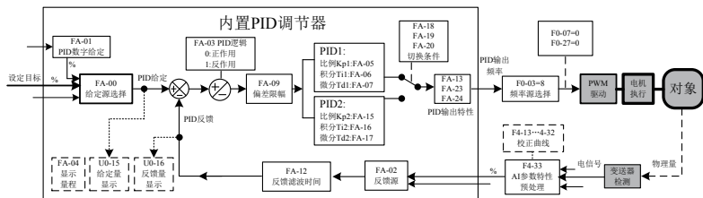
图 4-19 过程控制的频率闭环控制
