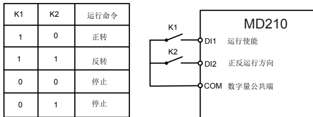
图 6-9 两线式模式 2
