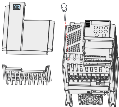
图 7-9 压敏电阻 (VAR) 和安规电容共同对 PE 连接的螺钉位置示意图
