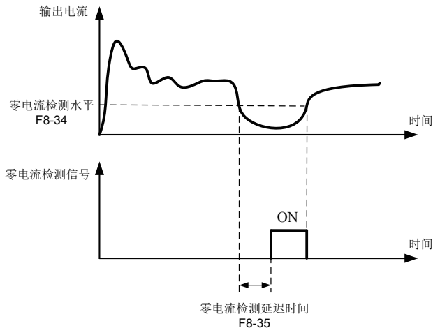
图 6-22 零电流检测示意图
