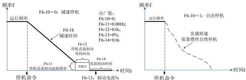
图 4-11 停机模式
