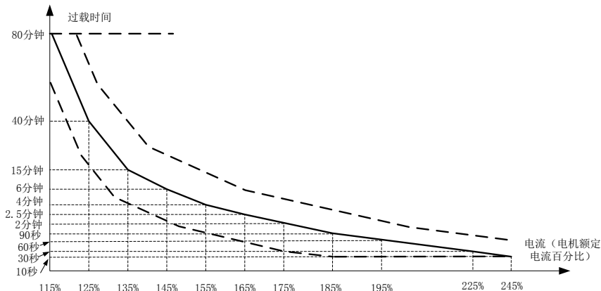
图 6-25 电机过载保护反时限曲线示意图
