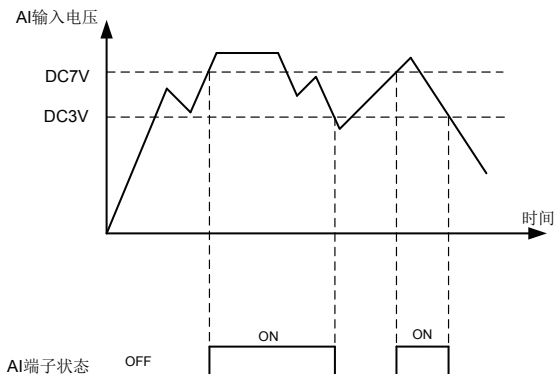
图 6-33 AI 端子有效状态判断
