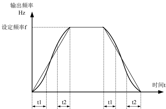
图 6-13 S 曲线加减速 A 示意图
