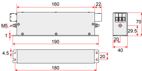
图 7-1 FN3258 系列 7A 滤波器尺寸图 (单位: mm)
