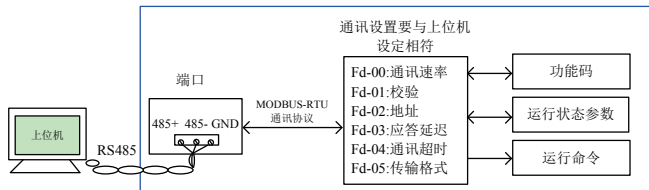
图 4-24 串行通讯设置
