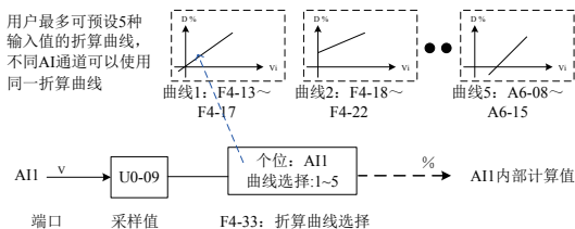
图 4-23 AI 输入信号处理
