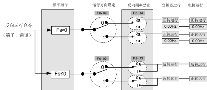
图 4-22 电机运转方向设置
