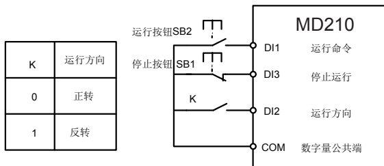
图 6-11 三线式控制模式 2
