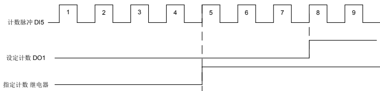
图 6-31 设定计数值给定和指定计数值给定示意图
