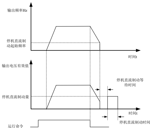
图 6-15 停机直流制动示意图
