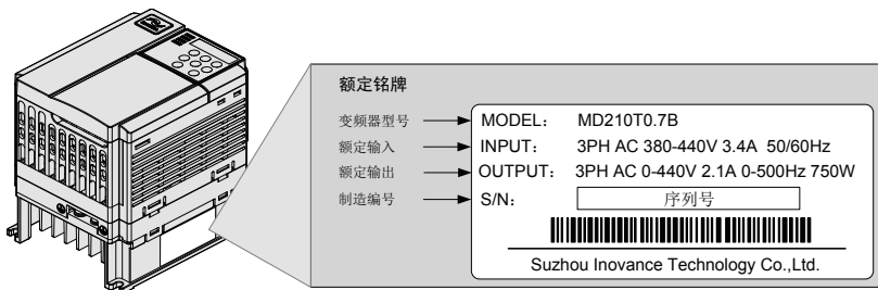
图 2-2 MD210 系列变频器铭牌
