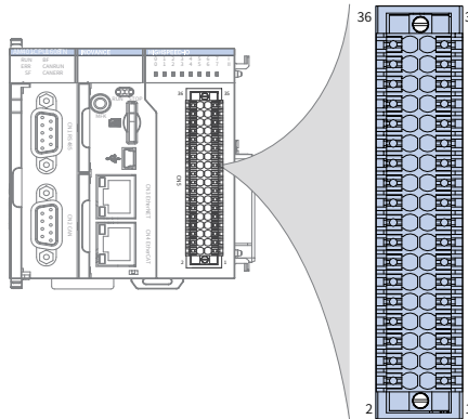
图4 CPU 模块接线端子排列
