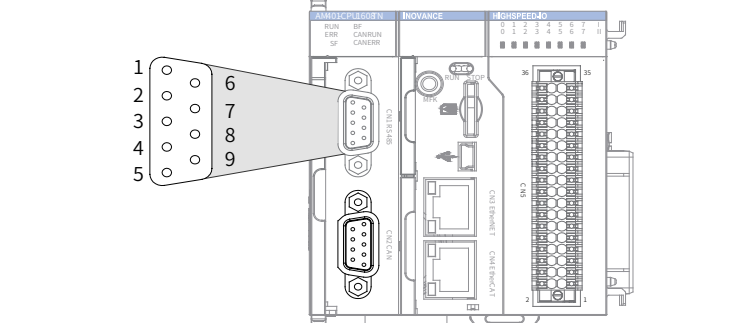
图 10 CPU 模块上的 RS485 通讯端子定义
