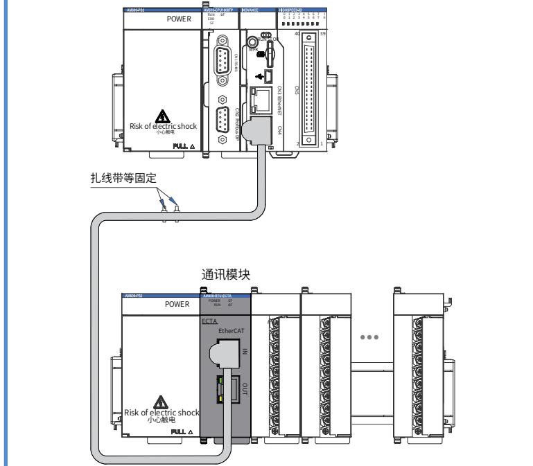
图8 通讯线缆在靠近设备侧需做必要固定
