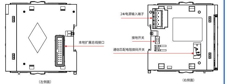
图3 CPU 模块接口示意图 2
