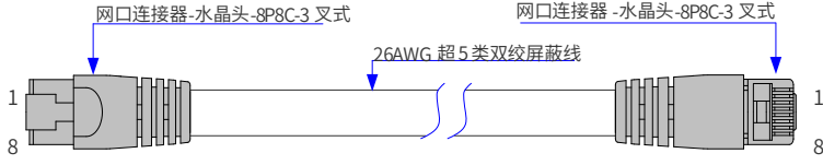
图 9 EtherCAT 网线制作要求
