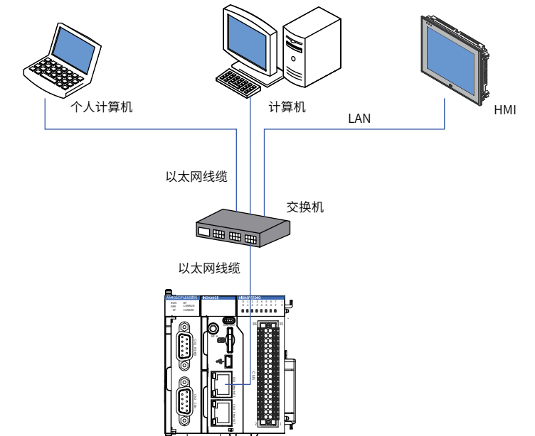
图 12 CPU 模块通过交换机与其他设备连接
