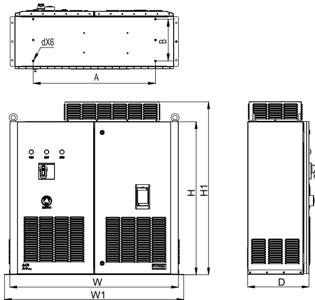
图 1-6 变频柜外形尺寸示意图 (200kW~355kW)
