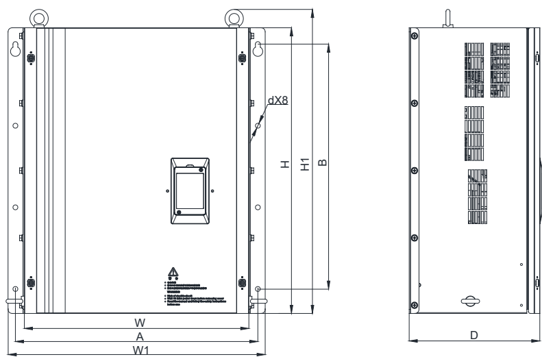
图 1-8 变频器外形尺寸示意图（200kW~355kW）
