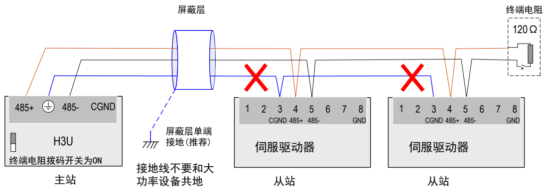
图 3-30 错误的 485 连接方法
