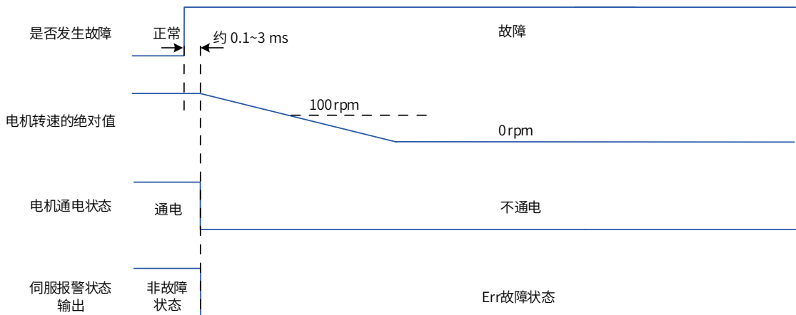
图 5-17 故障 2 时自由停机保持自由运行状态时序图
