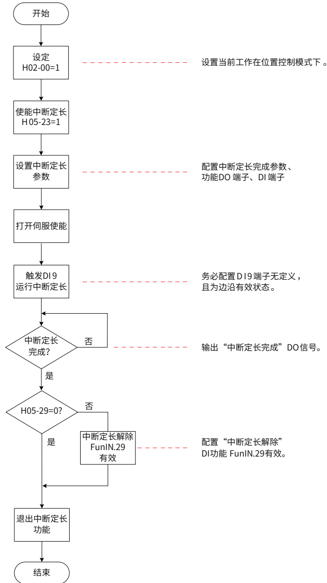
图 5-47 中断定长功能信号流程图
