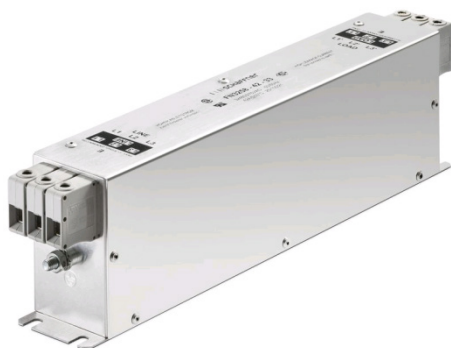
图 12-3 夏弗纳 (SCHAFFNER) FN3258 系列滤波器外形图
