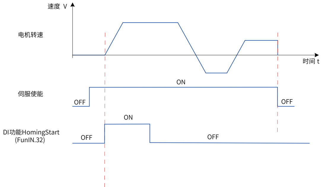
图 5-65 时序图举例
