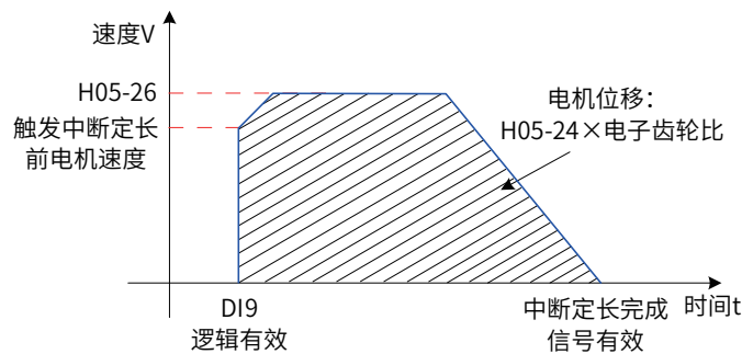
图 5-48 中断定长功能电机运行曲线
