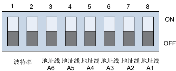
图 11-14 H3u 拨码拨码开关示意图
