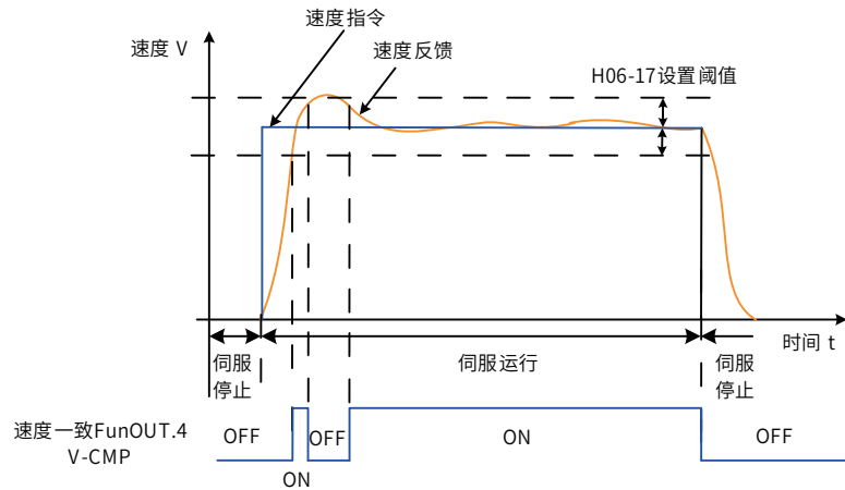
图 5-83 速度一致信号波形图
