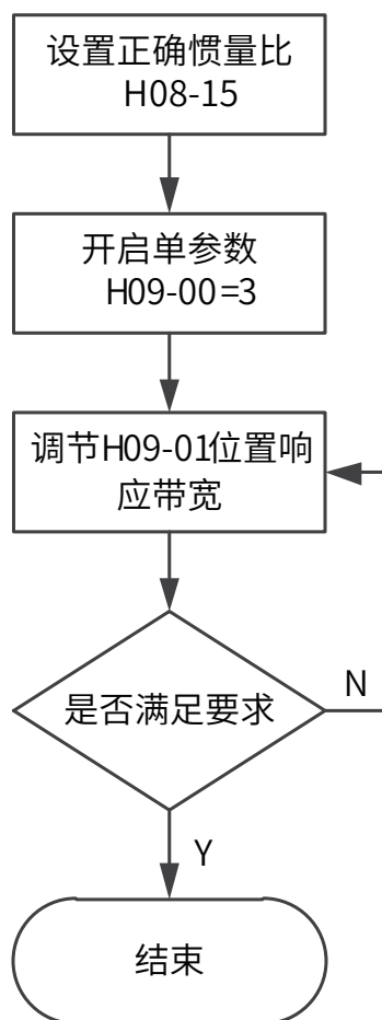
图 6-5 操作流程图
