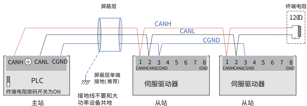
图 10-16 CANlink 接线示意图
