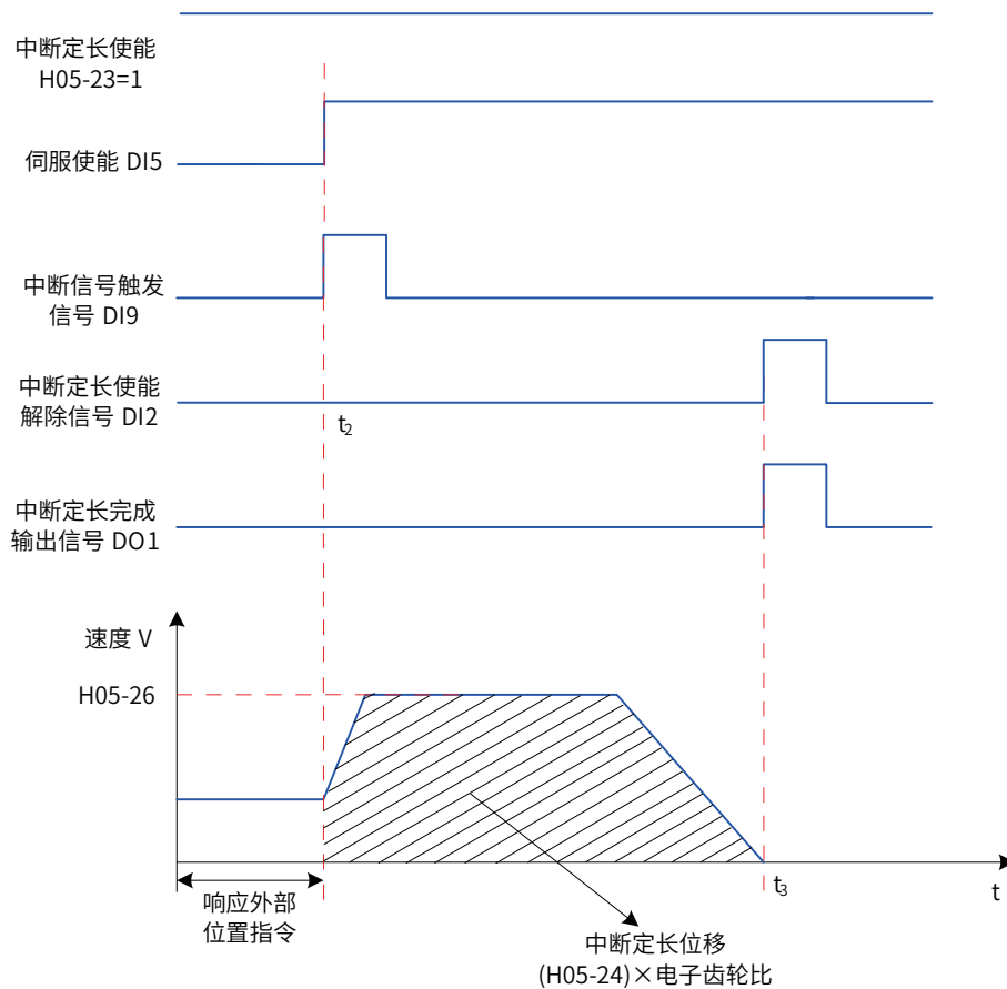
图 11-18 时序说明
