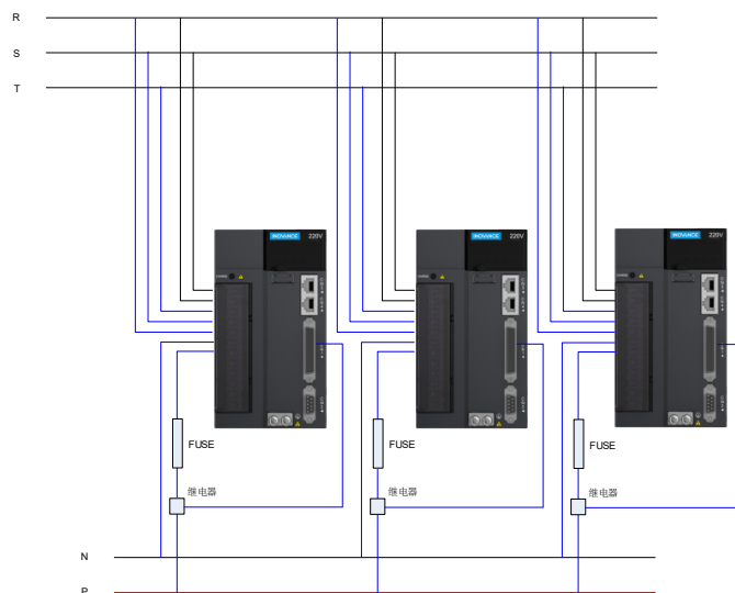
图 11-26 硬件接线图
