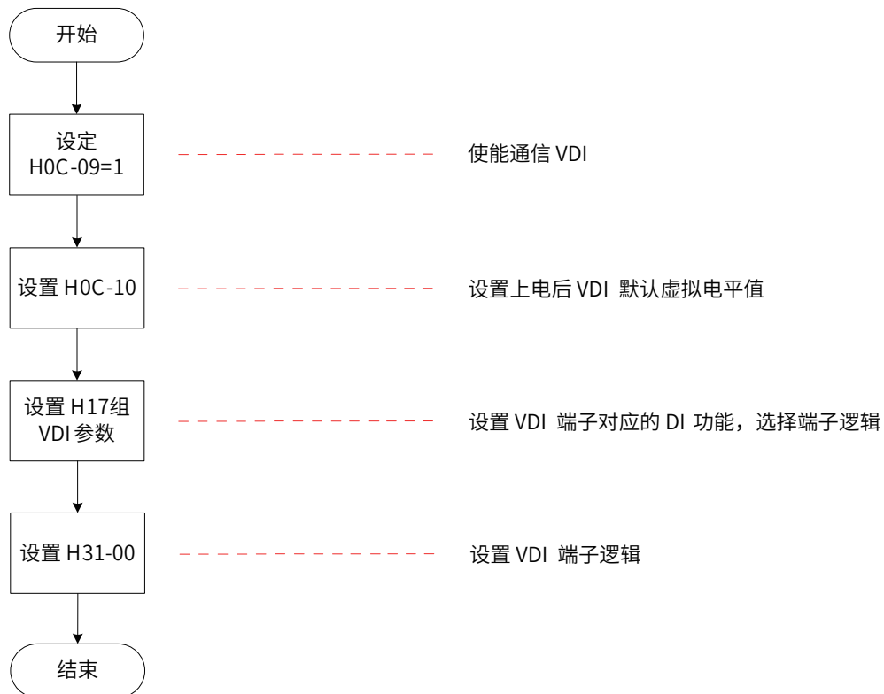
图 10-18 VDI 使用流程图
