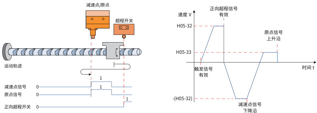
图 5-51 模式 0 原点回零电机运行曲线③与转速说明
