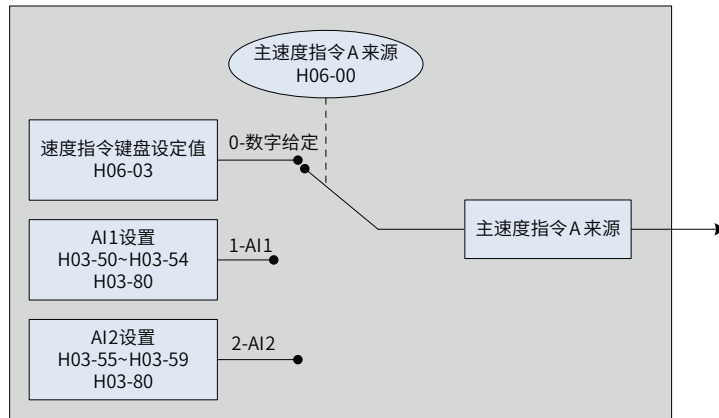
图 5-69 主速度指令 A 来源图
