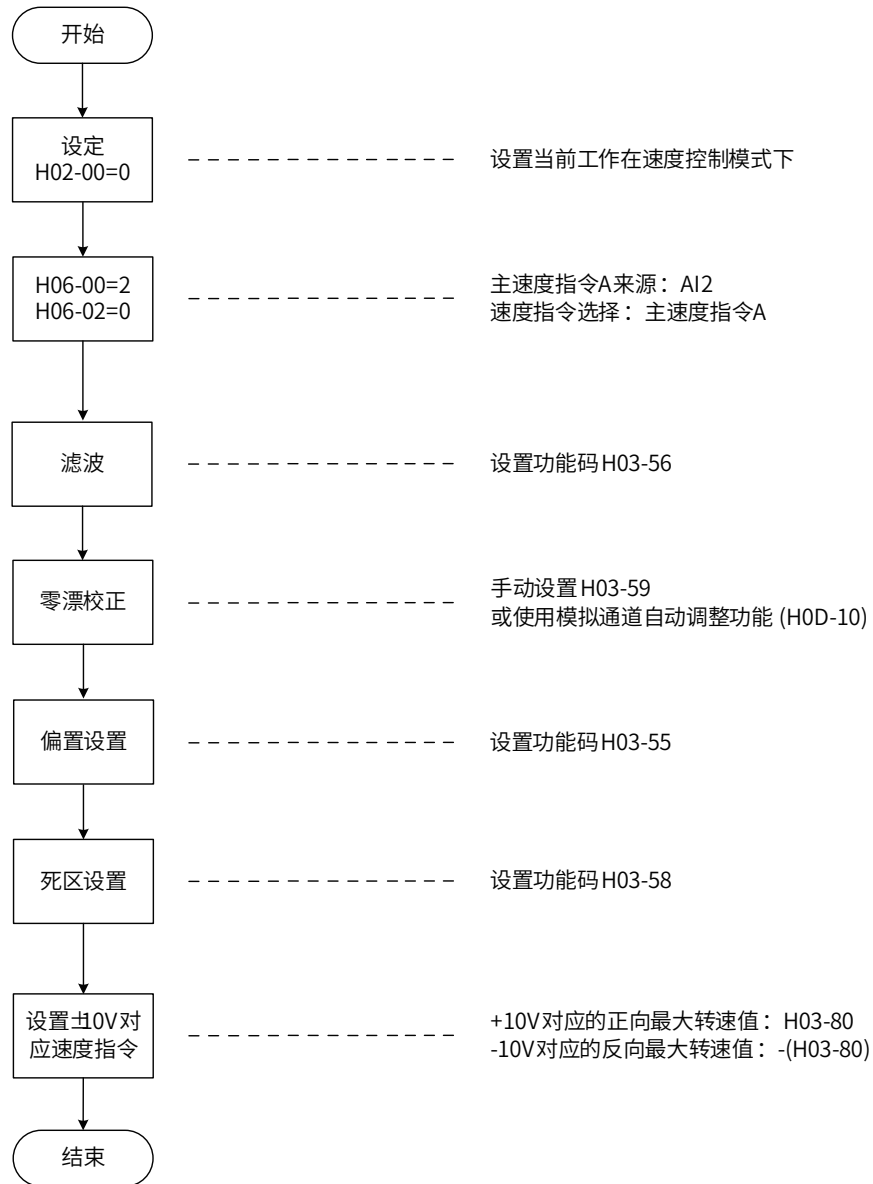
图 5-70 模拟量电压速度指令操作流程图
