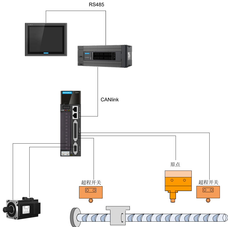
图 11-12 案例原理图
