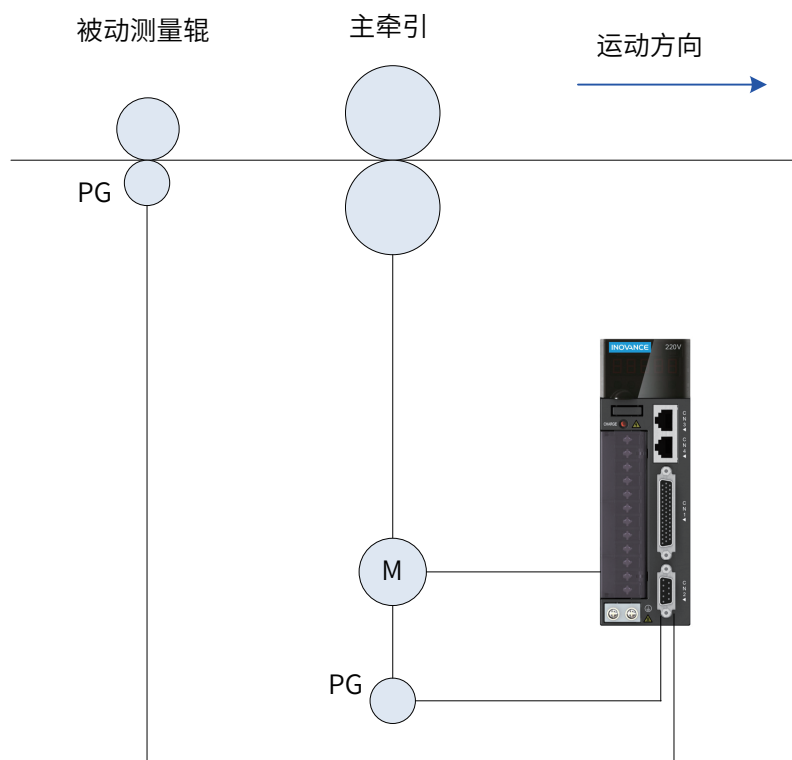
图 11-19 案例原理图
