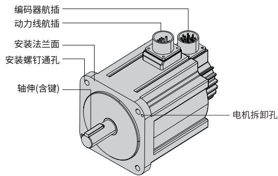
图 1-9 航插型电机部件说明示意图
