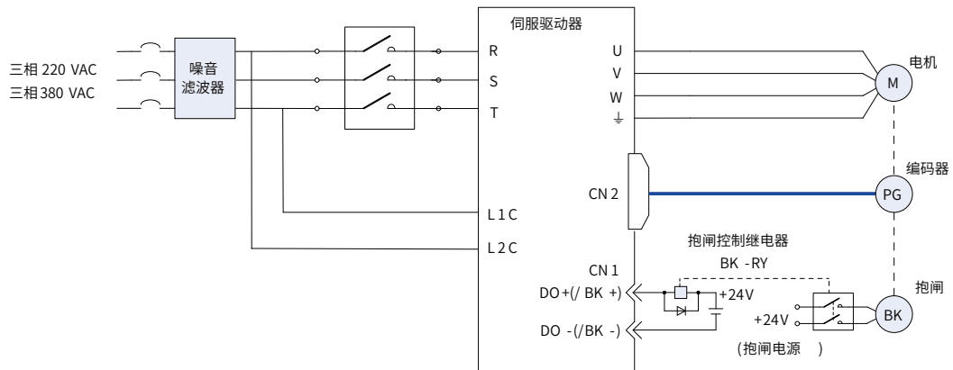
图 3-21 抱闸配线图
