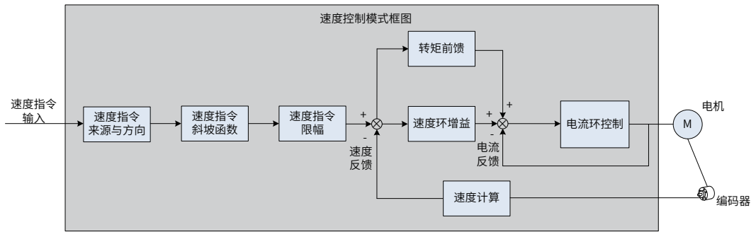
图 5-66 速度控制框图
