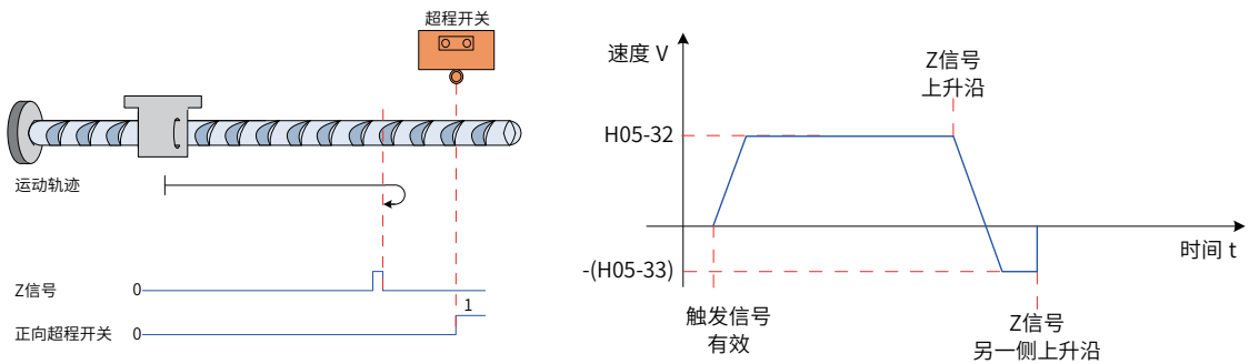
图 5-52 模式 2 原点回零电机运行曲线①与转速说明
