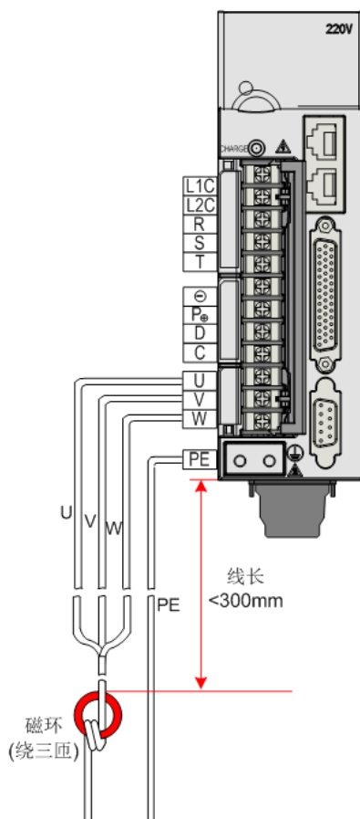
图 12-12 输出磁环（外置）安装图示
