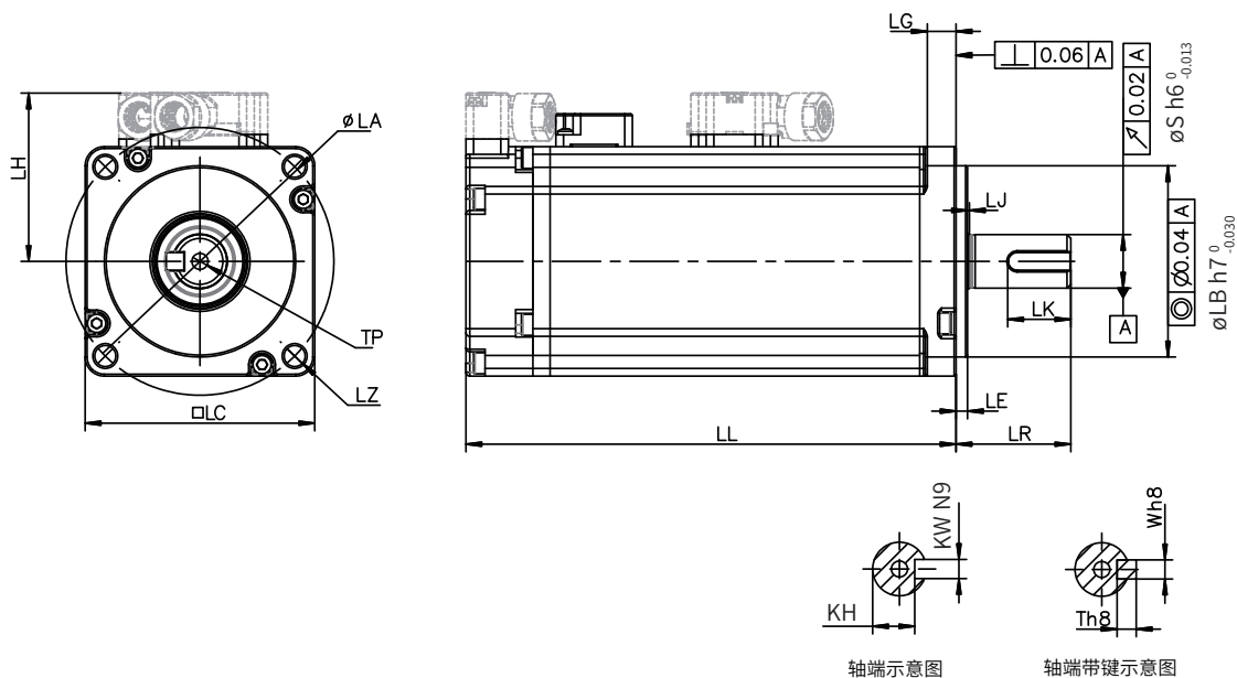
轴端示意图
