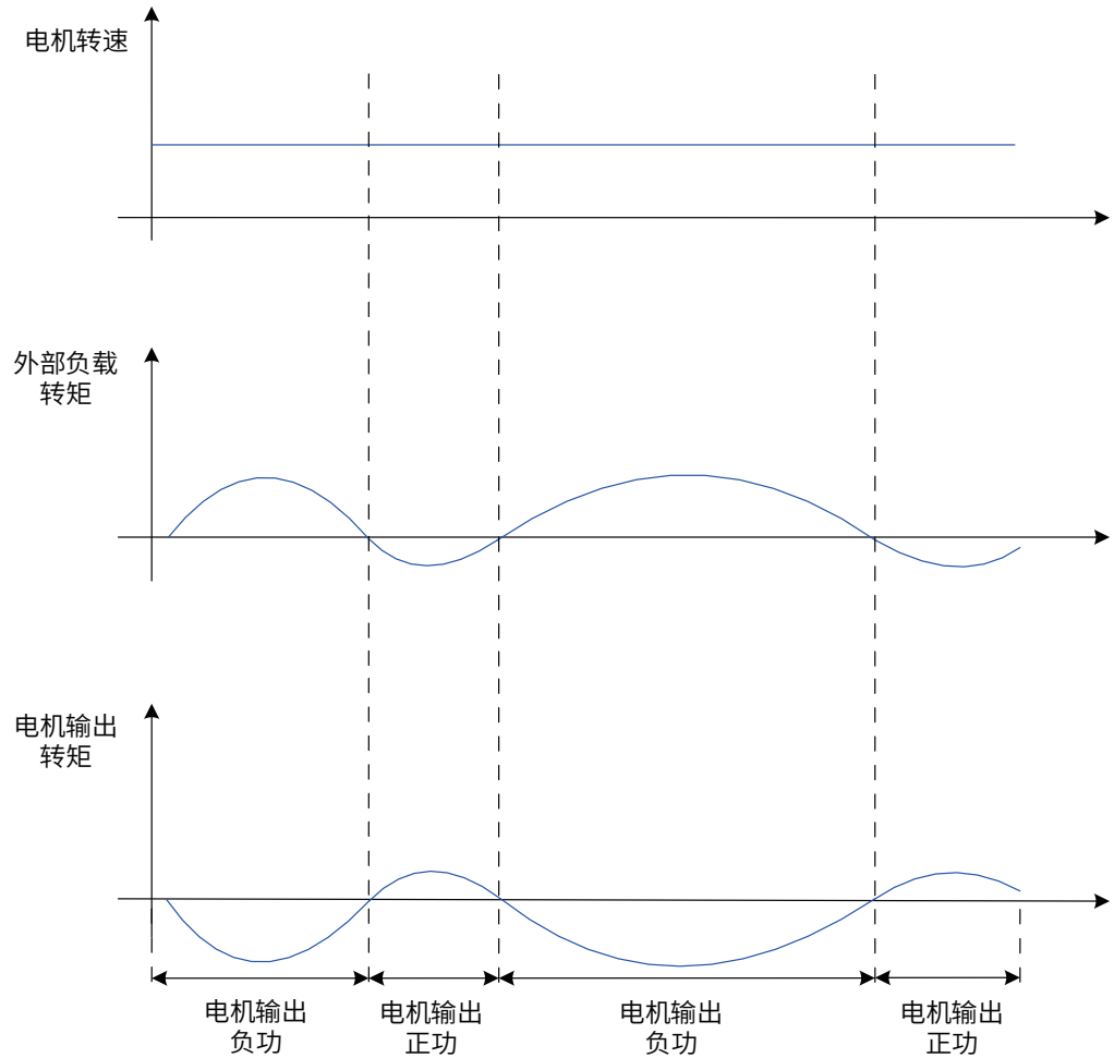
图 5-14 外部负载扭矩存在情况下曲线举例
