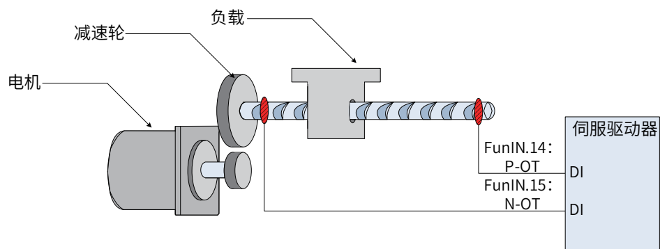
图 5-118 限位开关的安装示意图
