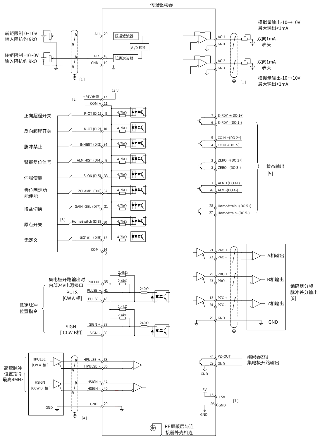
图 3-40 位置模式配线图
