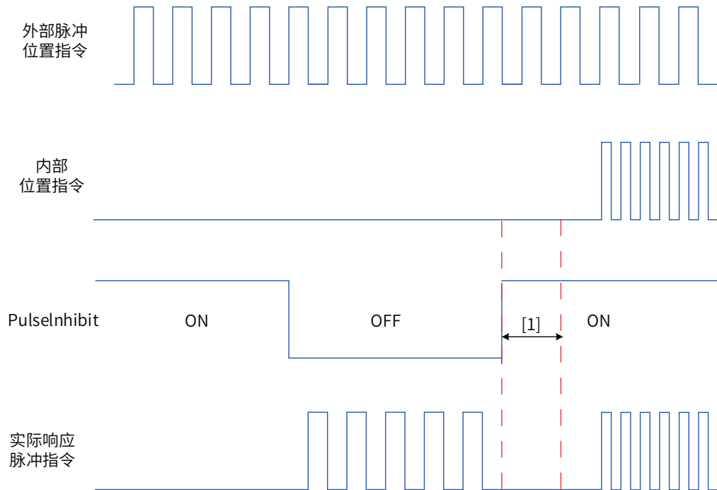
图 5-36 脉冲指令禁止功能波形举例
