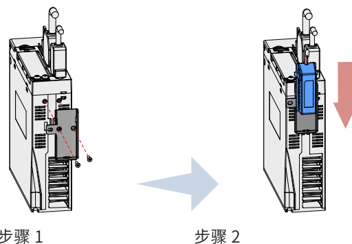
图 3-14 绝对值编码器电池盒安装示例图 (sizeA 机型，仰视图)
