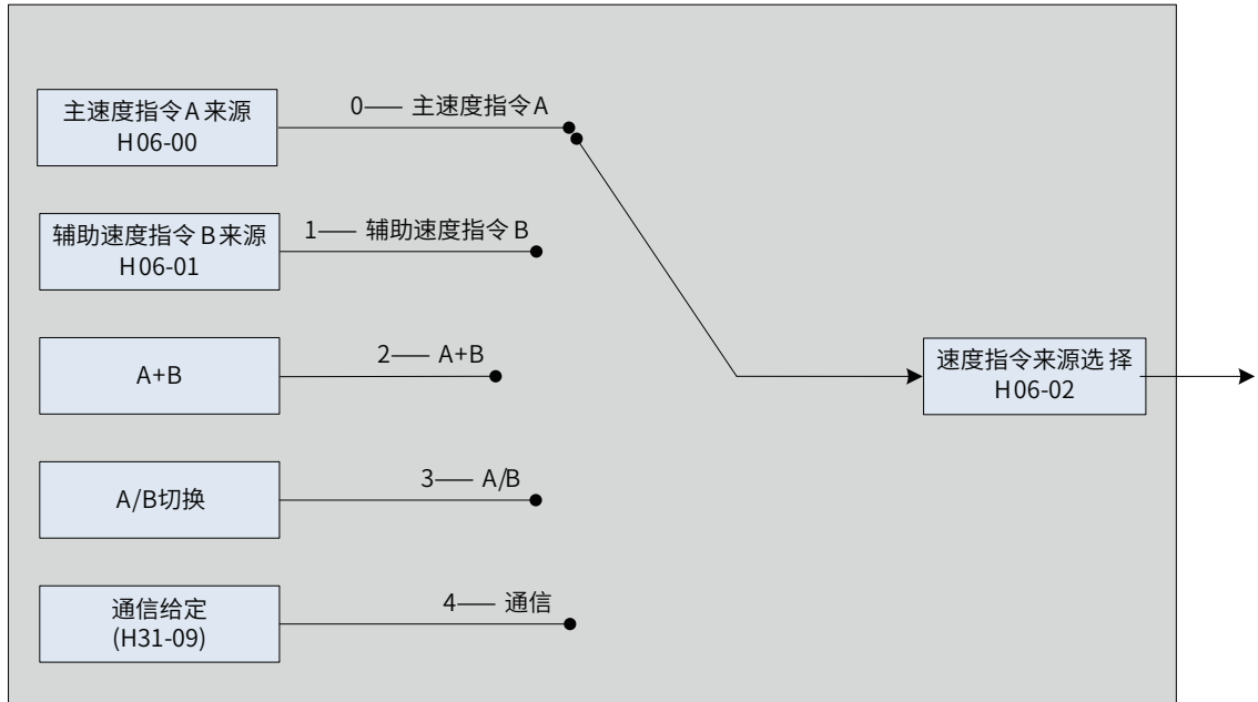
图 5-68 速度指令来源图
