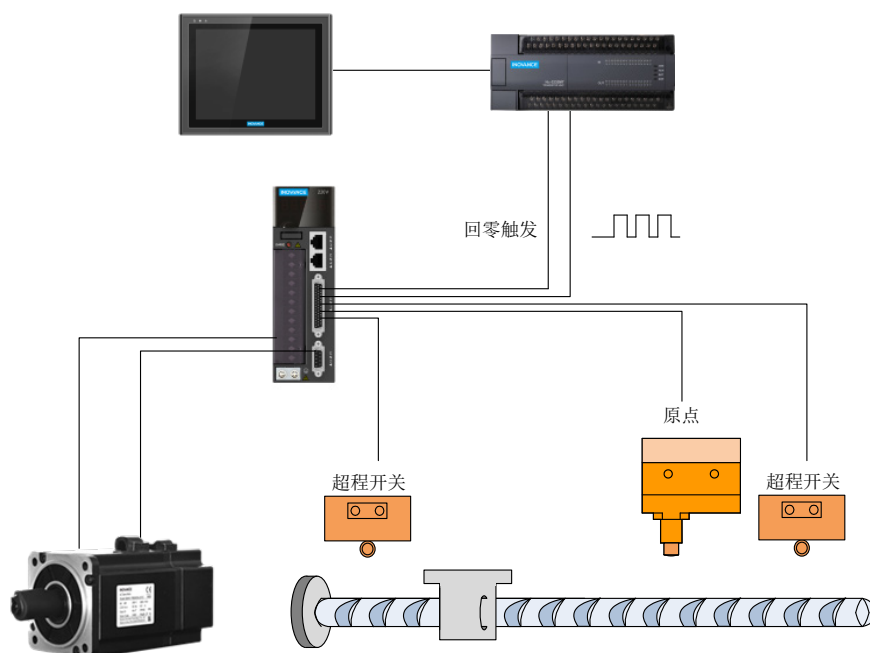
图 11-1 案例原理图
