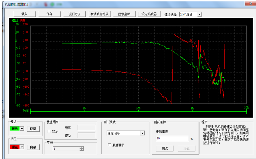
图 6-21 波形实例
