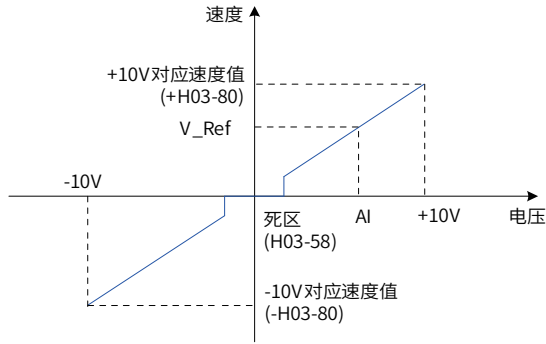
图 5-73 无偏置 AI2 示意图
