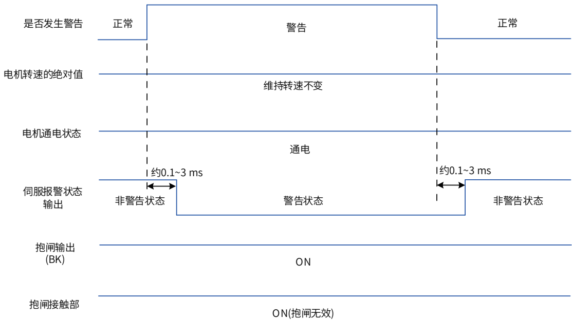
图 5-21 非停机警告时序图
