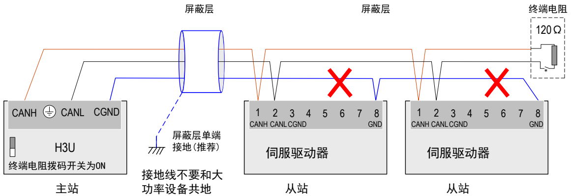
图 3-26 错误的 CAN 连接方法
