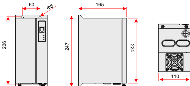
图 8-12 MDBUN 系列制动单元外形尺寸图 (单位: mm)
