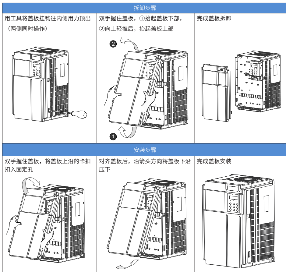
图 3-24 CP300T18.5G~CP300T37G 机型盖板拆卸与安装
