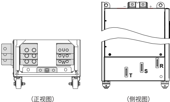
图 3-29 CP300T200G~CP300T280G 主回路端子分布图
