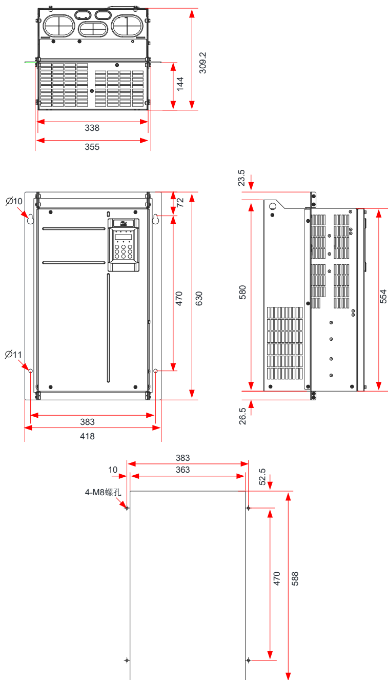
图 8-6 CP300T75G-CP300T110G 中部安装支架及开孔尺寸
