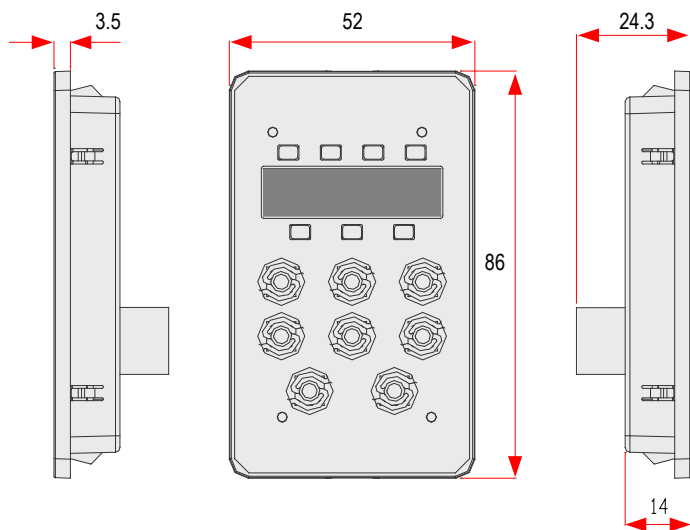
图 8-17 MD310-KEY1 外引操作面板尺寸
