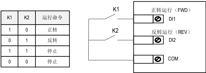
图 5-4 两线式模式 1
