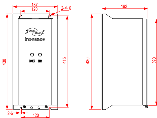
图 8-14 MDBU 系列制动单元 (MDBU-200-X) 外形尺寸图 (单位: mm)
