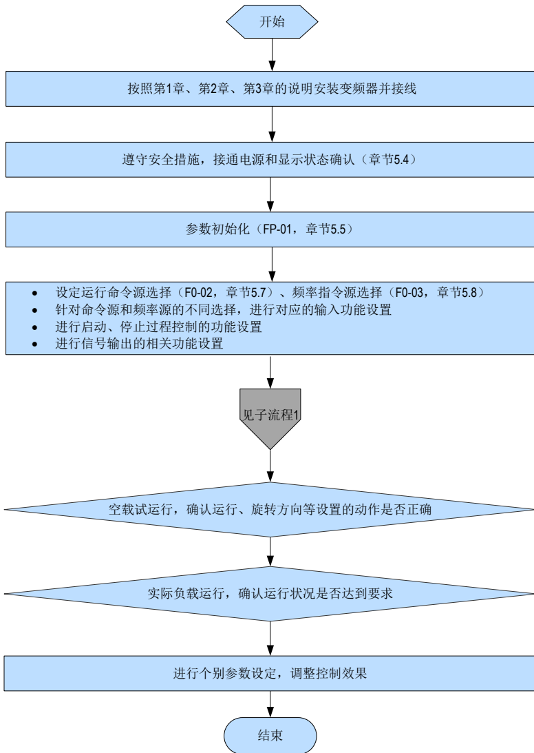
图 5-2 变频器调试总流程图
