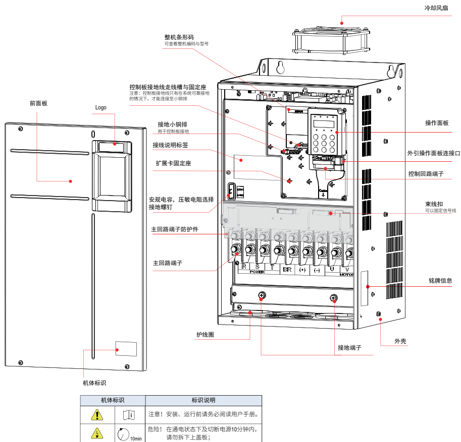
图 1-4 产品部件示意图【三相 380V~480V，CP300T45G ~ CP300T160G】
