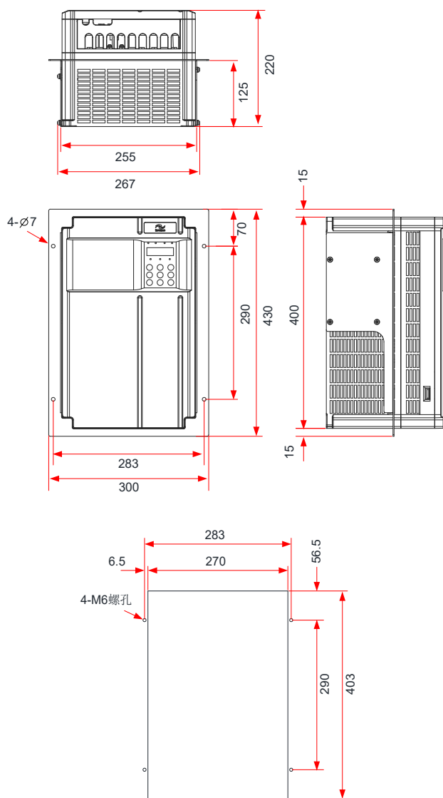
图 8-4 CP300T30G-CP300T37G 中部安装支架及开孔尺寸
