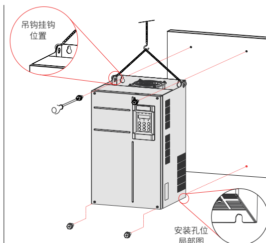
图 3-8 CP300T45G~CP300T160G/ 机型壁挂式安装示意图
