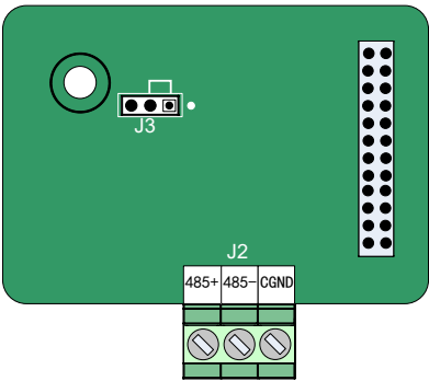
图 A-2 MD38TX1 端子分布示意图
