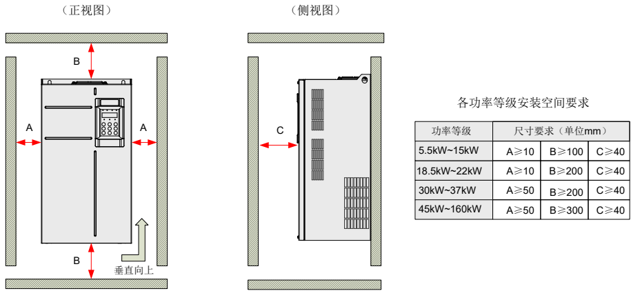
图 3-2 单台机器 (CP300T5.5G-CP300T160G) 安装空间
