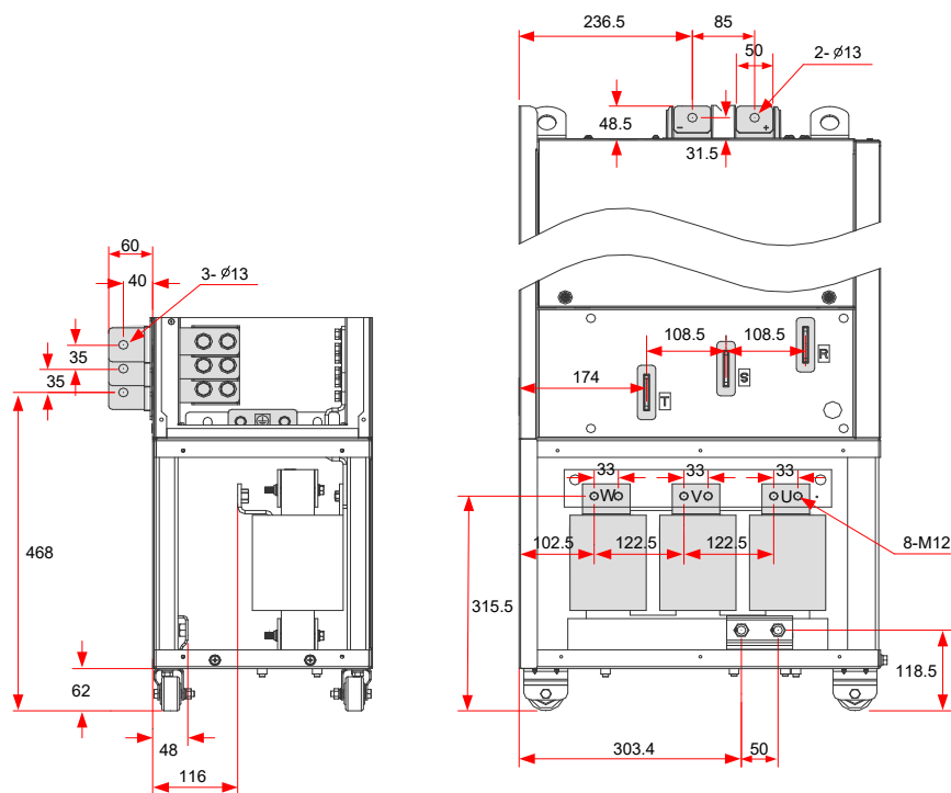
图 3-47 CP300T200G-L~CP300T220G-L 主回路端子尺寸 (带输出电抗器)
