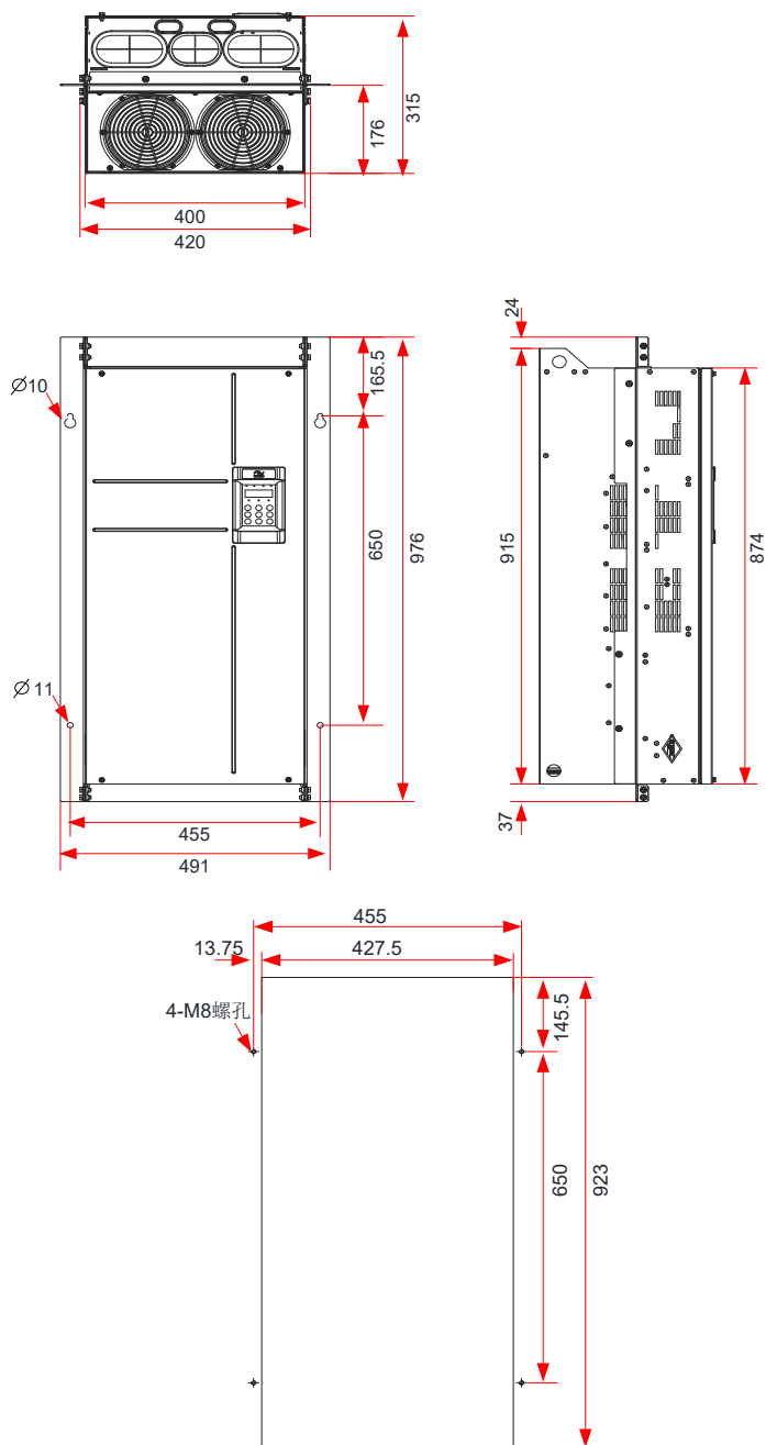
图 8-7 CP300T132G-CP300T160G 中部安装支架及开孔尺寸
