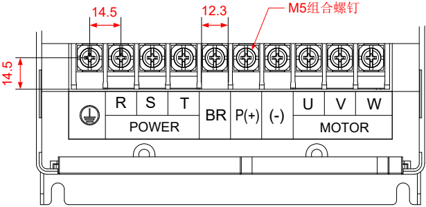
图 3-40 CP300T15G 主回路端子尺寸
