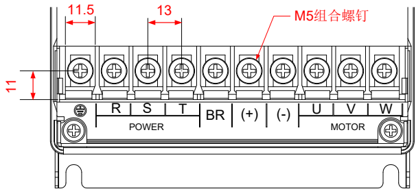
图 3-39 CP300T7.5G~CP300T11G 主回路端子尺寸
