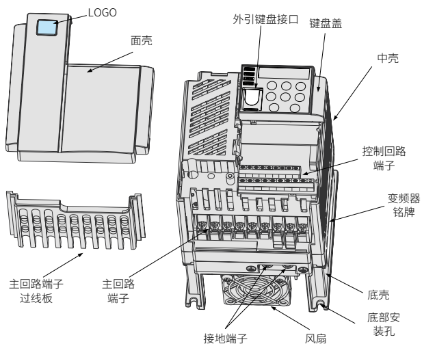
图 1-2 产品部件示意图【三相 380V~480V，CP300T5.5G ~ CP300T15G】
