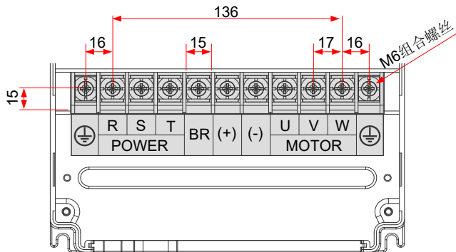
图 3-41 CP300T18.5G~CP300T22G 主回路端子尺寸
