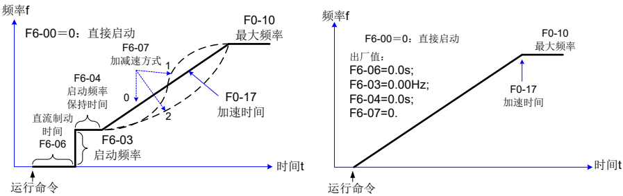
图 5-8 直接启动方式
