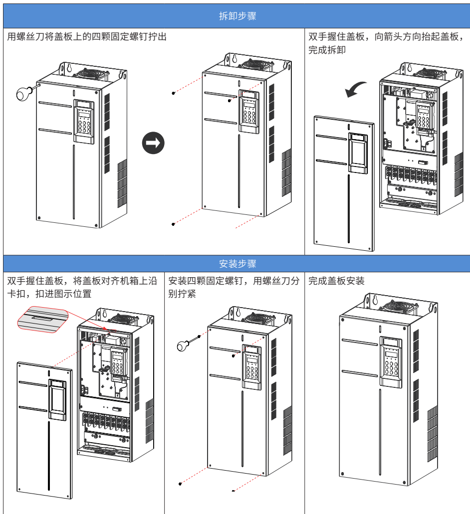
图 3-25 CP300T45G~CP300T160G 机型盖板拆卸与安装
