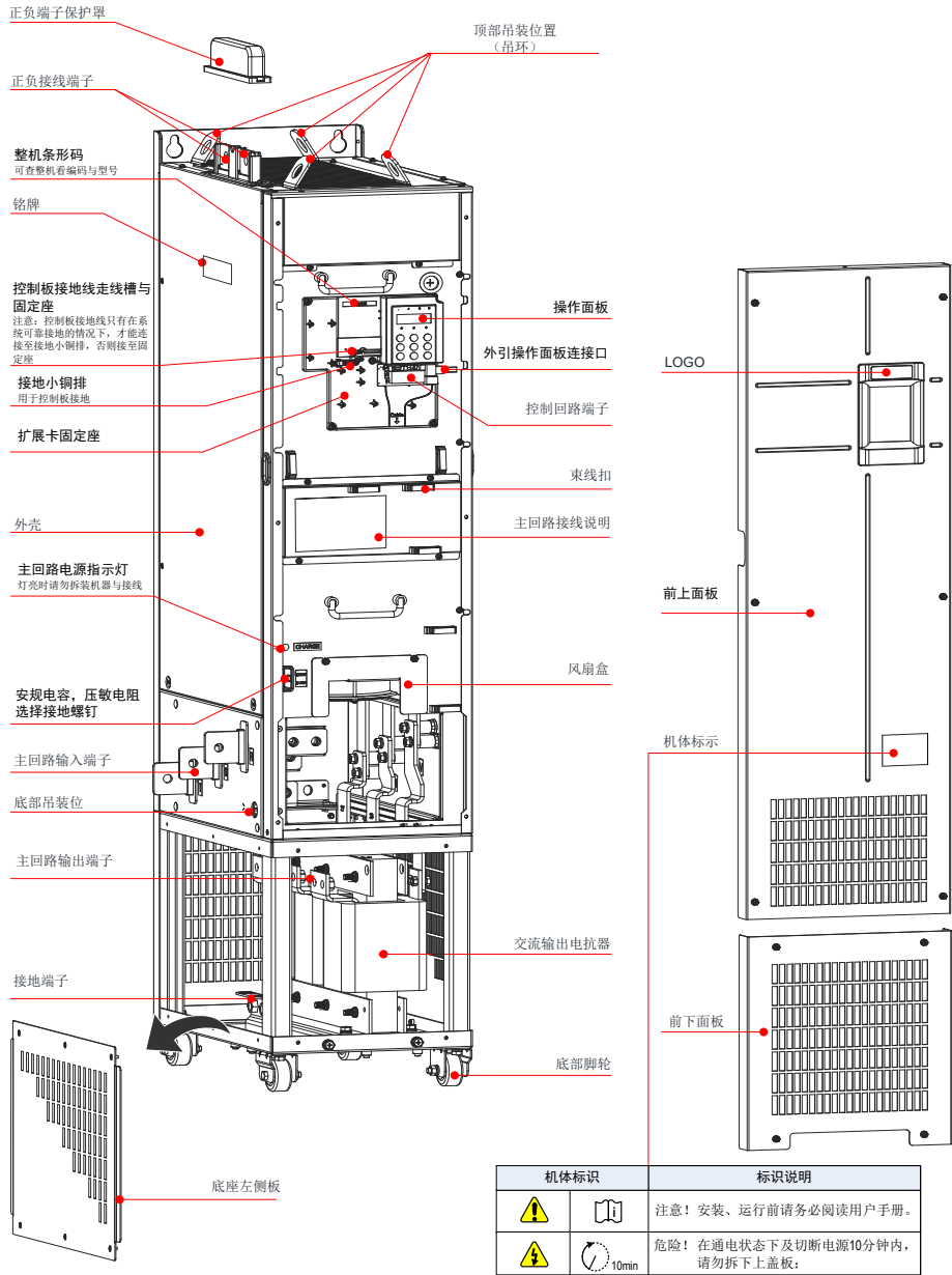
图 1-6 产品部件示意图【三相 380V~480V，CP300T200G-L ~ CP300T280G-L】
