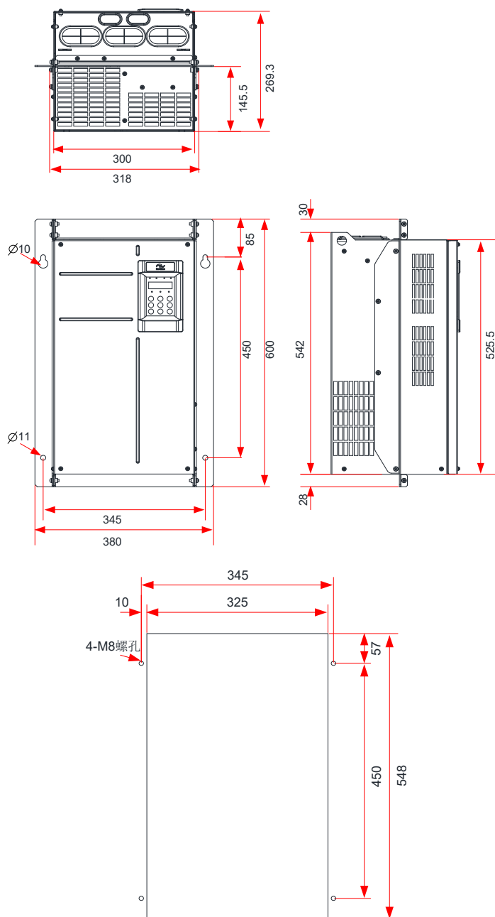
图 8-5 CP300T45G-CP300T55G 中部安装支架及开孔尺寸
