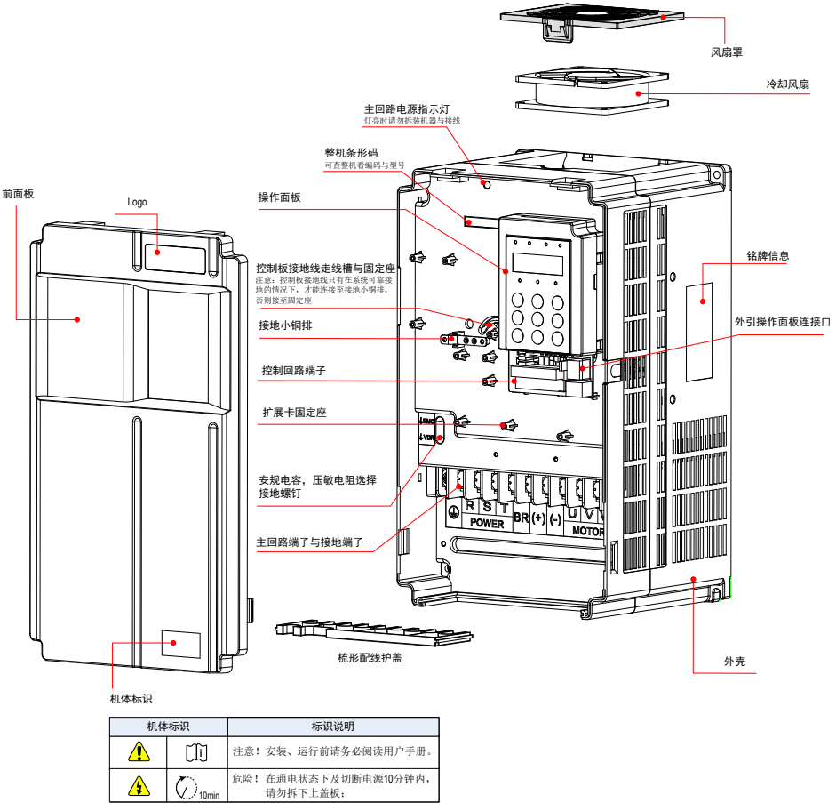
图 1-3 产品部件示意图【三相 380V~480V，CP300T18.5G ~ CP300T37G】
