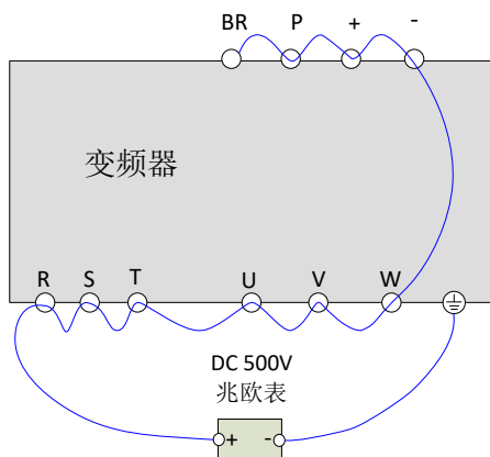
图 7-1 主回路绝缘测试示意图
