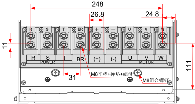
图 3-43 CP300T45G~CP300T55G 主回路端子尺寸
