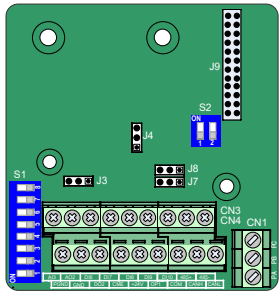
图 A-3 MD38IO1 端子分布示意图
