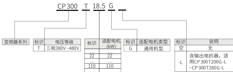
图 1-1 产品命名与铭牌标识
