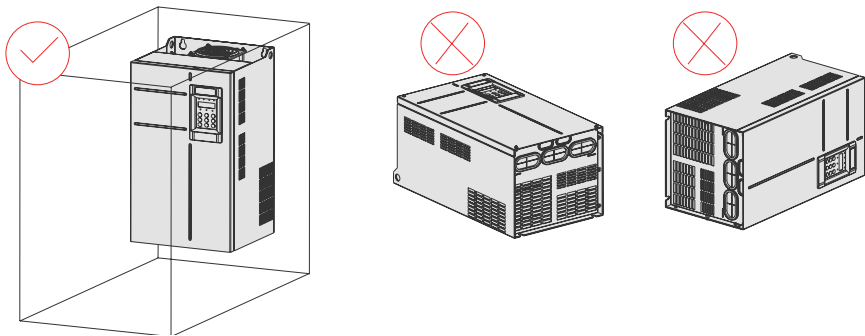
图 3-6 安装方向示意图
