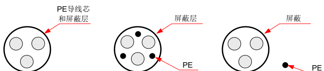
图 3-30 推荐的动力电缆类型
