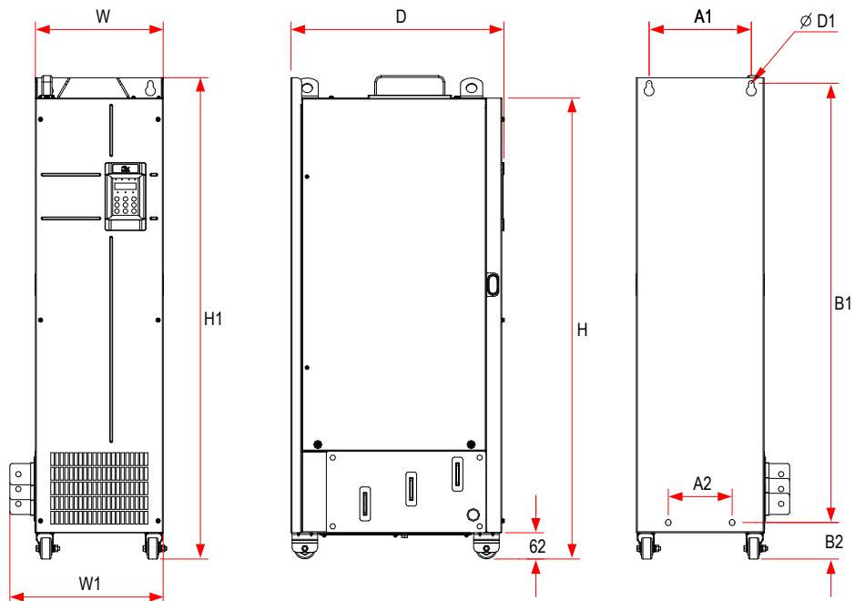
图 8-8 CP300T200G ~ CP300T280G 外型尺寸及安装尺寸示意图
