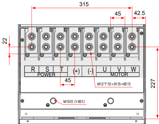
图 3-45 CP300T132G~CP300T160G 主回路端子尺寸
