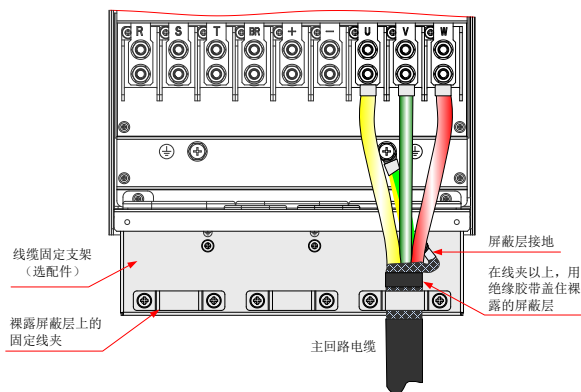
图 3-33 屏蔽层接线
