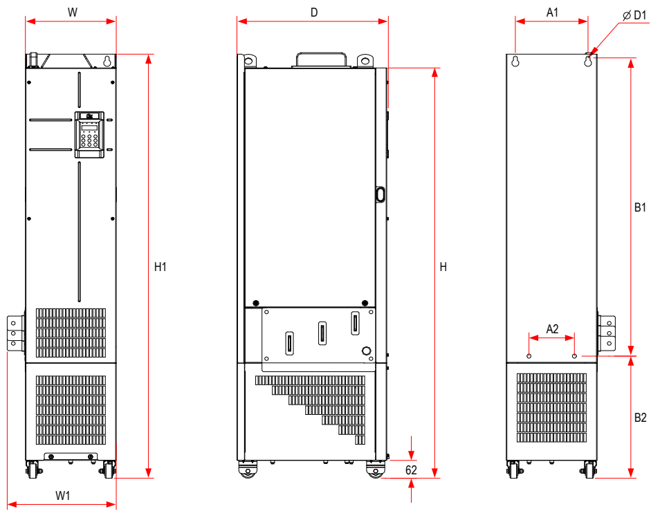
图 8-9 CP300T200G-L ~ CP300T450G-L 外型尺寸及安装尺寸示意图（带电抗器底座）
