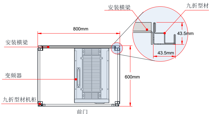
图 3-15 CP300T200G(-L)~CP300T280G(-L) 机柜俯视示意图
