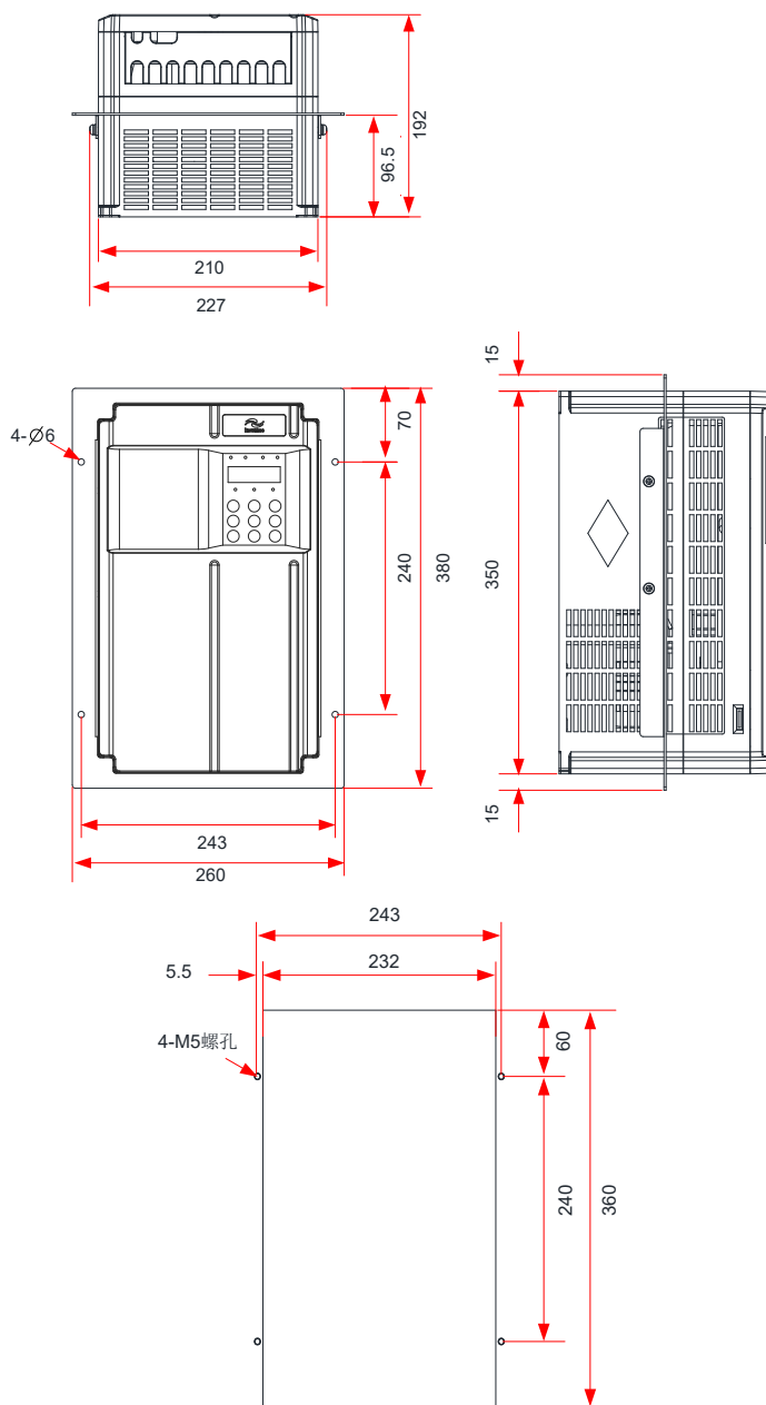
图 8-3 CP300T18.5G-CP300T22G 中部安装支架及开孔尺寸
