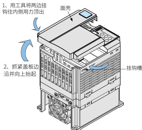
图 3-23 CP300T5.5G~CP300T15G 机型盖板拆卸步骤
