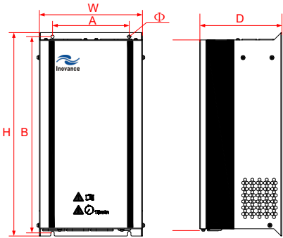
图 8-15 MD051 系列 AFE 单元外形尺寸图（单位：mm）
