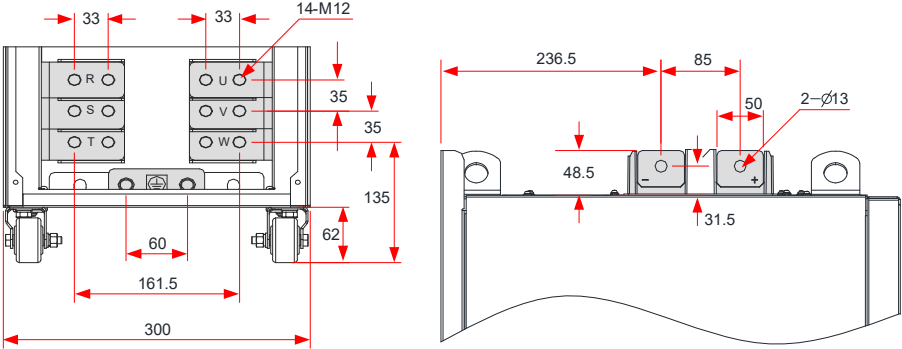
图 3-48 CP300T200G-L~CP300T220G-L 主回路端子尺寸（不带侧出铜排，不带输出电抗器）
