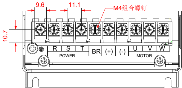
图 3-38 CP300T5.5G 主回路端子尺寸
