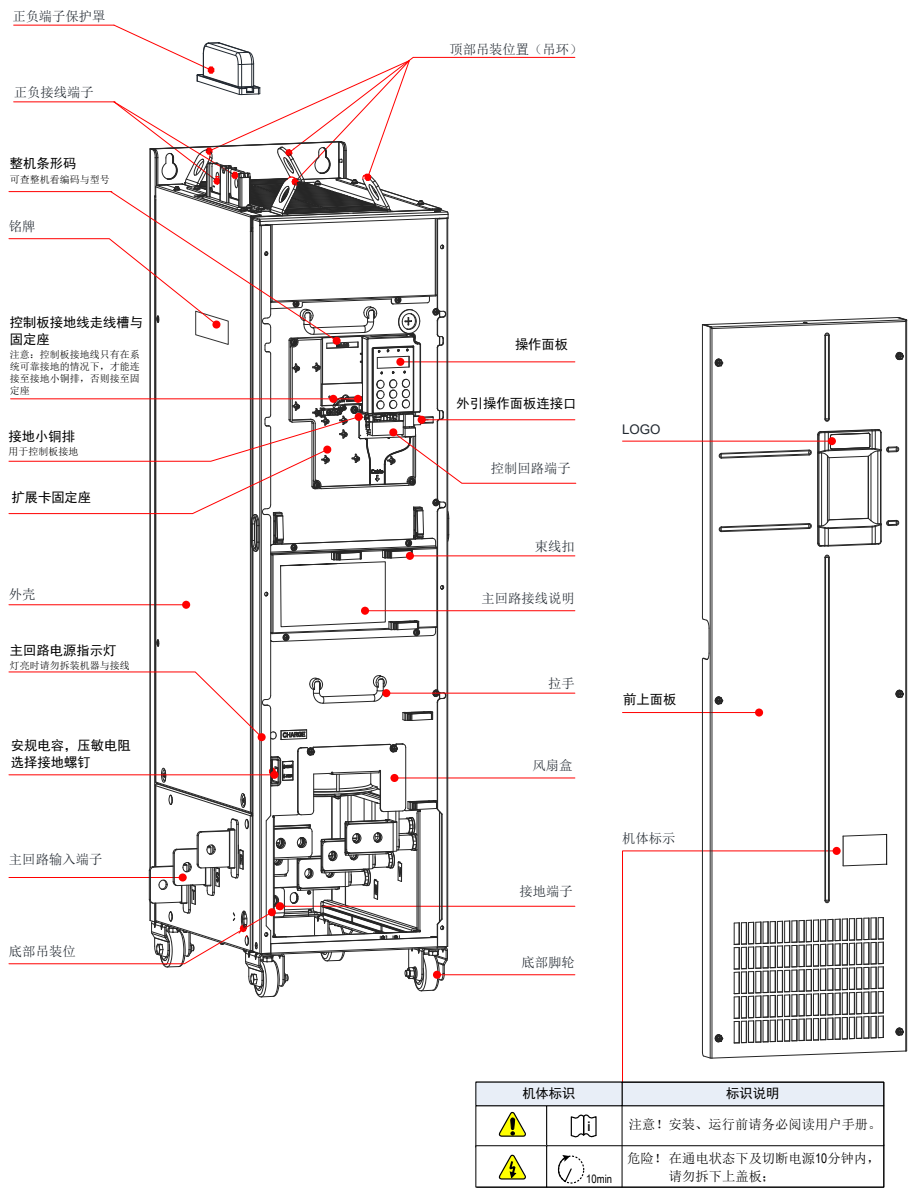
图 1-5 产品部件示意图【三相 380V~480V，CP300T200G ~ CP300T280G】
