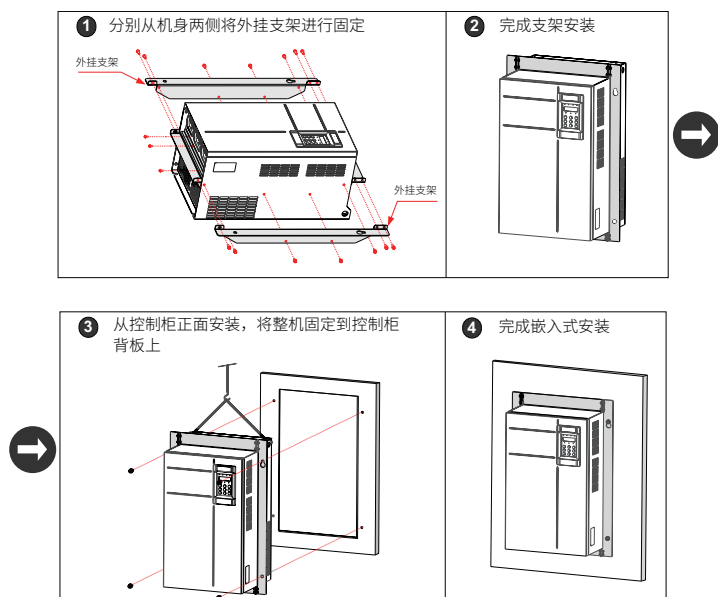
图 3-10 CP300T45G~CP300T160G 机型嵌入式安装示意图
