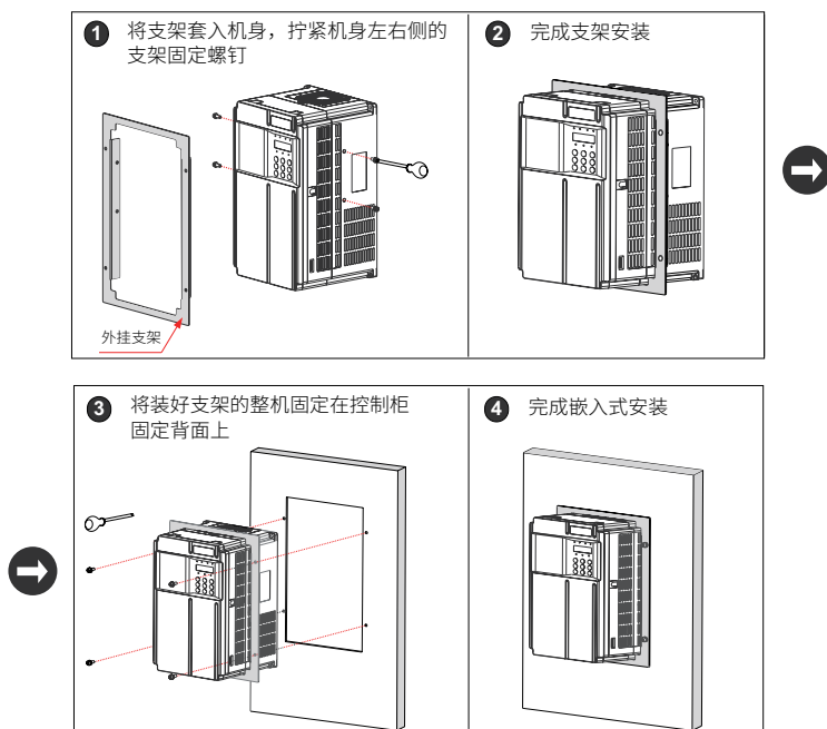
图 3-9 CP300T18.5GP~CP300T37G 机型嵌入式安装示意图
