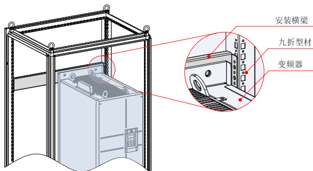
图 3-16 CP300T200G(-L)~CP300T280G(-L) 机柜 3D 示意图
