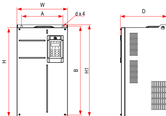
图 8-2 CP300T45G5-CP300T160G 外型尺寸及安装尺寸示意图
