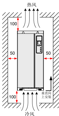
图 8-13 MDBUN 系列制动单元安装尺寸图 (单位: mm)
