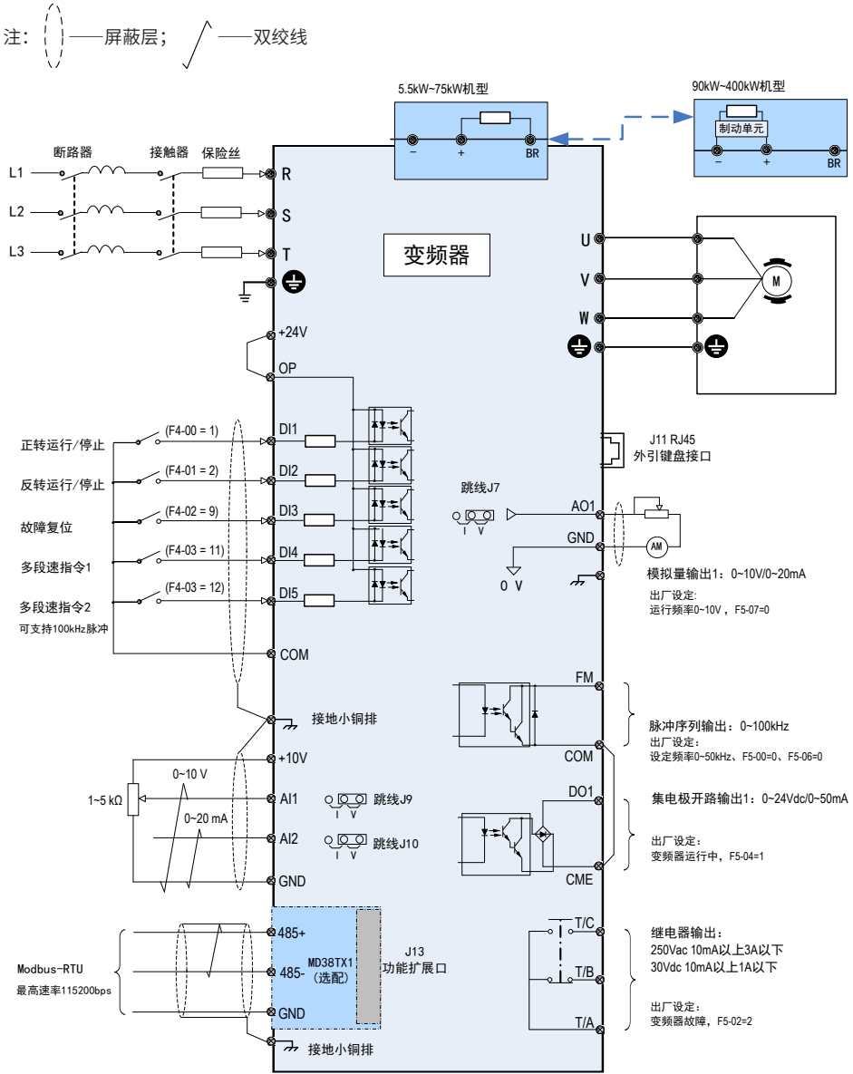
图 3-27 三相 380~480V 典型接线图
