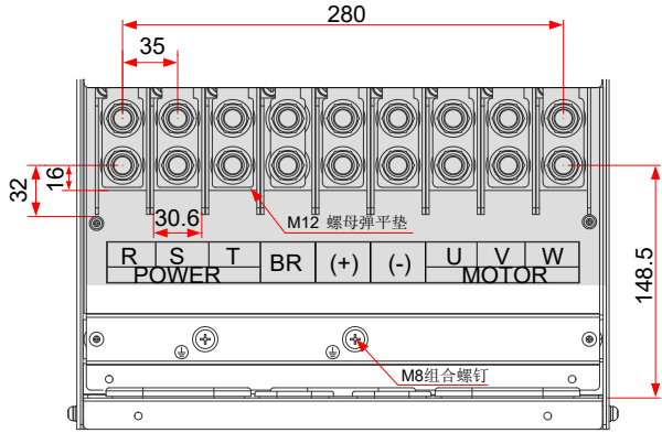
图 3-44 CP300T75G~CP300T110G 主回路端子尺寸
