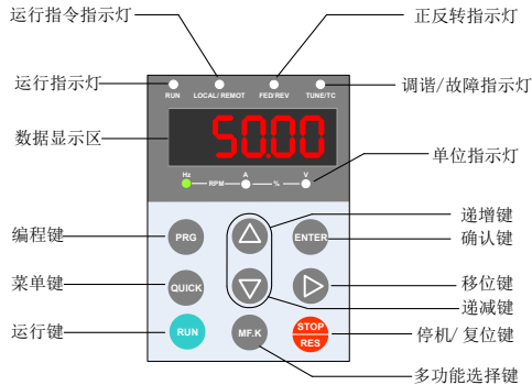
图 4-1 操作面板示意图
