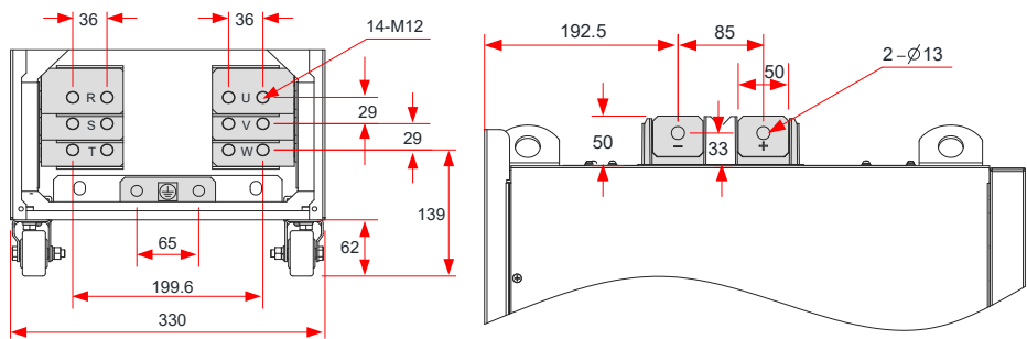
图 3-51 CP300T250G-L~CP300T280G-L 主回路端子尺寸（不带侧出铜排，不带输出电抗器）
