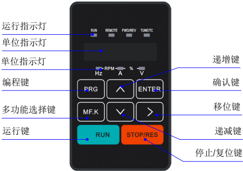
图 4-6 LED 外引操作面板 (MD310-KEY1) 外观示意图
