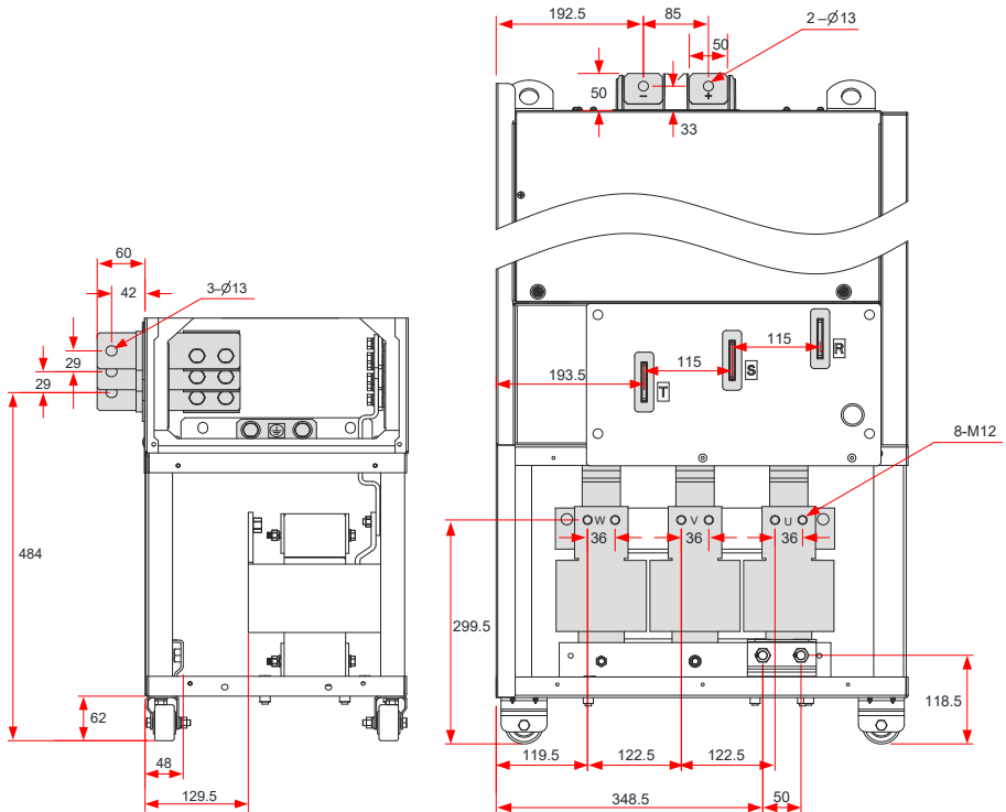
图 3-50 CP300T250G-L~CP300T280G-L 主回路端子尺寸（带输出电抗器）
