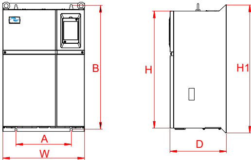
图 8-16 MD050 系列 AFE 单元外形尺寸图（单位：mm）
