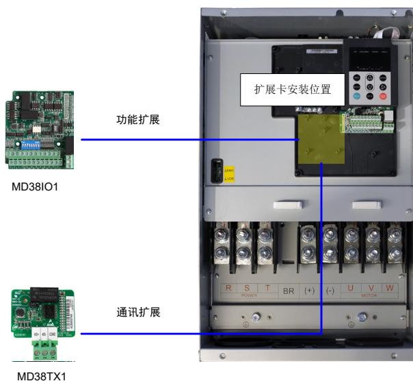
图 A-1 扩展卡的安装位置
