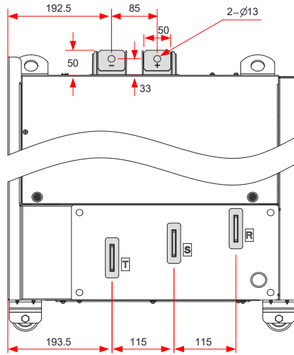
图 3-49 CP300T250G~CP300T280G 主回路端子尺寸（不带输出电抗器）
