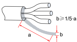
图 3-35 电机电缆屏蔽层引出示意图
