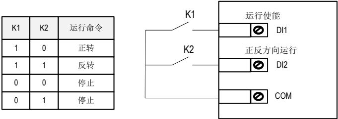
图 5-5 两线式模式 2
