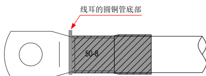
图 3-36 线缆导体加套管热缩示意图
