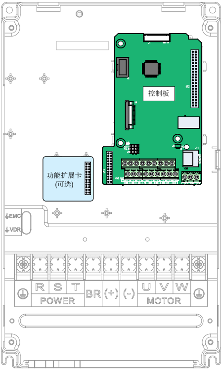
图 3-52 CP300 控制板
