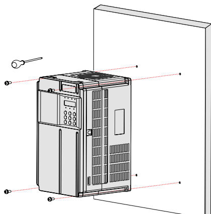
图 3-7 CP300T5.5G~CP300T37G 机型壁挂式安装示意图
