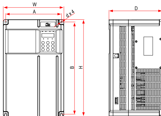
图 8-1 CP300T5.5G-CP300T37G 外型尺寸及安装尺寸示意图
