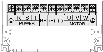
图 3-28 CP300T5.5G~CP300T160G 主回路端子分布图
