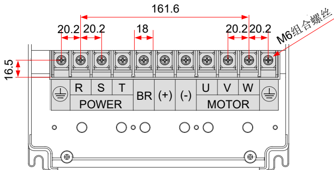
图 3-42 CP300T30G~CP300T37G 主回路端子尺寸
