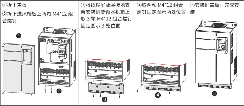
图 3-34 线缆屏蔽层接地支架安装示意图
