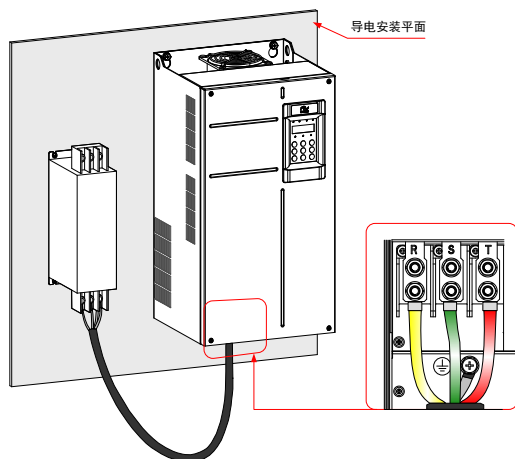
图 3-32 滤波器安装示意图
