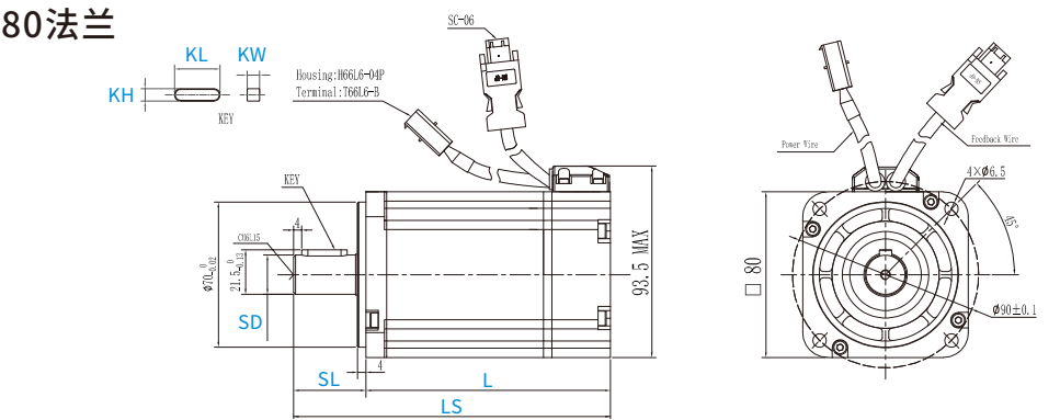
80法兰 (带抱闸)
