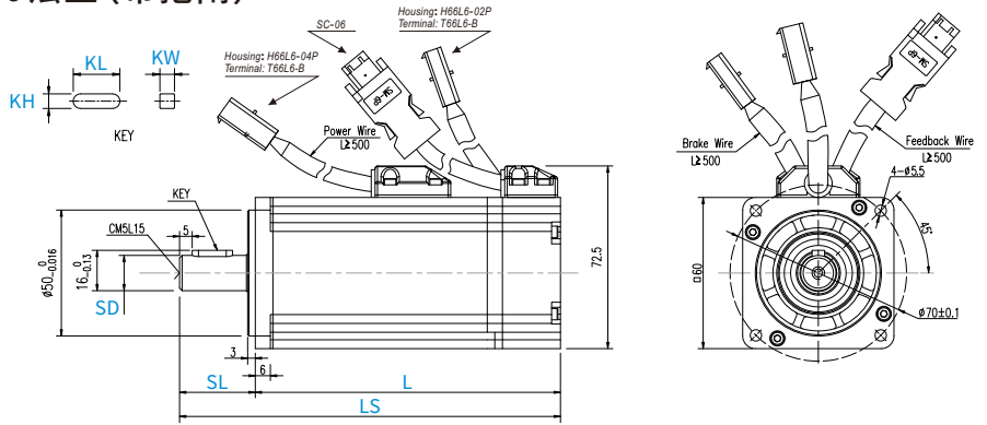
60法兰(带抱闸)
