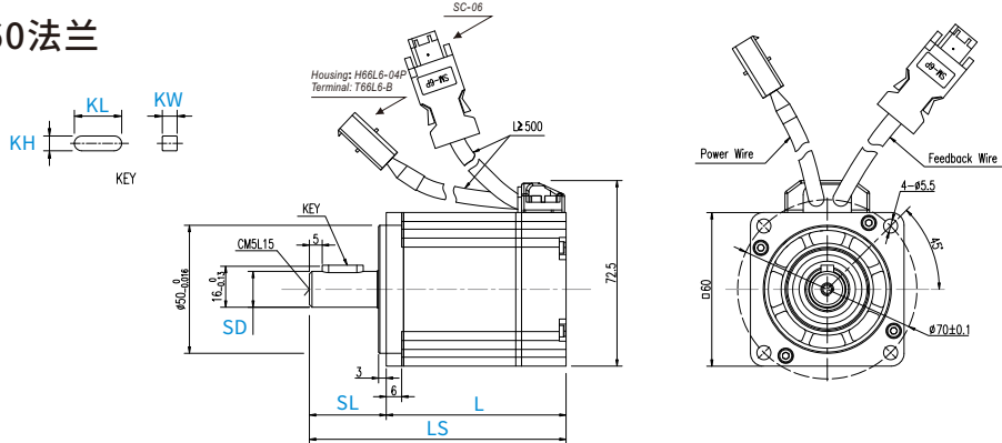
60法兰(带抱闸)
