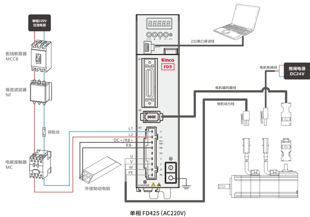
单相 FD425 (AC220V)
