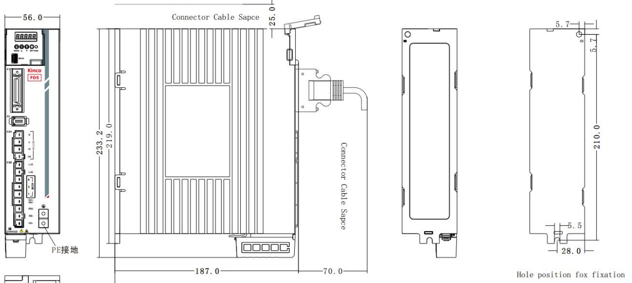
图 2-3 FD435-□A 产品安装图
