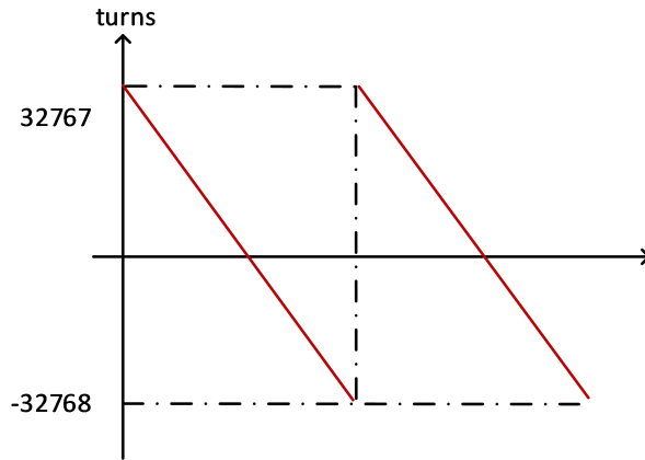
图 6-15 多圈数据范围
