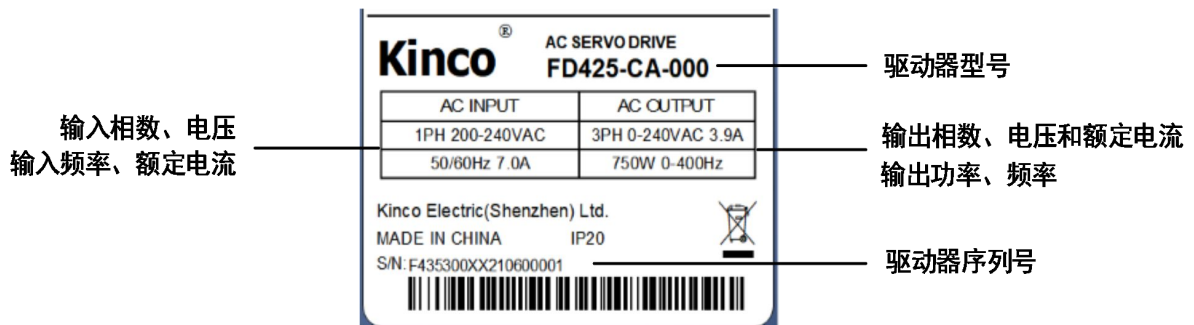
图 1-2 驱动器铭牌说明
