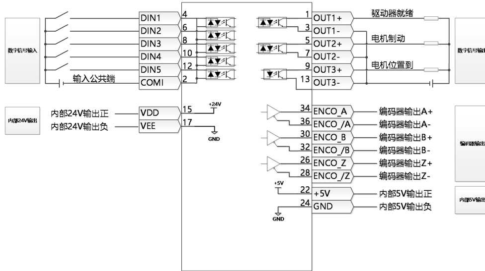
图 3-20 FD5-PA 驱动器 IO 口默认定义
