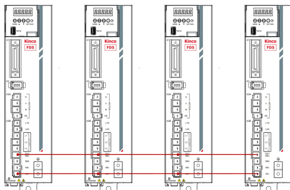
图 3-14 FD425 共直流母线
