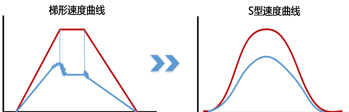
图 7-7 S 型速度阶跃曲线
