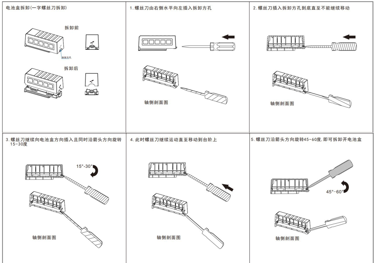
图 6-16 电池盒拆卸方式
