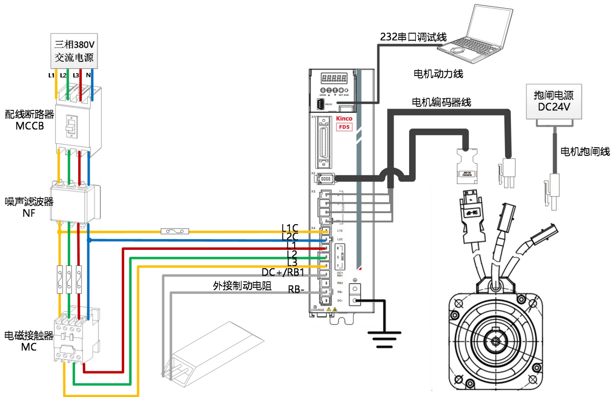
图 3-5 FD625 外部接线图
