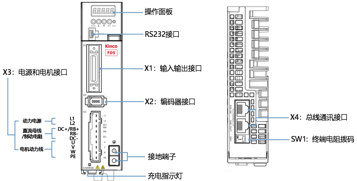
图 3-1 FD425 驱动器外观图
