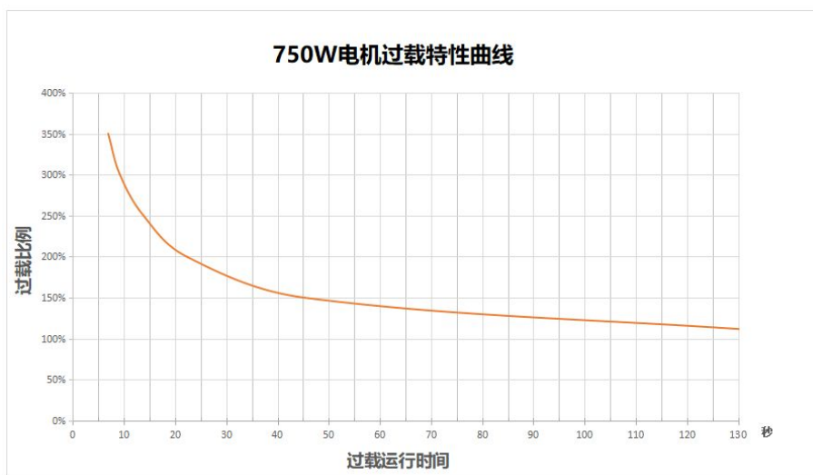
图 3-13 750W 电机过载特性曲线
