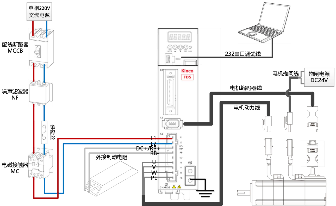
图 3-3 FD425 外部接线图
