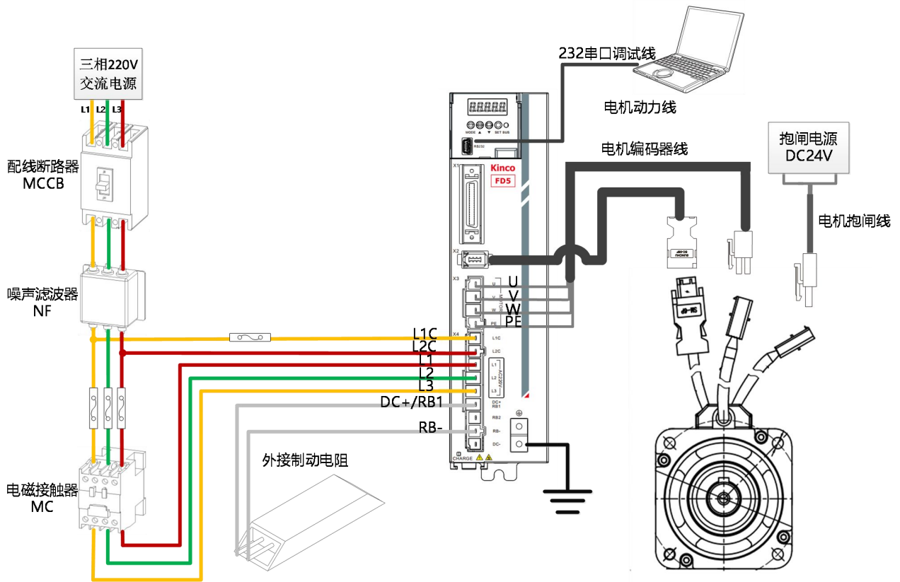
图 3-4 FD435 外部接线图
