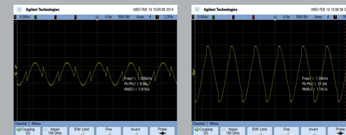
1. 当输出频率小于负载谐振频率, 电流波形有明显缺失, 输出电流较小, 内部功率模块发热较严重。 2. 当输出频率等于负载谐振频率, 电流波形无明显缺失, 输出电流大, 电源效率高。
