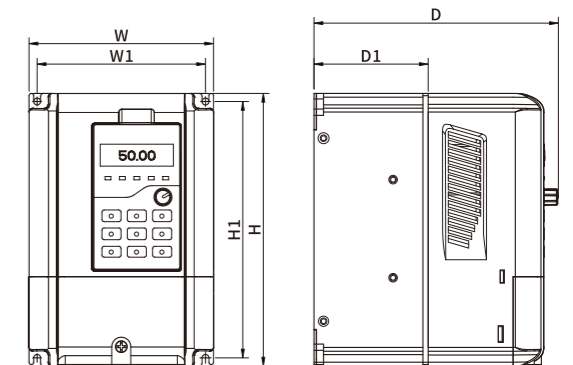
HP20-2S-0007G ~ HP20-000-00185G
