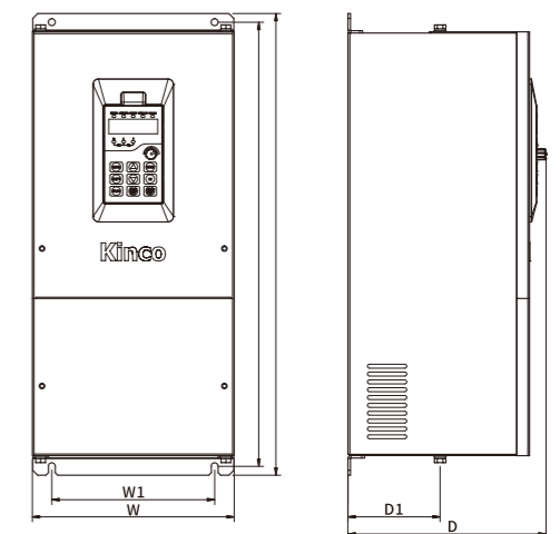
HP20-000-00220G ~ HP20-000-06000G
