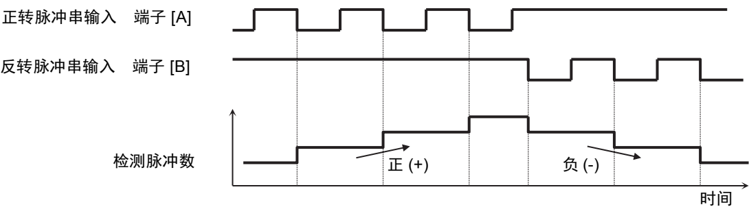
(c) 模式 2: [CA-91]=02 正转脉冲串+反转脉冲串
