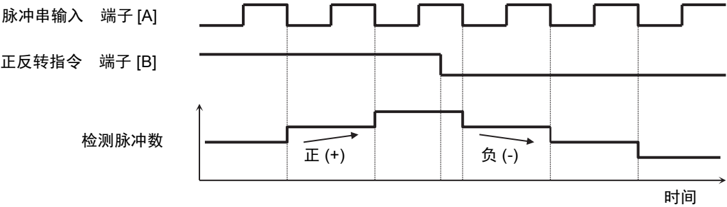
(b) 模式 1: [CA-91]=01 正反转指令+脉冲串
