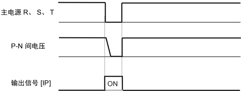
瞬时停电示例
