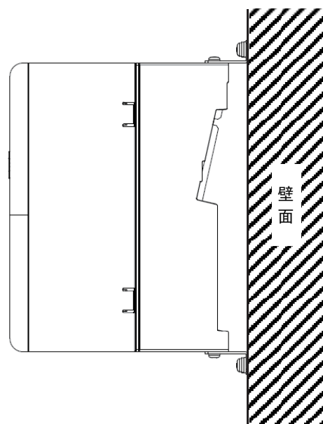
平面·右侧面图
