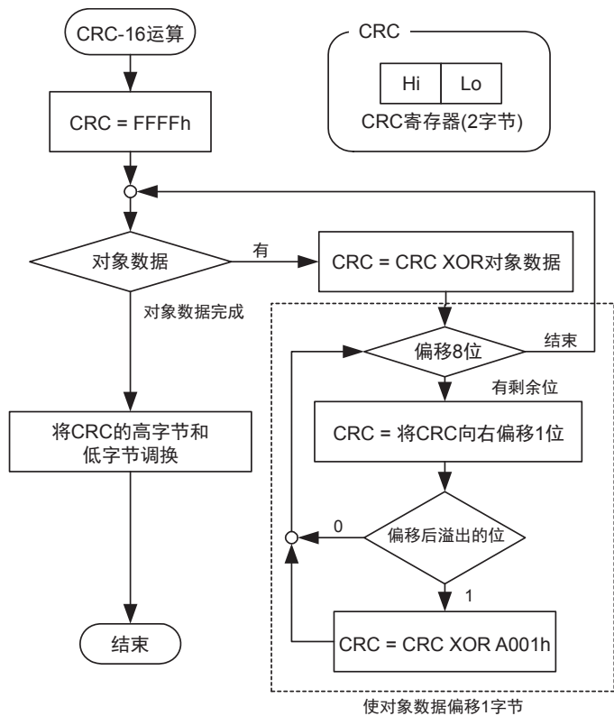
CRC-16 计算步骤例
