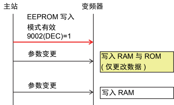
数据写入模式
