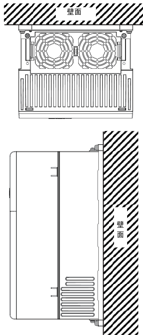
平面·右侧面图
