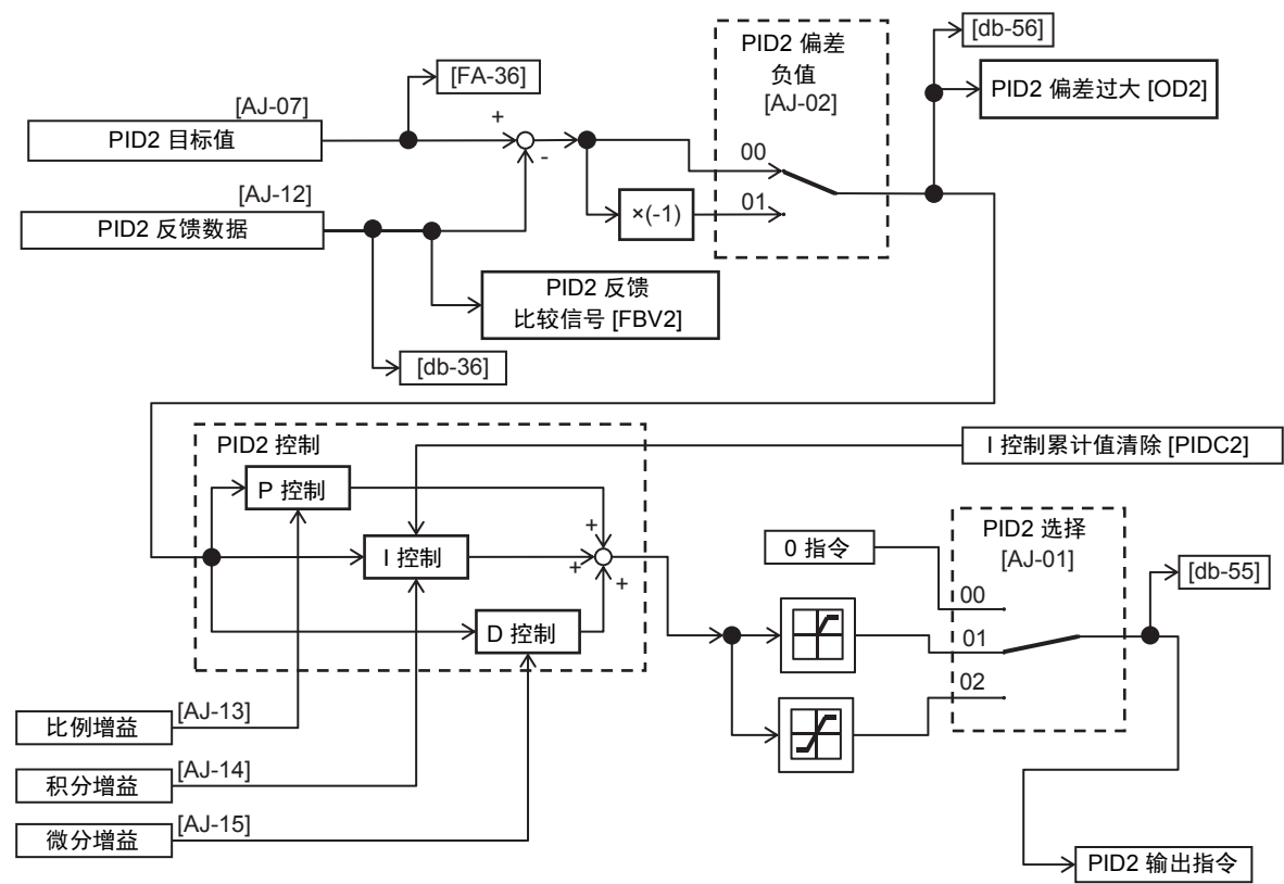
PID2 控制的概略图
