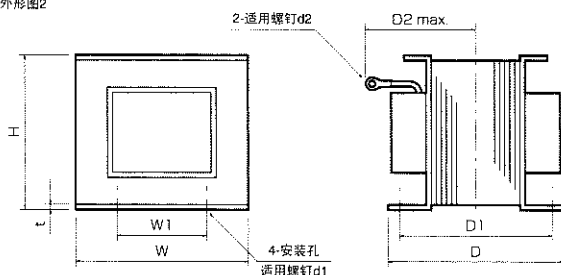
外形图2
