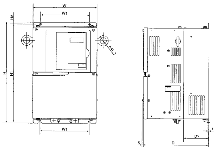
外形图: B
