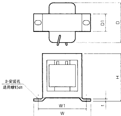
外形图1
