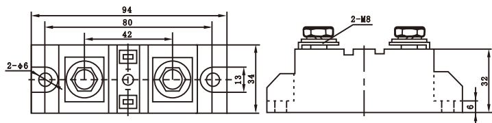
200-350A外形及安装尺寸图
