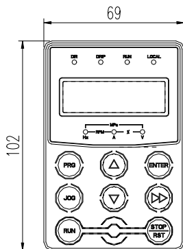
图 2-7 KEYC
