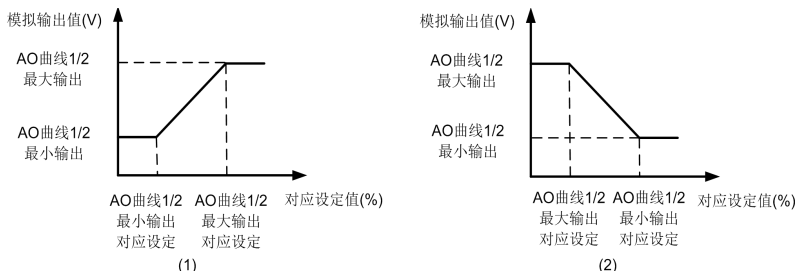
图 6-15 AO 曲线作用示意图
