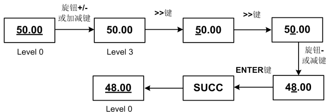
图 4-13 快速编辑操作示例——频率设定
