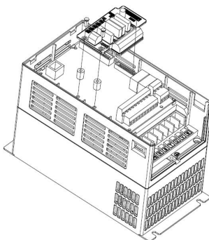
图 10-1 扩展卡安装示意图
