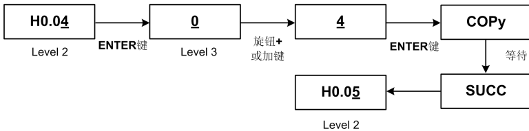
图 4-18 参数下载操作示意图
