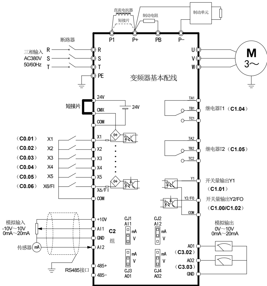
图 3-21 CDE500 矢量变频器接线示意图
