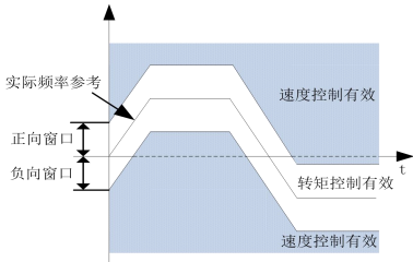
图 6-26 速度限幅模式 4
