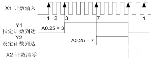
图 6-44 设定计数值到达和指定计数值到达示意图
