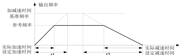
图 6-2 加减速时间示意图
