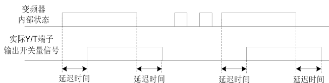
图 6-12 Y/T 端子（开关量输出）延迟时间作用示意图
