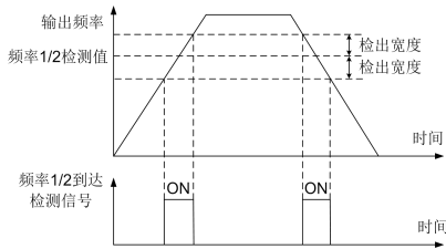
图 6-49 频率 1/2 到达功能示意图
