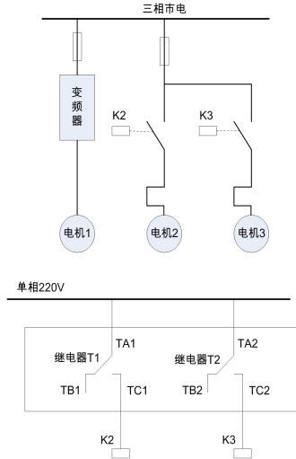
图 6-38 变频固定方式 (E6.00 = 1 或 2) 接线图
