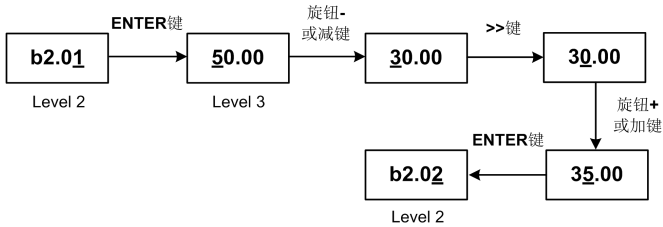
图 4-8 参数设置操作示例 1
