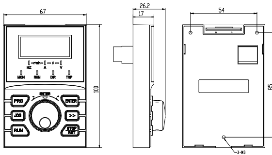
图 2-3 KEYA
