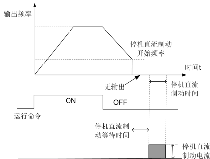
图 6-5 停机直流制动逻辑示意图
