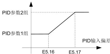
图 6-32 PID 有效参数与 PID 输入偏差的关系示意图
