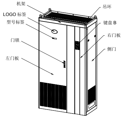
WG02 (钣金)
