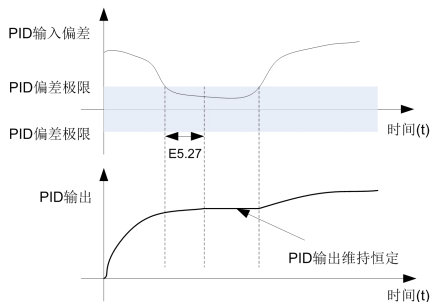
图 6-33 PID 偏差极限功能作用示意图
