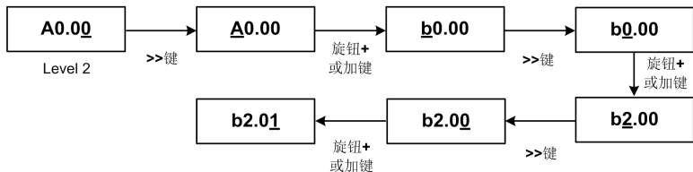
图 4-7 功能码选择操作方法（二）
