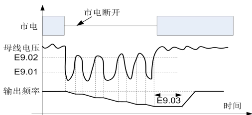
图 6-46 瞬停停电工作示意图（ E9.00 = 1）
