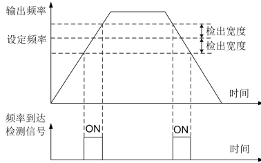
图 6-48 频率到达检测示意图
