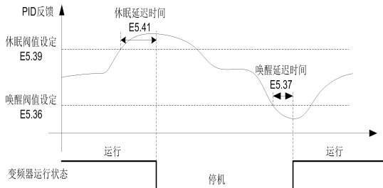
图 6-36 依据 PID 反馈进行休眠（ E5.38=1 ）的工作模式
