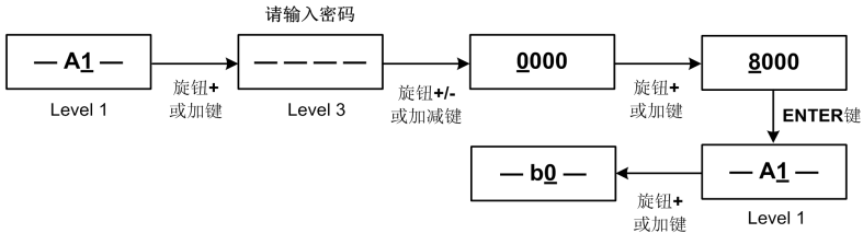
图 4-15 验证密码操作示例流程图
