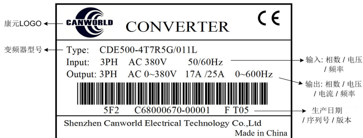
图 2-2 铭牌标贴
