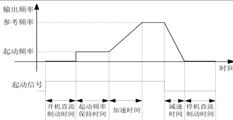
图 6-4 从启动频率启动（ b1.05 = 0 ）逻辑示意图
