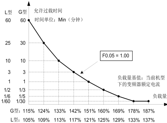
图 6-54 变频器过载保护反时限特性曲线
