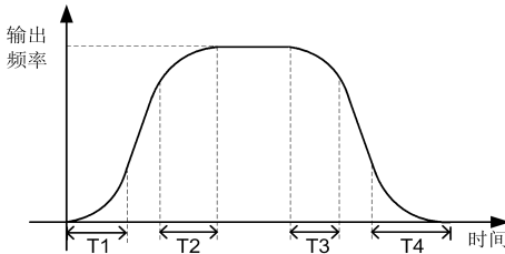
图 6-3 S 曲线加减速示意图
