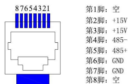
图 3-37 键盘接口脚位示意图
