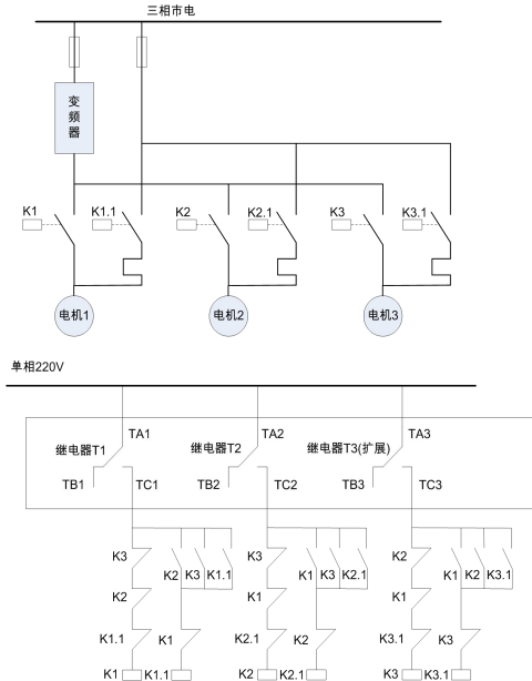
图 6-39 变频循环方式 (E6.00 = 3 或 4) 接线图
