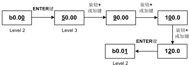
图 4-10 参数设置操作示例 2 方法（二）
