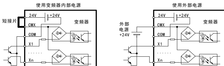
图 3-43 源极接线方式
