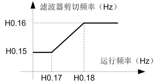
图 6-56 运行频率和滤波器剪切频率之间的关系
