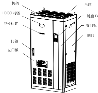
WG01 (钣金)
