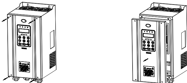
图 3-18 IP54 机型面盖拆卸
