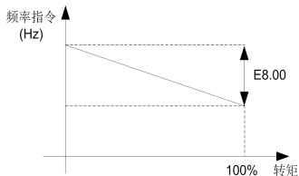
图 6-45 下垂控制作用示意图
