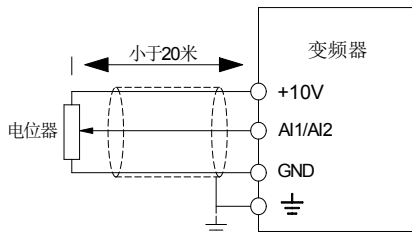
图 3-39 模拟输入端子接线图 1
