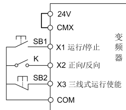
图 6-11 三线式 2 配线示意图
