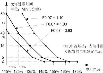
图 6-55 电机过载反时限特性曲线及示例
