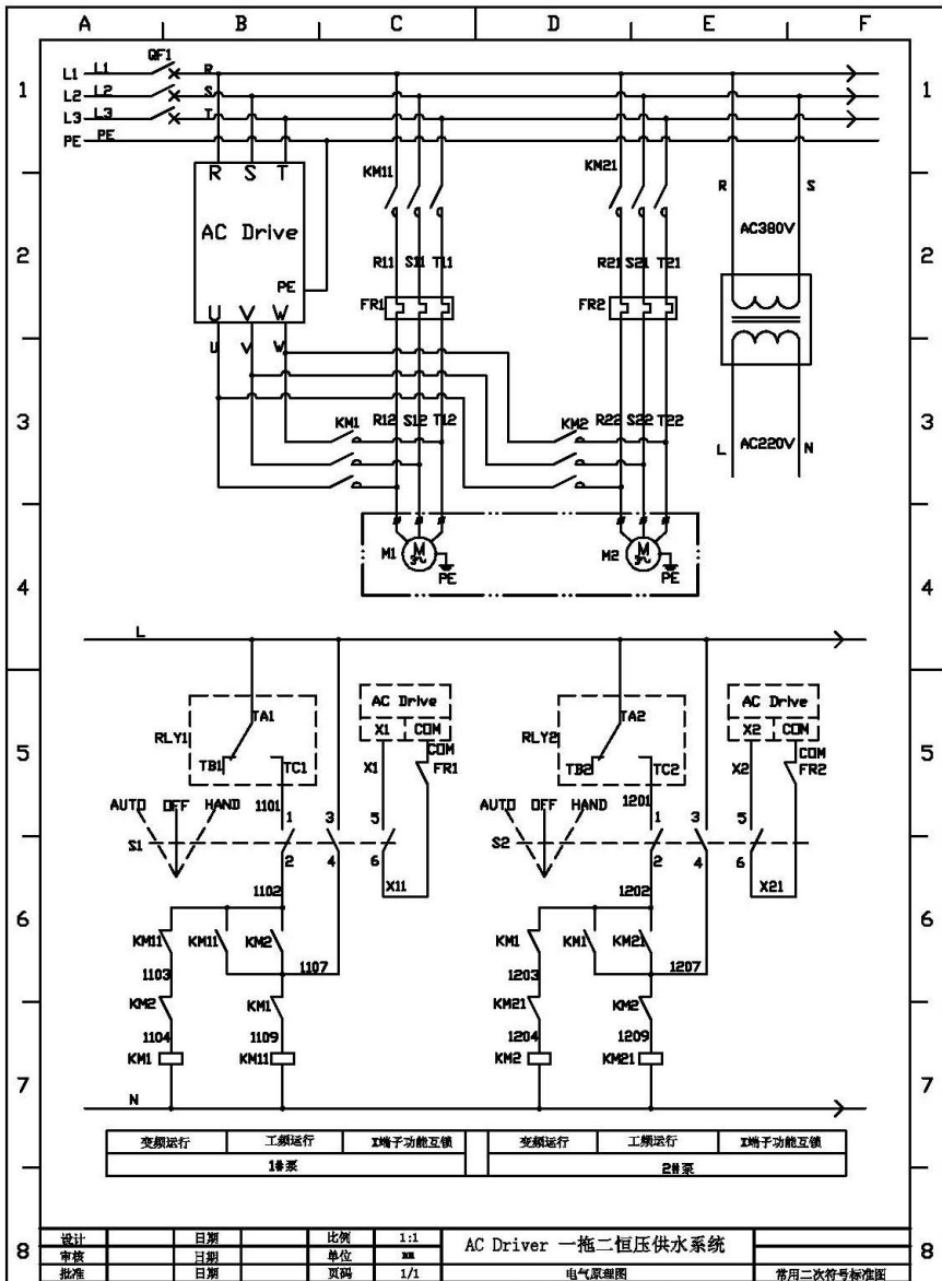
图 6-42 多泵控制一拖二供水接线原理图
