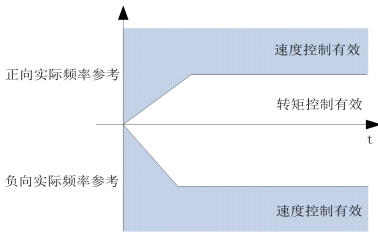
图 6-24 速度限幅模式 2
