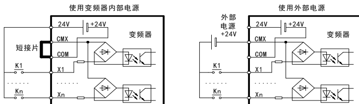
图 3-42 干接点共阳极接线示方式
