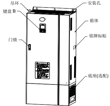
W06 (钣金)
