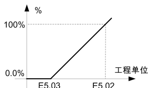
图 6-31 工程单位值与变频器内部标幺量对应关系
