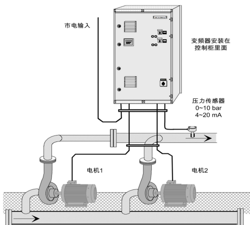
图 6-37 多泵控制接线示意图
