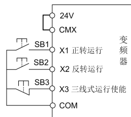
图 6-10 三线式 1 配线示意图
