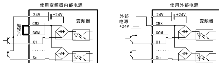
图 3-44 漏极接线方式
