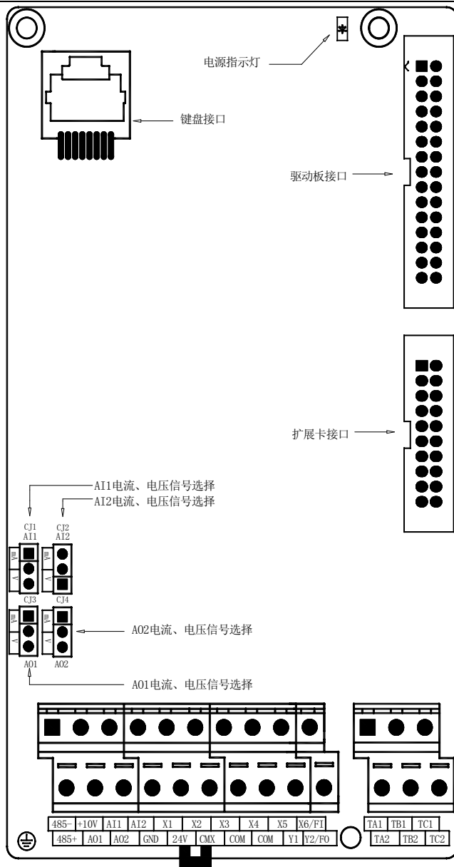
图 3-38 CDE500 矢量变频器控制端子布局图
