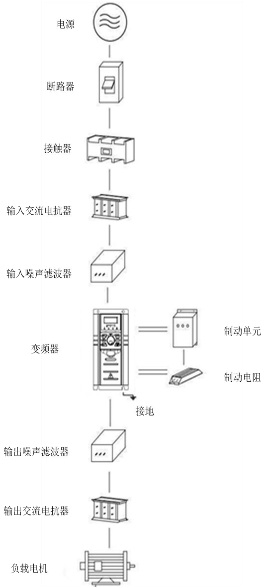
图 3-20 与外围设备的连接图
