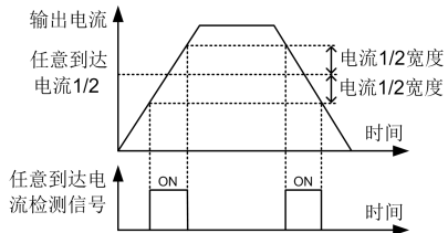
图 6-53 任意到达电流检测示意图
