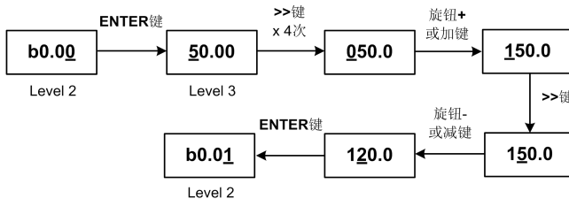
图 4-9 参数设置操作示例 2 方法（一）
