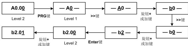
图 4-6 功能码选择操作方法（一）
