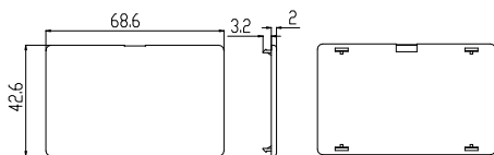
图 2-8 防尘板 A
