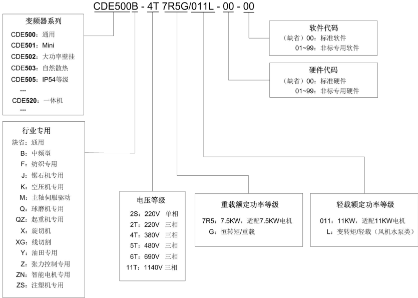
图 2-1 产品型号命名规则
