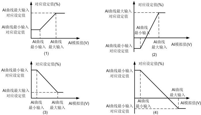
图 6-14 AI 曲线常见设置示意图
