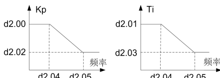
图 6-19 速度环高低速 PI 参数过渡示意图
