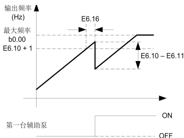
图 6-40 依据输出频率进行加泵逻辑示意图
