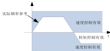
图 6-27 速度限幅模式 5
