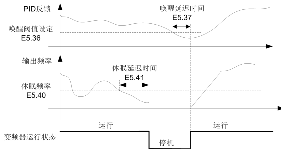
图 6-35 依据输出频率进行休眠（ E5.38=0 ）的工作模式
