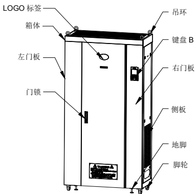
WG03 (钣金)
