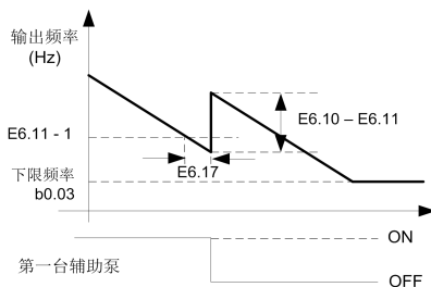
图 6-41 依据输出频率进行减泵示意图
