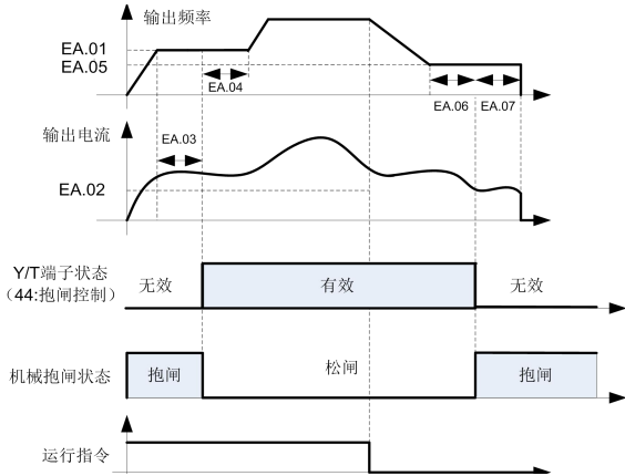
图 6-47 抱闸工作原理图
