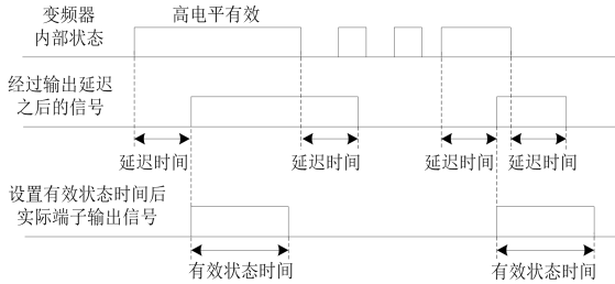
图 6-13 Y/T 端子(开关量输出)有效状态时间作用示意图
