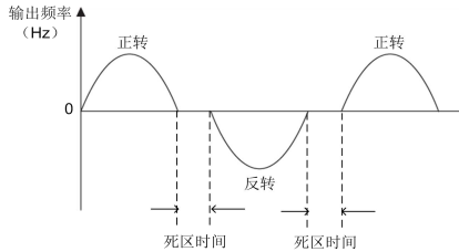
图 6-6 正反转死区时间示意图
