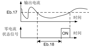
图 6-51 零电流检测示意图
