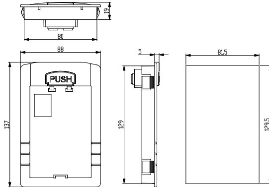
图 2-4 KEYA 底座
