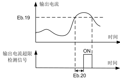
图 6-52 输出电流超限示意图
