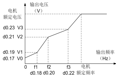
图 6-17 多段 V/F 曲线示意图
