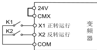
图 6-8 两线式 1 配线示意图
