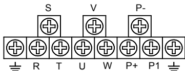
图 3-33 CDE500-6T037G/045L~075G/090L
