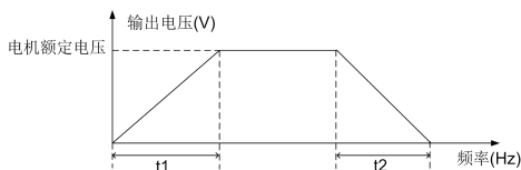
图 6-18 V/F 分离示意图
