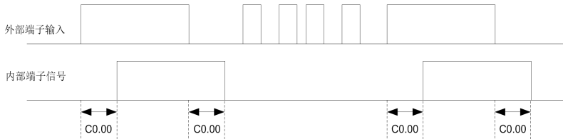
图 6-7 X1~X10 端子 (开关量输入) 滤波时间
