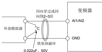
图 3-40 模拟输入端子接线图 2
