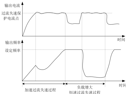
图 6-16 过流失速示意图
