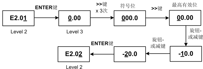
图 4-11 参数设置操作示例 3
