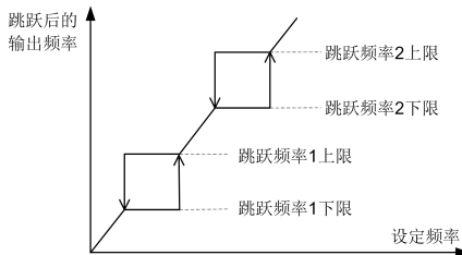
图 6-28 跳跃频率示意图
