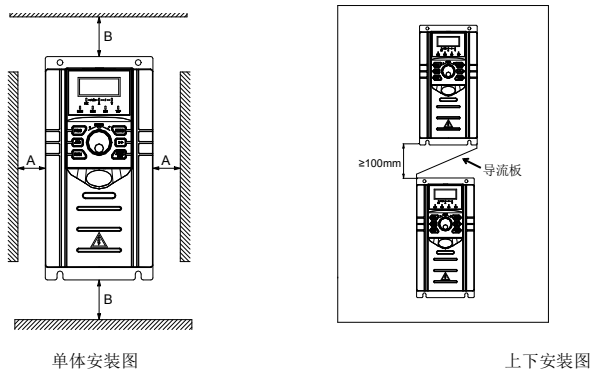
图 3-1 CDE500 系列变频器安装示意图
