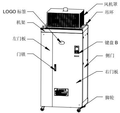
WG04 (钣金)
