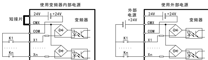
图 3-41 干接点共阴极接线方式
