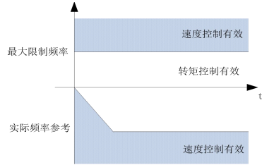
图 6-25 速度限幅模式 3
