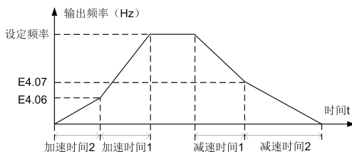
图 6-30 加减速时间切换示意图
