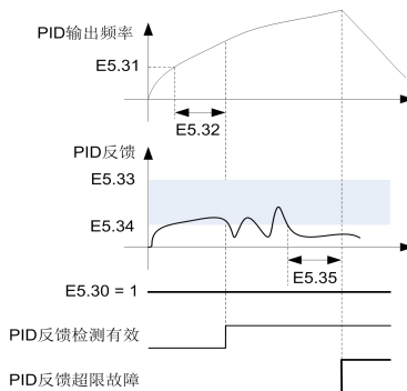
图 6-34 PID 反馈检测保护动作示意图
