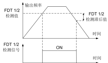
图 6-50 FDT 检测示意图
