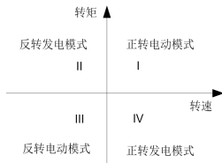
图 6-20 电机四象限运行示意图
