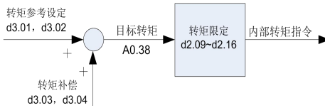
图 6-21 转矩参考作用示意图
