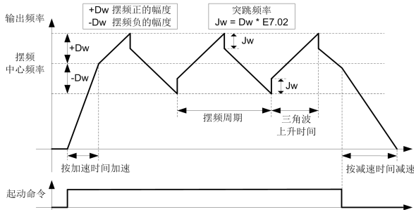
图 6-43 摆频示意图
