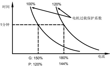
图 6-15 电机过载保护系数设定示意图
