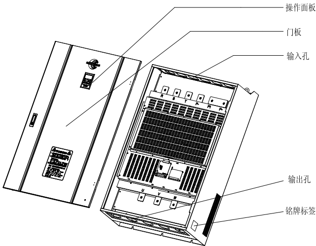
图 1-1 产品外型图
