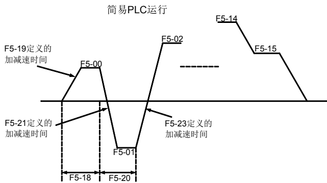
图 6-12 简易 PLC 运行示意图
