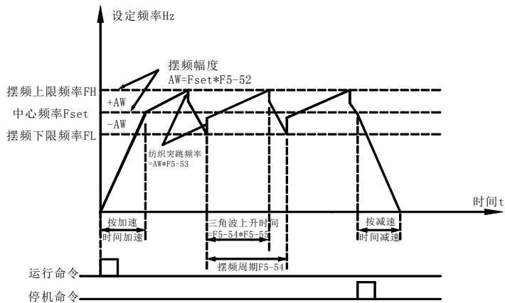
图 6-13 摆频工作示意图
