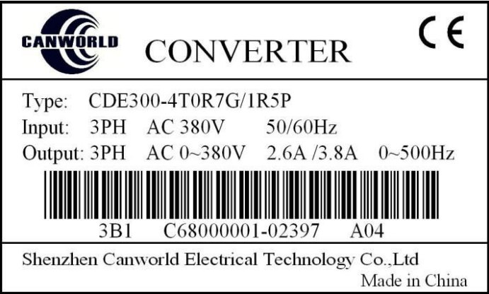
图 2-2 铭牌
