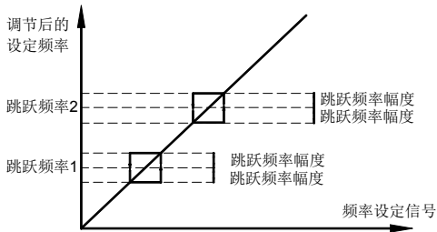
图6-8 跳跃频率示意图
