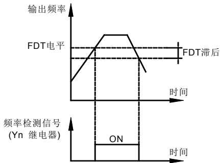
图 6-10 FDT 电平示意图
