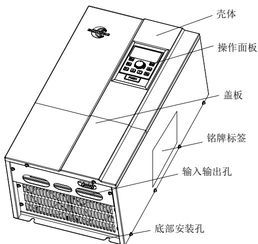
图 2-4 CDE300 5.5kW~132kW（铁壳）外型图
