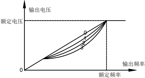
图 6-18 V/F 曲线示意图
