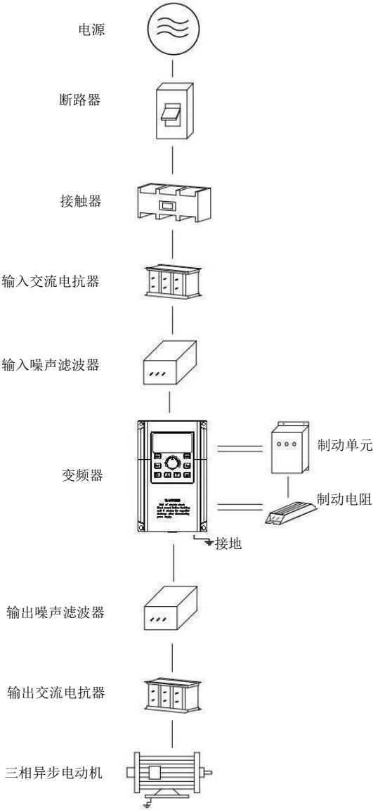
图 3-4 与外围设备的连接图
