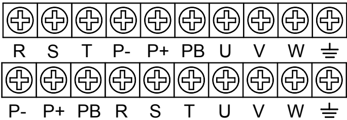
图 3-6 CDE300 0.75kW~2.2kW 主回路功率端子图
