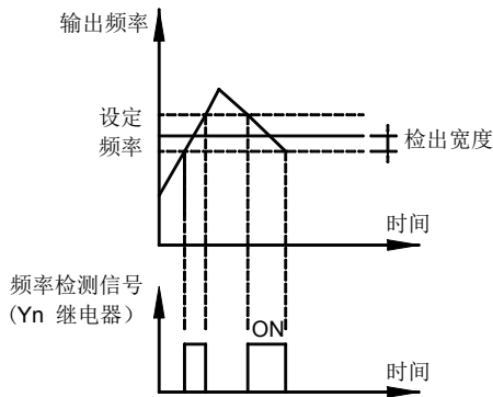
图 6-11 频率到达检出示意图
