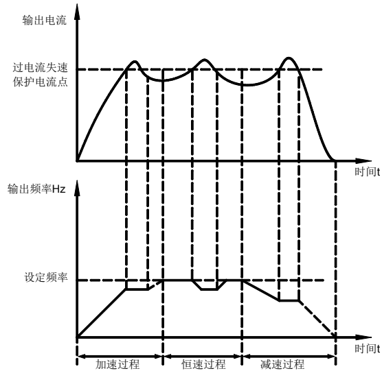
图 6-16 过流失速保护
