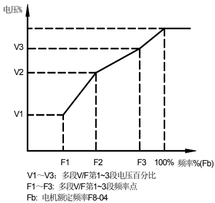
图 6-19 多点 V/F 曲线设定示意图
