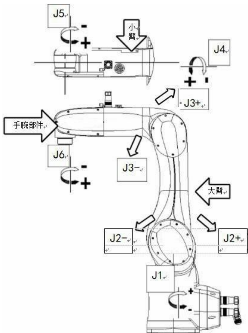
图 2.2.1 机器人机械系统组成图
