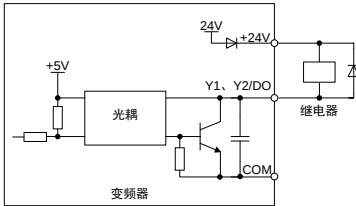
a) 使用内部电源
