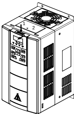
图 3-4 操作面板的拆卸
