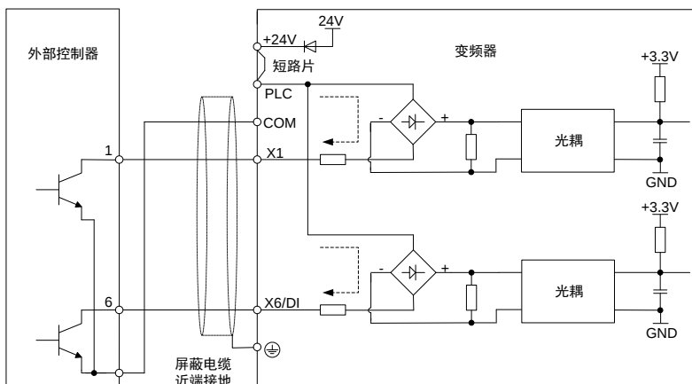
图 3-19 使用内部电源开路集电极 NPN 接线方式
