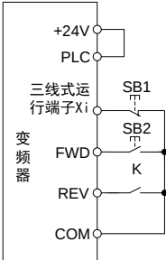
图 6-20 三线式模式 2
