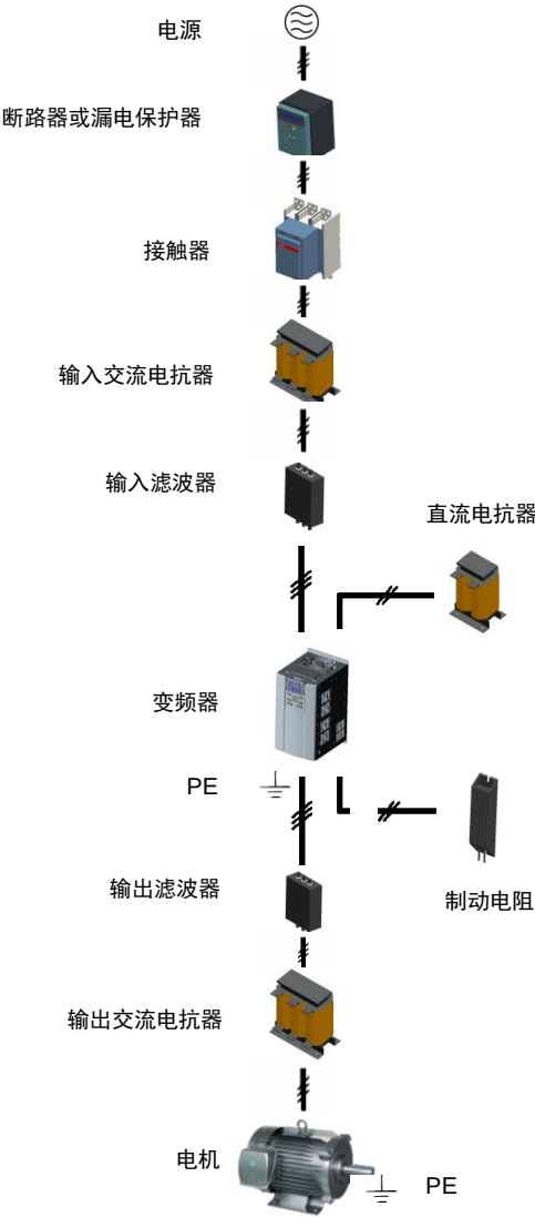
图 3-12 产品外围器件的标准配置图
