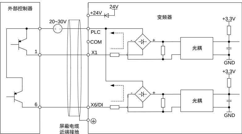
图 3-22 使用外部电源开路集电极 PNP 接线方式
