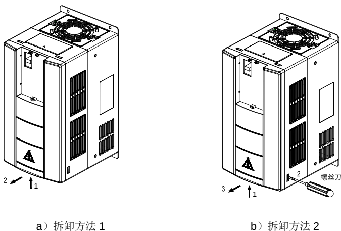
图 3-6 盖板的拆卸
