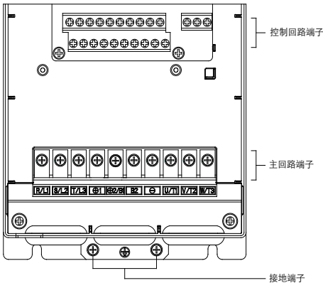
图 3-13 产品端子配置
