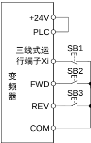
图 6-19 三线式模式 1
