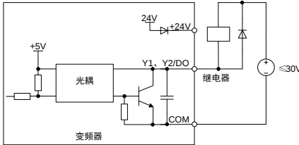
b) 使用外部电源
