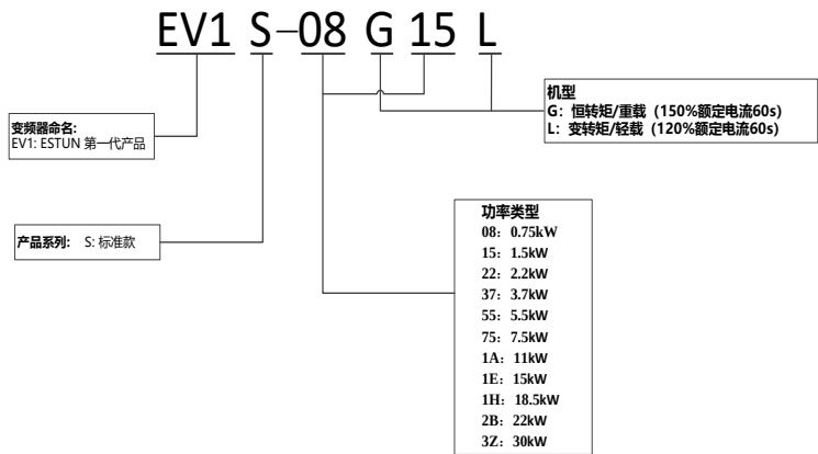
图 2-1 产品型号命名规则
