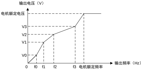
图 6-41 用户自定义多段 V/f 曲线
