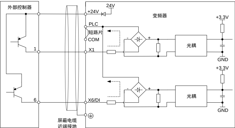
图 3-21 使用内部电源开路集电极 PNP 接线方式
