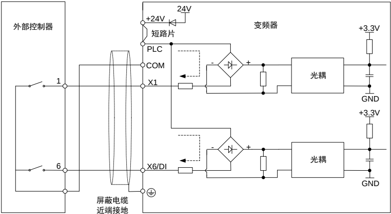
图 3-17 使用内部电源干接点方式
