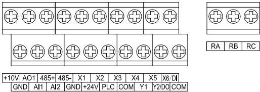
图 3-16 控制端子排列顺序
