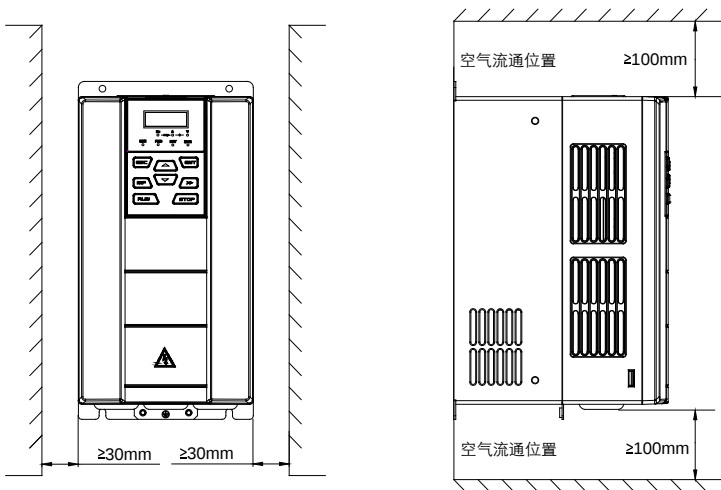
图 3-1 安装方向和空间要求
