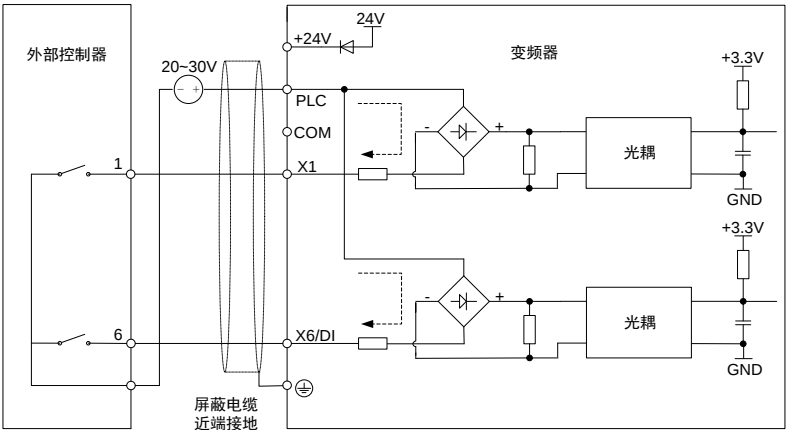
图 3-18 使用外部电源干接点方式
