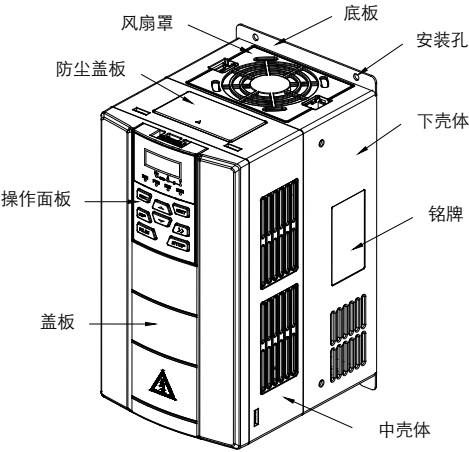
图 2-3 产品部件图
