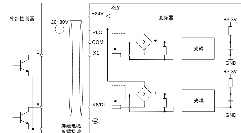
图 3-20 使用外部电源开路集电极 NPN 接线方式
