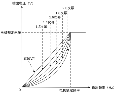
图 6-42 1.2~2.0 次幂 V/f 曲线
