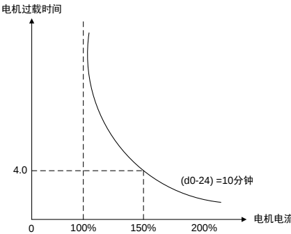
图 6-40 普通电机 10Hz 运行时的过载保护曲线
