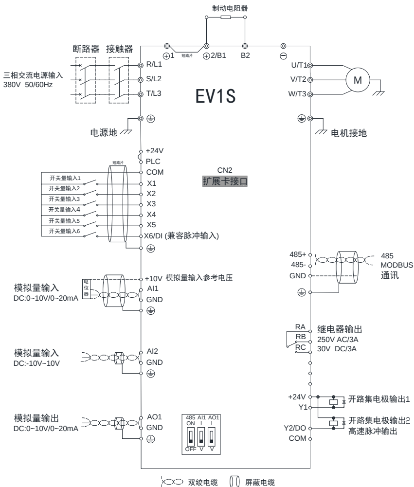
图 3-15 标准接线图
