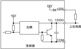
a) 使用内部电源
