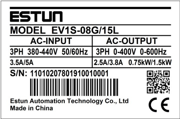
图 2-2 产品铭牌说明
