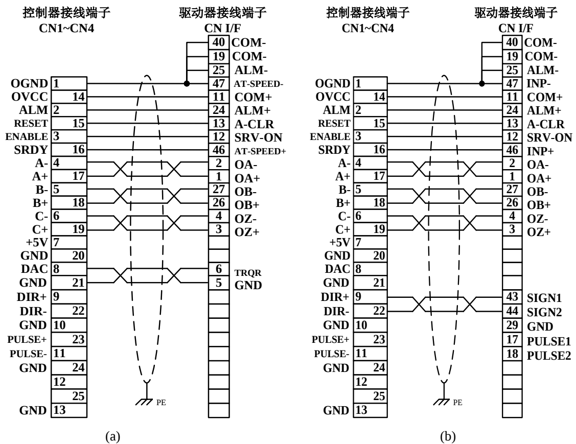
图 6-6 三洋 R2 系列驱动器速度控制方式接线
