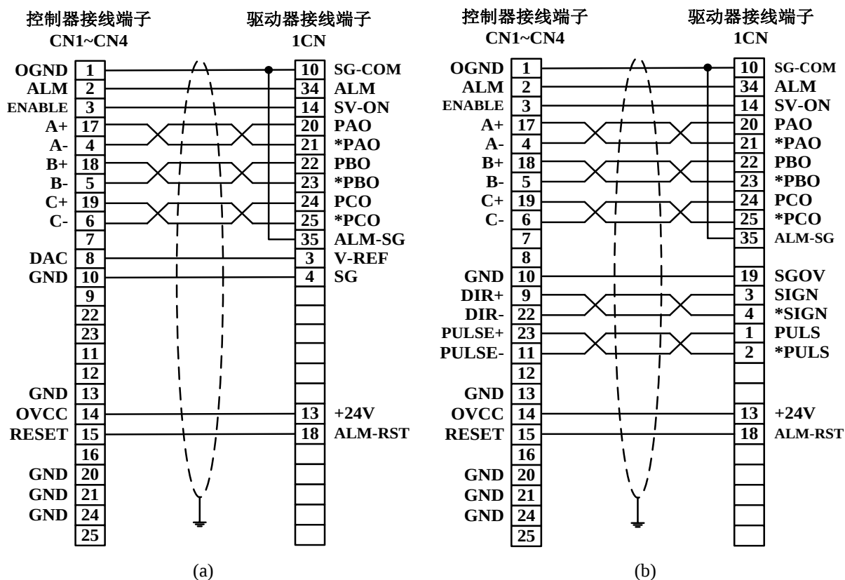
图 6-8 安川 YASKAWA SERVOPACK 系列驱动器速度&amp;力矩控制方式(a)接线/位置控制方式(b)接线
