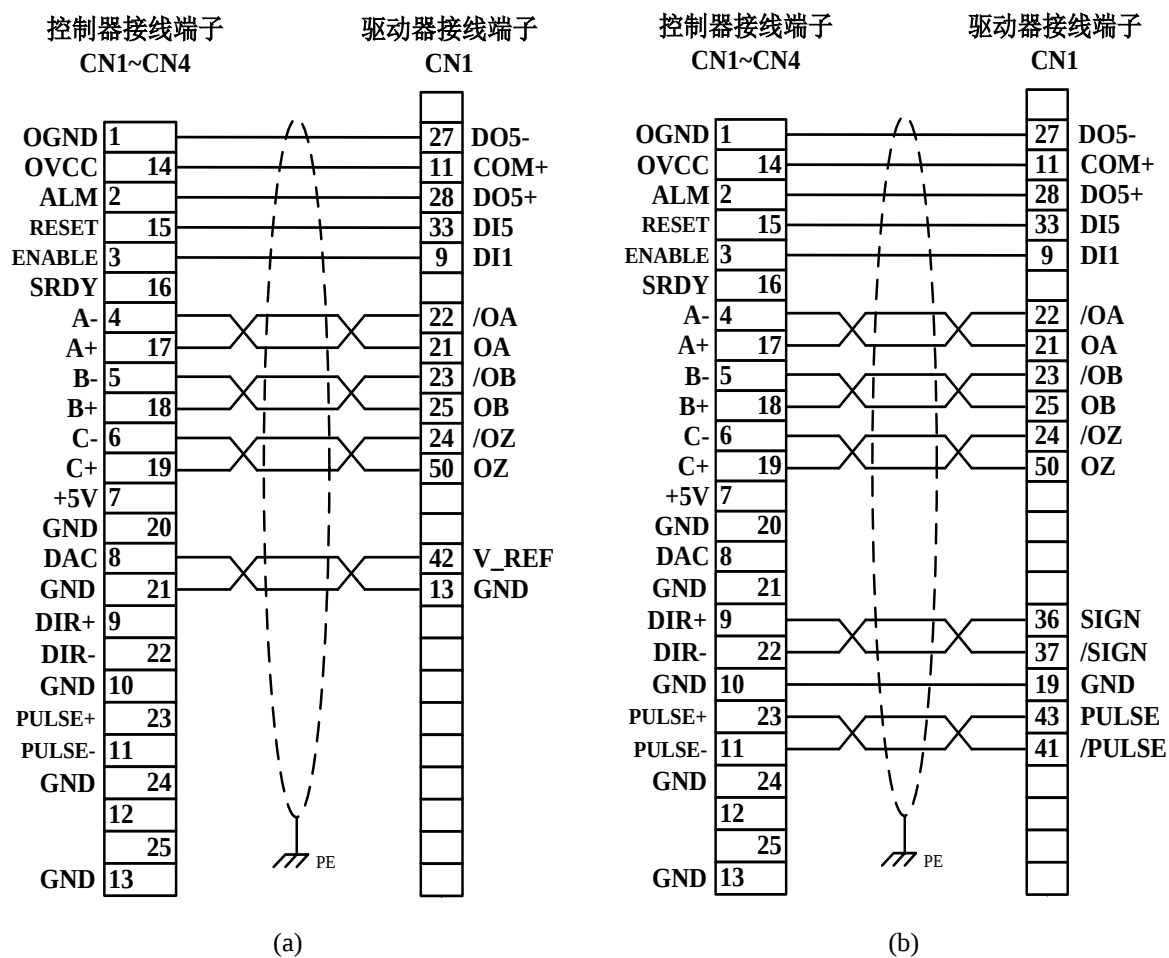
图 6-14 台达 ASDA-AB 系列驱动器速度控制方式(a)/位置控制方式(b)接线
