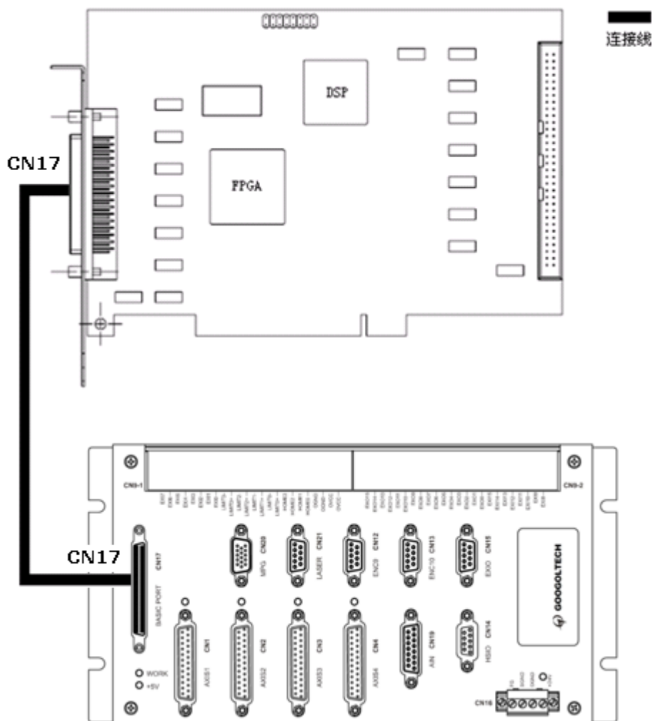
图 2-20 运动控制器与 4 轴端子板连接示意图
