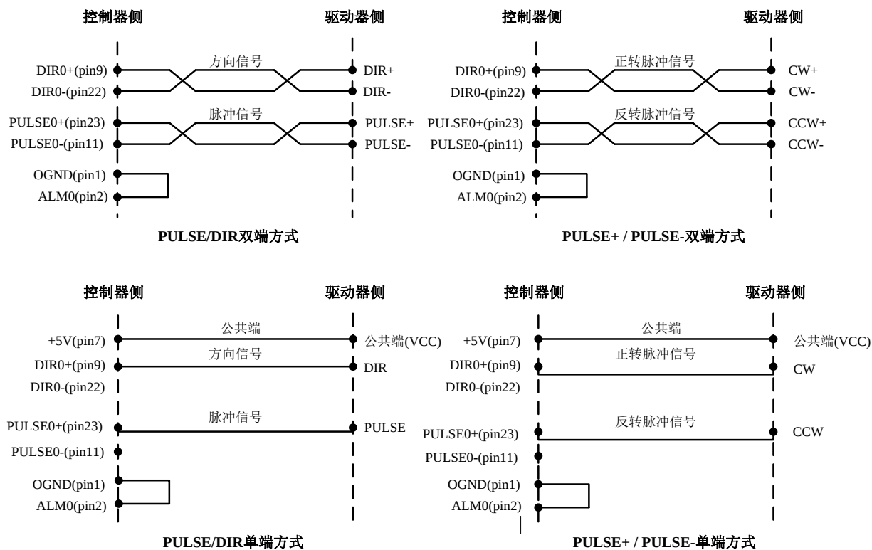
图 3-16 脉冲量输出信号连接图
