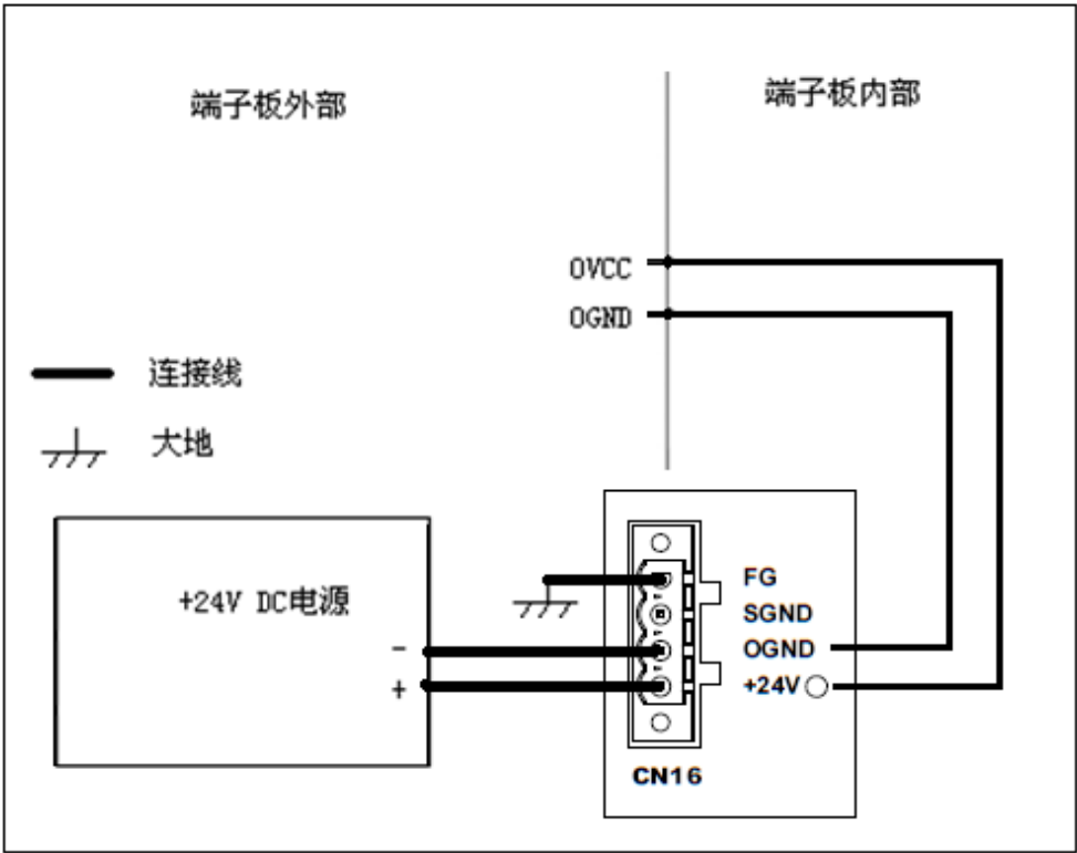
图 2-21 端子板电源连接图
