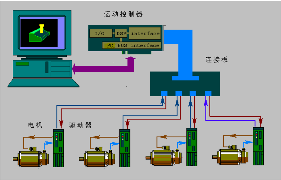
图 2-22 典型系统连接图
