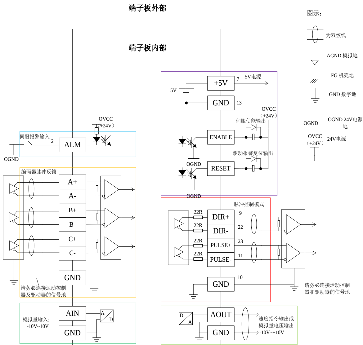
图 3-2 端子板轴信号接口内部电路
