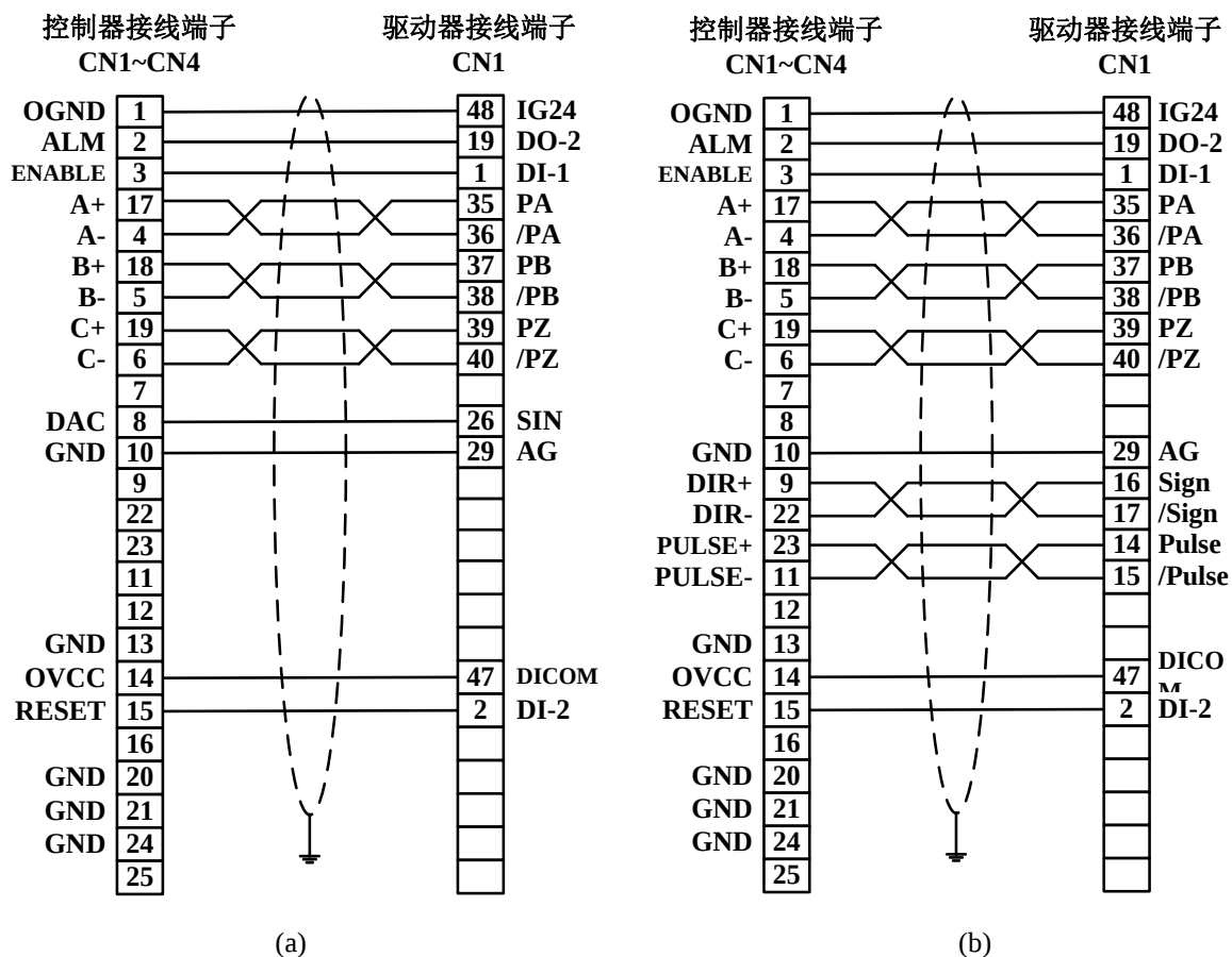
图 6-17 东元 TSTA 系列驱动器速度控制方式(a)/位置控制方式(b)接线
