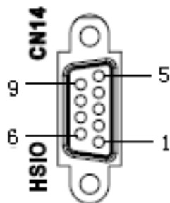
图 3-7 端子板 CN14 HSIO 接口引脚号说明
