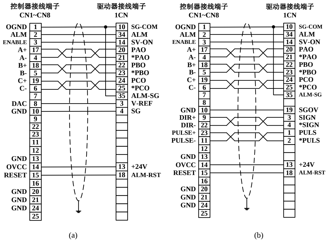
图 6-8 安川 YASKAWA SERVOPACK 系列驱动器速度&amp;力矩控制方式(a)接线/位置控制方式(b)接线
