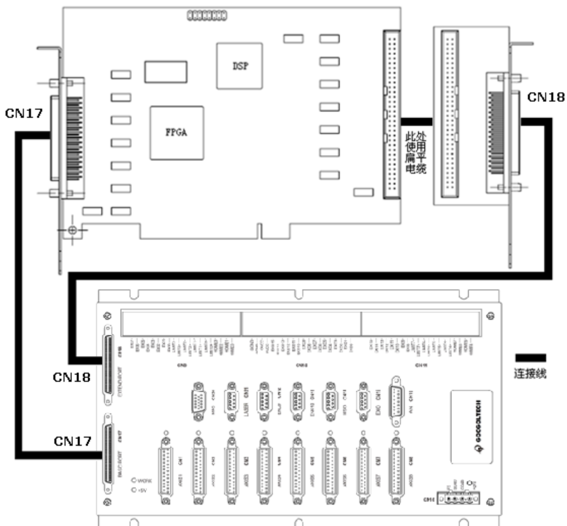
图 2-20 运动控制器与 8 轴端子板连接示意图
