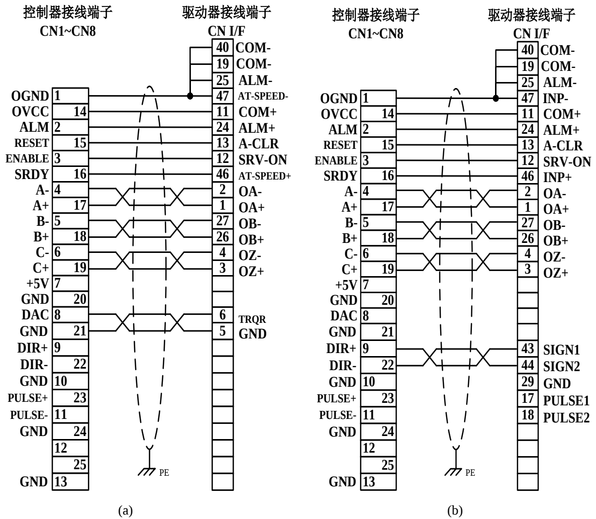
图 6-6 三洋 R2 系列驱动器速度控制方式接线
