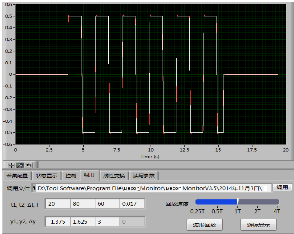
图 9.2.2-1 速度响应曲线 (白: 速度给定; 红: 速度反馈)
