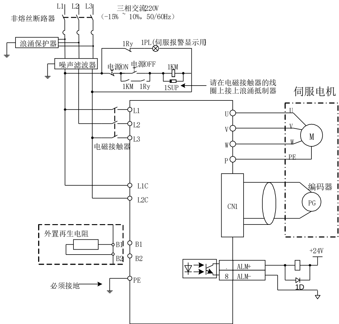
图 4.2.1-1 三相 220V 主电路配线
