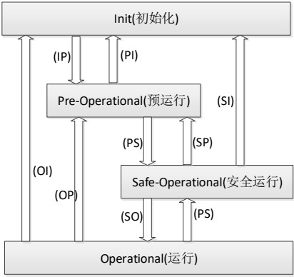
图 5.3.3-1 EtherCAT 状态机
