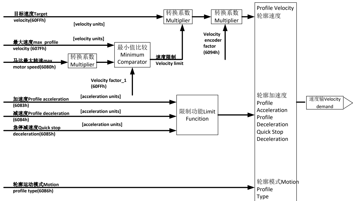
图 7.8.1-1 轮廓速度模式控制框图
