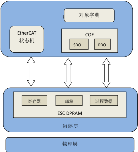
图 5.3.2-1 基于 CANOpen 应用层的 EtherCAT 通信结构
