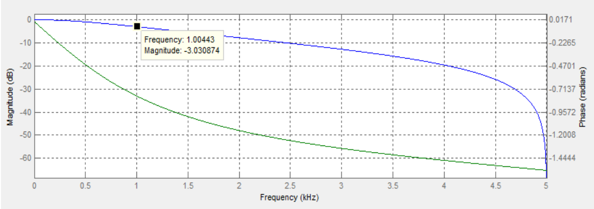
图 9.3.2-1 低通滤波器的伯德图
