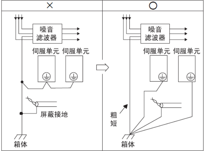
图4.7.2-3 单点接地示意图
