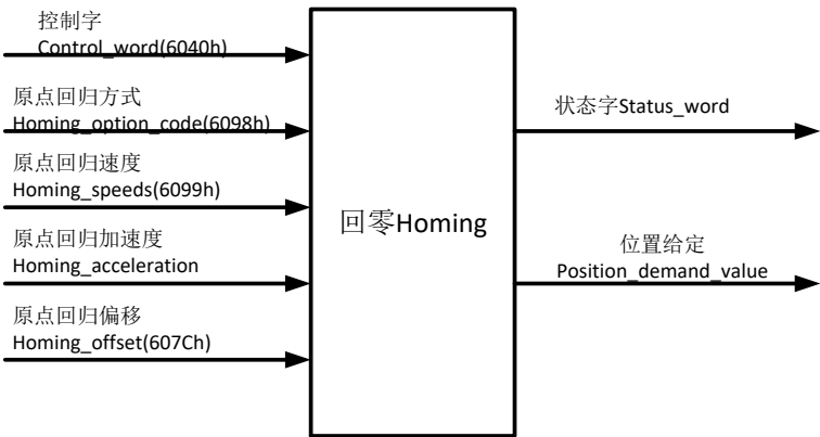
图 7.10.1-1 原点回归控制框图
