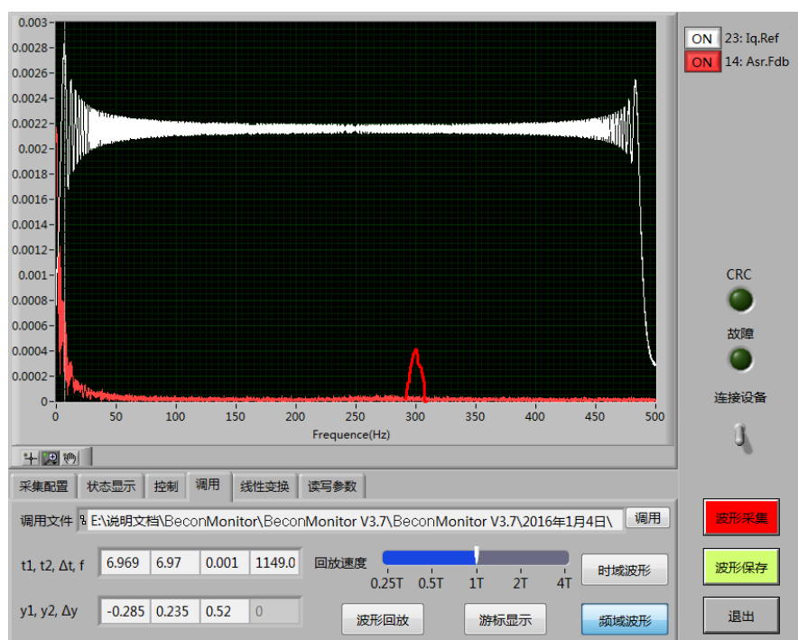
图 9.4.1-1 正弦扫频
