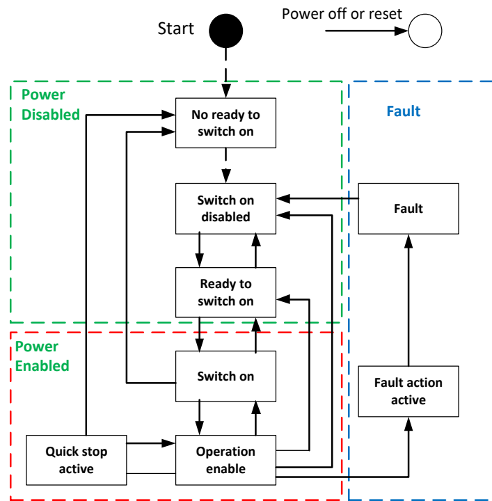
图 5.3.7-1 CIA402 状态切换图
