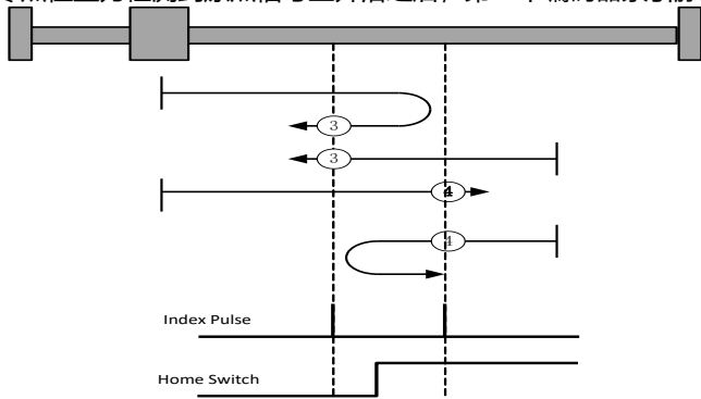
图 7.10.3-3 回零方法 3 和 4
