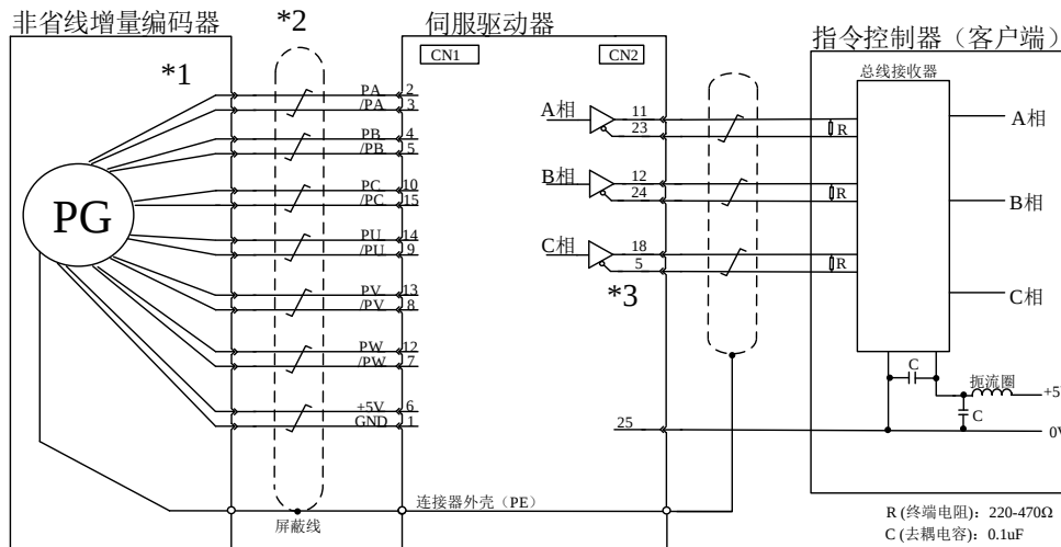
图 4.4.1-2 增量标准式编码器接线示意图
