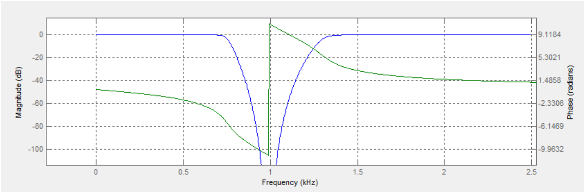
图 9.3.2-2 陷波滤波器的伯德图
