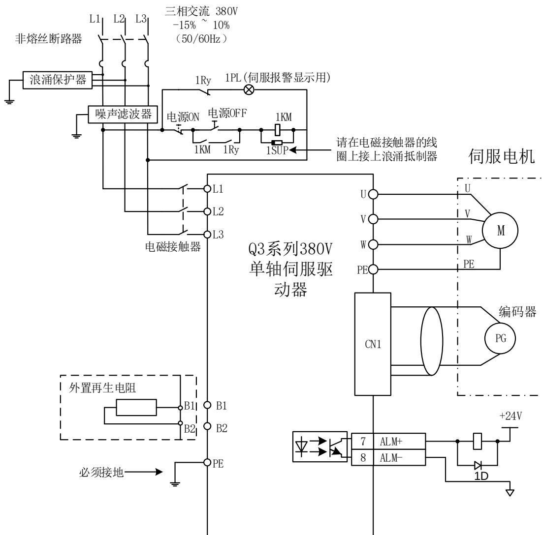
图 4.2.2-1 三相 380V 主电路配线
