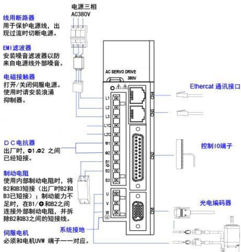
图 3.3.3-1 三相 380V 系统配置图
