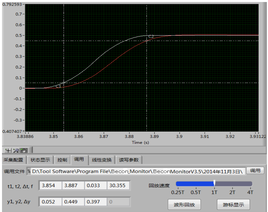
图 9.2.2-2 速度响应曲线 (白: 速度给定; 红: 速度反馈)
