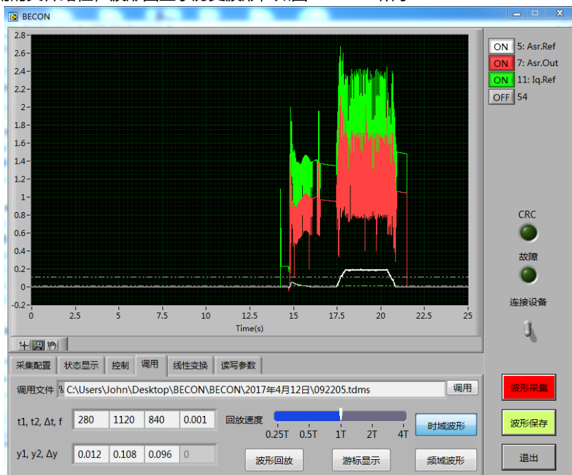
图 12.6.1-1 调用的历史波形
