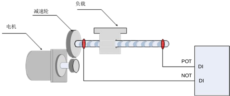
图 7.1.8-1 限位开关的安装示意图
