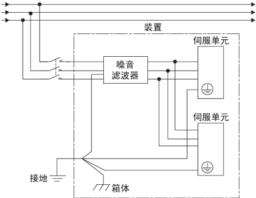
图4.7.2-4 噪音滤波器地线处理示意图
