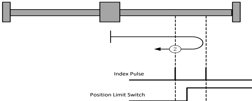
图 7.10.3-2 回零方法 2
