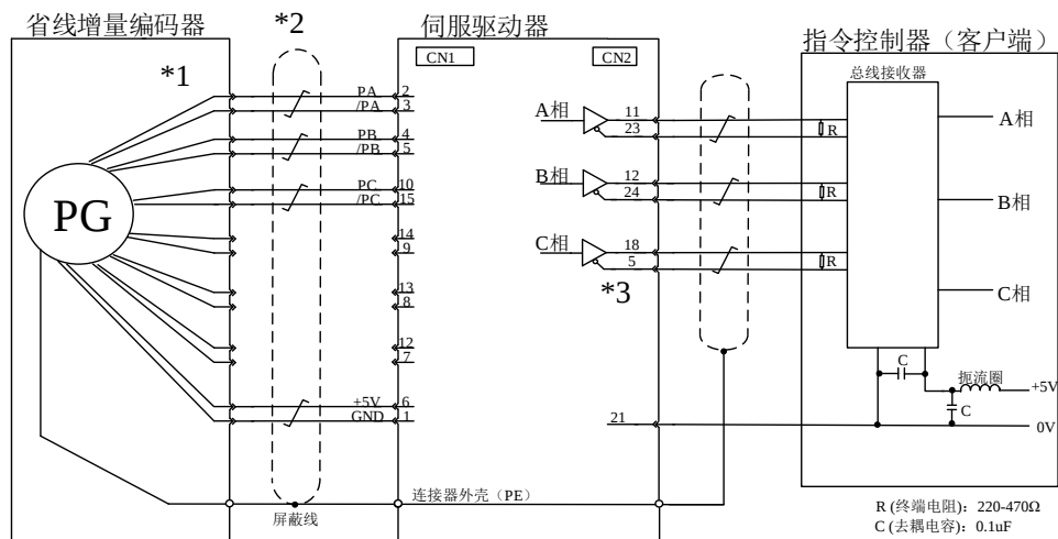
图 4.4.1-1 增量省线式编码器接线示意图
