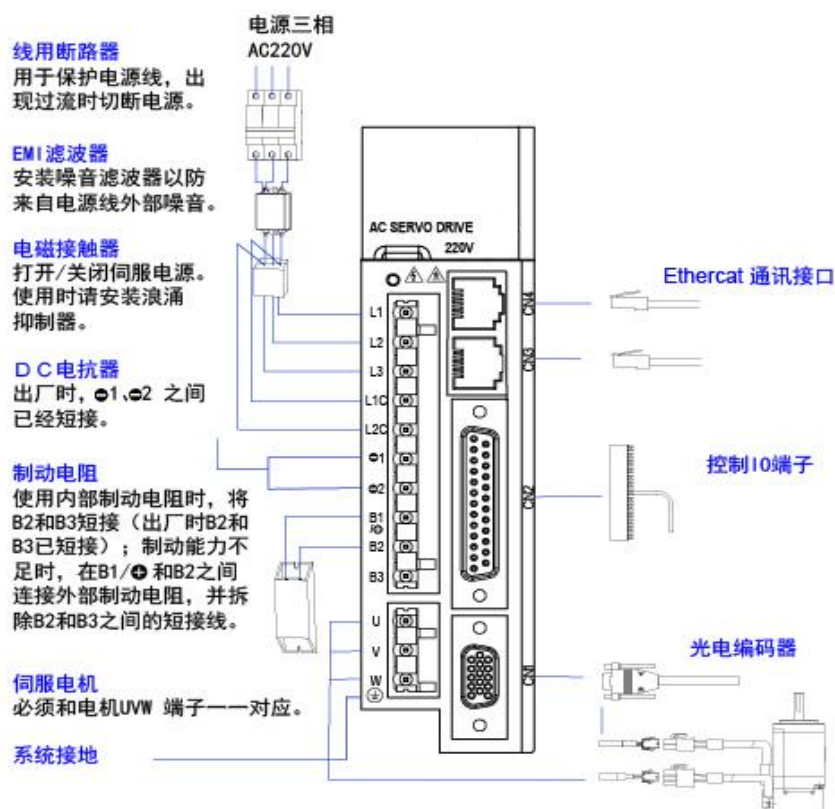
图 3.3.2-1 三相 220V 系统配线图
