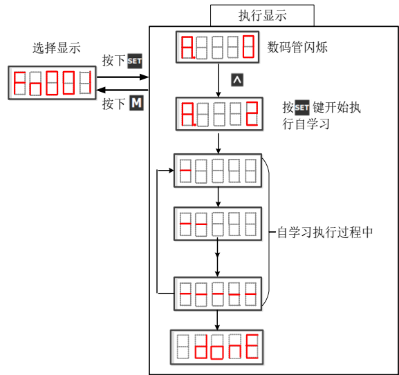
图 9.5.1-1 面板校零操作步骤
