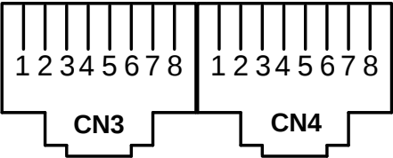
图 4.6-1 通信信号连接器引脚定义
