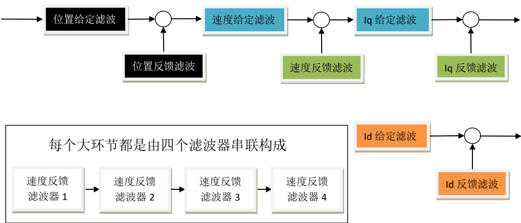
图 9.3.1-1 滤波器的结构
