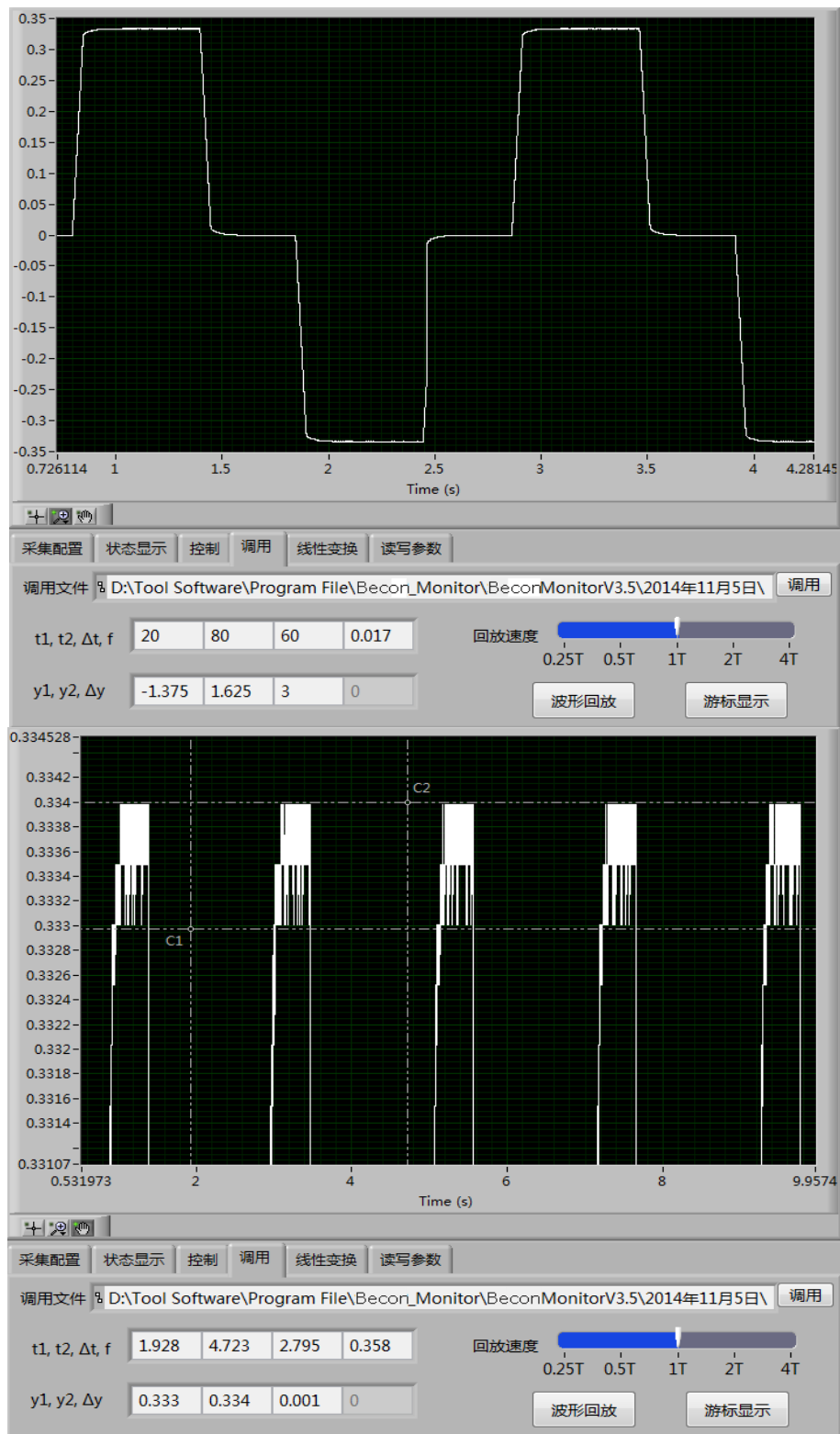
图 9.2.3-1 位置输出曲线 Asr.Ref
