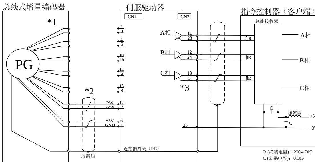
图 4.4.1-3 总线式增量型编码器接线示意图
