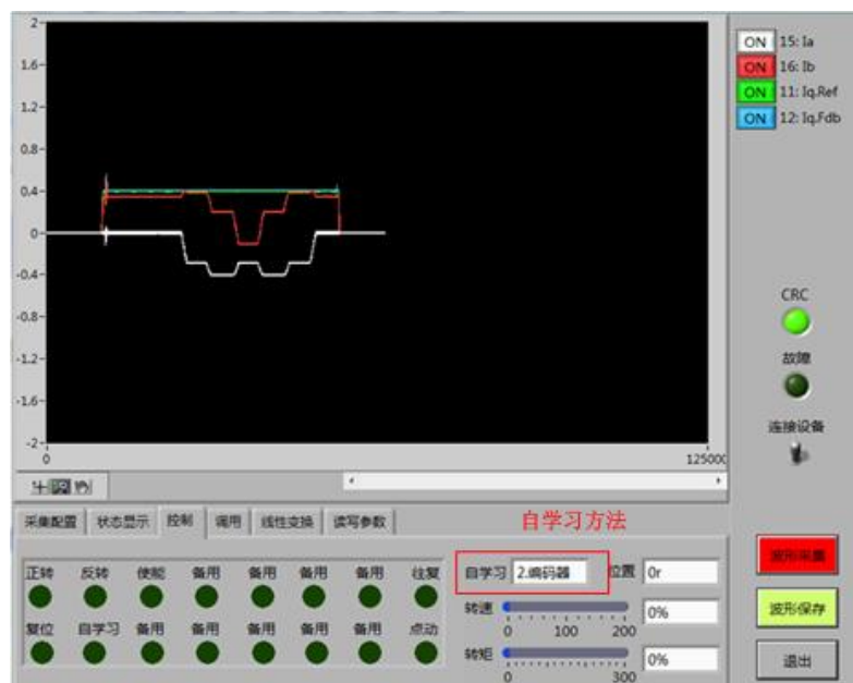
图 12.5.5-1 编码器偏移校零状态图
