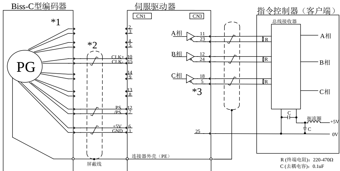
图 4.4.1-4 Biss-C 型编码器接线示意图
