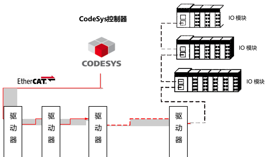
图 5.1-1 EtherCAT 组网示意图
