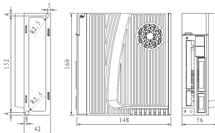
(3) 1.5kW 和 2.2kW (220V) 及 1.8kW 和 3kW (380V) 的安装及外观尺寸:
