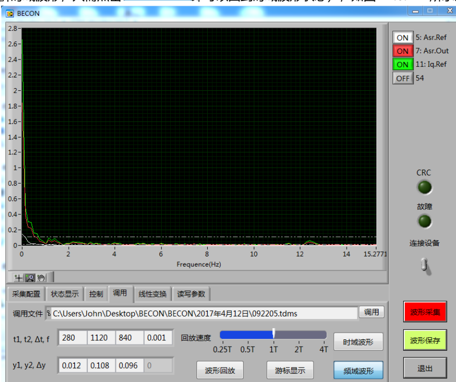
图 12.6.2-4 频域历史波形
