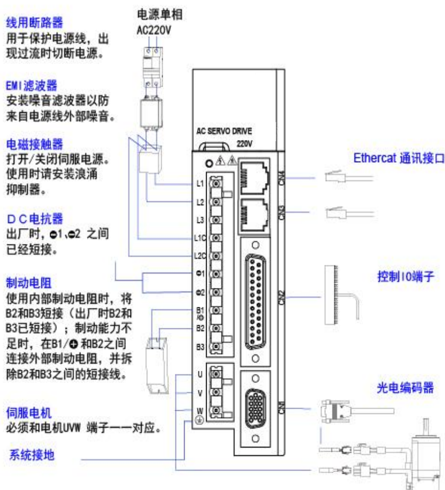
图 3.3.1-1 单相 220V 系统配线图
