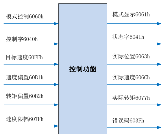
图 7.5.1-2 输入输出对象
