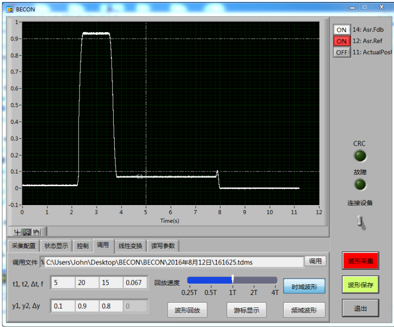
图 12.2.3-1 历史波形页面
