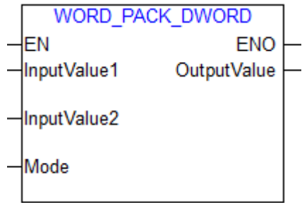
图 103 WORD_PACK_DWORD 功能块
