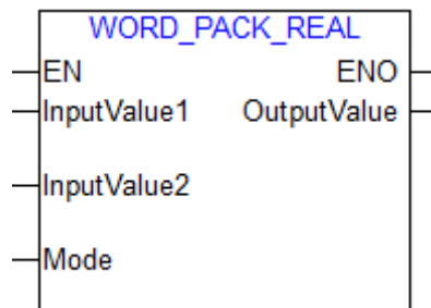
图 105 WORD_PACK_REAL 功能块
