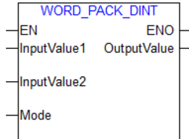
图 104 WORD_PACK_DINT 功能块
