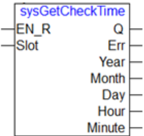
图 135 sysGetCheckTime 指令
