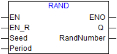
图 120 RAND 功能块
