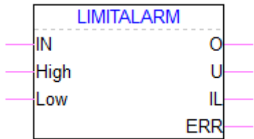
图 127 LIMITALARM 功能块
