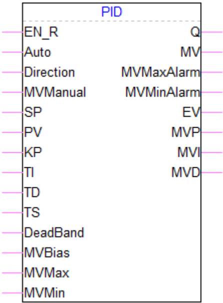
图 113 PID 功能块
