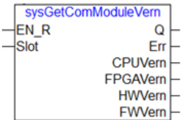
图 134 sysGetComModuleVern 指令
