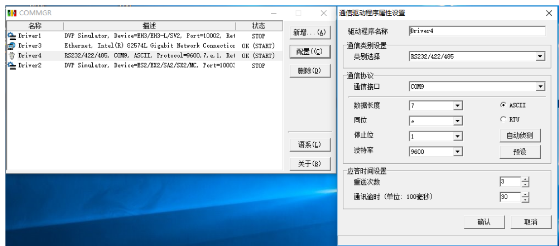
新增通信驱动
