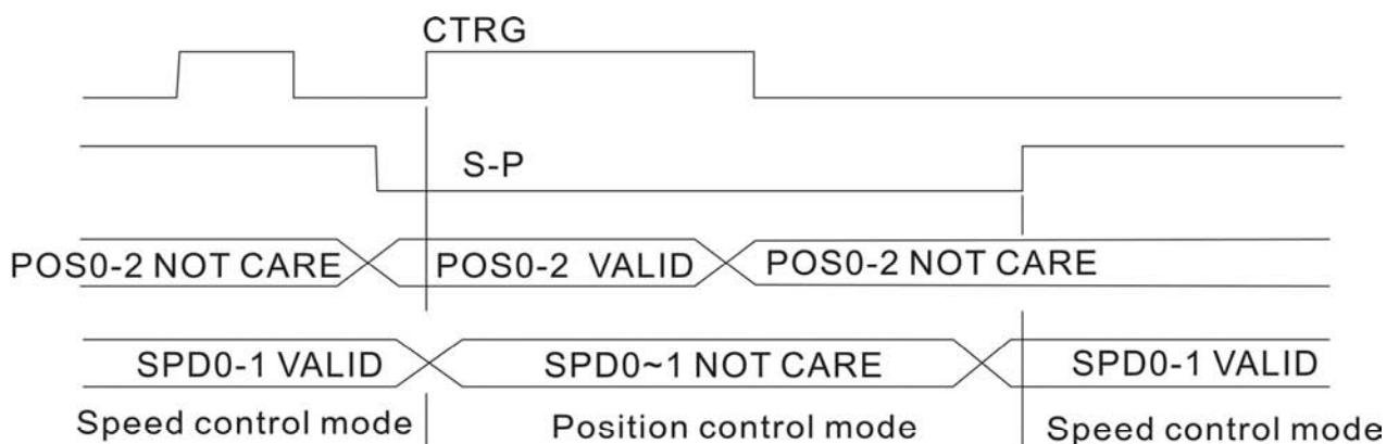
图一：速度/位置混合控制模式
