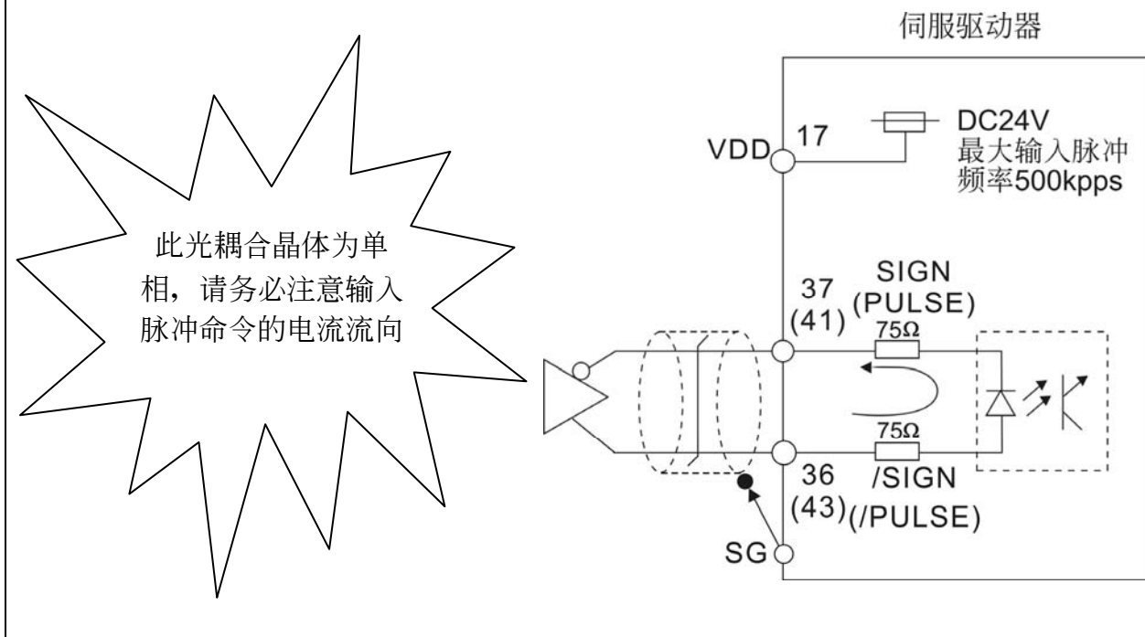
C4-2: 高速脉冲命令输入（差动输入）
