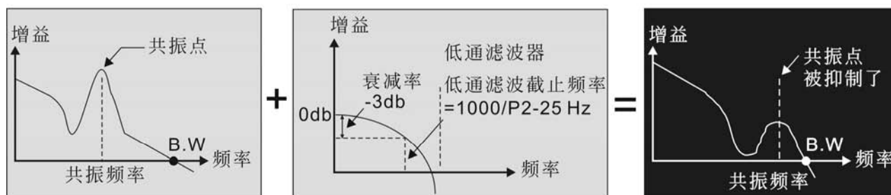
使用低通滤波器抑振
