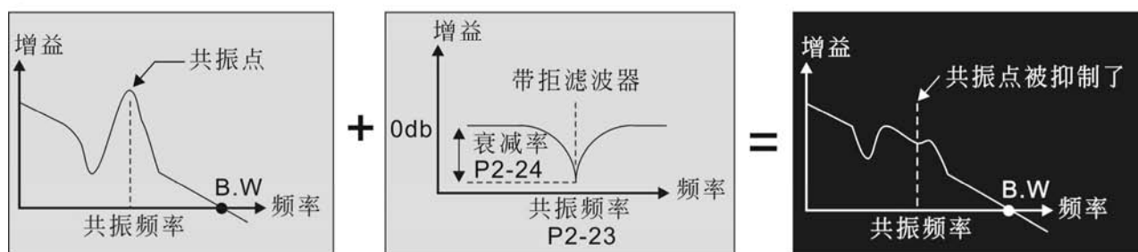
使用带阻滤波器抑振
