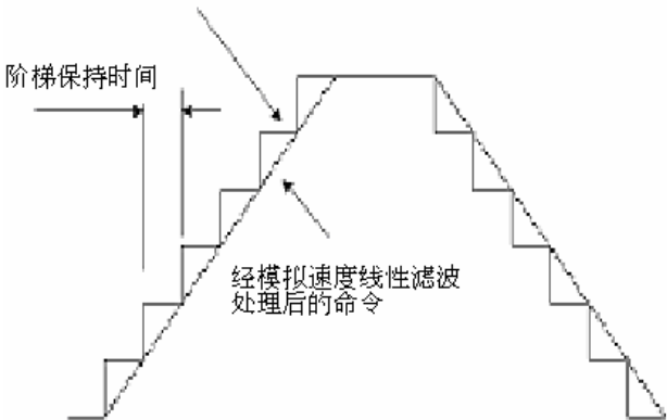
原始阶梯状模拟速度命令
