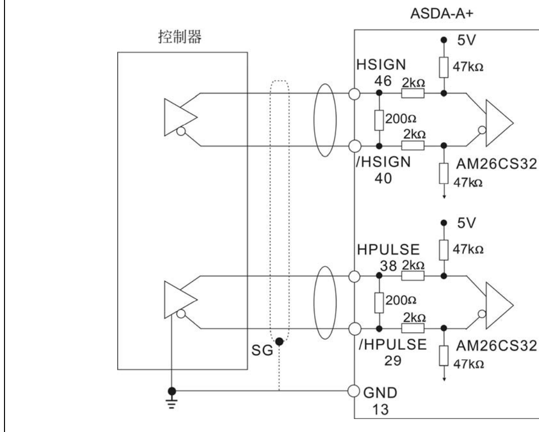
C4-2: 高速脉冲命令输入（差动输入）
