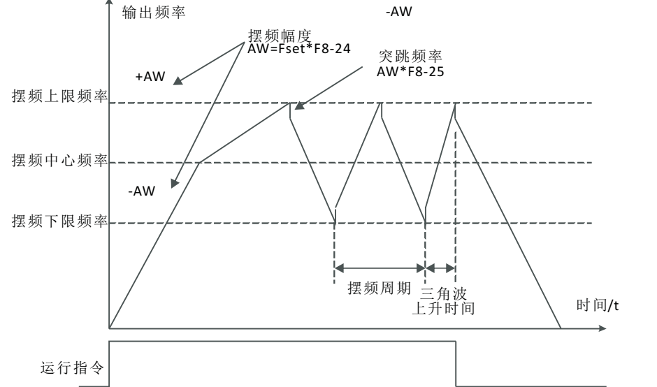
图5-24 摆频工作示意图
