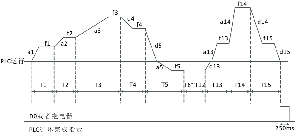
图5-31 简易PLC运行图
