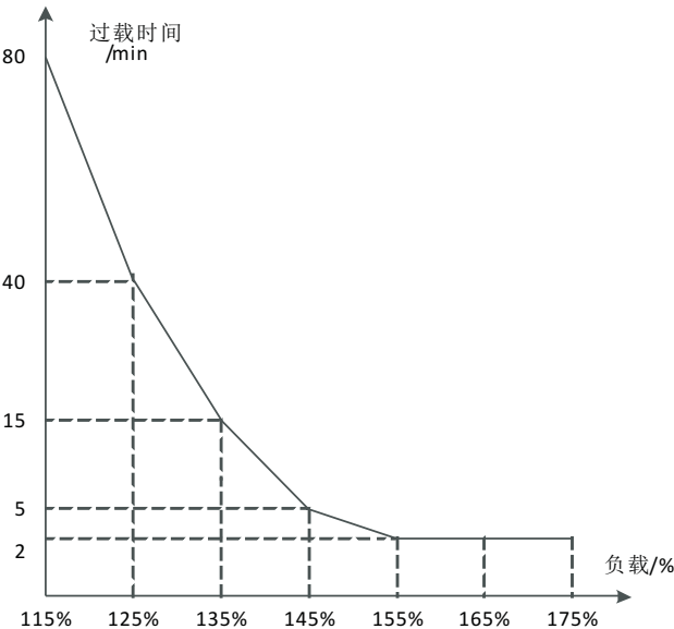
图5-25 过载电流与过载时间曲线
