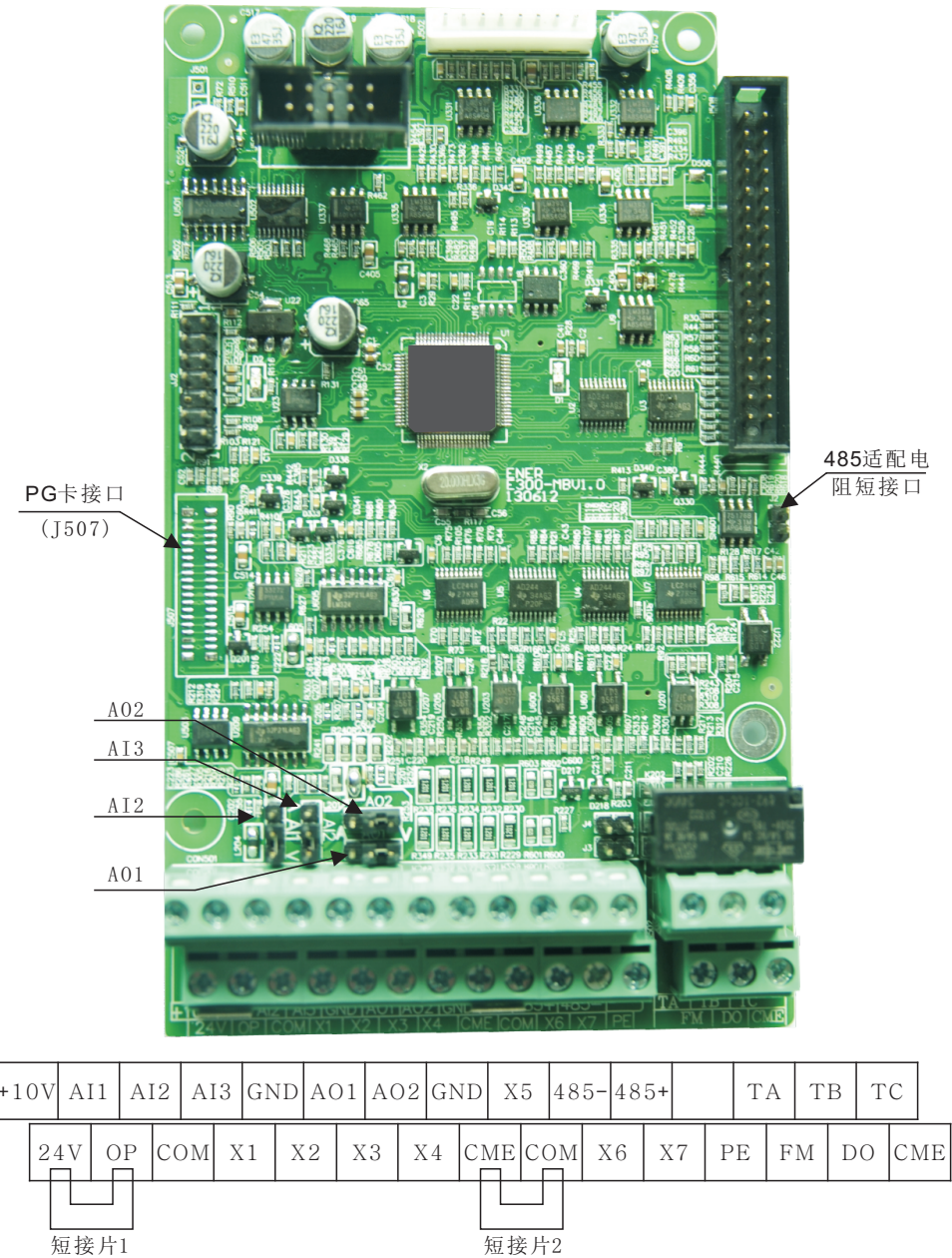
控制回路端子示意图
