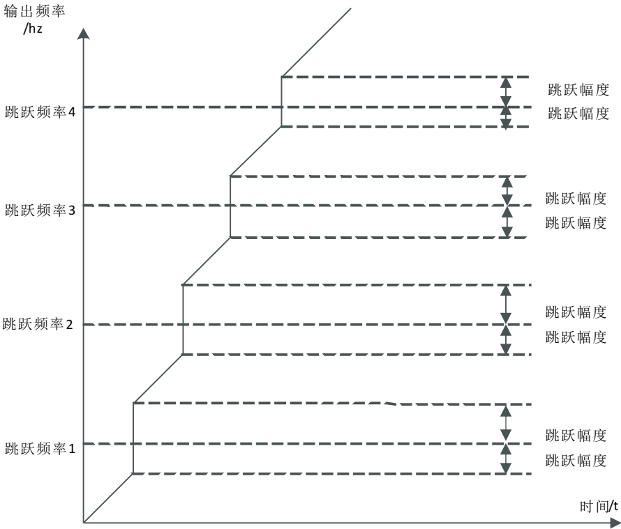
图5-23 加减速过程中跳跃频率有效示意图
