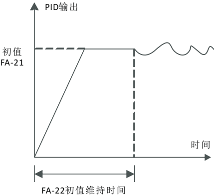
图5-30 PID初值功能示意图
