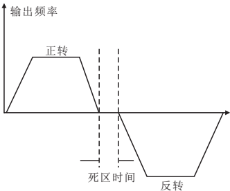
图5-02 正反转死区时间示意图
