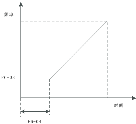
图5-18 启动频率与启动时间
