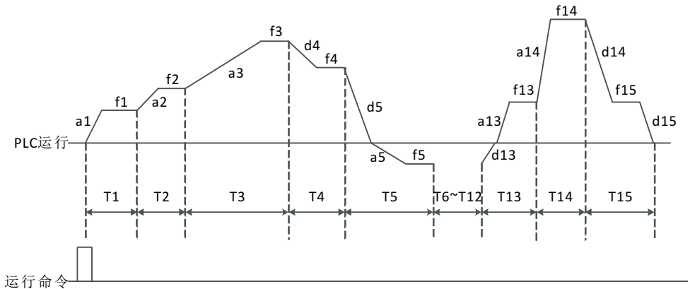
图5-32单循环后停机方式
