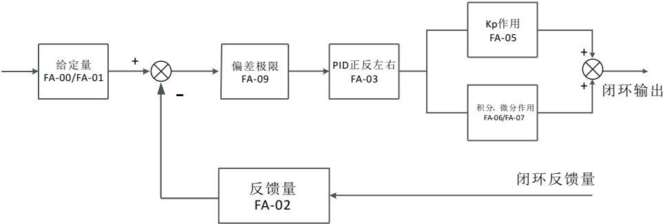
图5-27 过程PID原理框图
