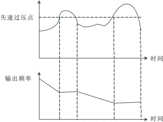
图5-26 过压失速功能
