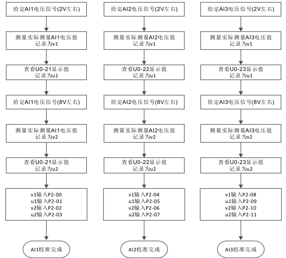
图5-34 AI校准方法示意图
