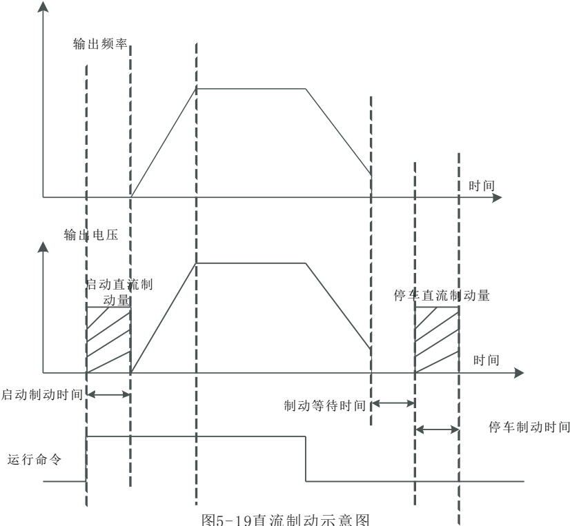
图5-19直流制动示意图
