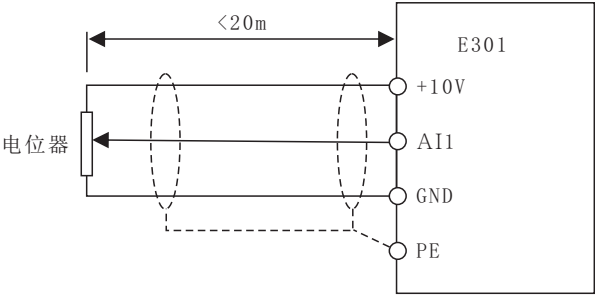
模拟量输入端子接线示意图
