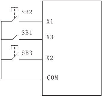
图5-14 三线式控制模式1
