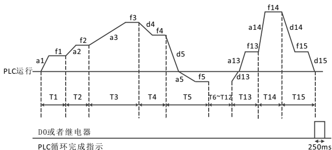
图5-31 简易PLC运行图
