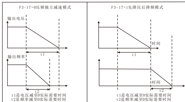
图5-07 V/F分离停机过程示意图
