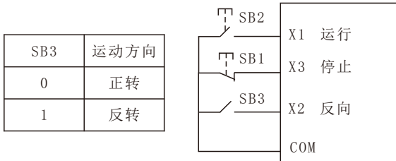
图5-15 三线式控制模式2
