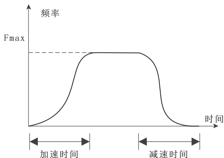
图5-21 S曲线加减速
