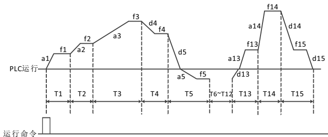
图5-32单循环后停机方式
