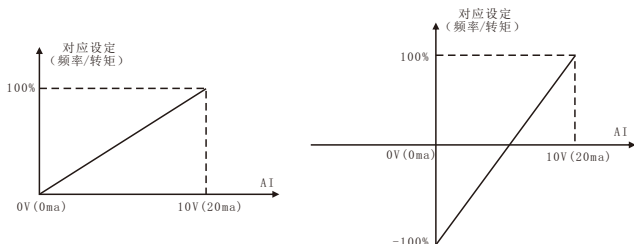
图5-16 模拟给定与设定量的对应关系
