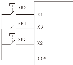
图5-14 三线式控制模式1
