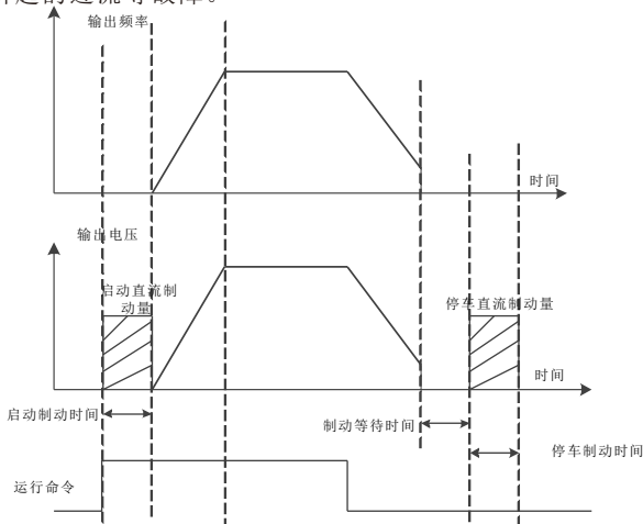
图5-19直流制动示意图
