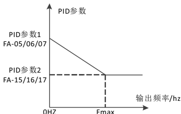
图5-29 PID根据运行频率切换示意图
