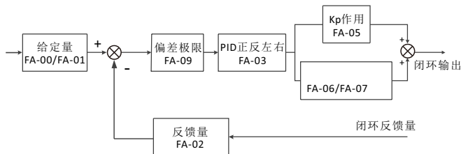
图5-27 过程PID原理框图
