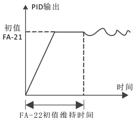
图5-30 PID初值功能示意图
