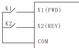
图5-12 两线式模式1
