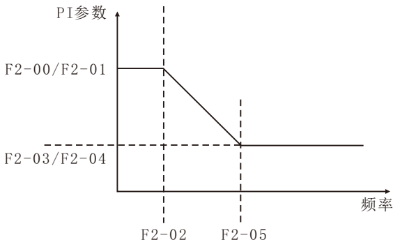
图5-03 PI参数示意图
