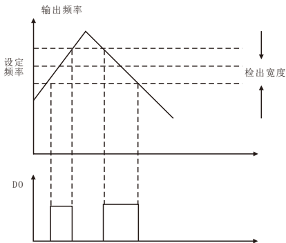
图5-10 频率到达检出幅值示意图
