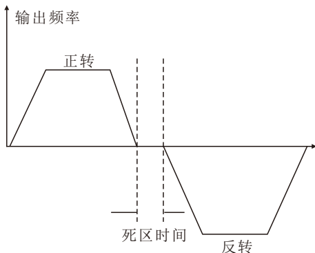
图5-02 正反转死区时间示意图
