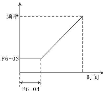
图5-18 启动频率与启动时间
