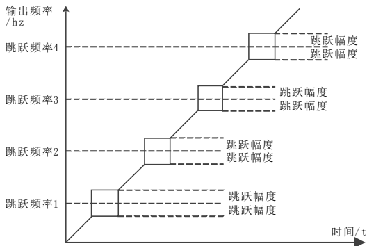
图5-22 跳跃频率示意图
