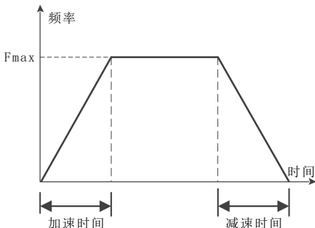
图5-20直线加减速
