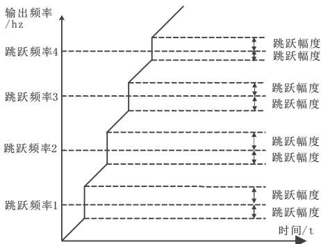
图5-23 加减速过程中跳跃频率有效示意图
