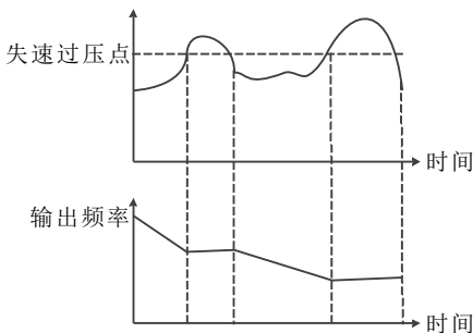
图5-26 过压失速功能
