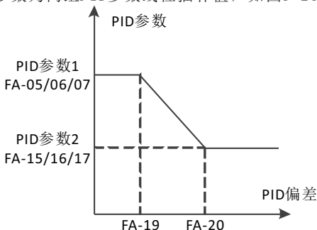
图5-28 PID根据偏差切换示意图
