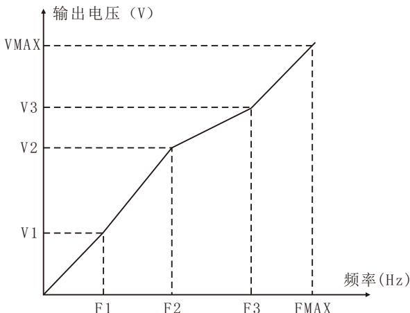
图5-05 多点V/F曲线设定示意图
