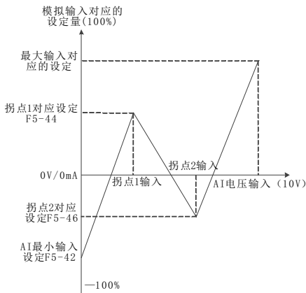
图5-17 4点曲线示意图
