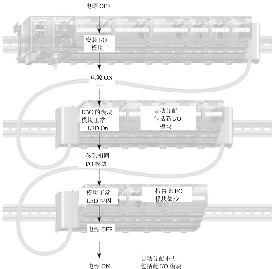
热插拔 I/O 模块时的 LED 指示灯
