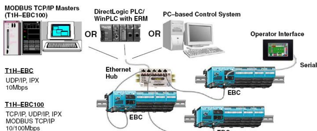
EBC 系统例：各种主局与 EBC 子局之间的连接
