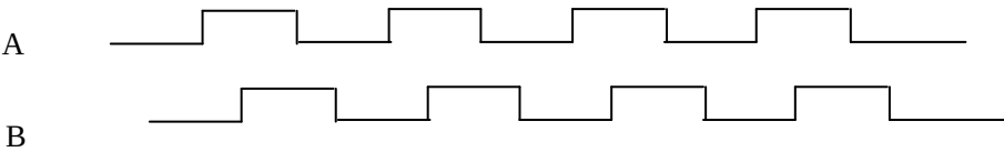
A 相比 B 相超前 90°，A 相的下降沿触发减计数
