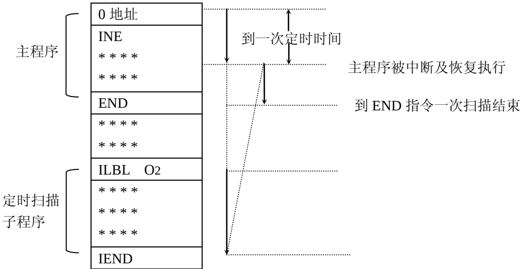
定时扫描过程图
