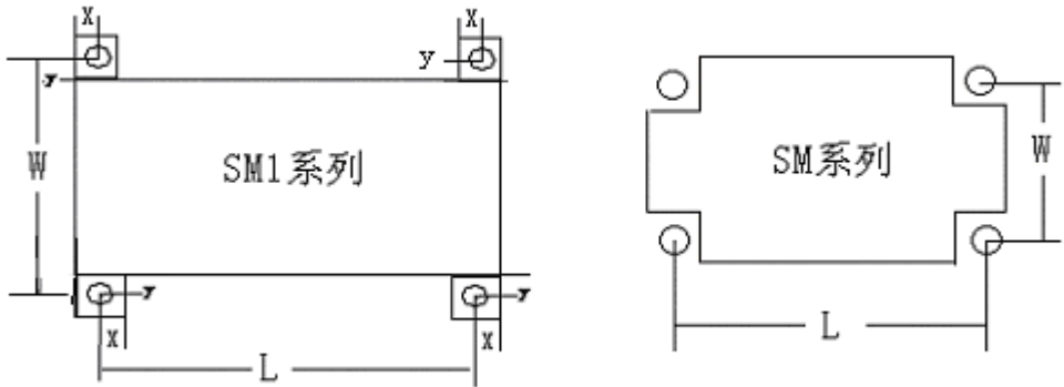
图 3-1 SM 系列 PLC 螺钉安装尺寸示意图
