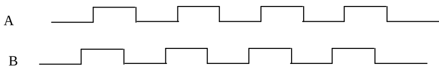
B 相比 A 相超前 90°，A 相的下降沿触发加计数
