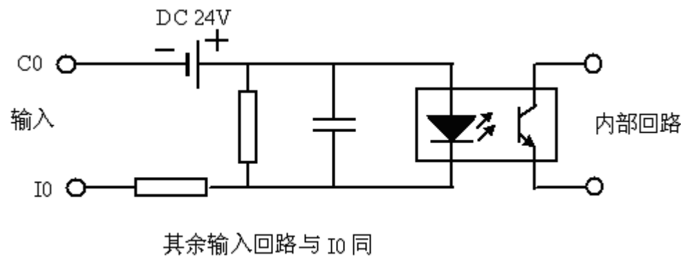
(3)DC24V 输入回路电气性能（PNP 型）（仅 SM）
