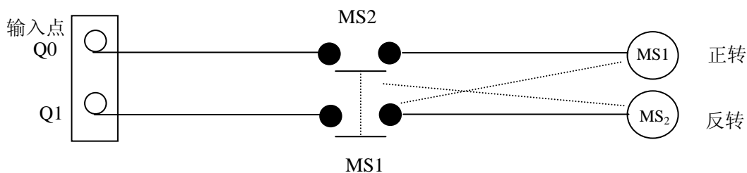
SH/SH1/SH2 系列 PLC 外部互锁回路图例
