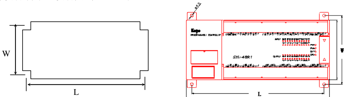
SH 系列 PLC 螺钉安装尺寸示意图
