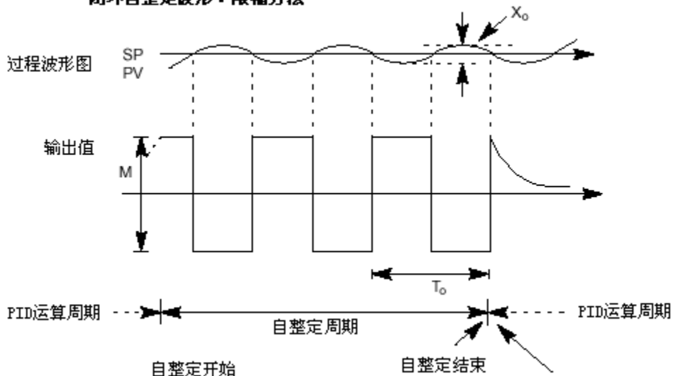
闭环自整定波形：限幅方法
