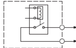
形式A触点继电器
