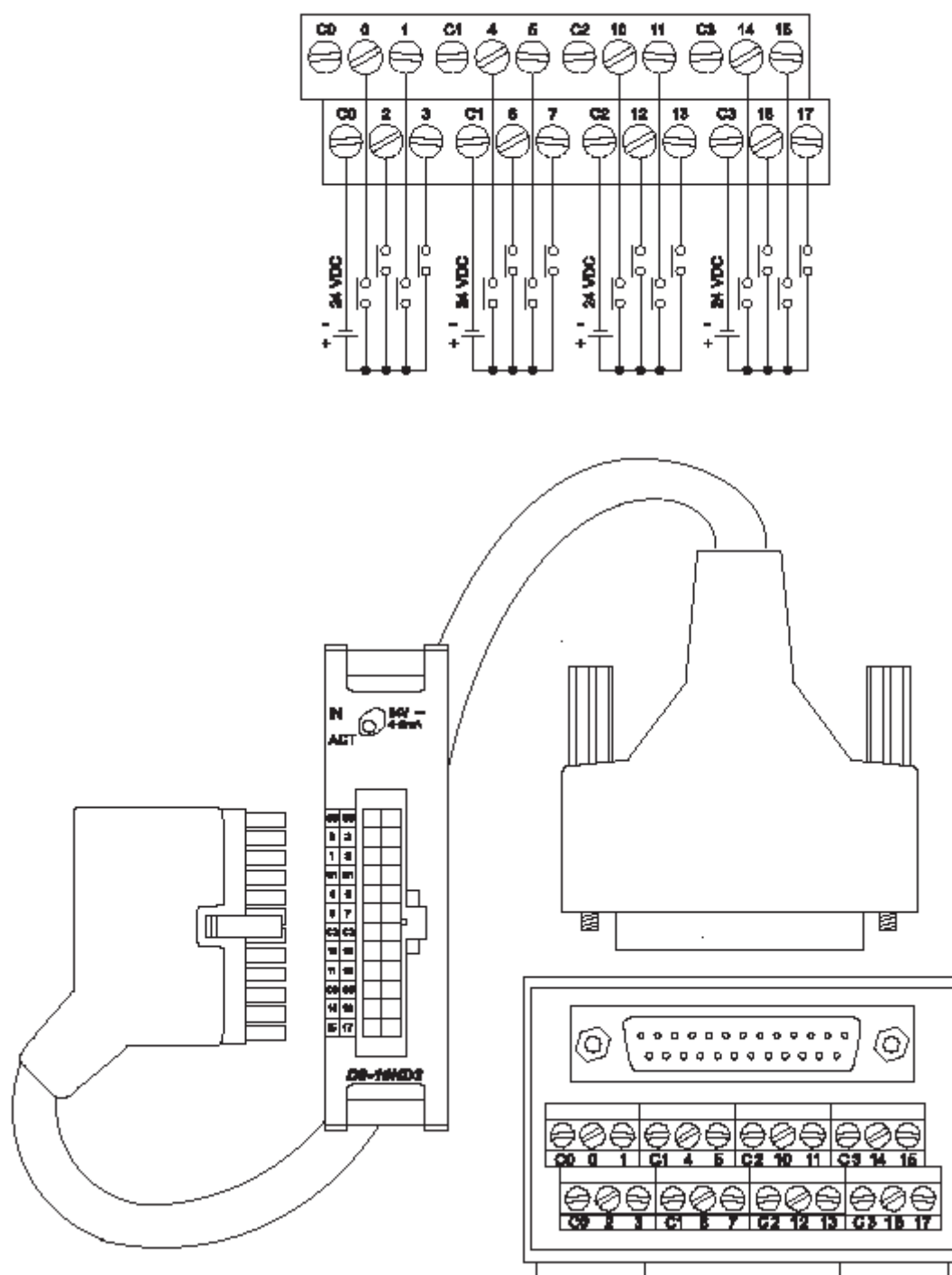
接线图
