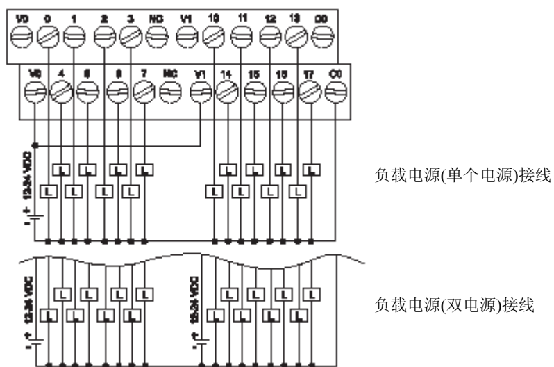
接线图
