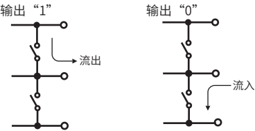
等价电路
