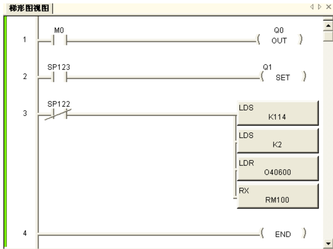
主局 PLC 程序
