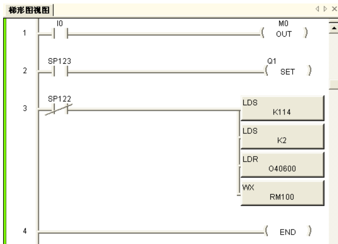
子局 PLC 程序
