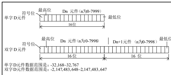
图3-5 D 元件
