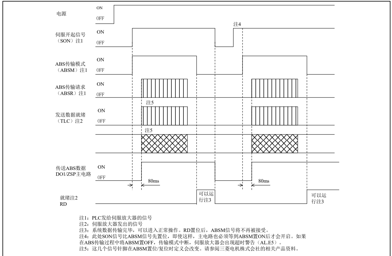
时序图
