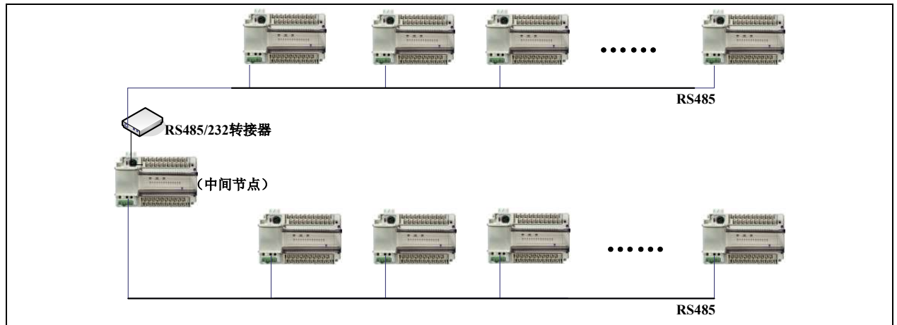
图10-8 YLbus 多层网络
