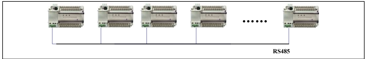
图10-7 YLbus 单层网络
