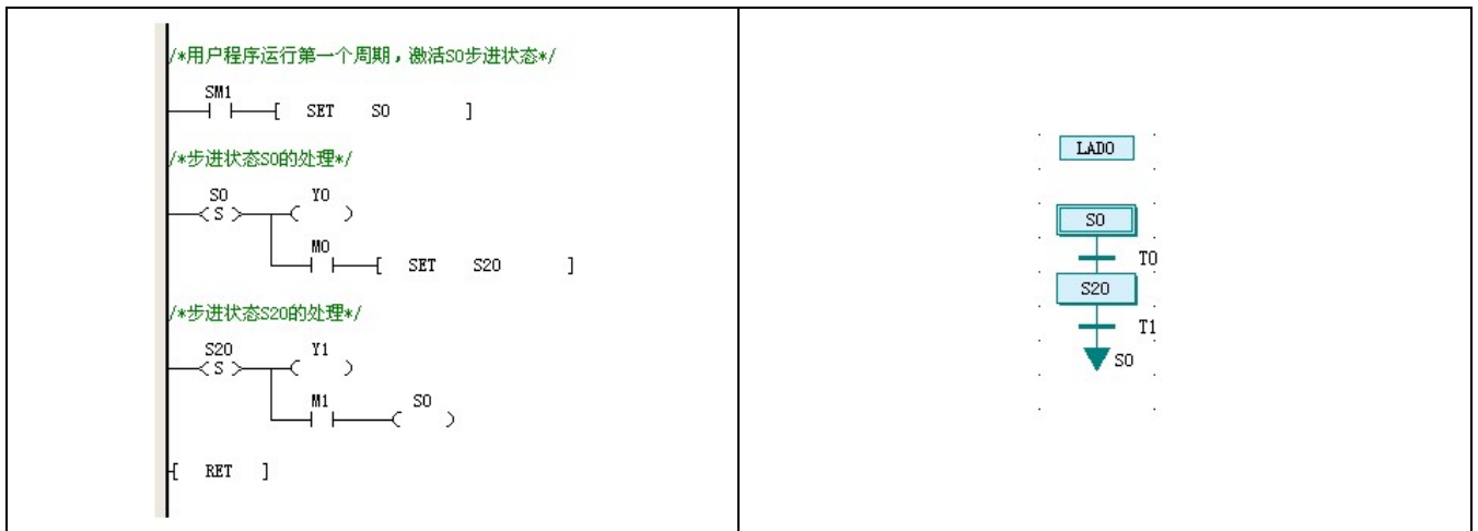
图4-3 顺序功能图示例
