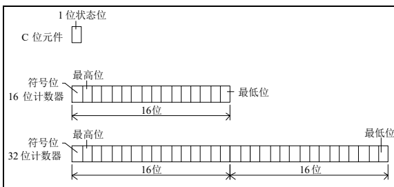
图3-4C 元件
