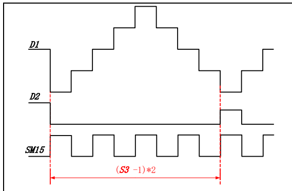
三角波指令执行过程分解如下图 (S3=5):
