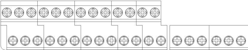
图 3-21 控制板端子示意图
