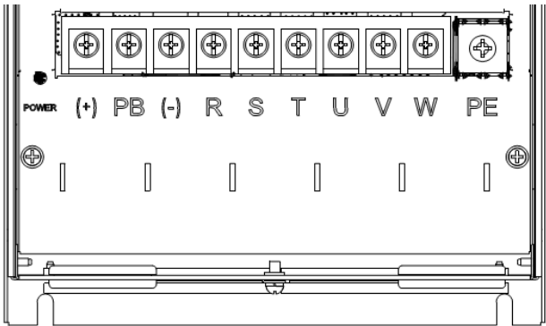
图 3-9 CT100-4T-15G/18.5P~CT100-4T-22G/37P 主回路接线端子图
