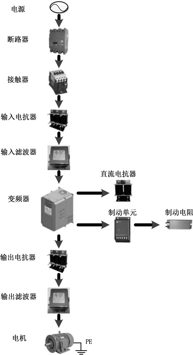
图 3-7 产品外围元器件的标准配置图
