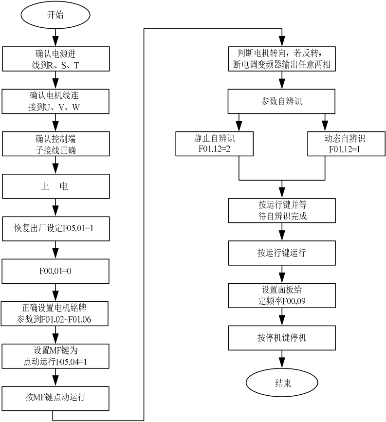
图 4-2 首次上电流程图
