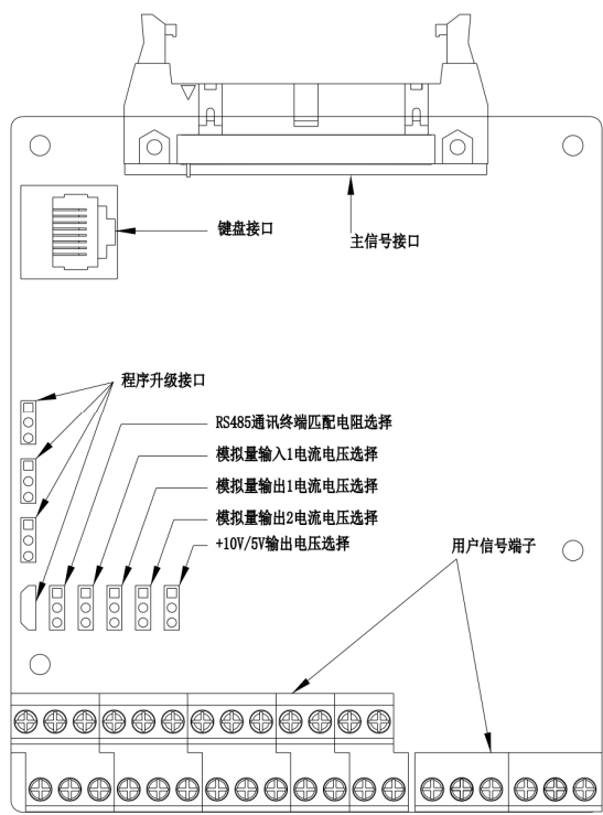
图 3-20 控制板示意图
