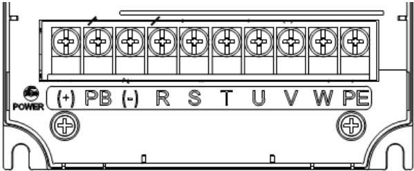
图 3-8 CT100-2S-2.2G、CT100-4T-11G/15P 及以下功率主回路接线端子图
