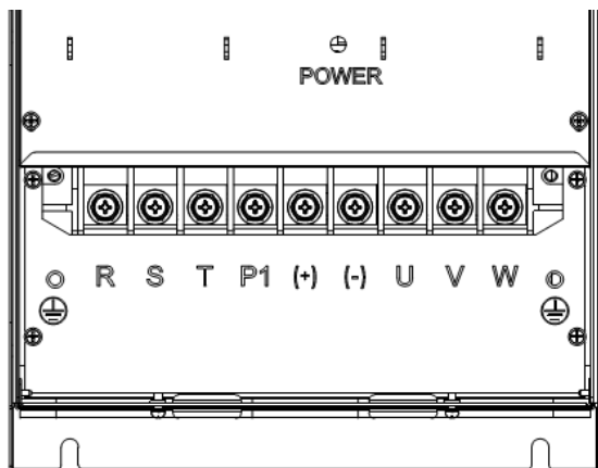
图 3-11 CT100-4T-45G/55P~CT100-4T-55G/75P 主回路接线端子图
