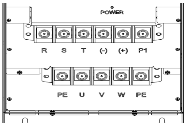
图 3-12 CT100-4T-75G/90P~CT100-4T-110G/132P 主回路接线端子图
