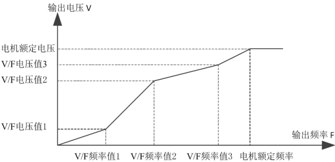
图 6-5 多点 V/F 曲线图
