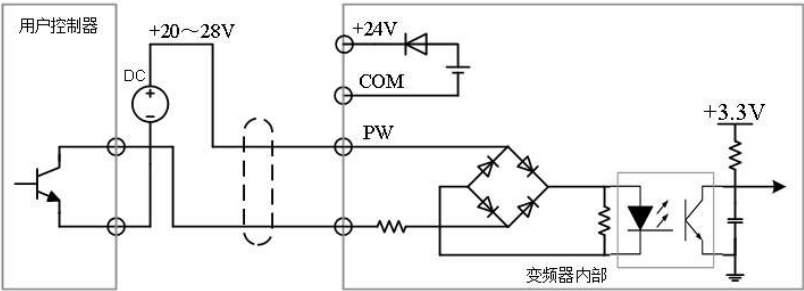
图 3-25 NPN 型灌电流接线方式
