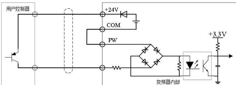
图 3-24 PNP 型拉电流接线方式
