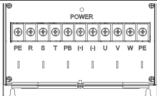
图 3-10 CT100-4T-30G/37P~CT100-4T-37G/45P 主回路接线端子图
