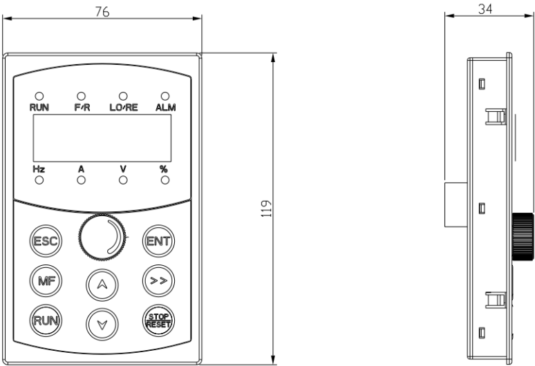
图 2-5 面板外形及尺寸图
