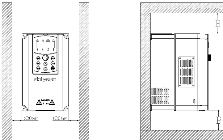
图 3-1 CT100-4T-11G/15P 及以下功率等级的安装方向和距离要求
