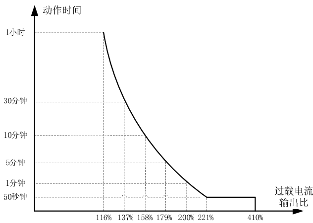
图 6-13 过载保护动作时间与电流比的关系
