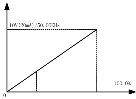
图 6-12 模拟量与高速脉冲输出对应关系
