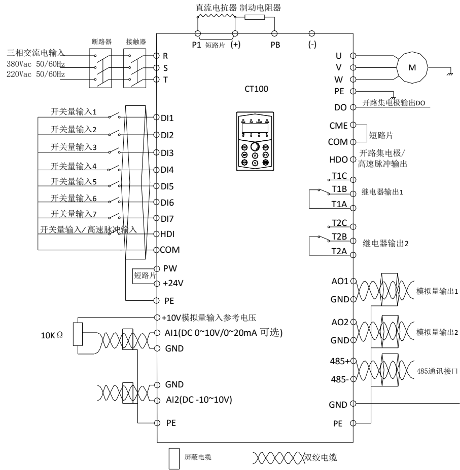
图 3-15 标准接线图
