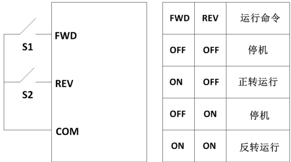
图 6-8 两线式控制 2
