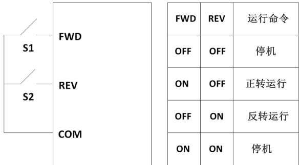
图 6-7 两线式控制 1
