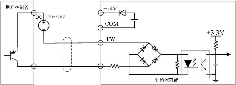
图 3-26 PNP 型拉电流接线方式
