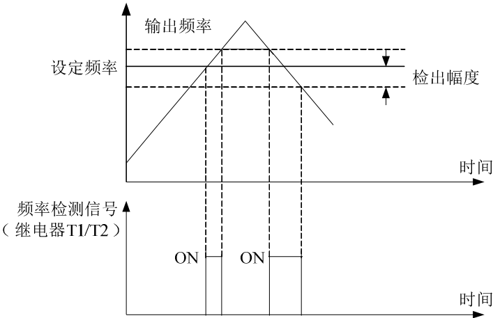
图 6-20 FDT 电平示意图
