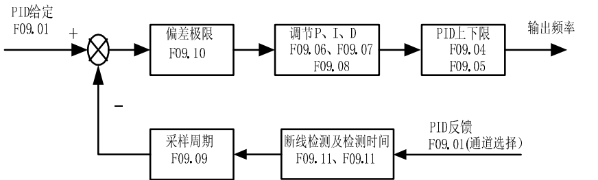
图 6-14 过程 PID 控制流程
