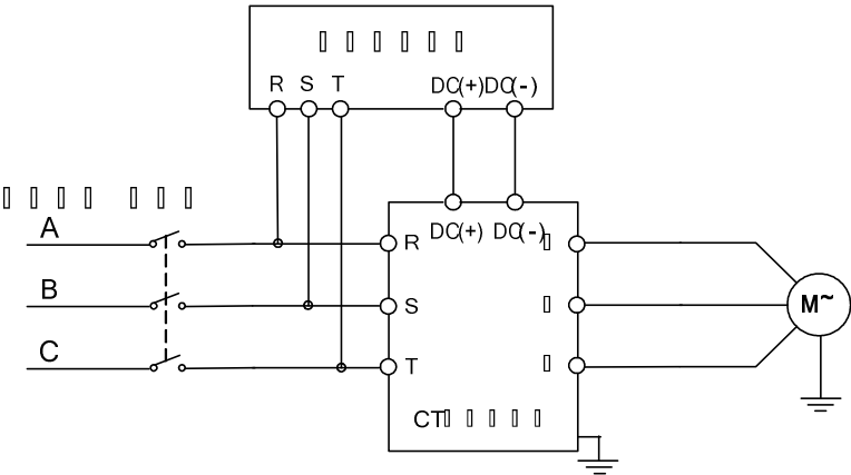
图 3-18 能量回馈单元连接图
