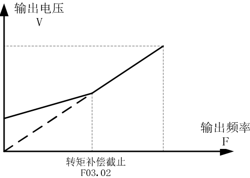
图 6-4 转矩补偿图
