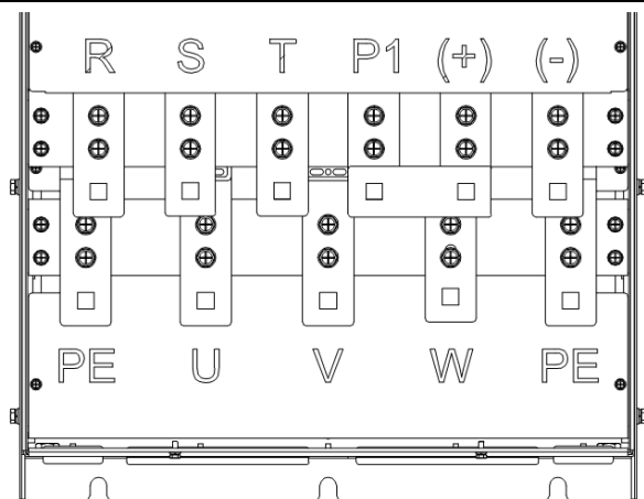
图 3-13 CT100-4T-132G/160P~CT100-4T-200G/220P 主回路接线端子图
