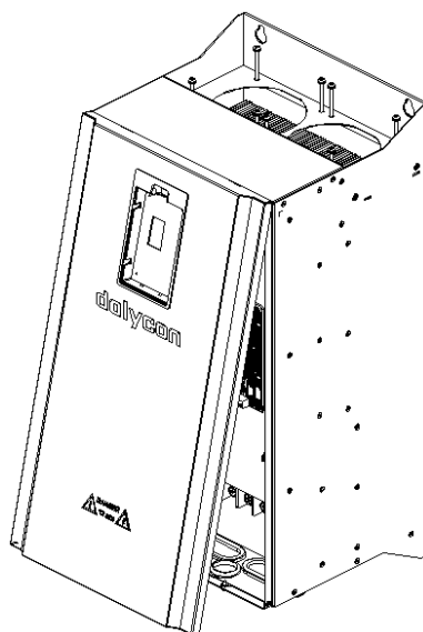
图 3-6 CT100-4T-15G/18.5P 及以上功率 盖板安装与拆卸图
