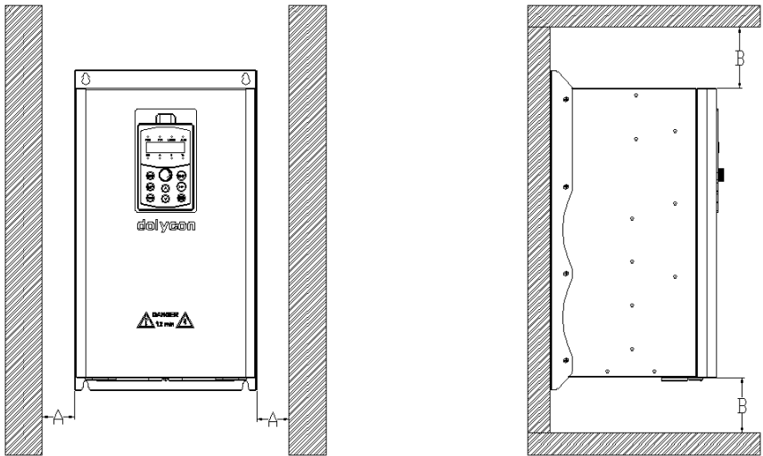
图 3-2 CT100-4T-15G/18.5P 及以上功率等级的安装方向和距离要求
