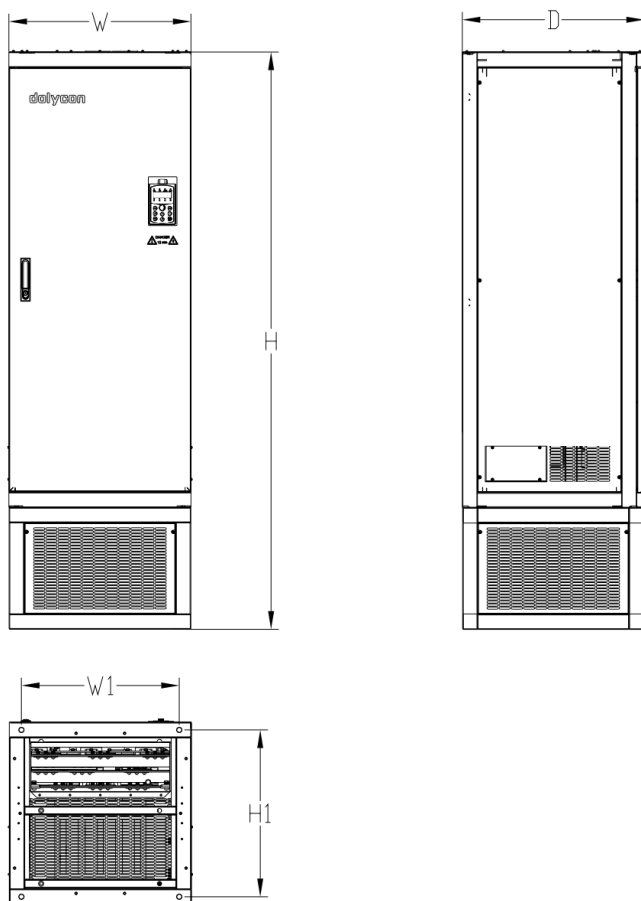
图 2-4 产品外形及安装尺寸图
