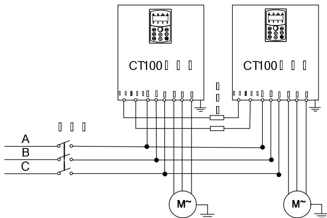
图 3-19 共直流母线的连接
