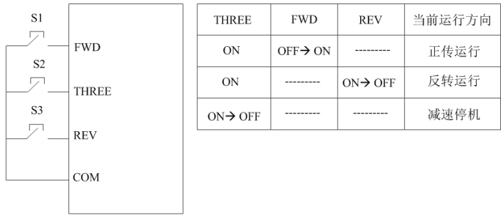
图 6-10 三线式控制 2
