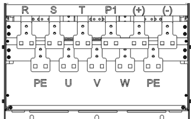
图 3-14 CT100-4T-220G/250P~CT100-4T-315G/350P 主回路接线端子图
