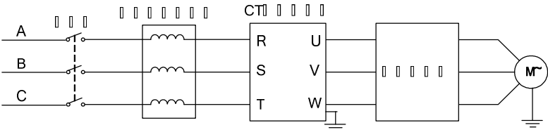
图 3-17 主回路电机侧连接图
