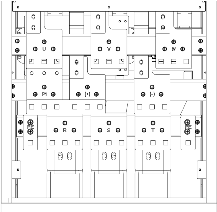
图 3-15 CT100-4T-350G~CT100-4T-500G 主回路接线端子图
