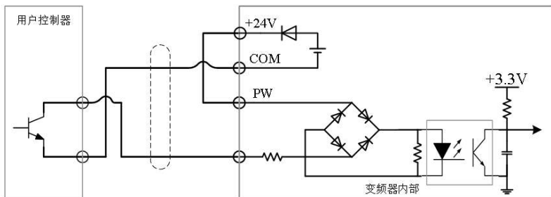
图 3-23 NPN 型灌电流接线方式
