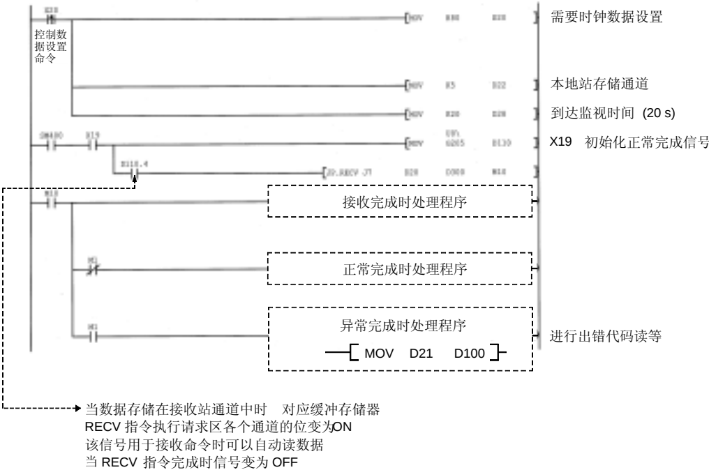
(b) 15 号站程序 (RECV 指令) 当以太网模块的 I/O 信号是 X/Y00 至 X/Y1F 时
