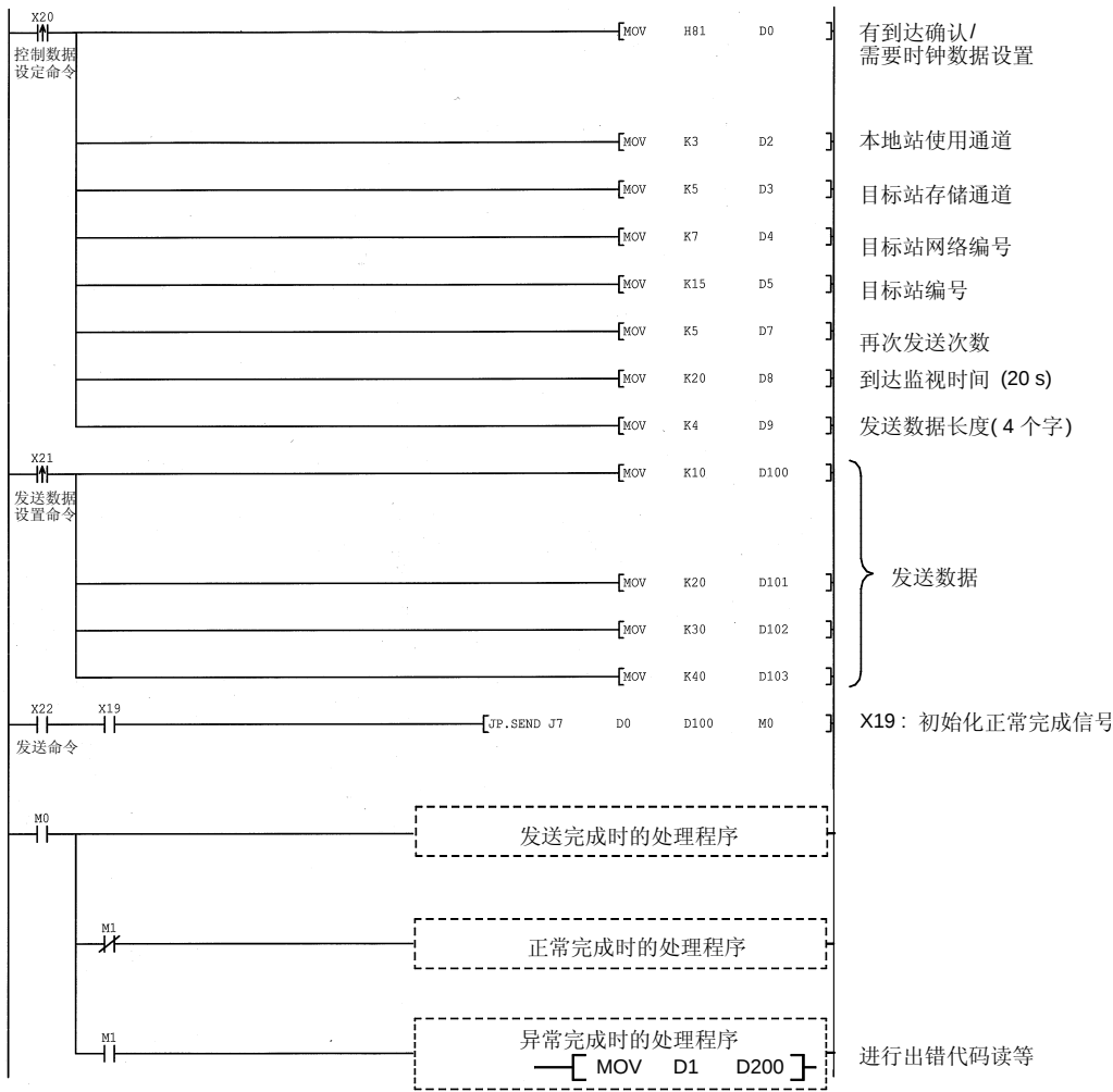
(a) 3 号站程序 (SEND 指令) 当以太网模块的 I/O 信号是 X/Y00 至 X/Y1F 时
