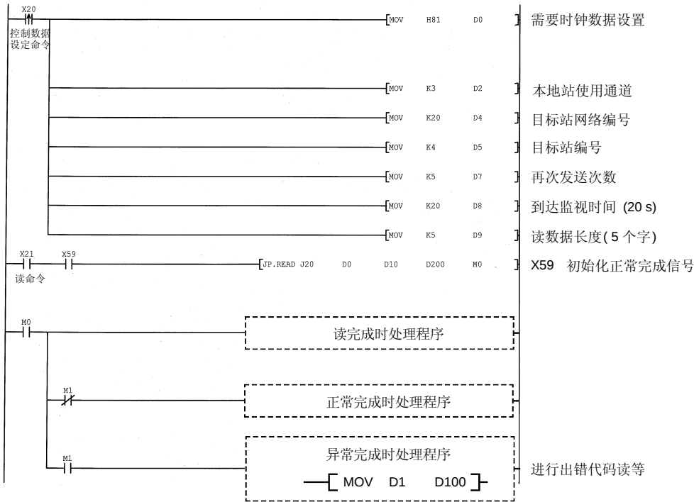
(a) 1 号站程序 (READ 指令) 当以太网模块的 I/O 信号是 X/Y40 至 X/Y5F 时
