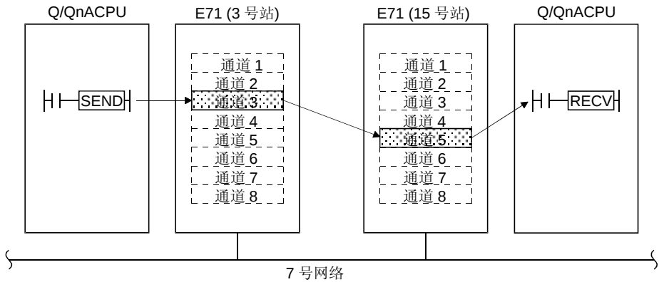
(a) 3 号站程序 (SEND 指令) 当以太网模块的 I/O 信号是 X/Y00 至 X/Y1F 时
