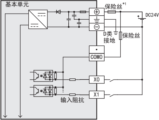
· 漏型输入接线 (FX3GC-32MT/DSS)
