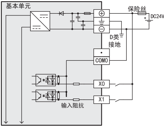
· 源型输入接线 (FX3UC-□□MT/DSS)
