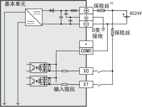
· 源型输入接线 (FX3GC-32MT/DSS)
