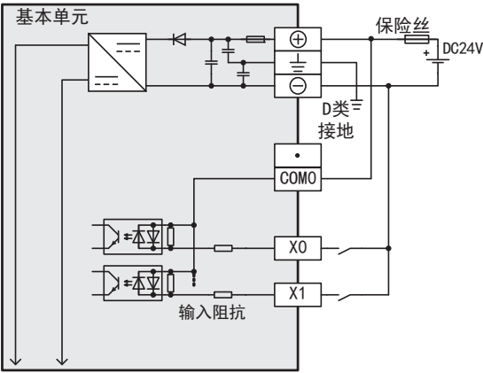
· 漏型输入接线 (FX3UC-□□MT/DSS)
