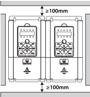
图 3-1 变频器并排安装
