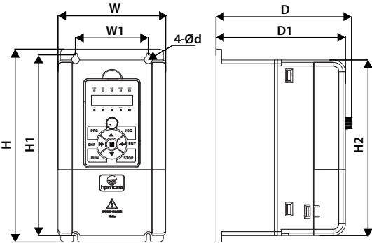
图 3-3 HD20 外型图
