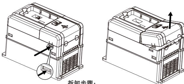
图 3-6 端子盖板拆卸示意图
