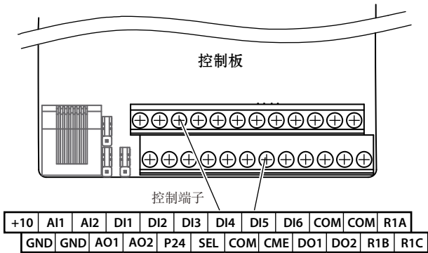
图 4-2 控制端子
