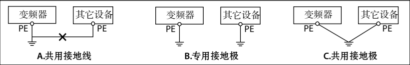
图 4-15 推荐的接地方式
