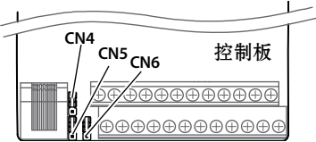
图 4-3 跳线位置
