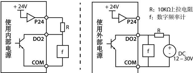
图 4-11 DO2 端子接线
