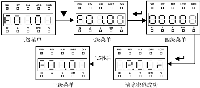
图 5-10 用户密码清除
