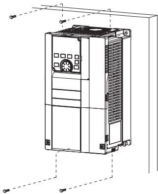
FR-F840-04320 (185K) 及以上 请请固定 6 处。
