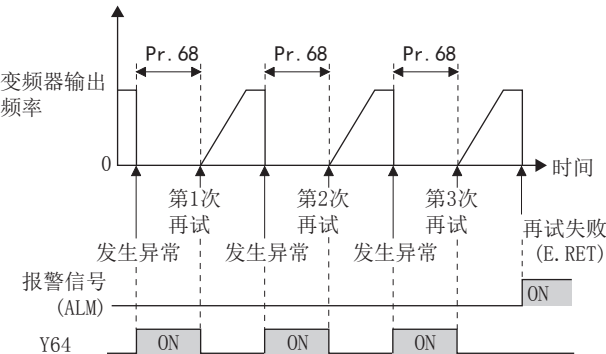
再试失败示例
