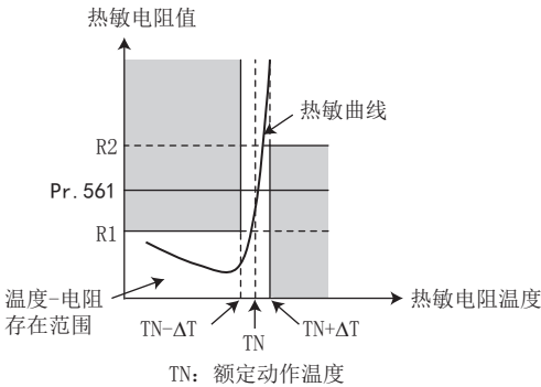
PTC 热敏电阻特性例
