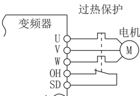
外部过热输入接线例
