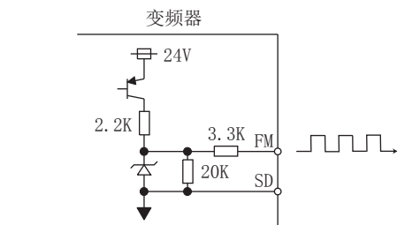
FM 输出回路
