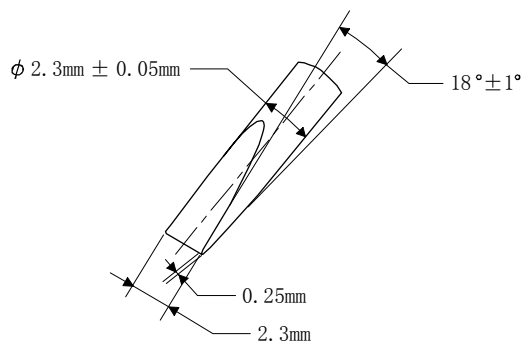
螺丝刀的形状 φ 2.3mm
