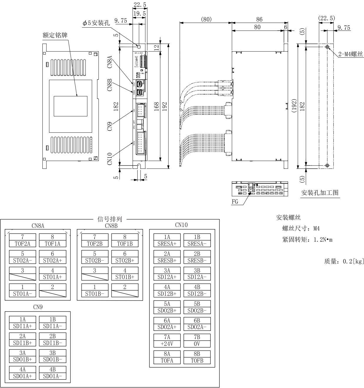
附5.12 外形尺寸图
