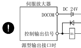
源型输出接口时
