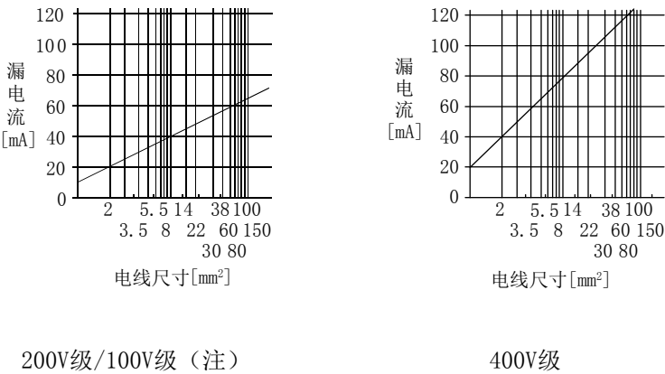
图11.13 CV电缆进行金属接线时每1km的漏电流示例（I g1 ，I g2 ）
