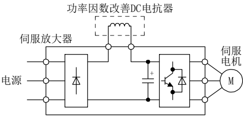
功率因数改善DC电抗器时
