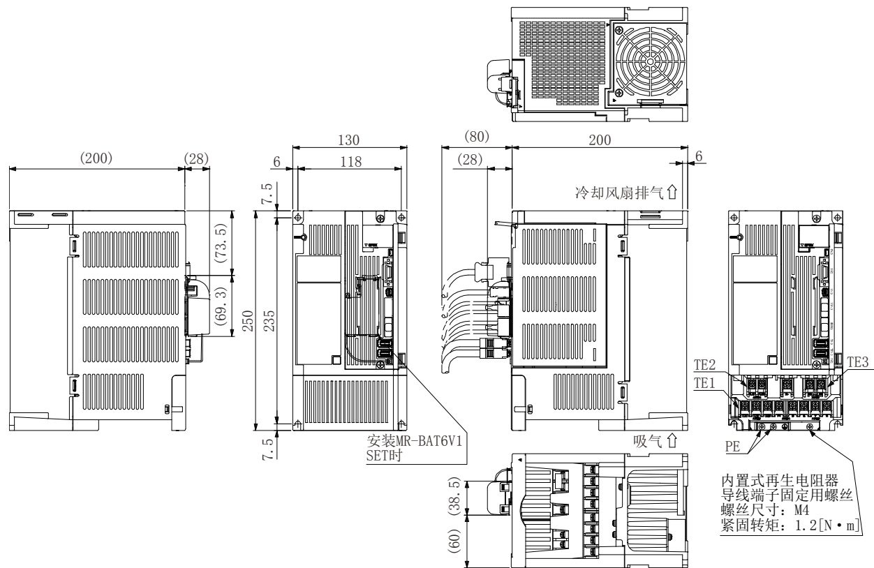
(d) MR-J4-500B4(-RJ)
