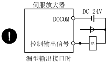
漏型输出接口时
