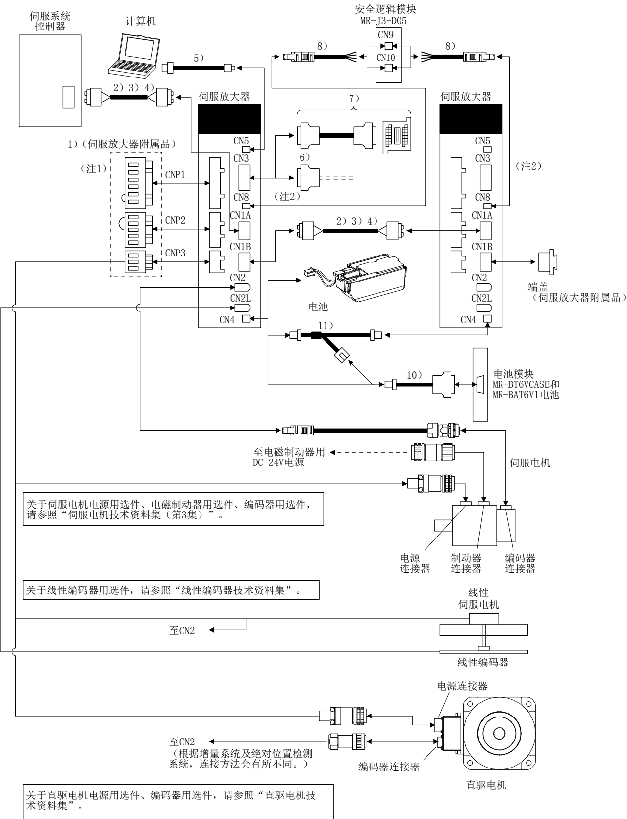
MR-J4-B-RJ伺服放大器时
