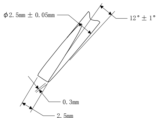
螺丝刀的形状 φ 2.5mm
