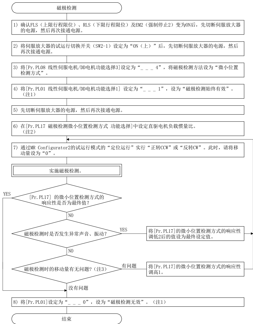
(b) 通过微小位置检测方式实施的磁极检测
