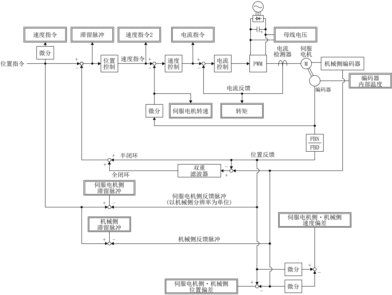
(b) 全闭环控制
