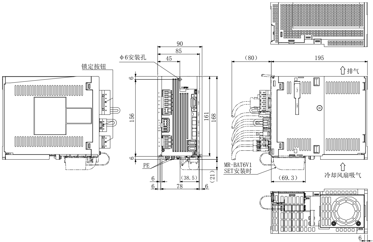
(d) MR-J4-200B (-RJ)
