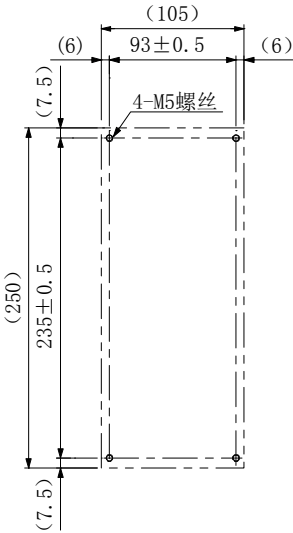
安装孔加工图
