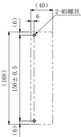
安装孔加工图
