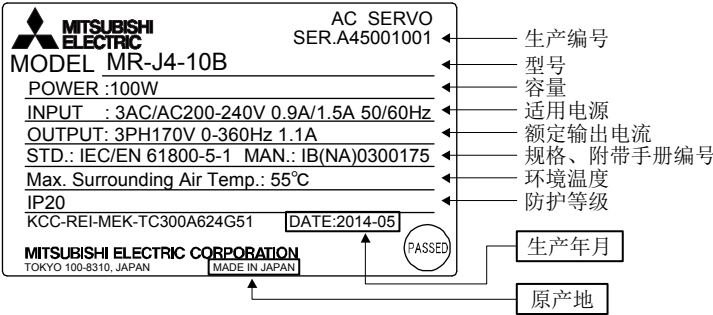
图附.3 识别原产地及生产月 额定铭牌的示例
