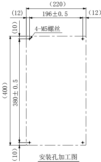
安装孔加工图
