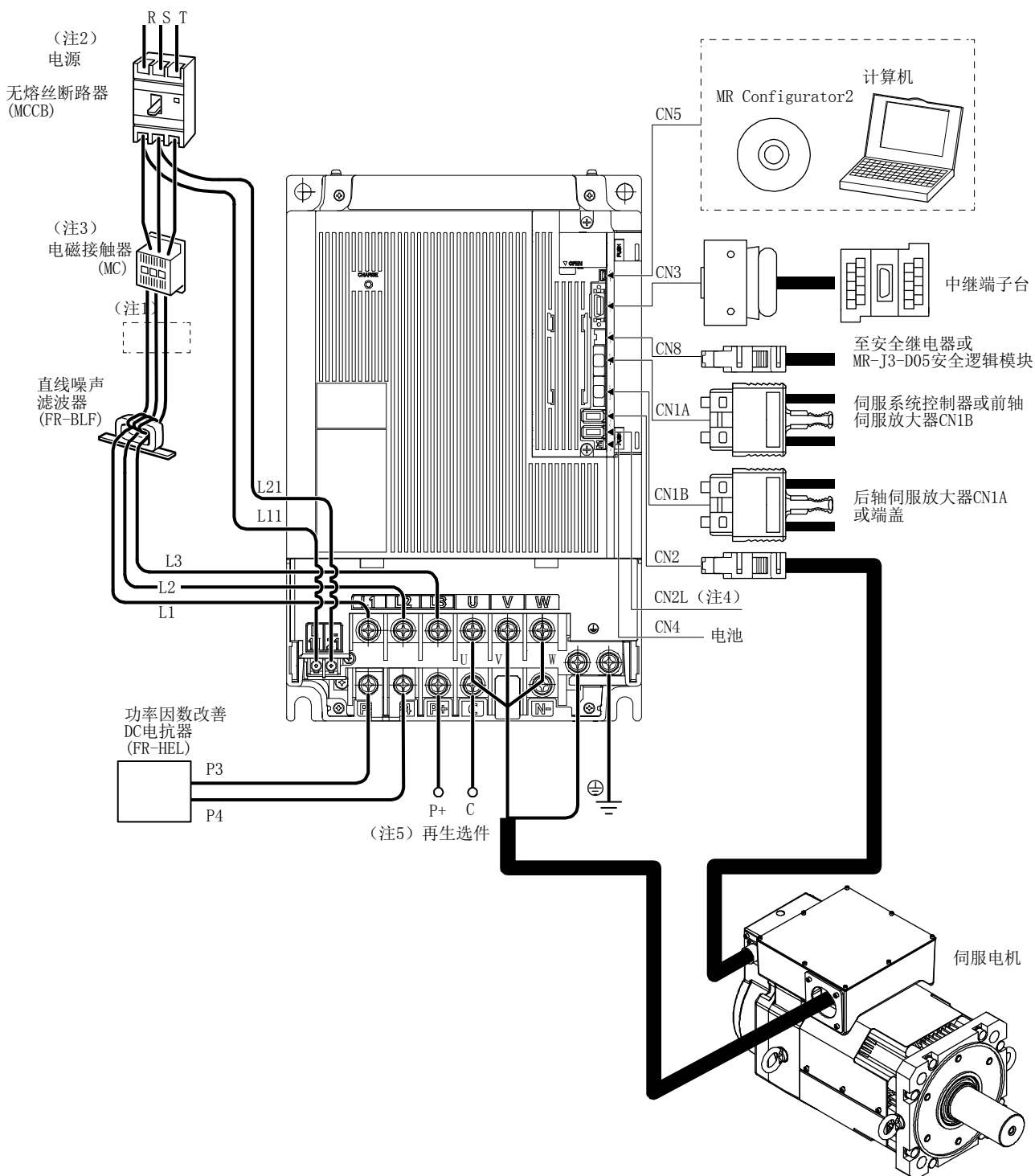
(f) MR-J4-22KB(-RJ)
