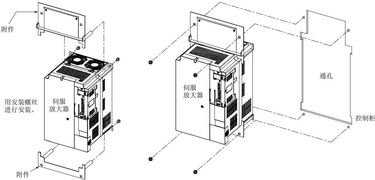
a. 散热片外装附件的安装方法
