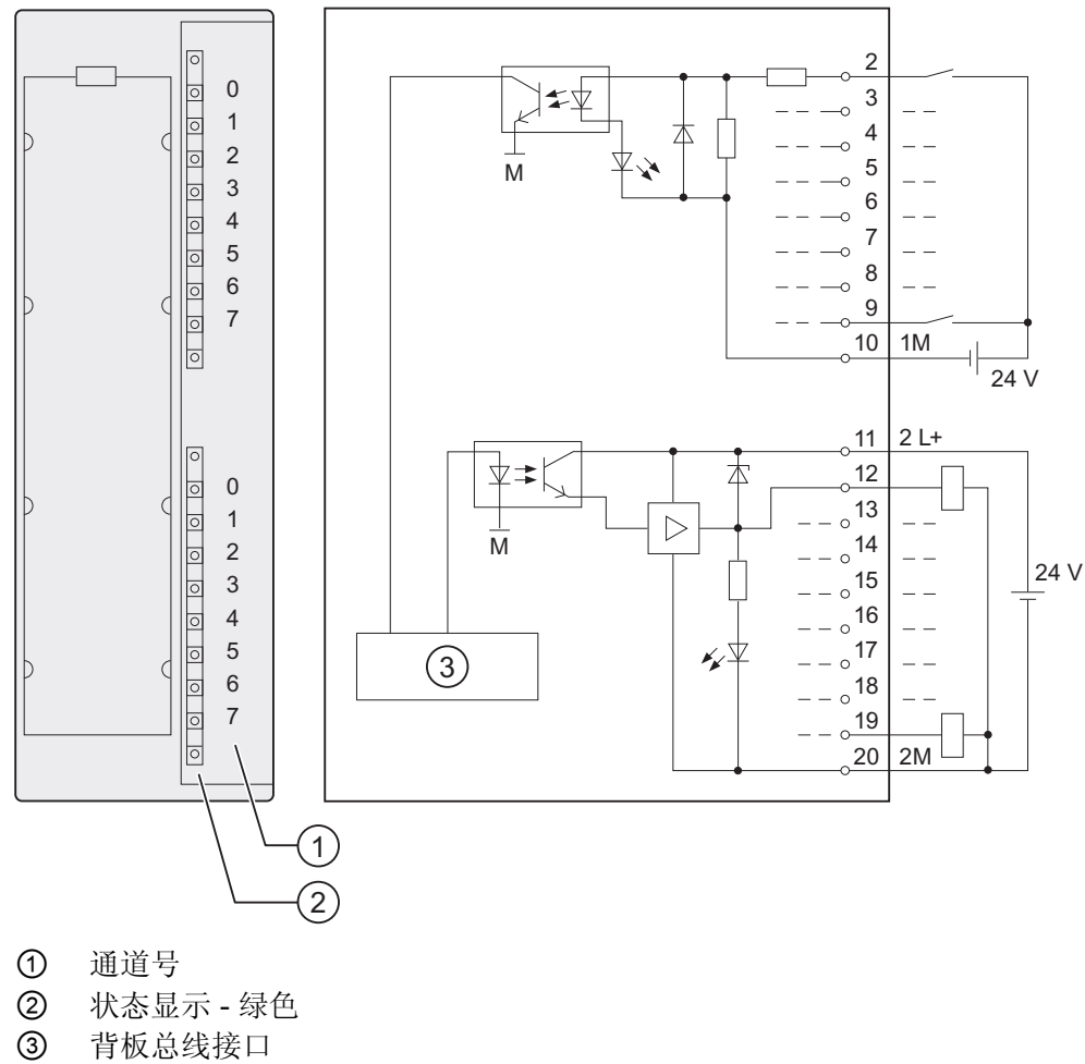
SM 323(DI 8/DO 8 x DC 24 V/0.5 A)的接线图和方框图
