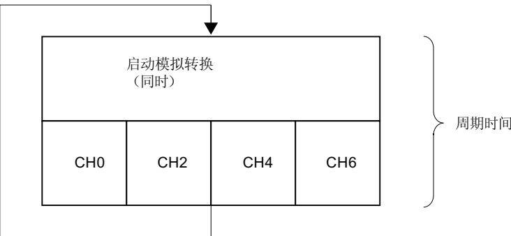
图 6-31 4 通道模式周期时间（硬件过滤器）
