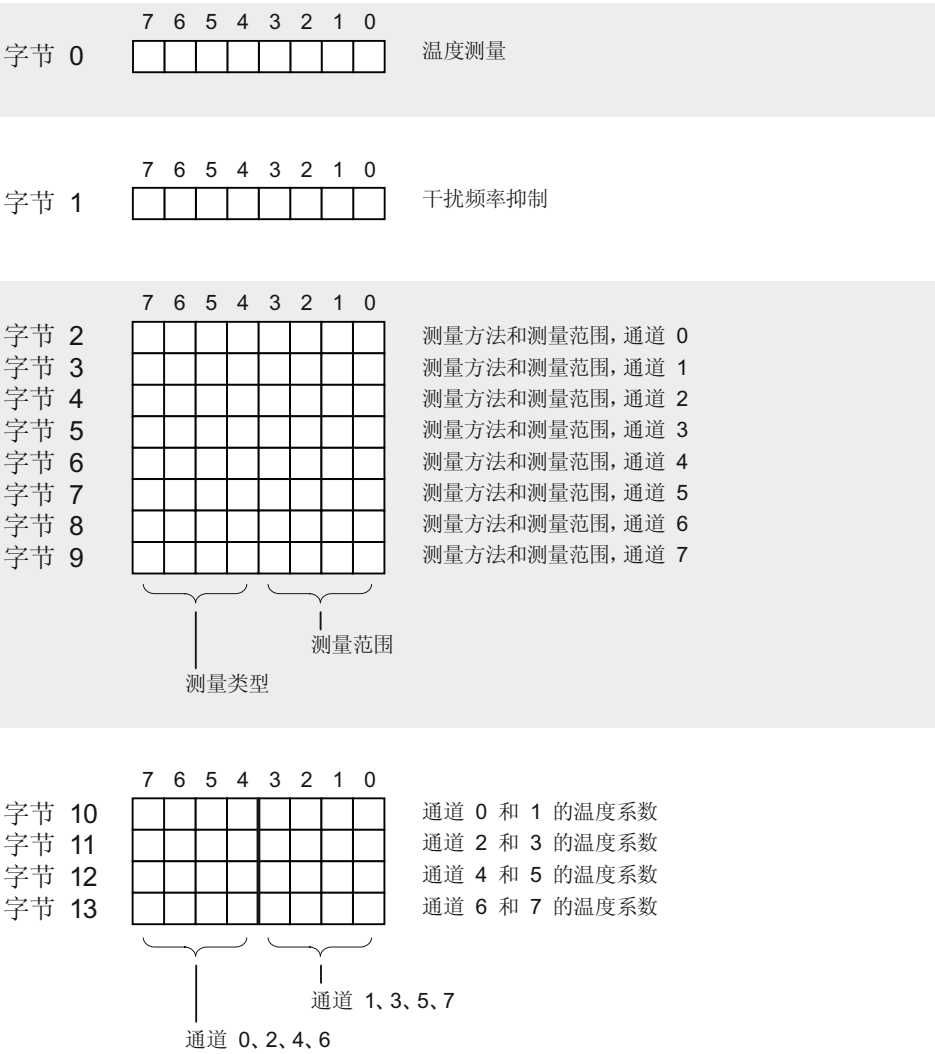
图 A-15 模拟量输入模块参数的数据记录 1
