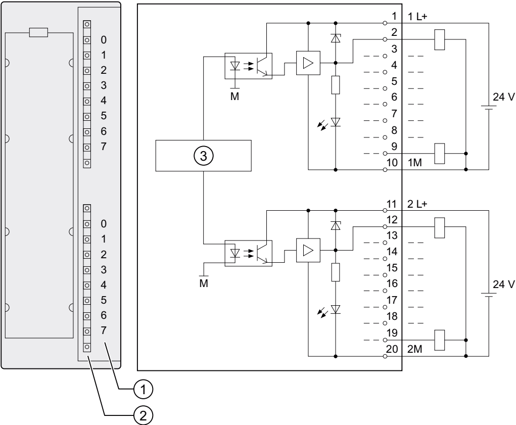
SM 322; DO 16 x DC 24 V/0.5 A 的接线图和方框图
