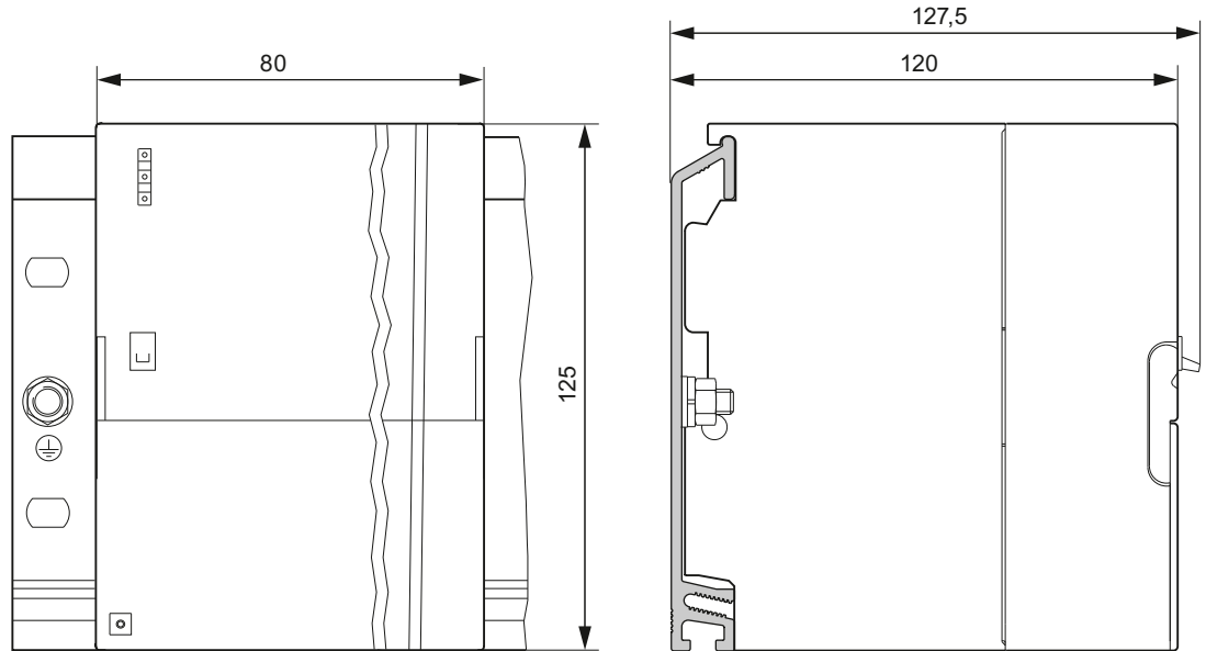
图 C-14 电源模块 PS 307；10 A
