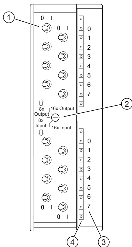
模块视图(没有前面板门)
