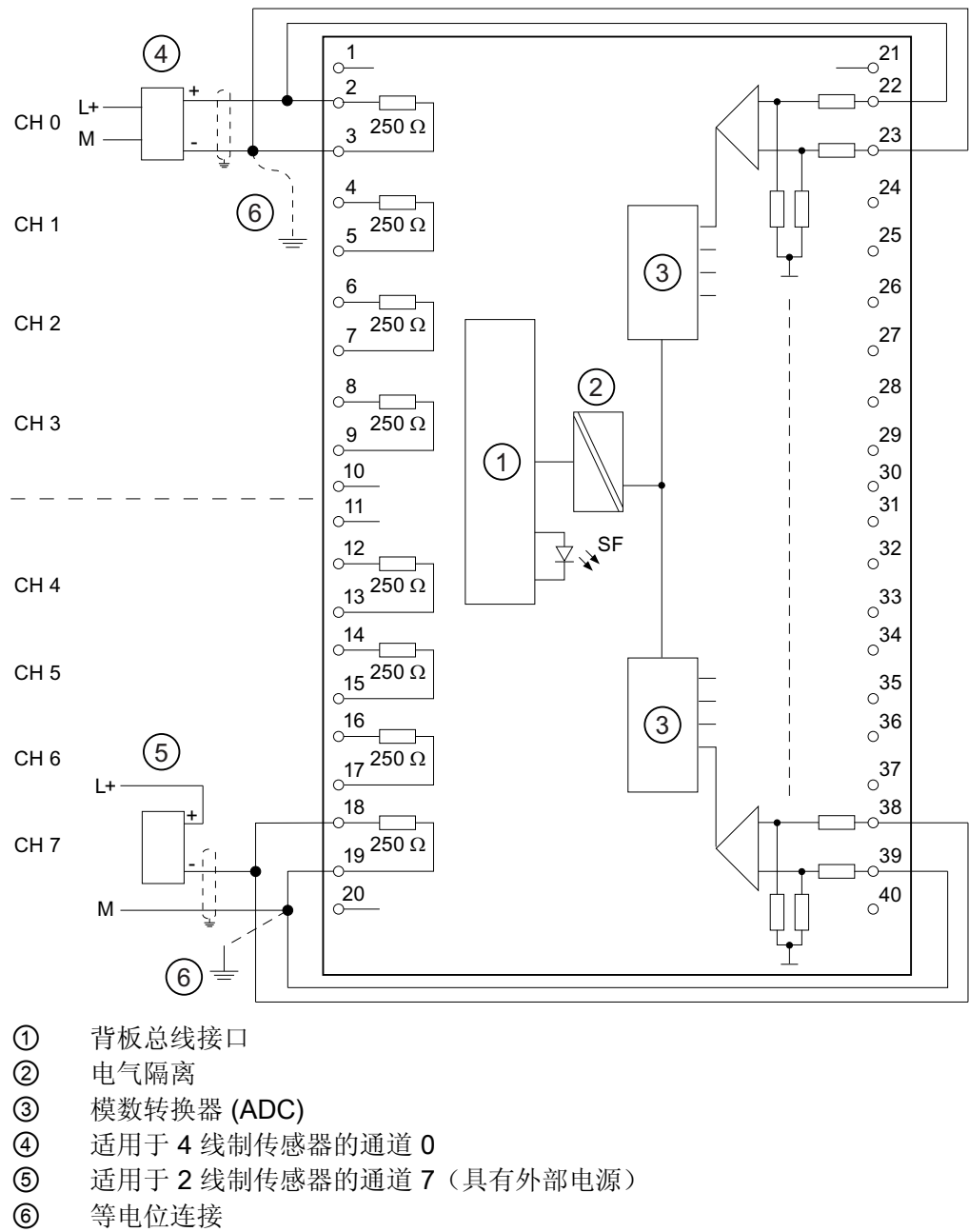
图 6-2 接线图和方框图
