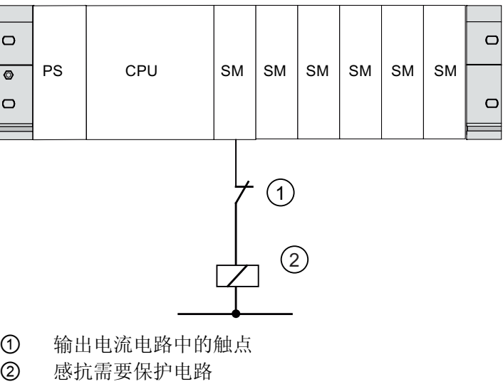
图 3-1 输出电流电路中用于急停的继电器触点
