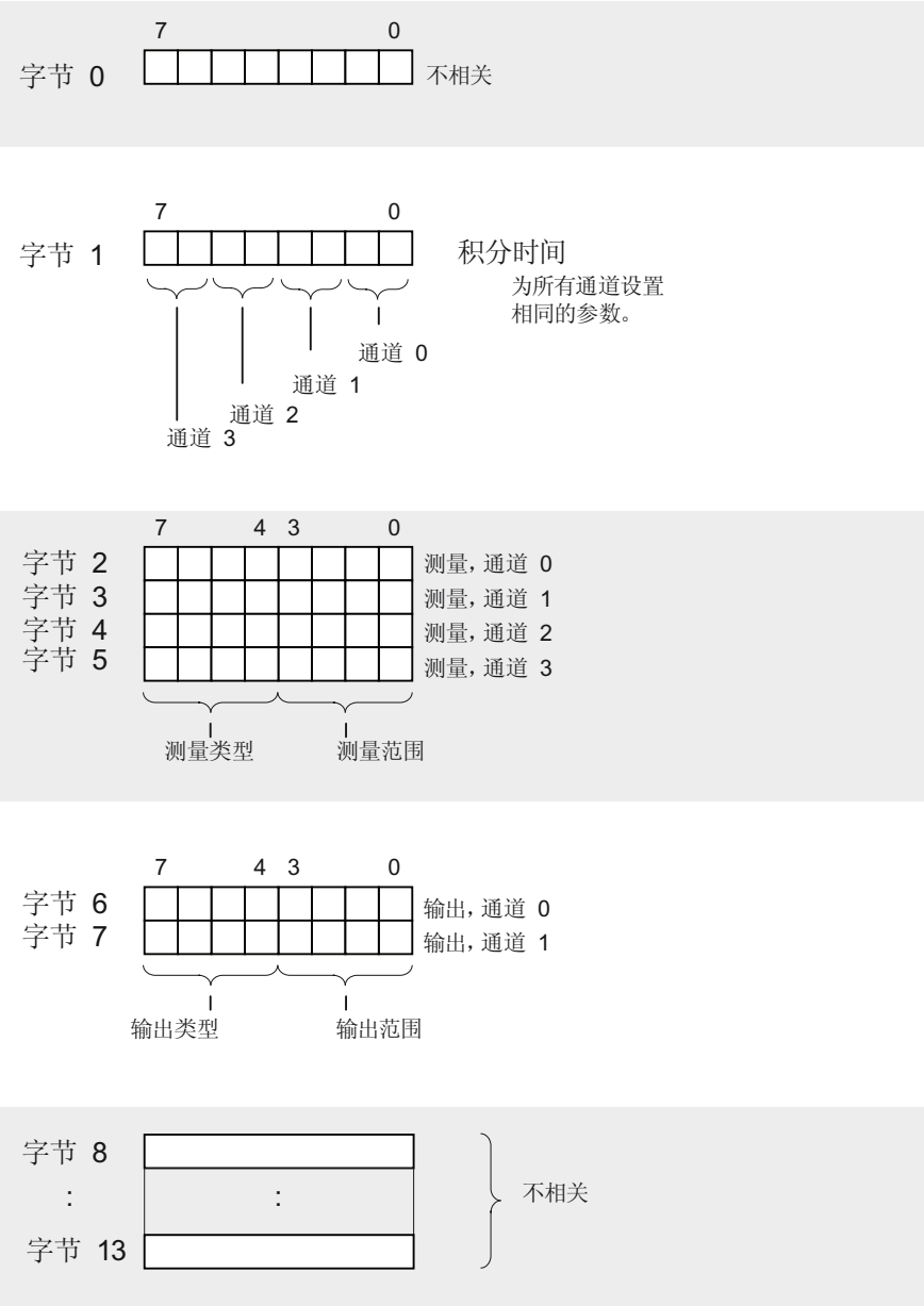
图 A-26 模拟量 IO 模块参数的数据记录 1
