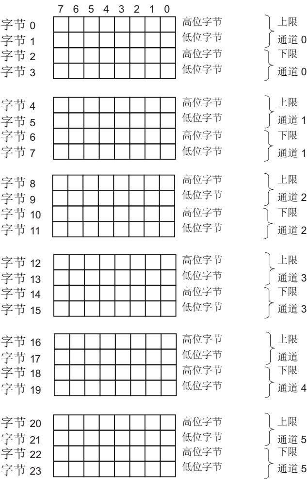
图 A-23 AI 6 x TC 的数据记录 128
