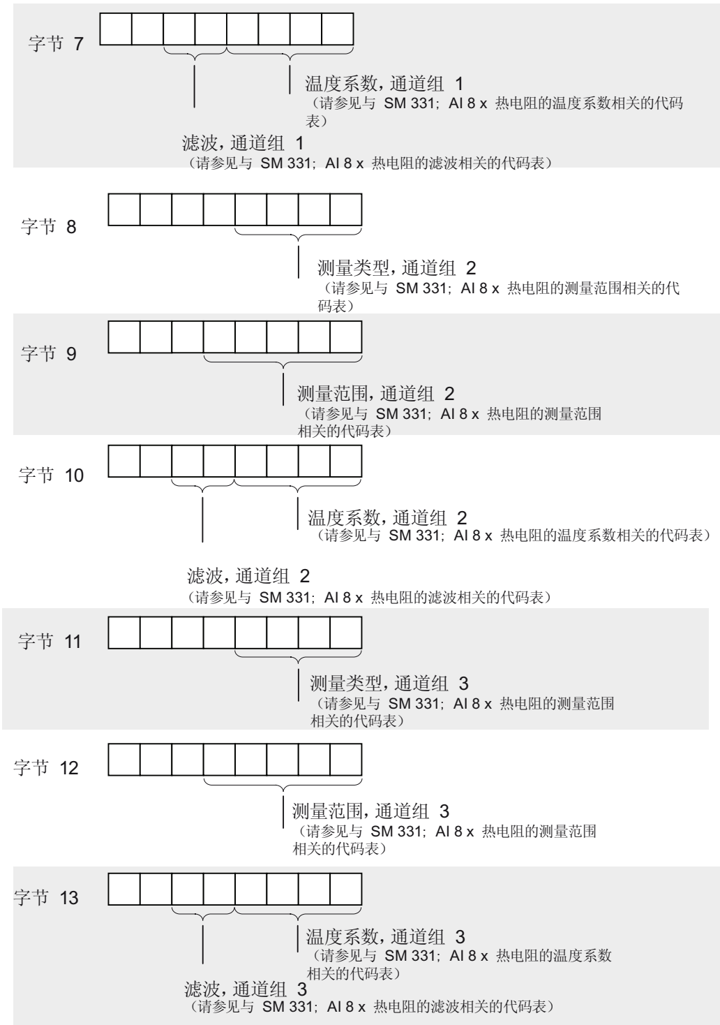
图 A-7 SM 331, AI 8 x RTD 的数据记录 128 (续)
