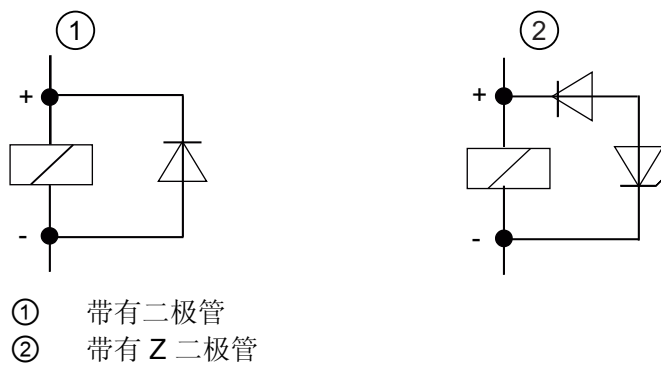
图 3-2 直流线圈的组态
