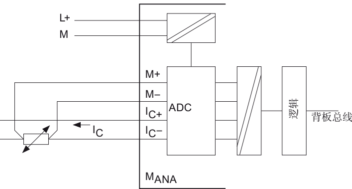
图 4-9 电阻温度计与电气隔离模拟量输入的 4 线制连接
