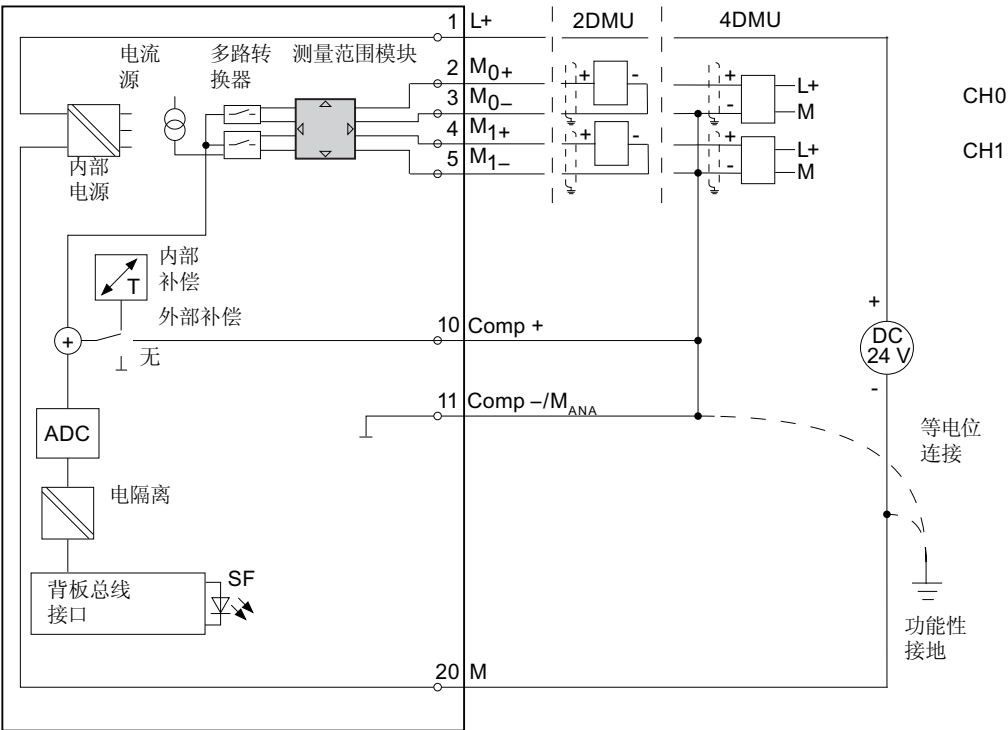
图 6-20 接线图和方框图
