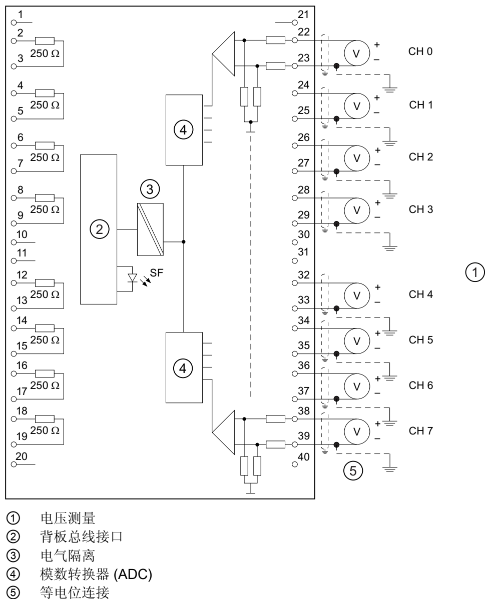
图 6-1 接线图和方框图
