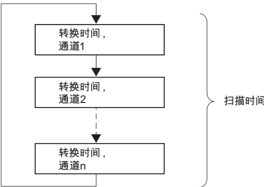
图 5-4 模拟量输入或输出模块的周期时间
