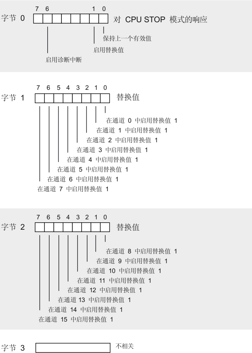
图 A-2 数字量输出模块参数的数据记录 1
