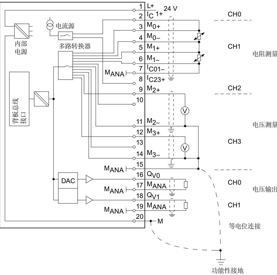
图 6-52 接线图和方框图
