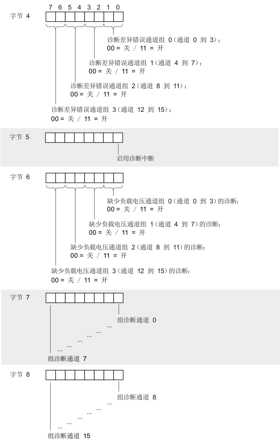
图 A-3 数据记录 1 的结构
