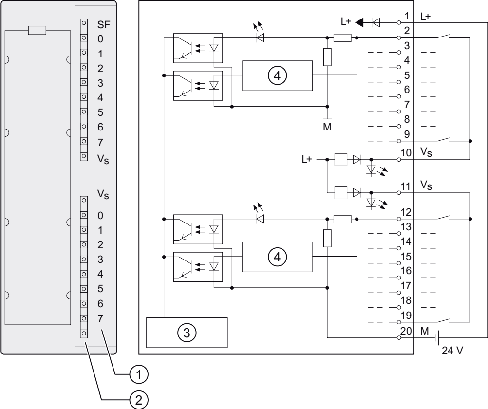
SM 321; DI 16 x DC 24 V 的接线图和方框图
