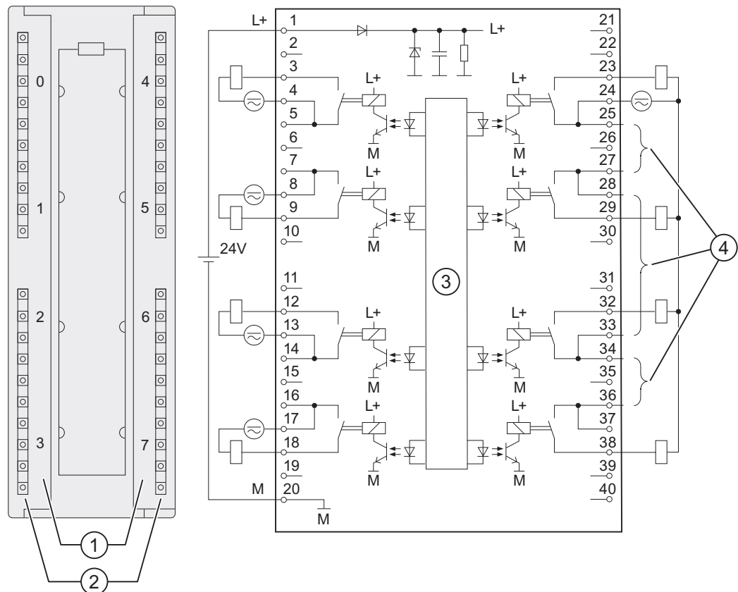
SM 322; DO 8 x Rel. AC 230 V/5 A 的接线图和方框图
