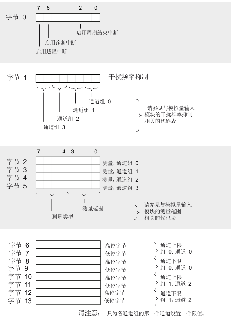
图 A-4 模拟量输入模块参数的数据记录 1
