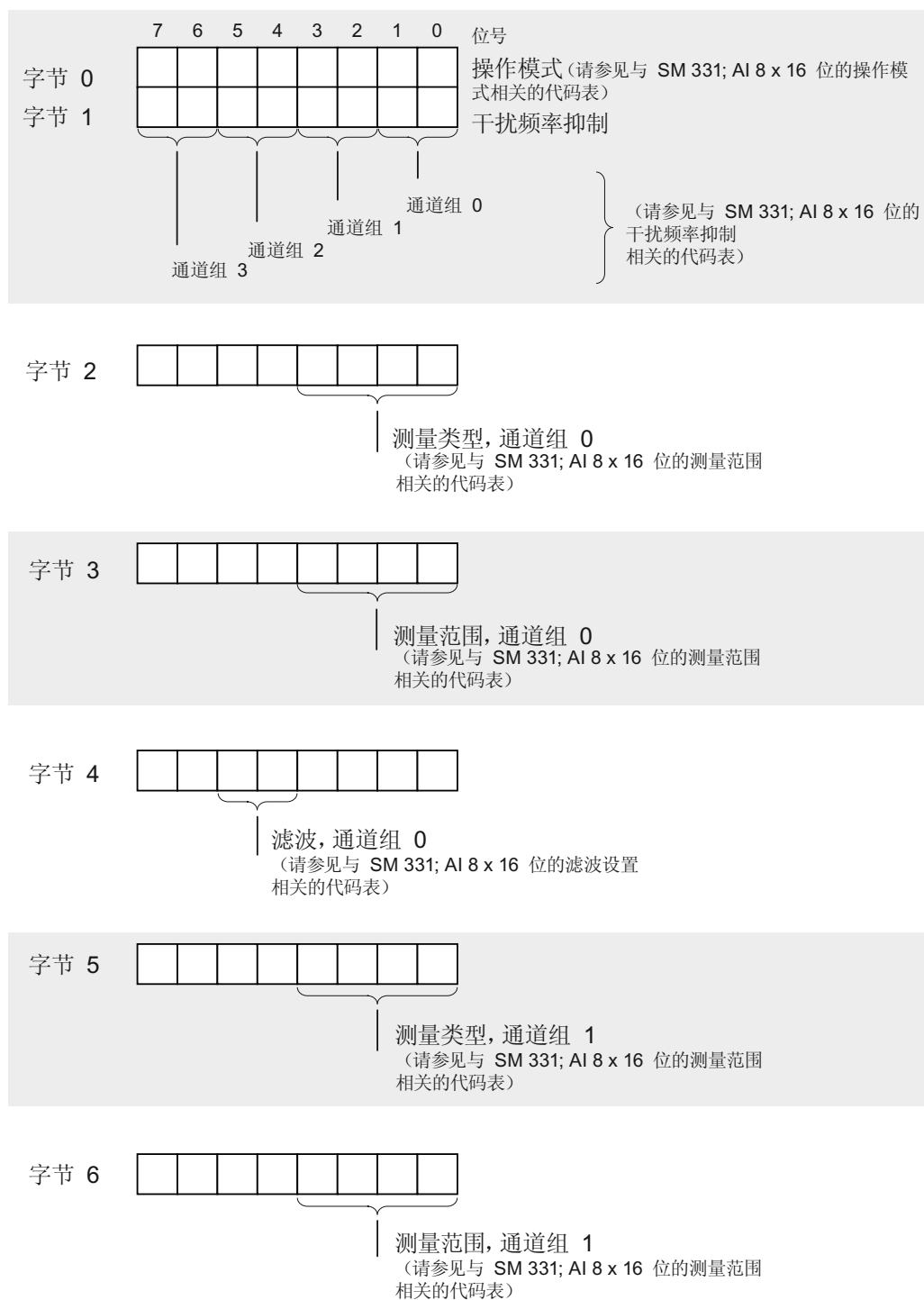
图 A-17 SM 331; AI 8 x 16 位参数的数据记录 128
