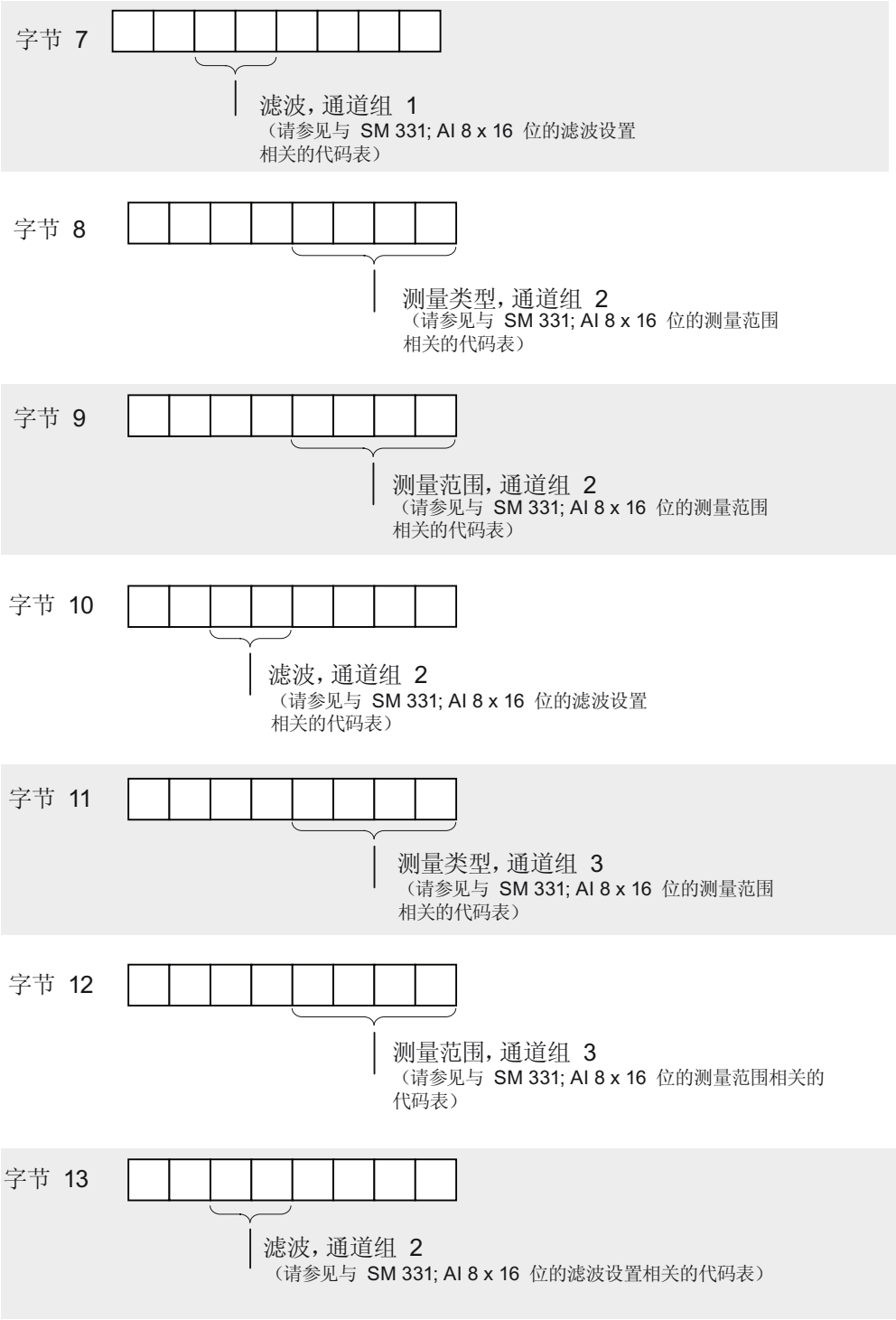
图 A-18 SM 331; AI 8 x 16 位参数的数据记录 128 (续)
