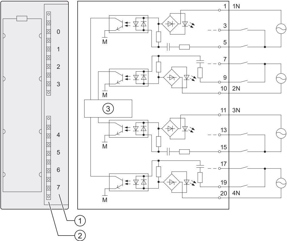
SM 321; DI 8 x AC 120/230 V 的接线图和方框图
