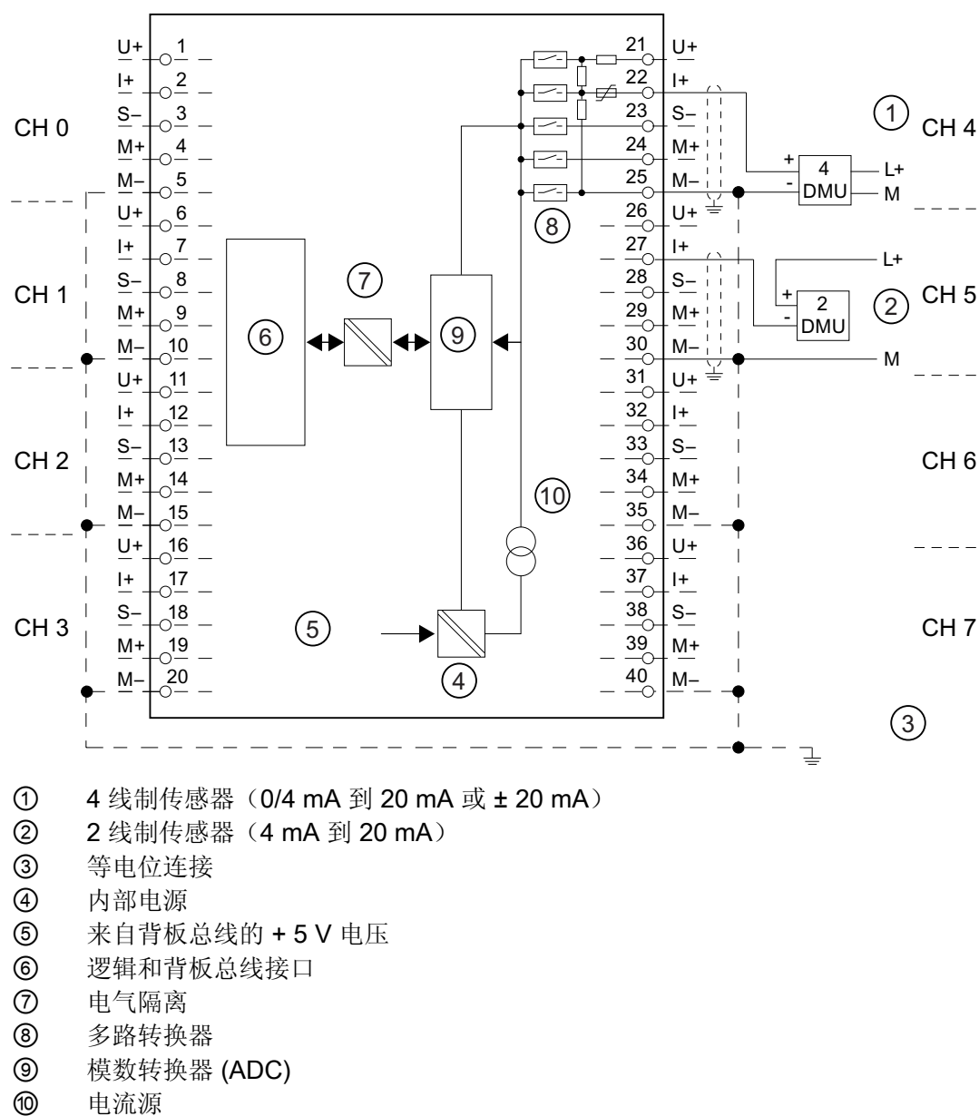
图 6-11 方框图和接线图
