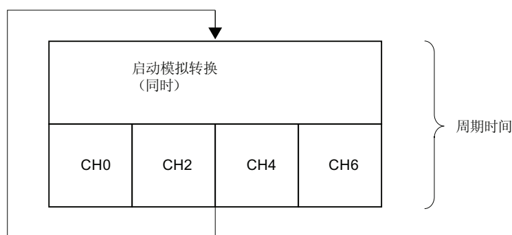
图 6-25 4 通道模式周期时间（硬件过滤器）
