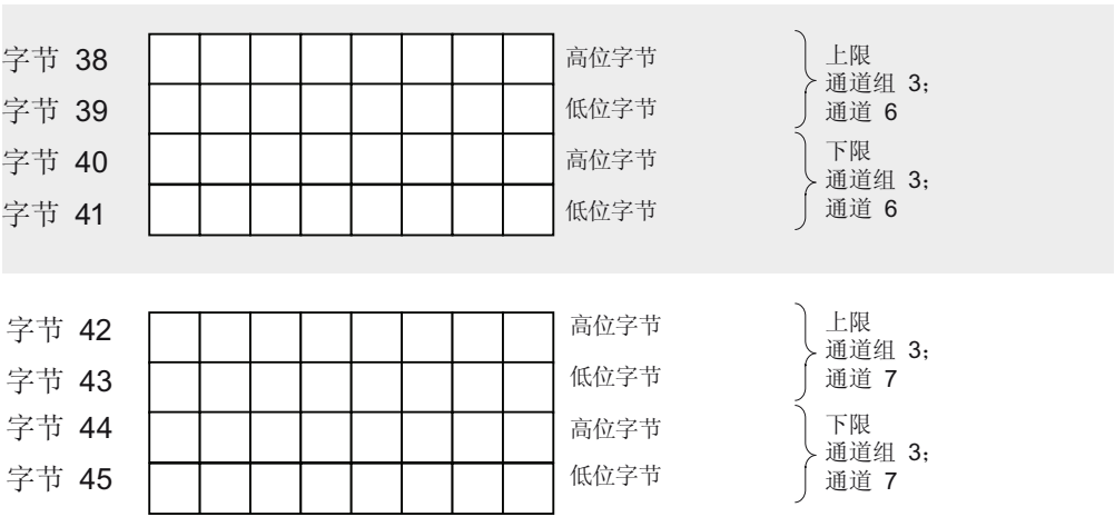
图 A-20 SM 331; AI 8 x 16 位参数的数据记录 128 (续 )
