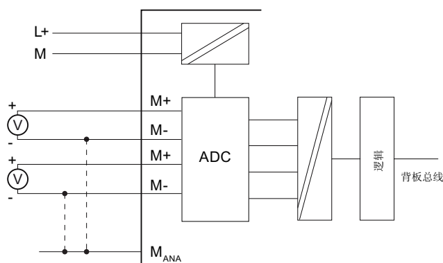
图 4-5 对电压传感器接线，并连接到电气隔离 AI
