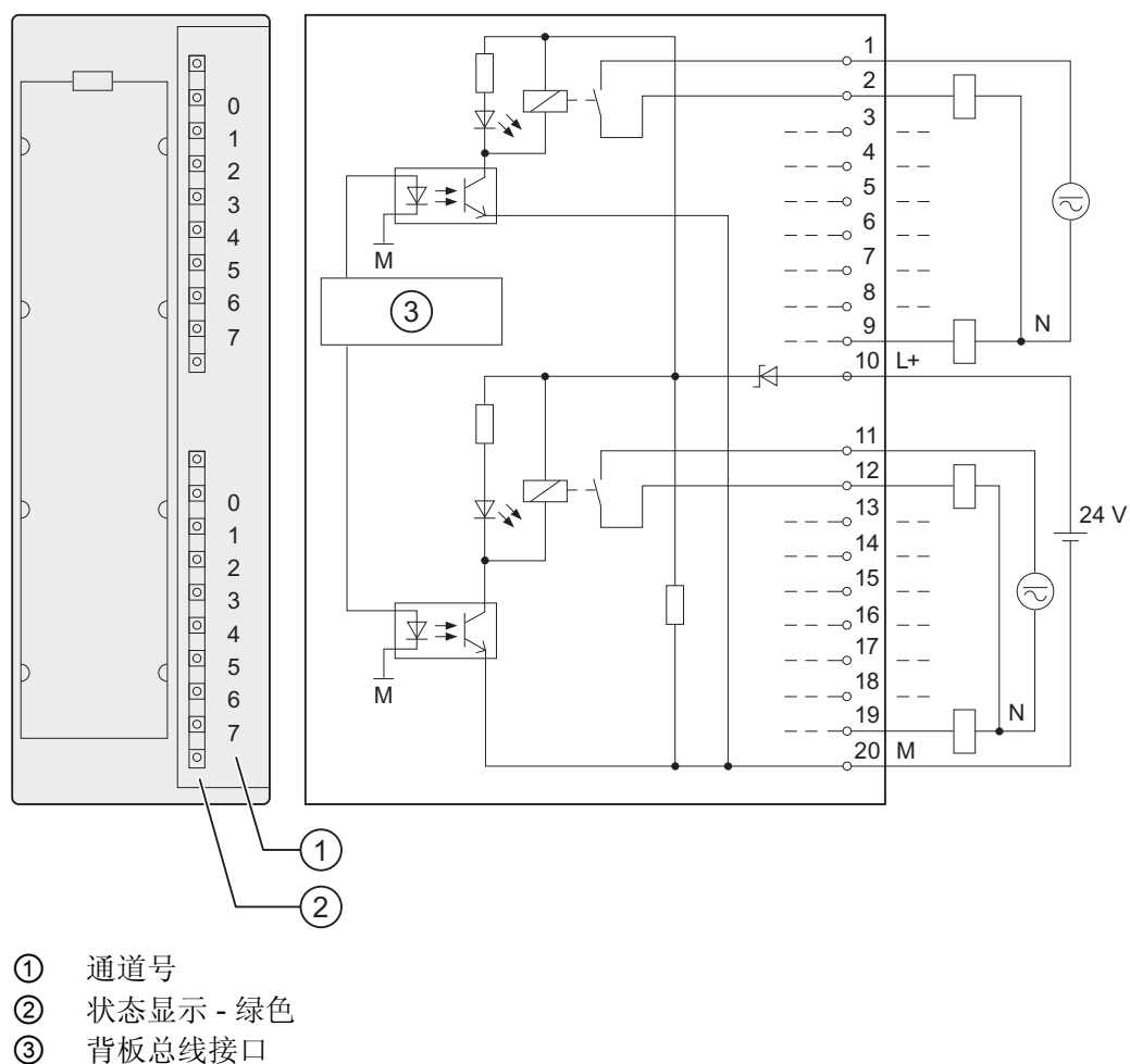
SM 322; DO 16 x Rel. AC 120/230 V 的接线图和方框图
