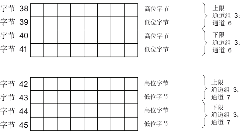
图 A-14 SM 331,AI 8 TC 的数据记录 128（续）
