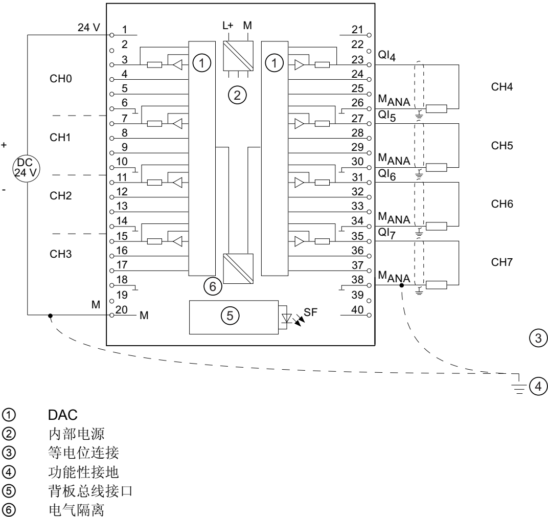
图 6-42 接线图和方框图
