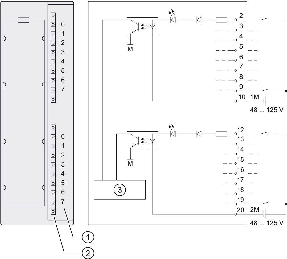
SM 321; DI 16 x DC 48-125 V 的接线图和方框图
