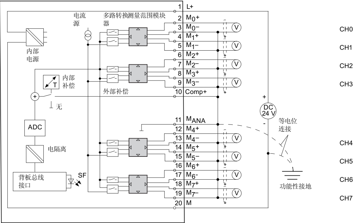
图 6-13 方框图和接线图
