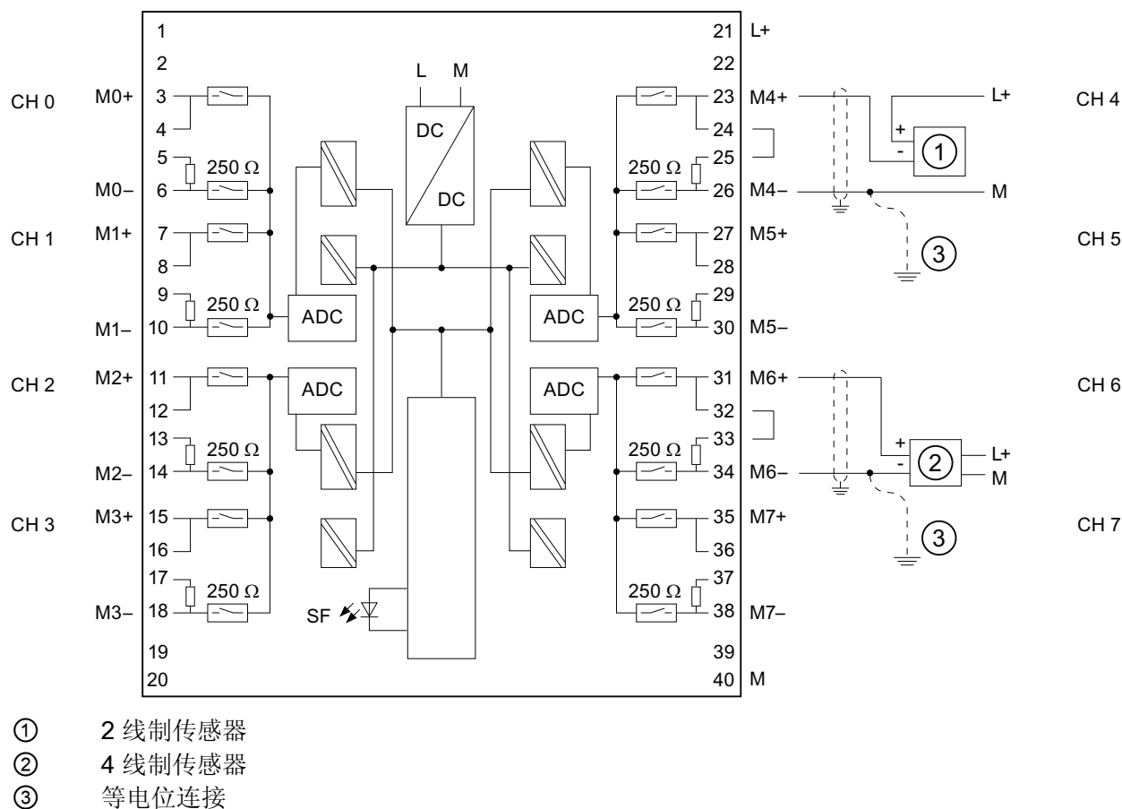
图 6-4 接线图和方框图
