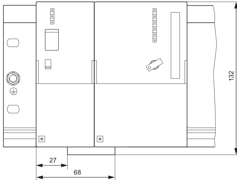
图 C-12 带有 CPU 313/314/315/315-2 DP 和电源模块 PS 307; 10 A 的尺寸图（正视图）
