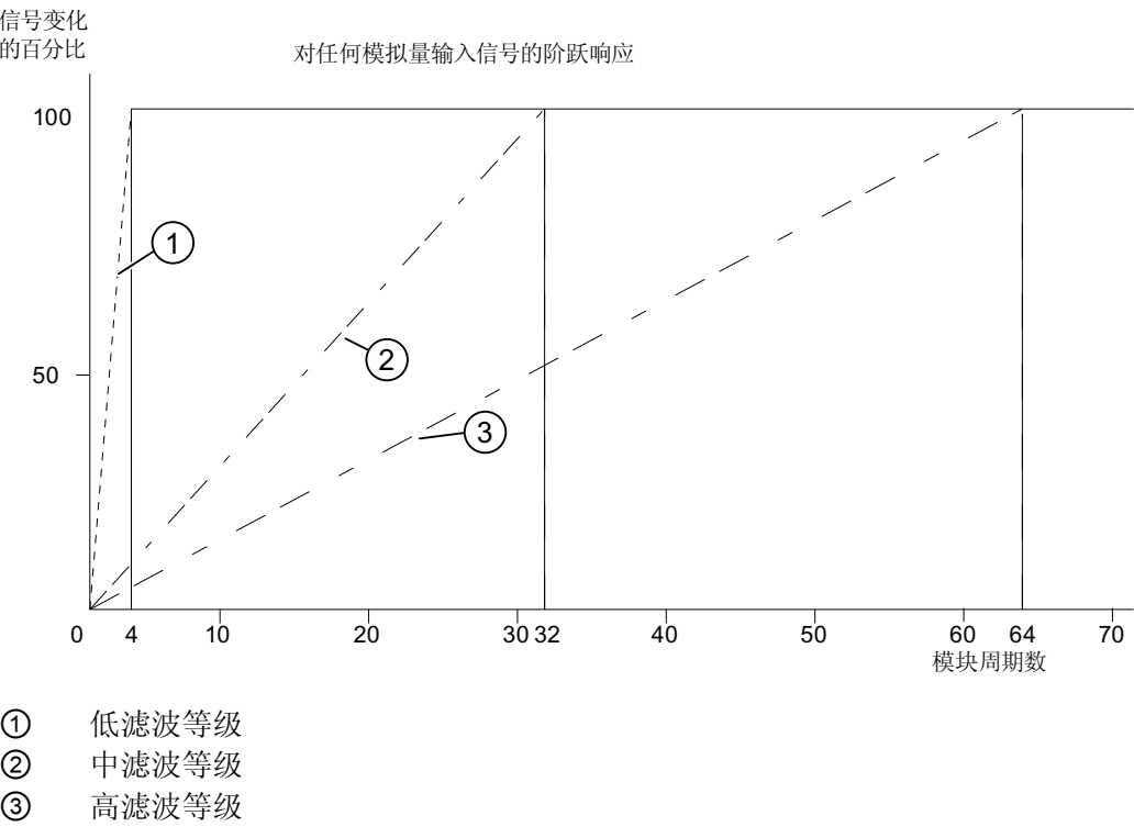
图 5-5 滤波对跳转响应的影响实例（AI 8 x 14 位）
