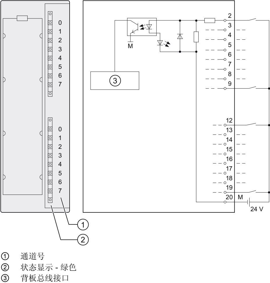
SM 321; DI 16 x DC 24 V 高速模块的接线图和方框图
