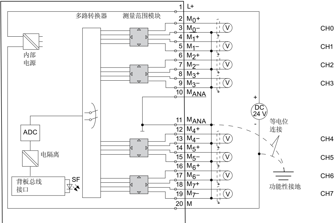
图 6-7 方框图和接线图
