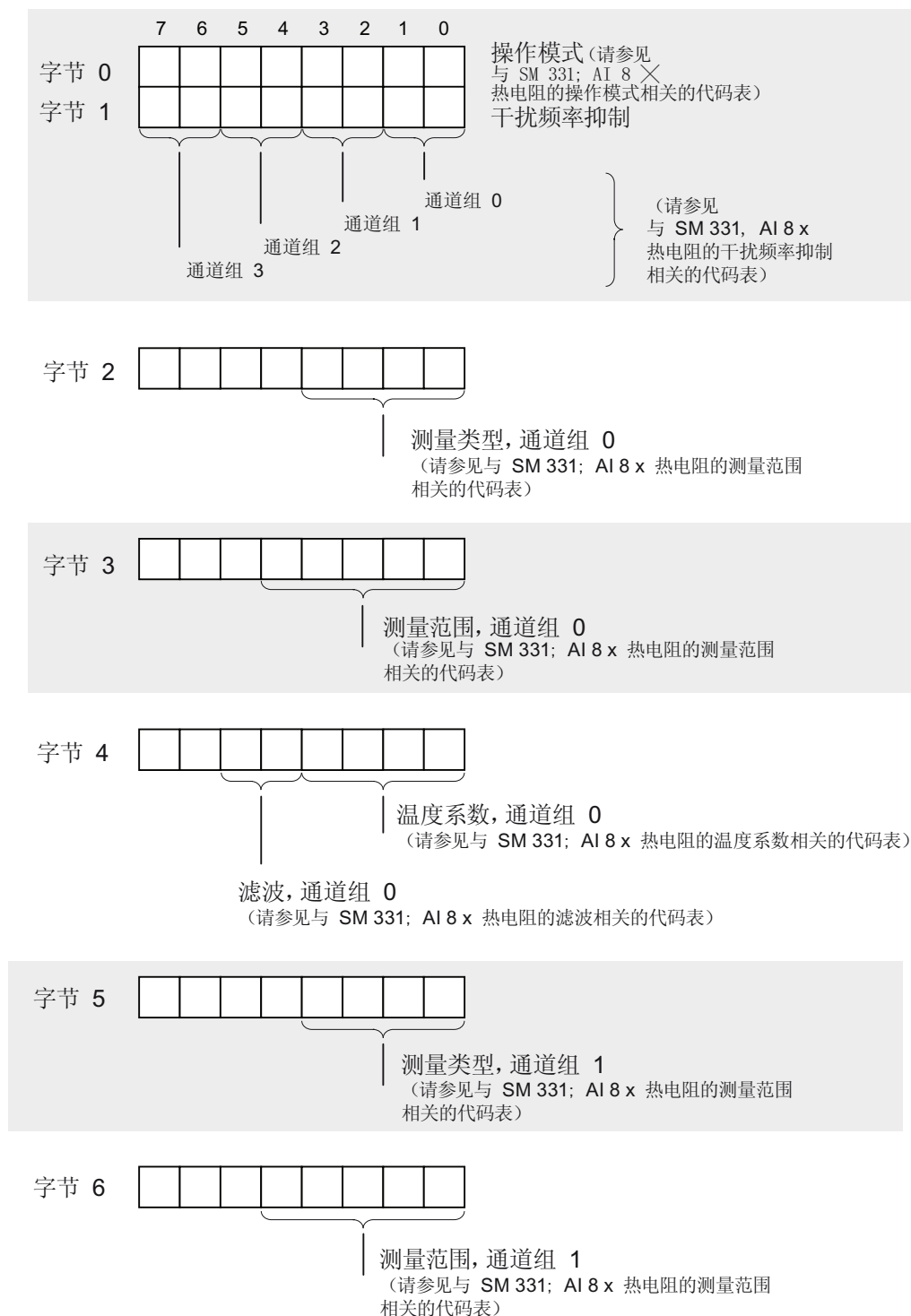
图 A-6 SM 331, AI 8 x RTD 的数据记录 128
