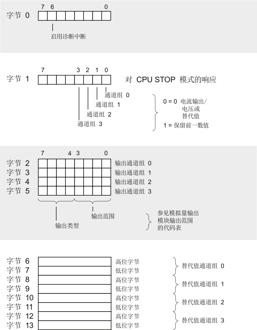
图 A-24 模拟量输出模块参数的数据记录 1
