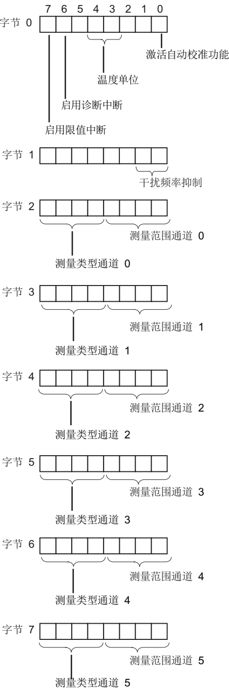
图 A-21 AI 6 x TC 的数据记录 1 的结构
