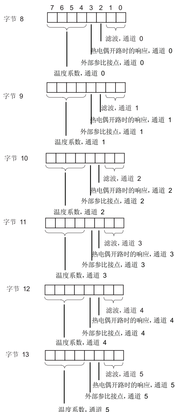
图 A-22 AI 6 x TC 的数据记录 1 的结构 (续)
