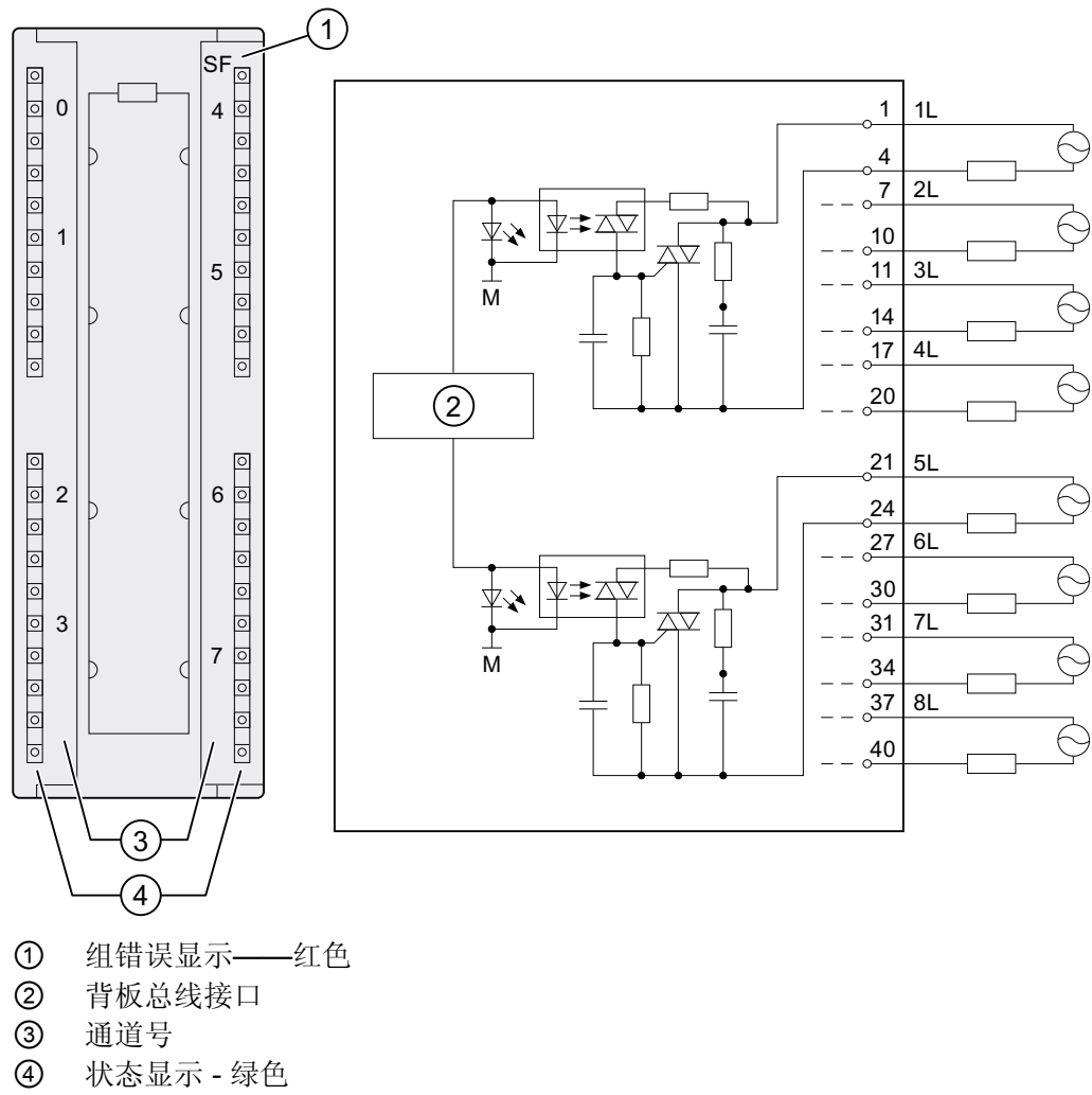
SM 322; DO 8 x AC 120/230 V/2 A ISOL 的接线图和方框图
