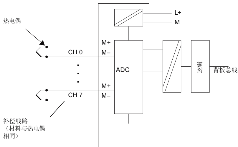
图 4-14 对带内部补偿的热电偶进行接线，并连接到电气隔离模拟量输入
