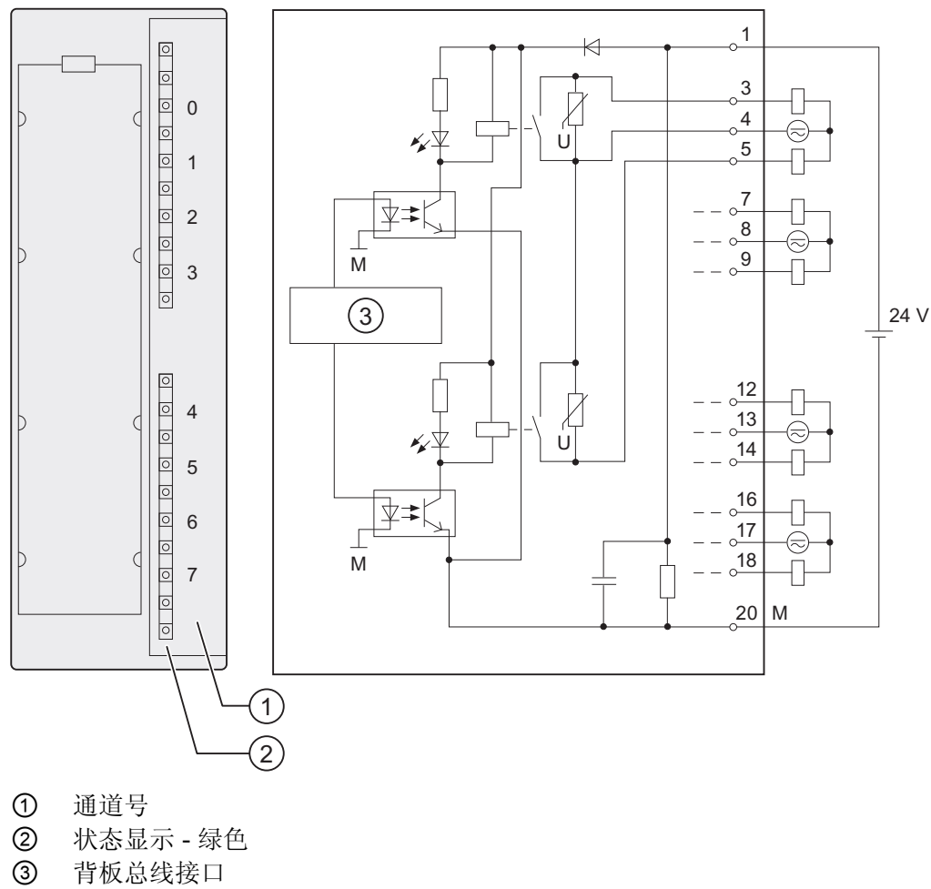
SM 322; DO 8 x Rel. AC 230 V 的接线图和方框图
