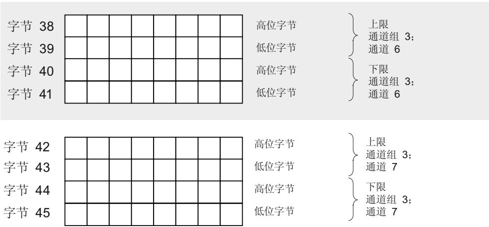
图 A-9 SM 331, AI 8 x RTD 的数据记录 128 (续 )
