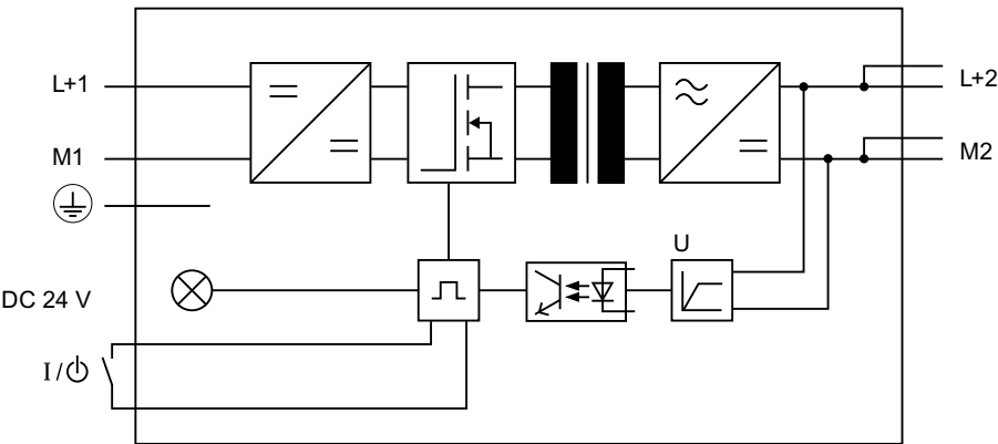
图 2-4 电源模块 PS 305; 2 A 的电路示意图
