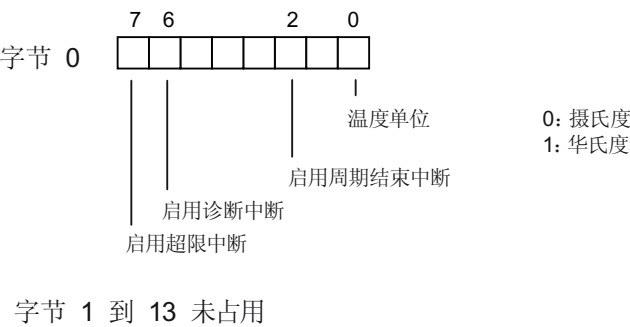
图 A-10 SM 331, AI 8 x TC 参数的数据记录 1
