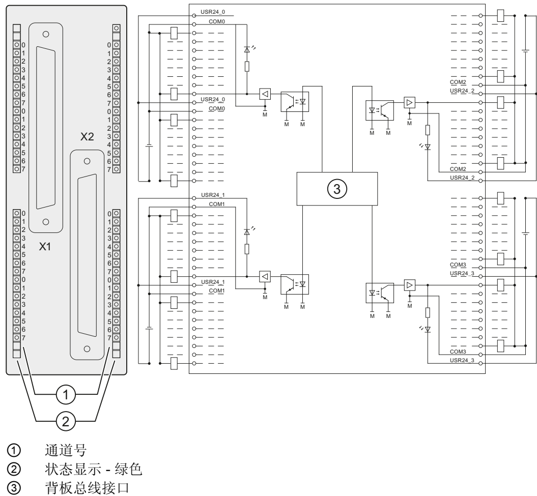
SM 322; DO 64 x DC 24 V/0,3 A Sourcing 的接线图和方框图
