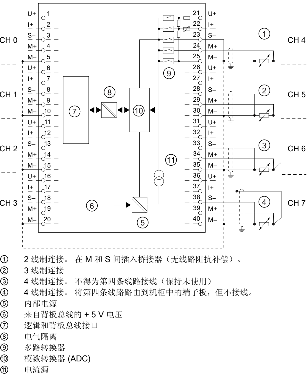
图 6-12 方框图和端子图
