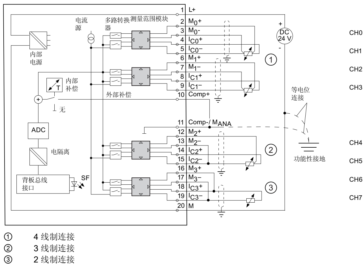
图 6-15 方框图和端子图
