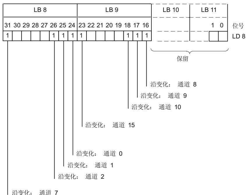
图 3-6 OB40 的启动信息：哪个事件触发了硬件中断
