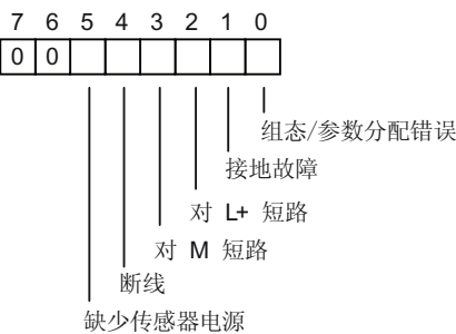
图 B-5 SM 321, DI 16 x DC 24 V 的数字量输入通道的诊断字节
