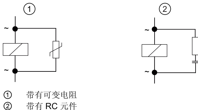
图 3-3 交流线圈的连接
