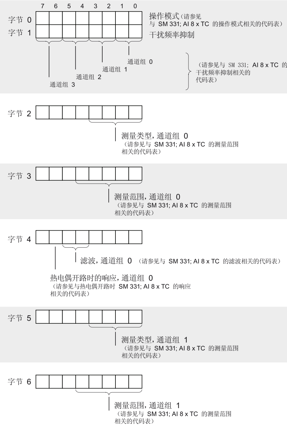
图 A-11 图 A-10 SM 331, AI 8 x TC 的数据记录 128 (续)
