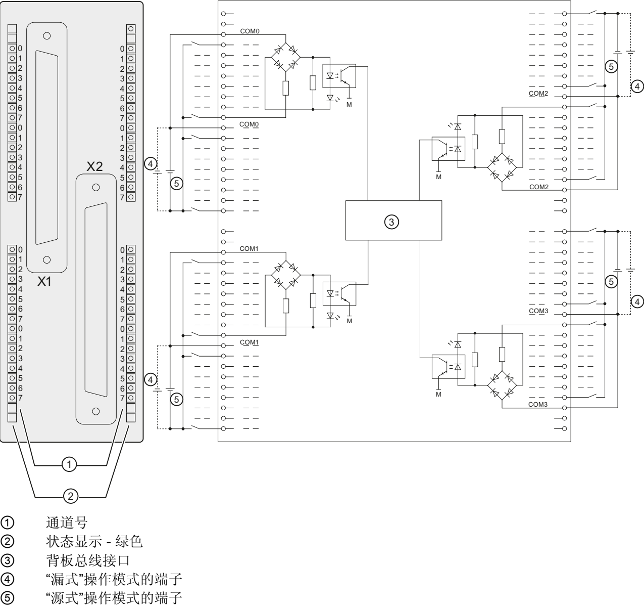
SM 321; DI 64 x DC 24 V, Sinking/Sourcing 的接线图和方框图
