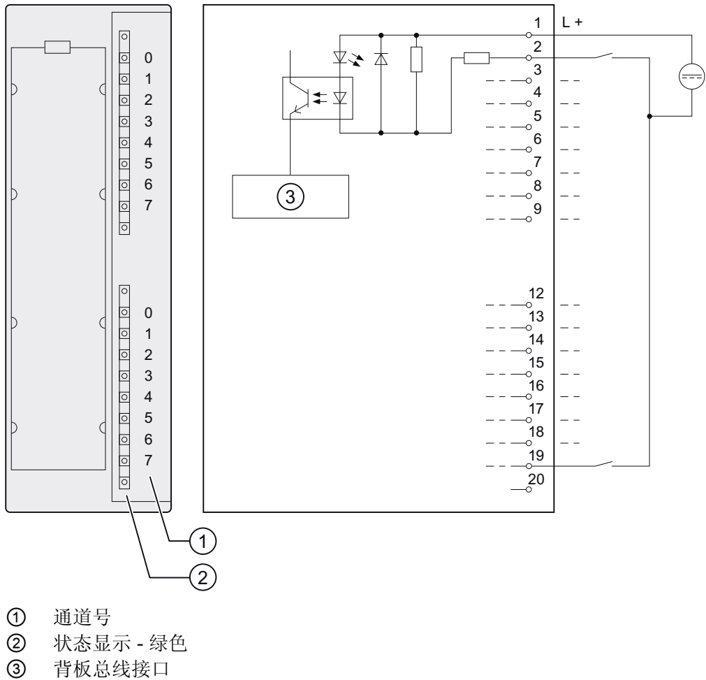
SM 321; DI 16 x DC 24 V 的接线图和方框图
