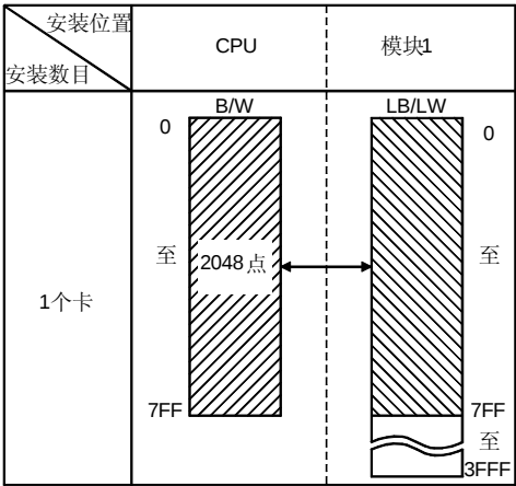
(b) Q00J/Q00/Q01CPU
