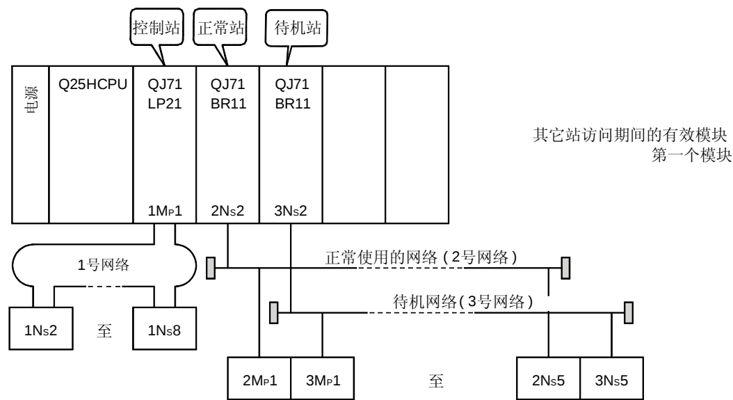
[系统配置]
