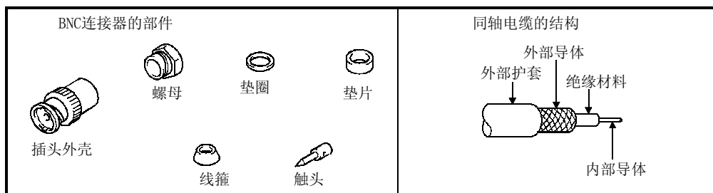
图 3.1 BNC 连接器和同轴电缆的结构
