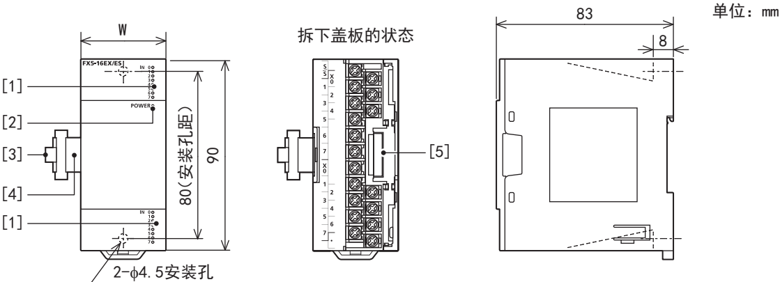
外形尺寸
