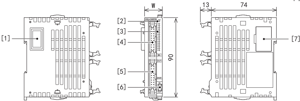
外形尺寸
