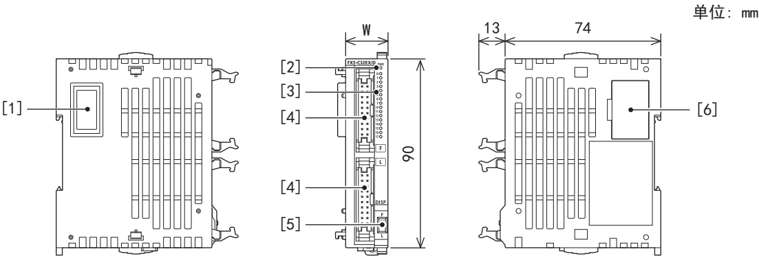
外形尺寸
