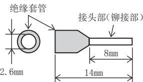
带绝缘套管的棒状端子的外形图
