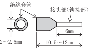
带绝缘套管的棒状端子的外形图
