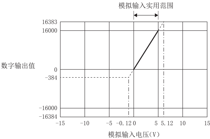
■电压输入特性图（1～5V）
