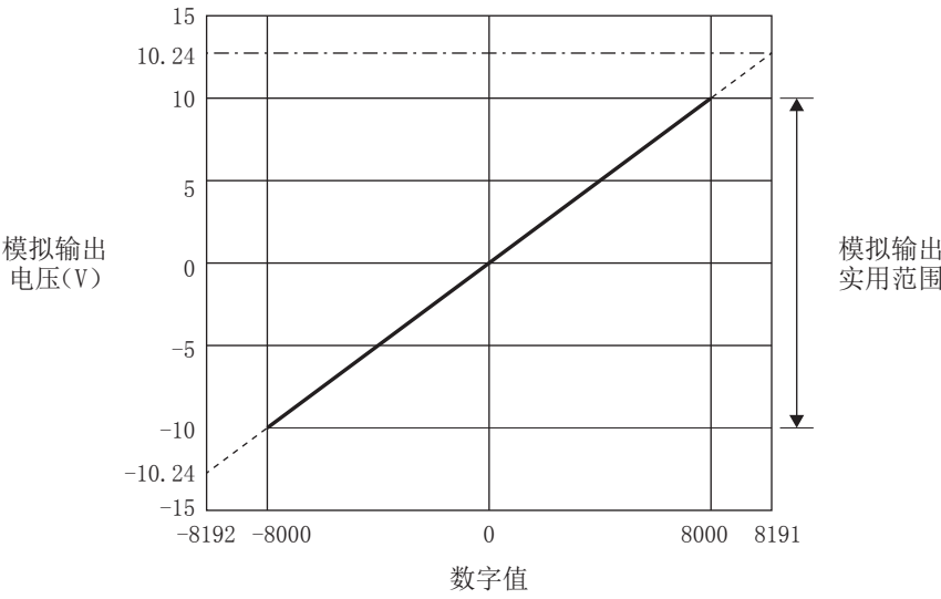
■电压输出特性图（-10~+10V）
