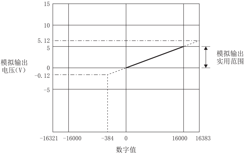
■电压输出特性图（1~5V）
