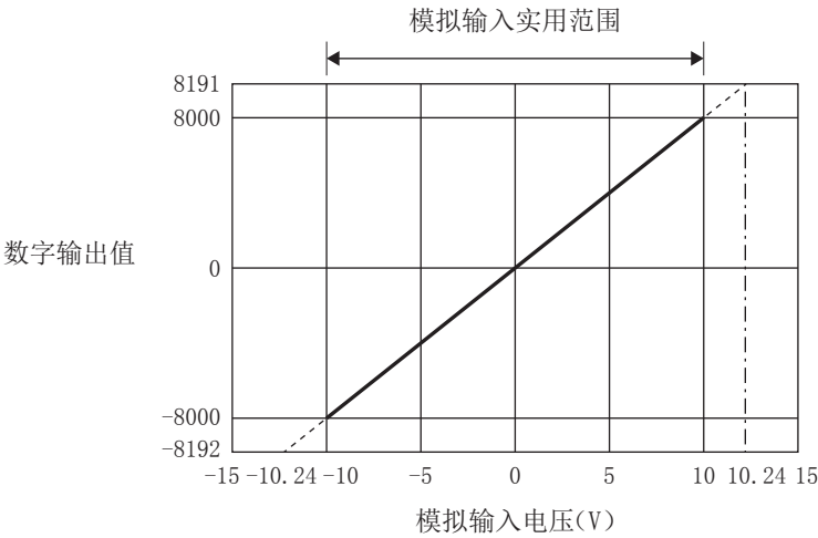
■电压输入特性图（-10～+10V）
